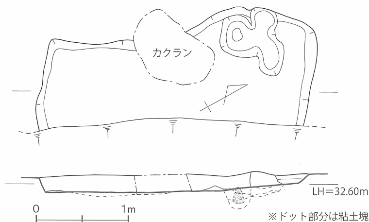
第 7 図 10号竪穴式住居 実測図 [1/40]
