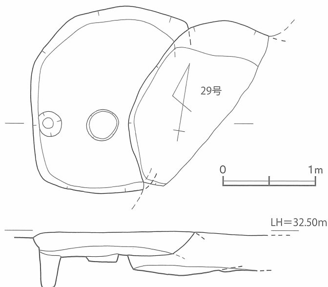
第32図 46号貯蔵穴 実測図〔1/40〕
