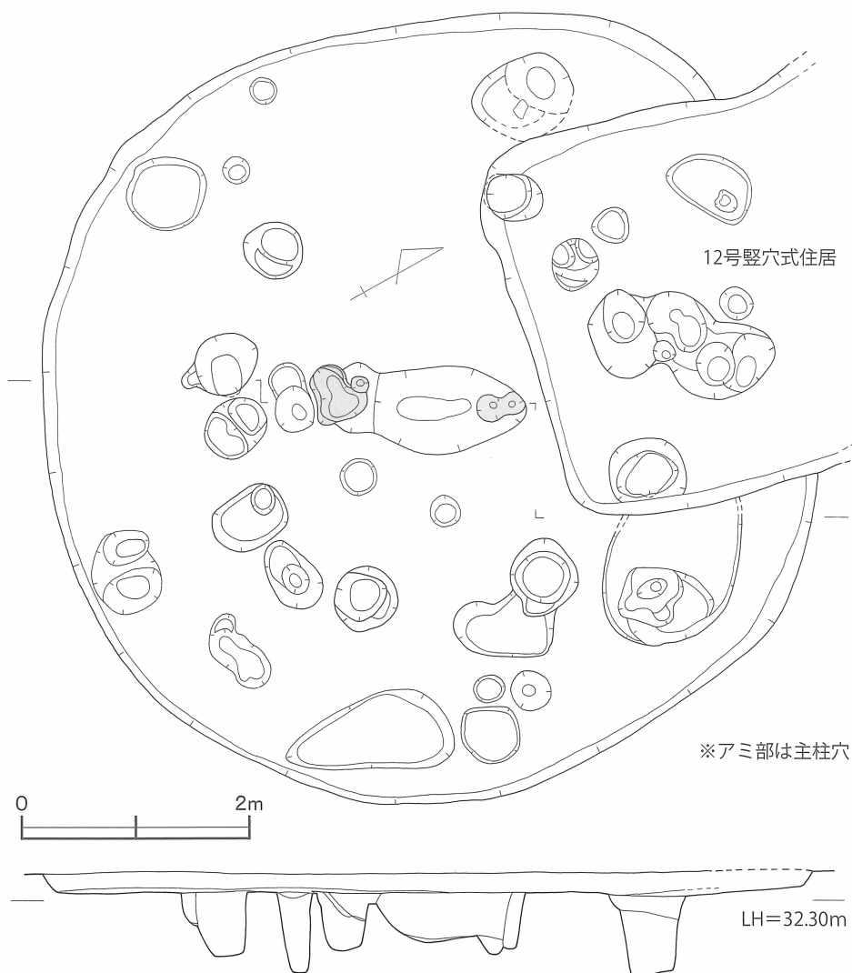
第30図 13号竪穴式住居 実測図 [1/60]
