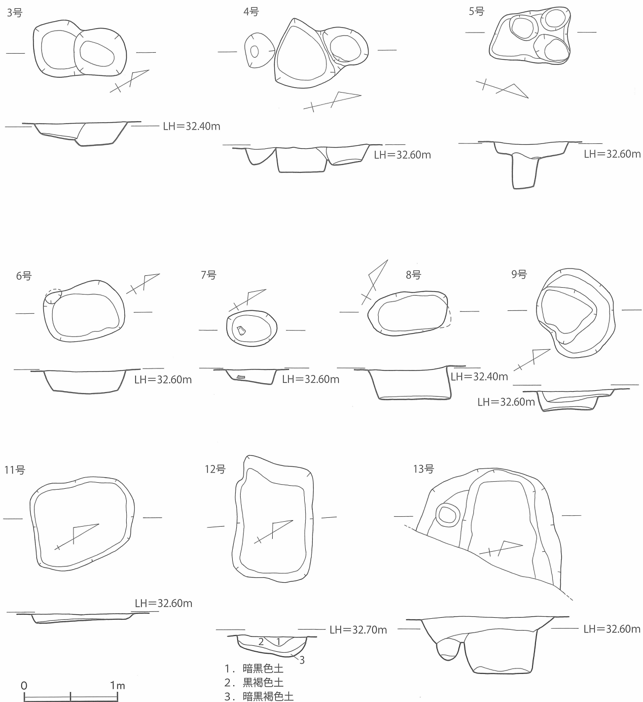
第20図 3～9・11～13号土坑 実測図 [1/40]
