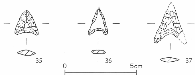
第26図 室岡・山ノ上遺跡2次調査 出土石鏃 実測図〔2/3〕
