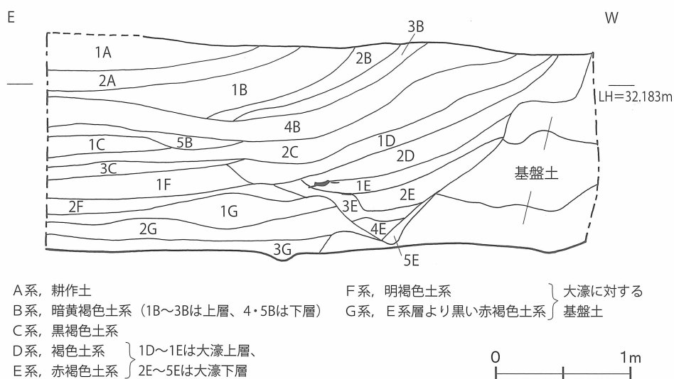
第21図 大濠土層断面 実測図 [1/40]
