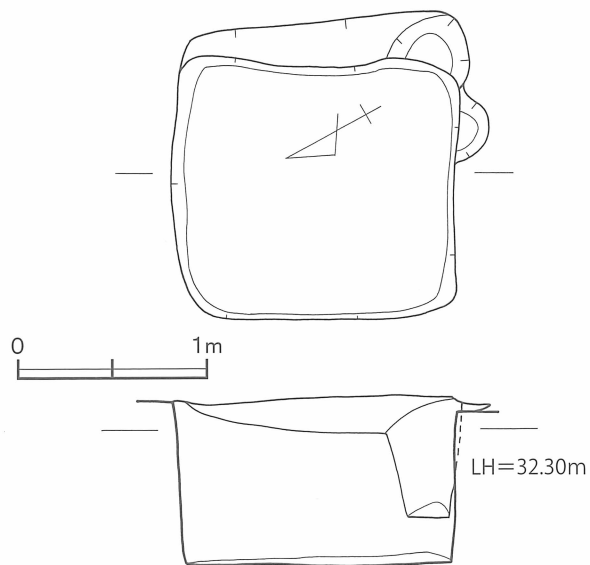
第34図 53号貯蔵穴 実測図 [1/40]
