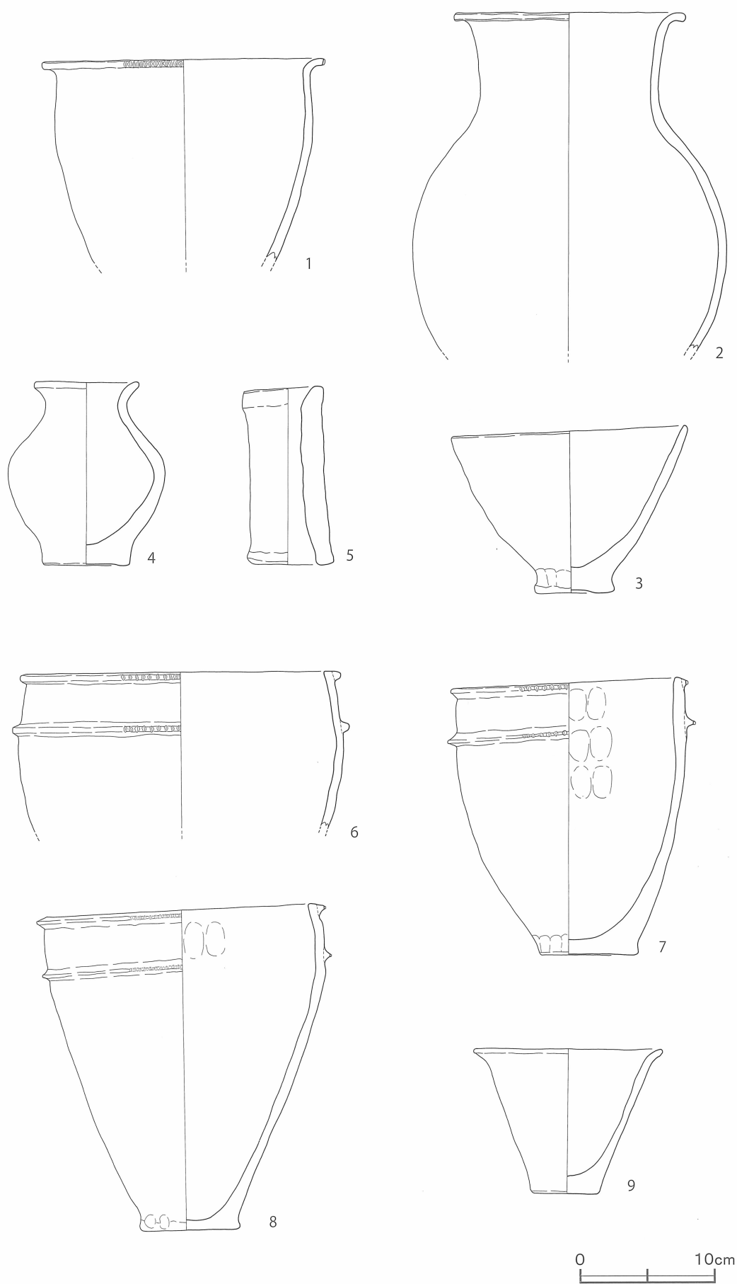
第22図 貯蔵穴 出土土器 実測図〔1／4〕
