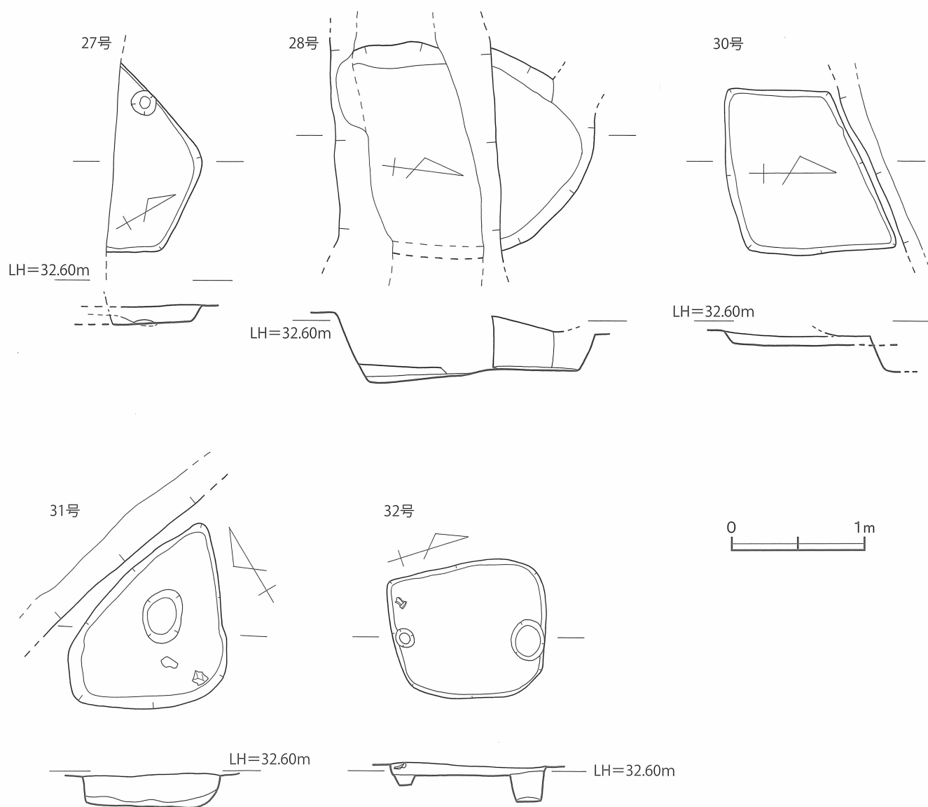
第12図 27・28・30～32号貯蔵穴 実測図 [1/40]
