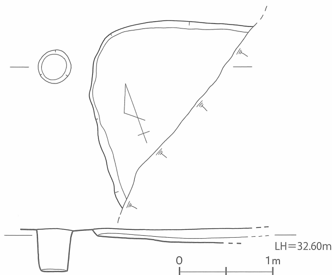
第 6 図 9号竪穴式住居 実測図 [1/40]
