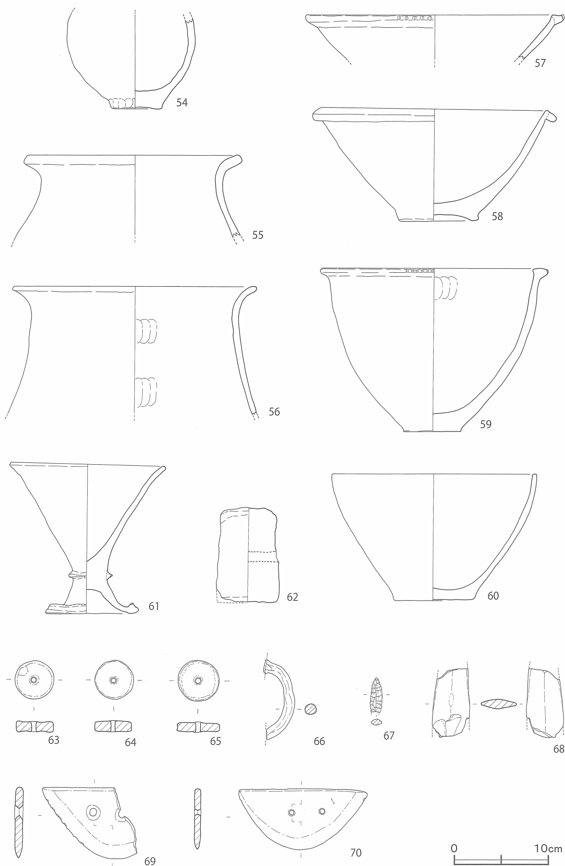
第39図 V字溝出土遺物実測図 (67は下層、他は中層) [1/4]
