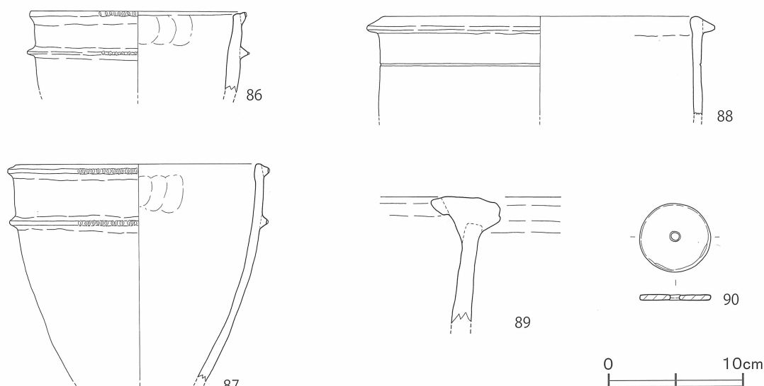
第41図 貯蔵穴 出土遺物実測図〔1／4〕
