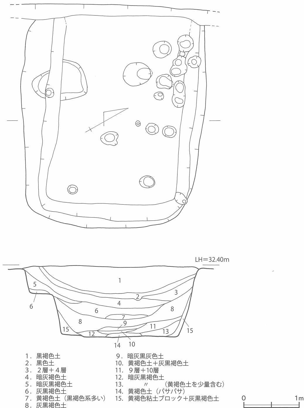
第35図 54号貯蔵穴 実測図 [1/40]
