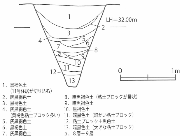
第 37 図 V 字溝南壁土層断面 実測図 [1/40]
