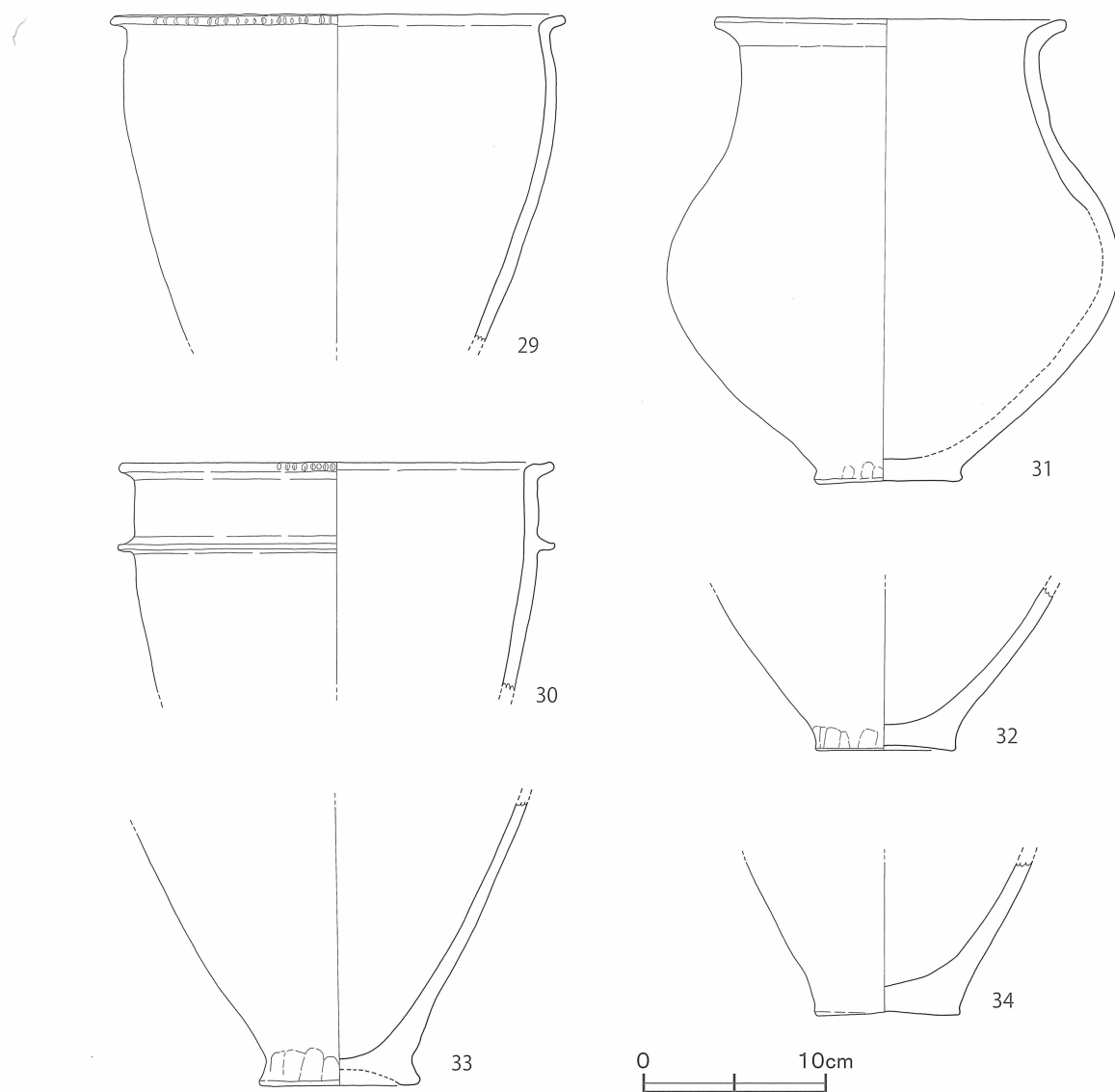
第25図 貯蔵穴 出土土器 実測図〔1/4〕
