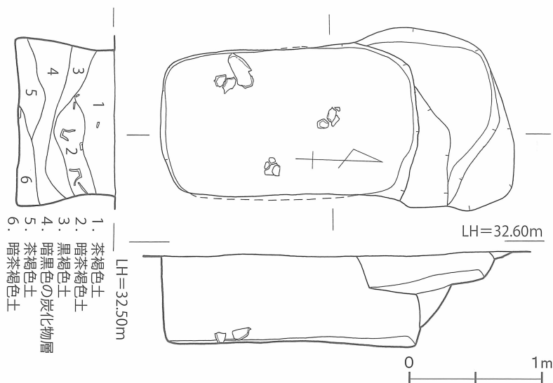
第10図 24号貯蔵穴 実測図 [1/40]
