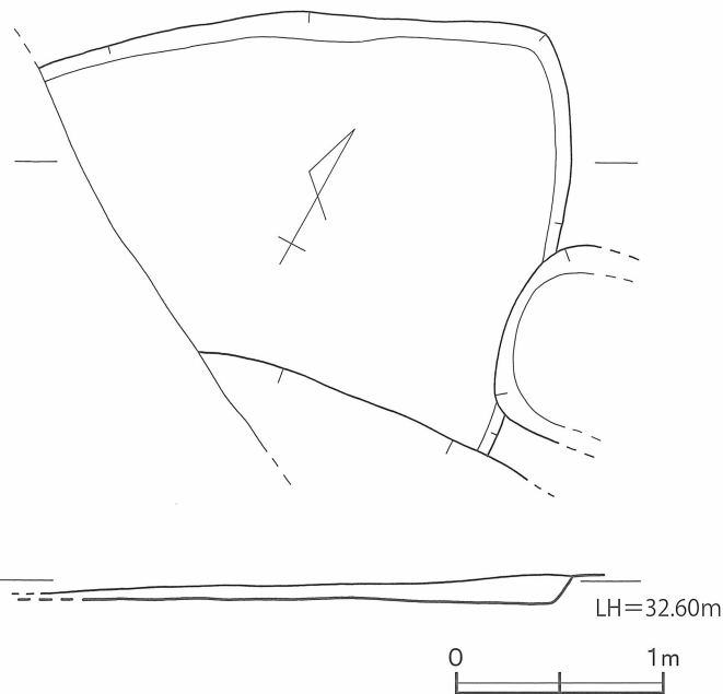
第4図 7号竪穴式住居 実測図 [1/40]
