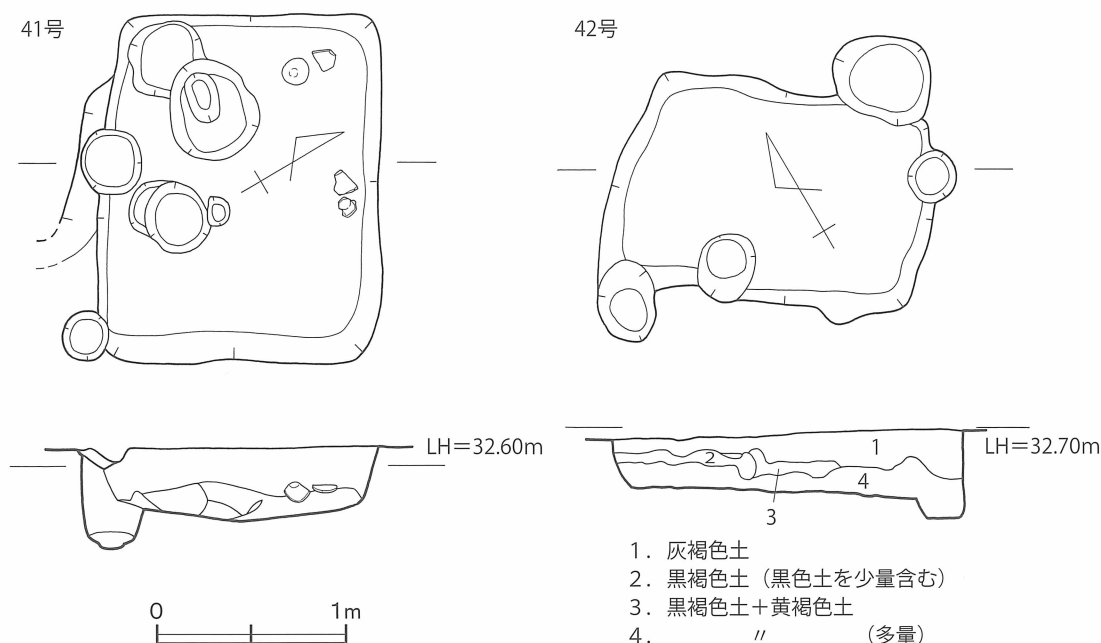
第17図 41・42号貯蔵穴 実測図 [1/40]
