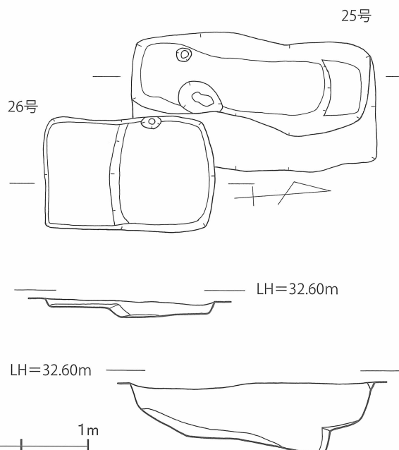
第11図 25・26号貯蔵穴 実測図 [1/40]
