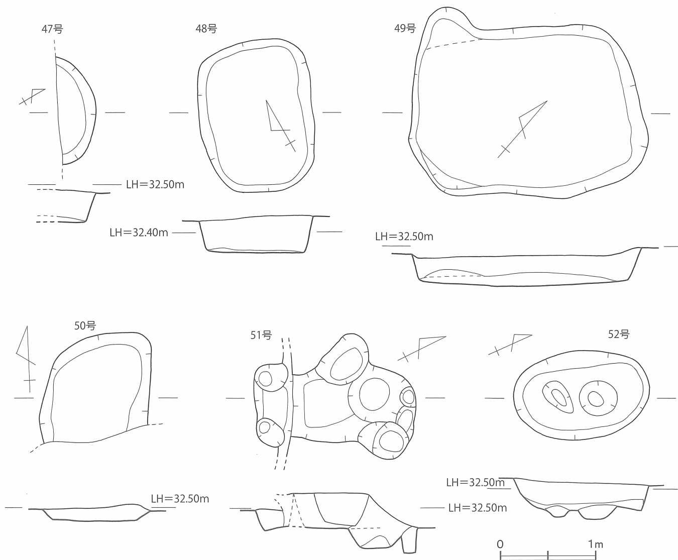
第33図 47～52号貯蔵穴 実測図 [1/40]
