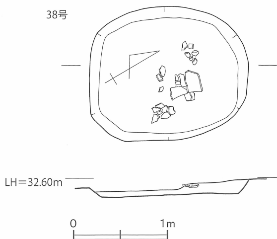
第14図 33~38号貯蔵穴 実測図 [1/40]
