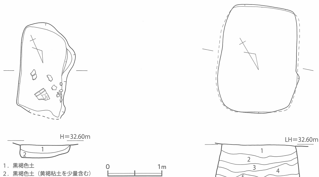
第15図 39号貯蔵穴 実測図 [1/40]
