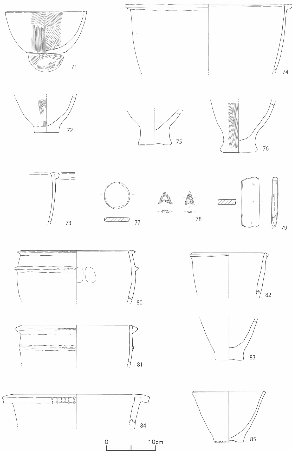
第40図 竪穴式住居及び貯蔵穴 出土遺物実測図 [1/4]
