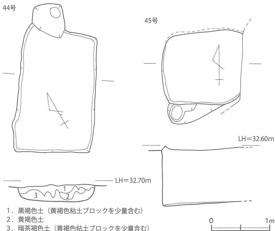
第19図 44・45号貯蔵穴 実測図 [1/40]
