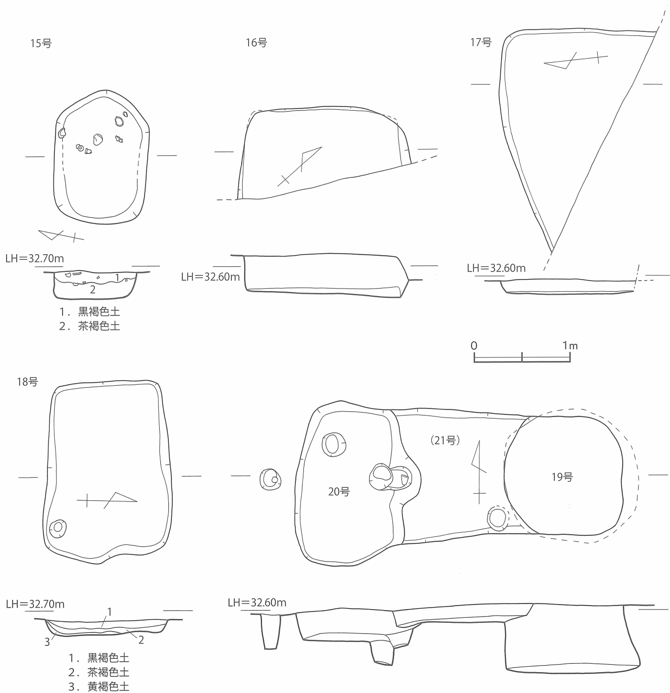
第 8 図 15～(21)号 貯蔵穴 実測図 [1/40]
