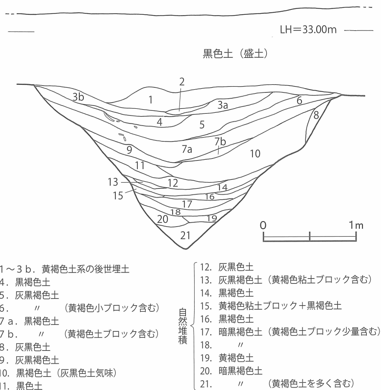
第 36 図 V 字溝西壁土層断面 実測図 [1/40]
