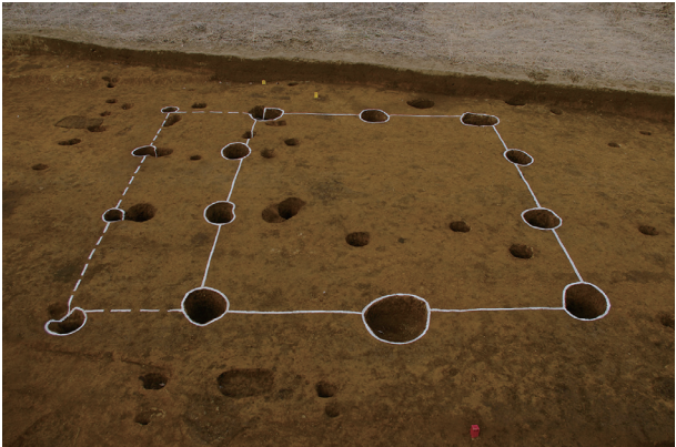
1 第9号掘立柱建物跡
