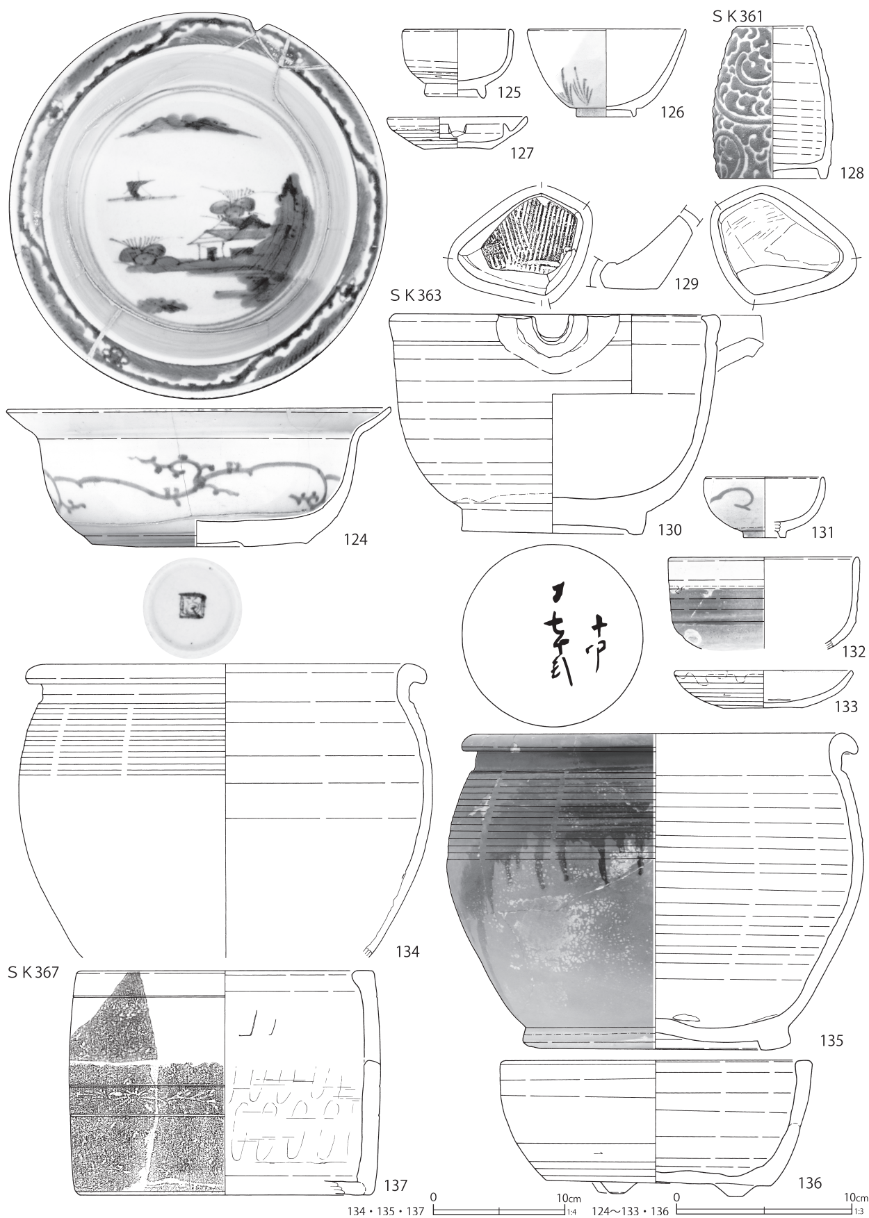
第 155 図 土壇出土遺物 (21)
