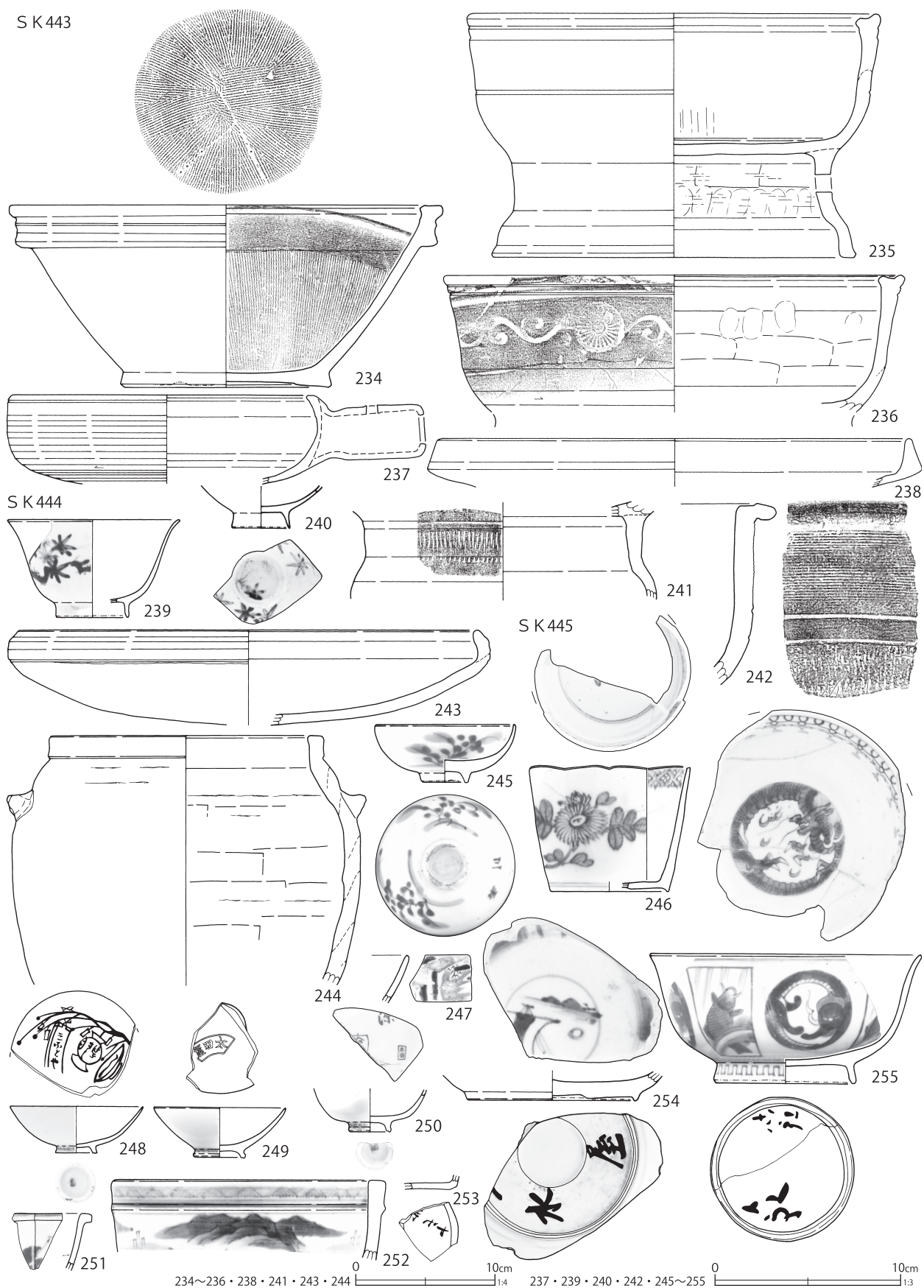
第 160 図 土壙出土遺物 (26)
