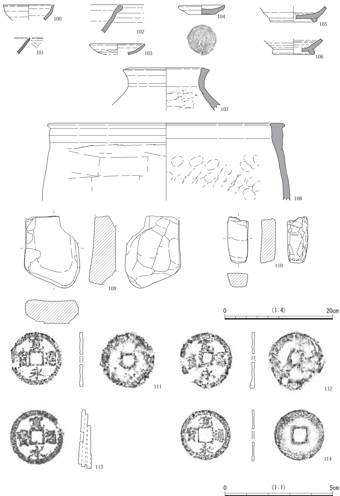
Fig.61 II c 区南部 出土遺物 (2)
