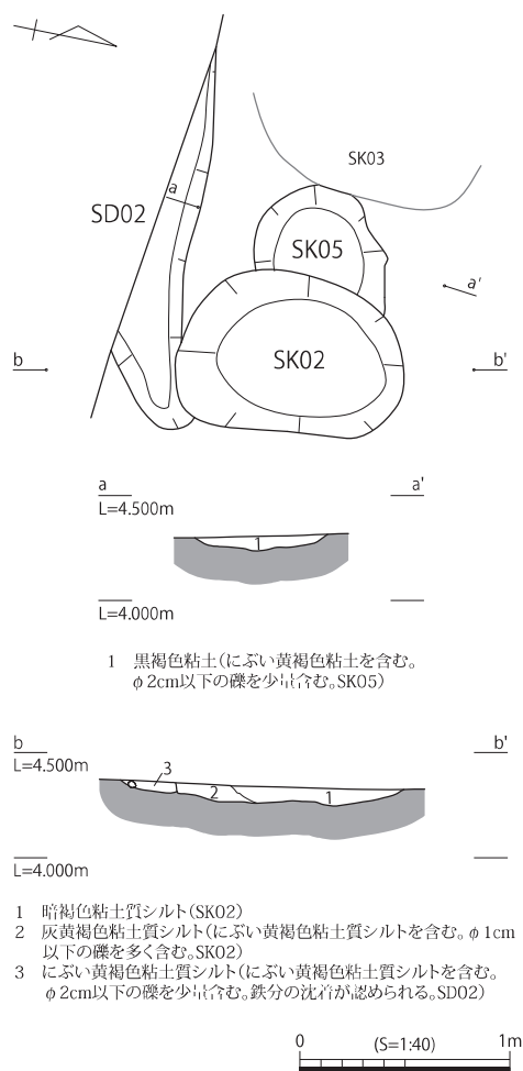
Fig.72 IV区 SD02・SK02・SK05 遺構図
