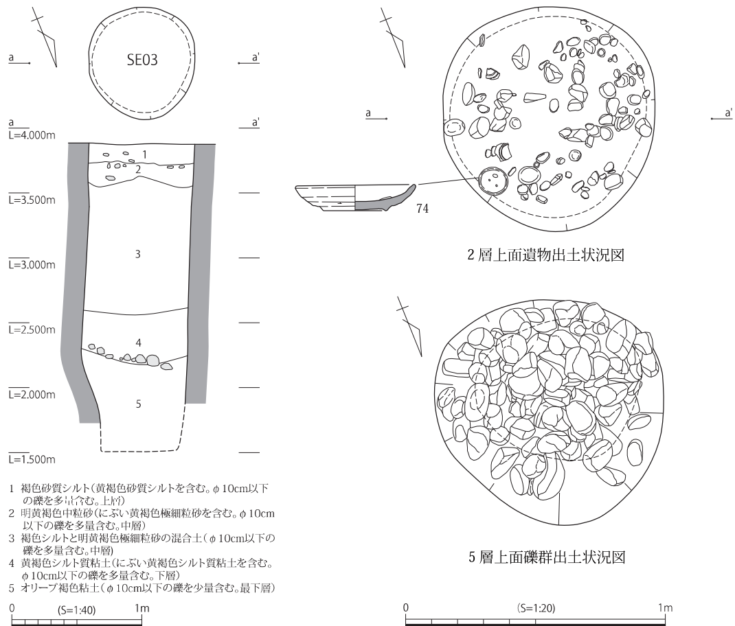
Fig.46 II c 区北部 SE03 遺構図
