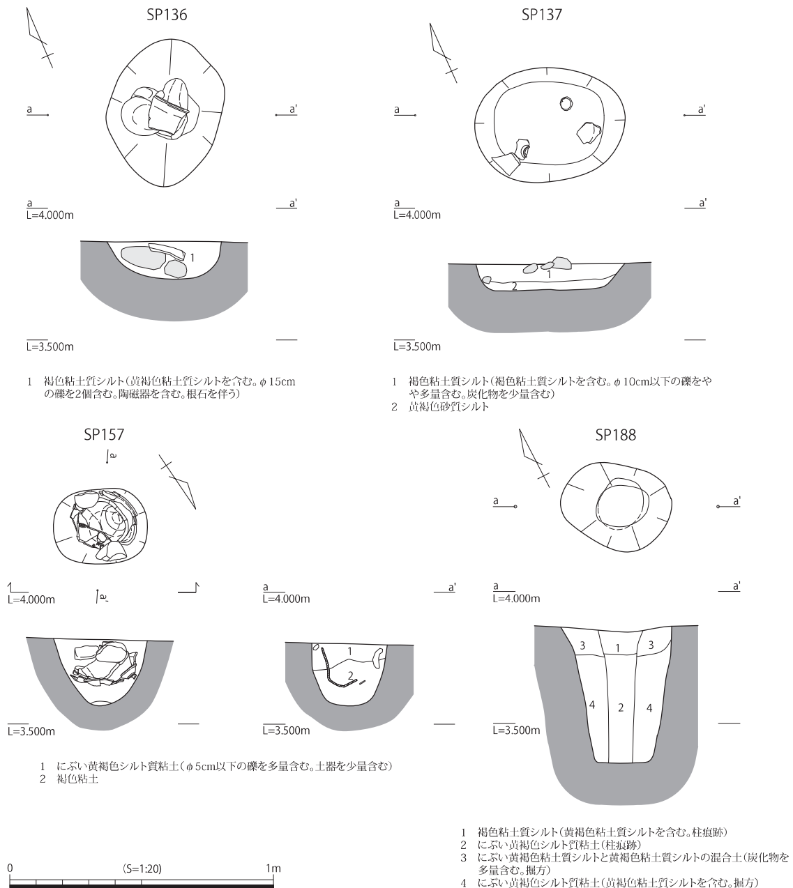
Fig.52 II c 区南部 遺構図 (3)
