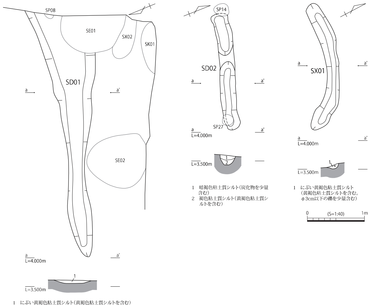
Fig.20 I区 遺構図(1)
