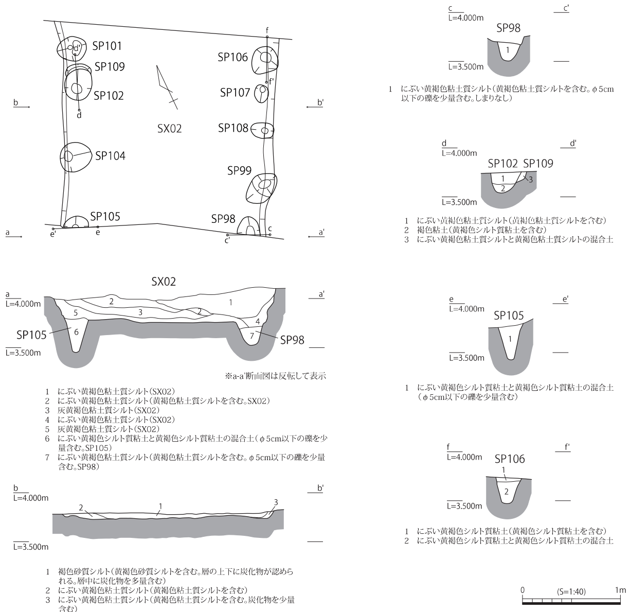
Fig.54 II d 区 SX02 遺構図
