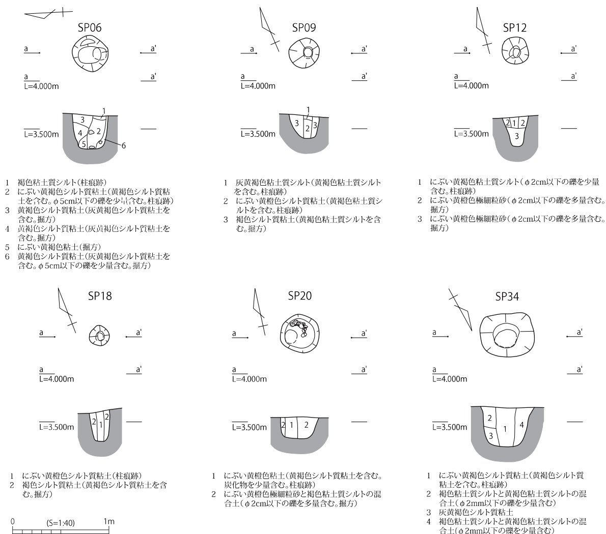
Fig.24 I 区 遺構図(2)
