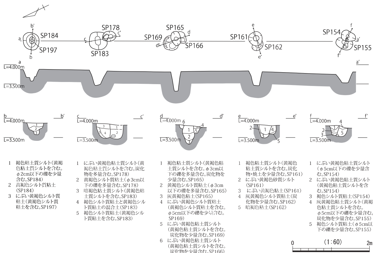
Fig.57 II c 区南部 SA02 遺構図
