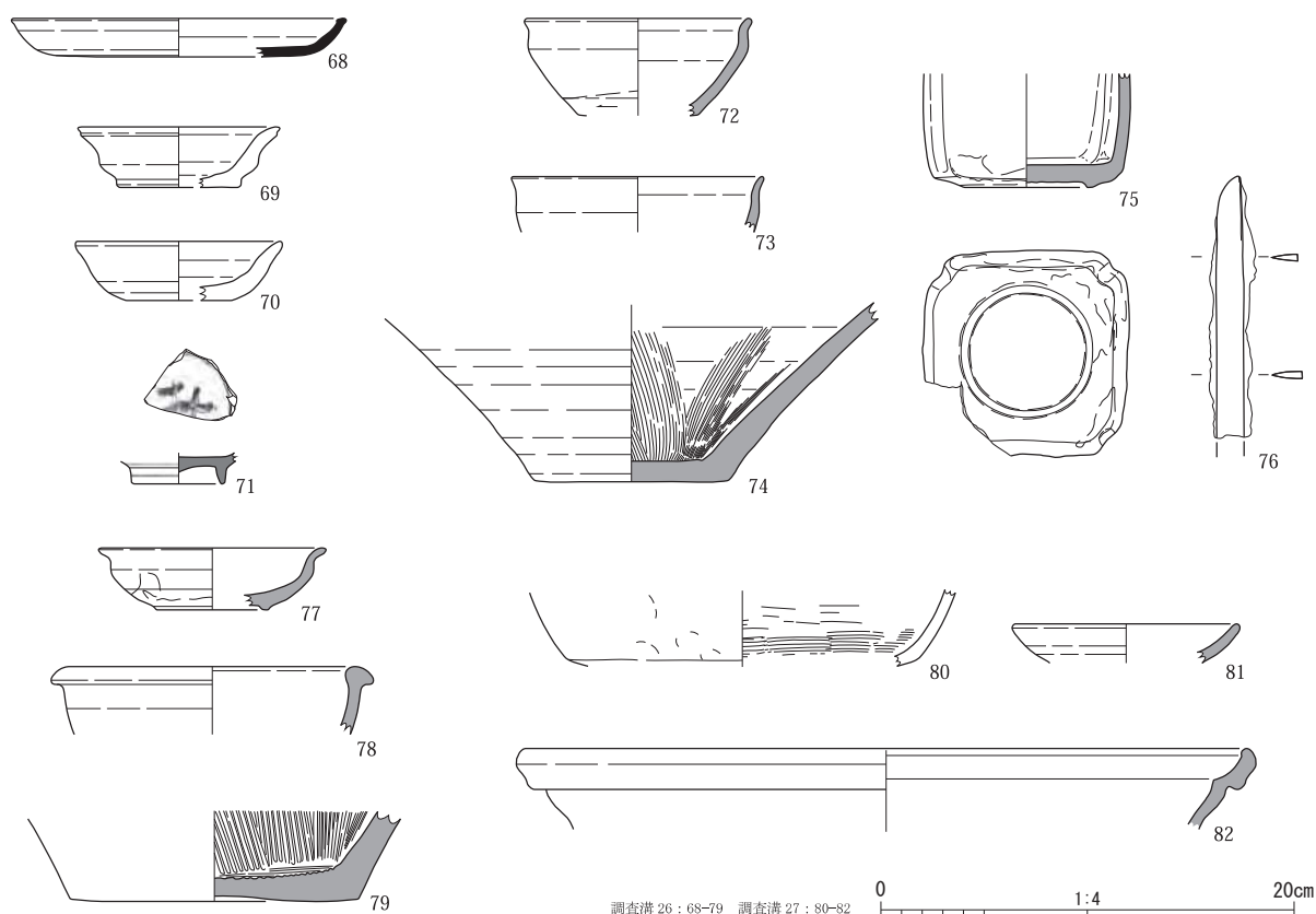
Fig.12 8次調査出土遺物
