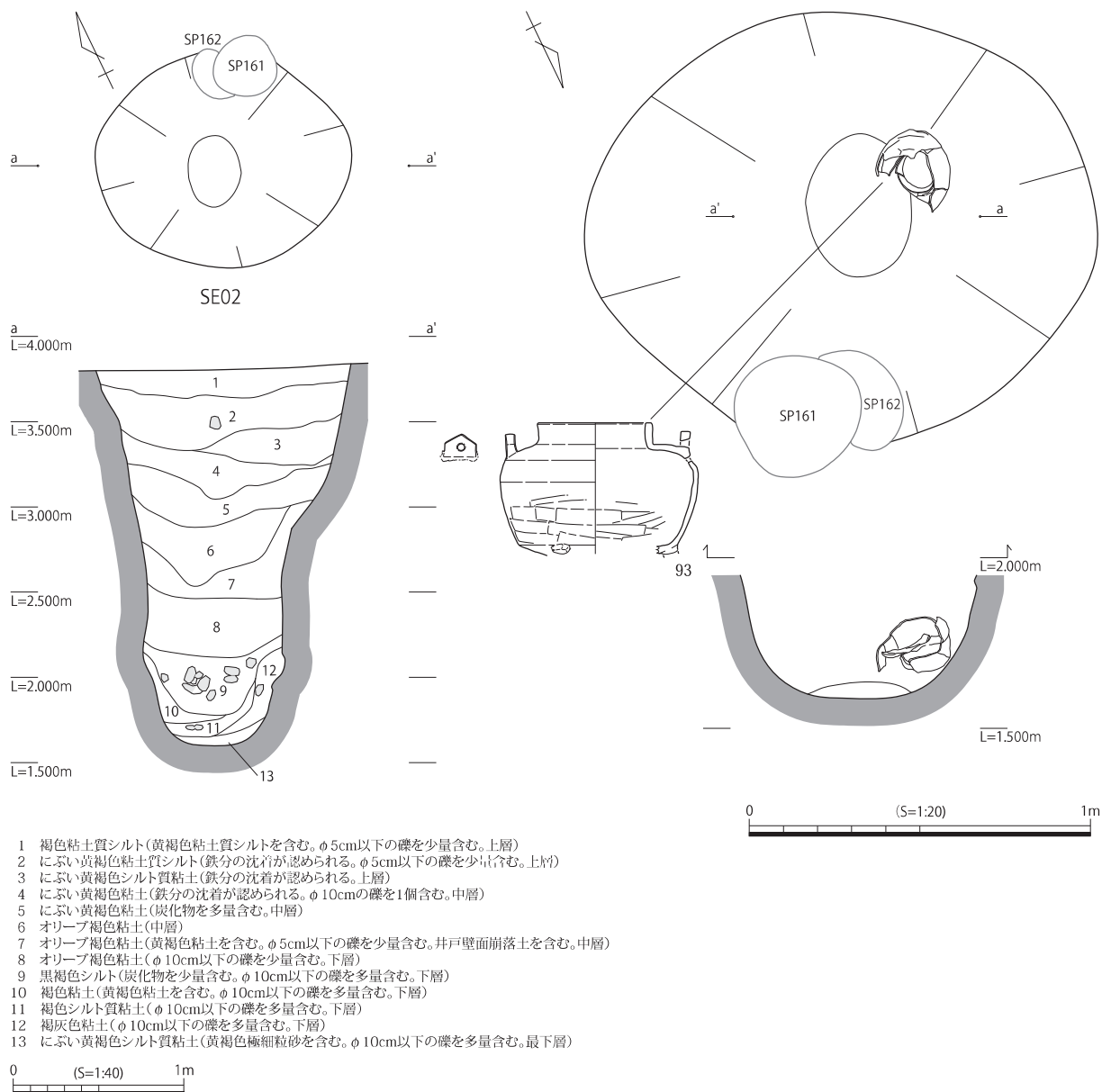
Fig.45 II c 区南部 SE02 遺構図
