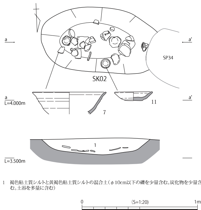
Fig.23 I 区 SK02 遺物出土状況図
