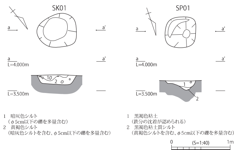
Fig.67 III区 遺構図
