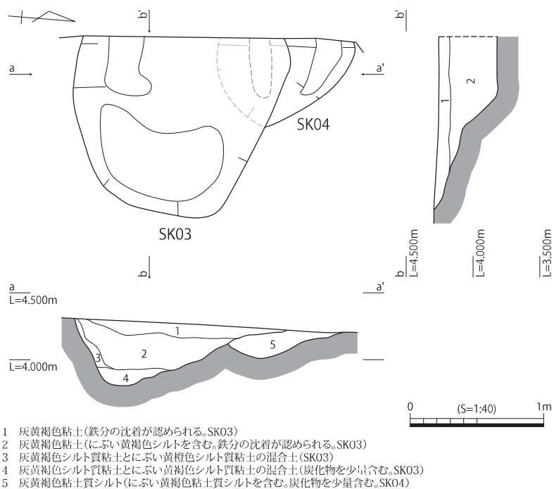
Fig.73 IV区 SK03・SK04 遺構図
