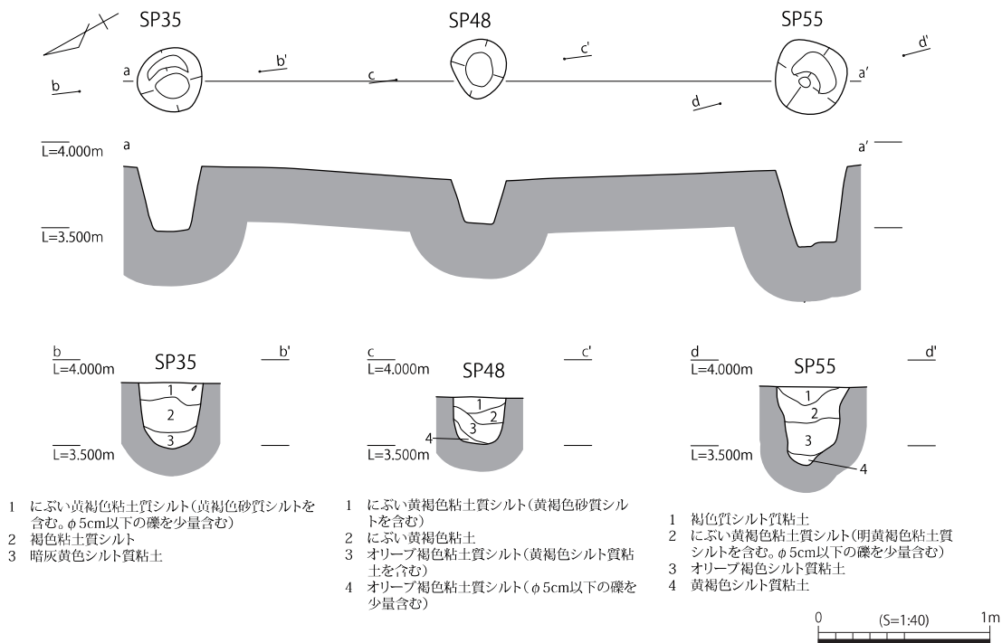
Fig.56 II a 区 SA01 遺構図
