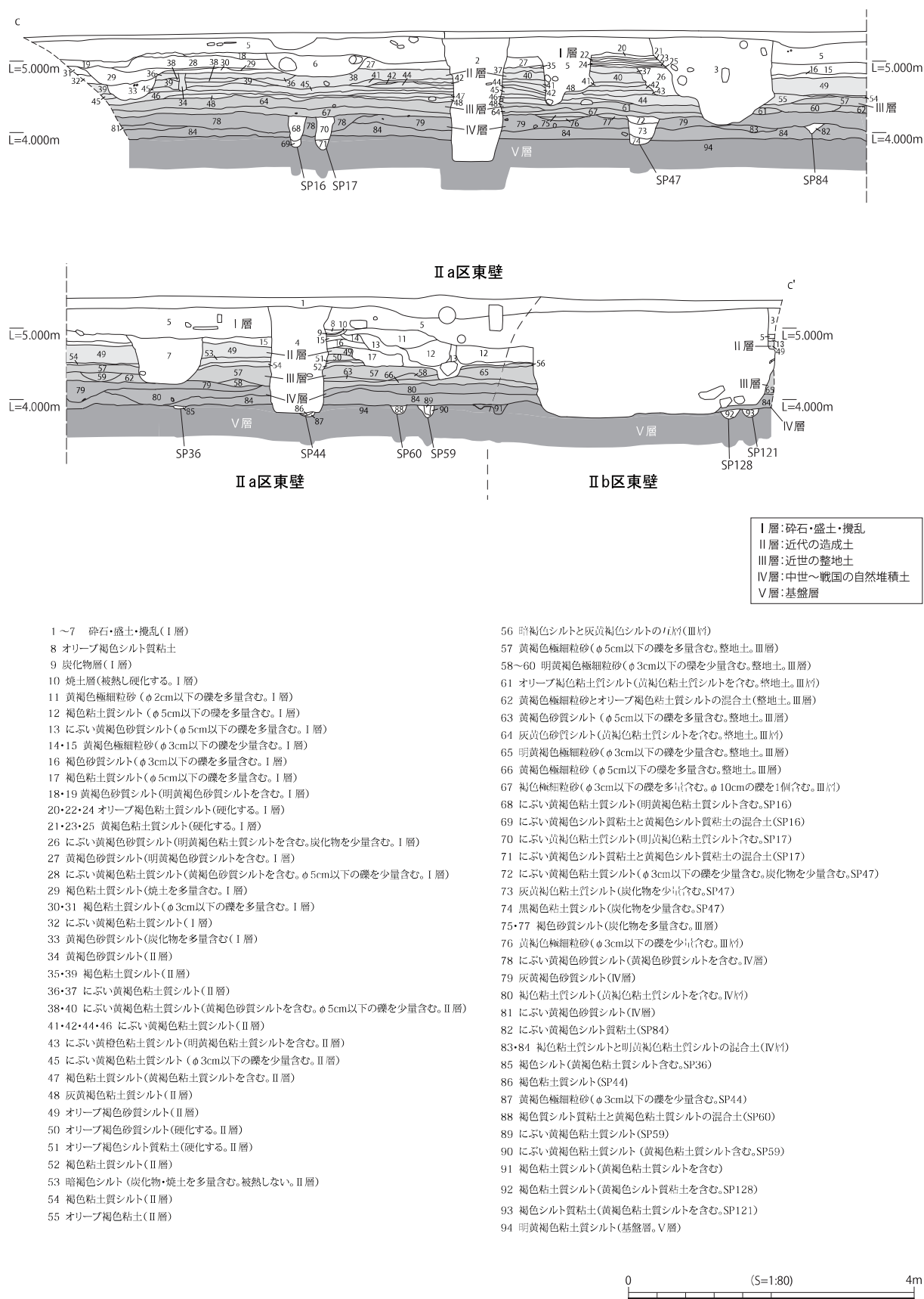
Fig.32 II a · II b 区 壁面図 (2)
