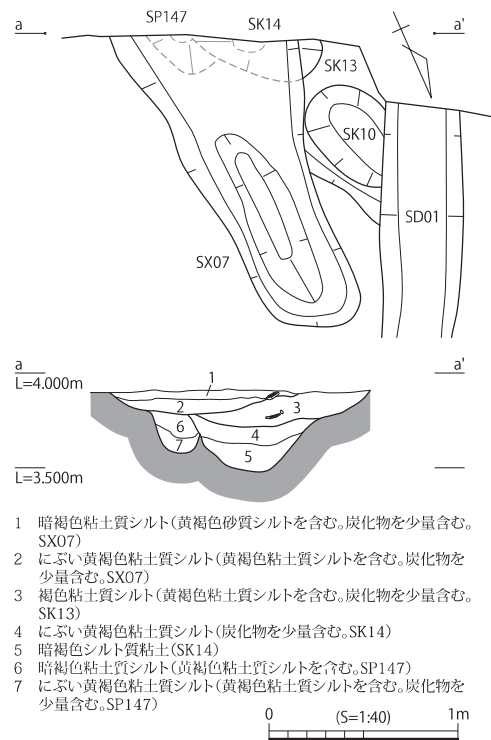
Fig.49 II c 区北部 遺構図 (1)
