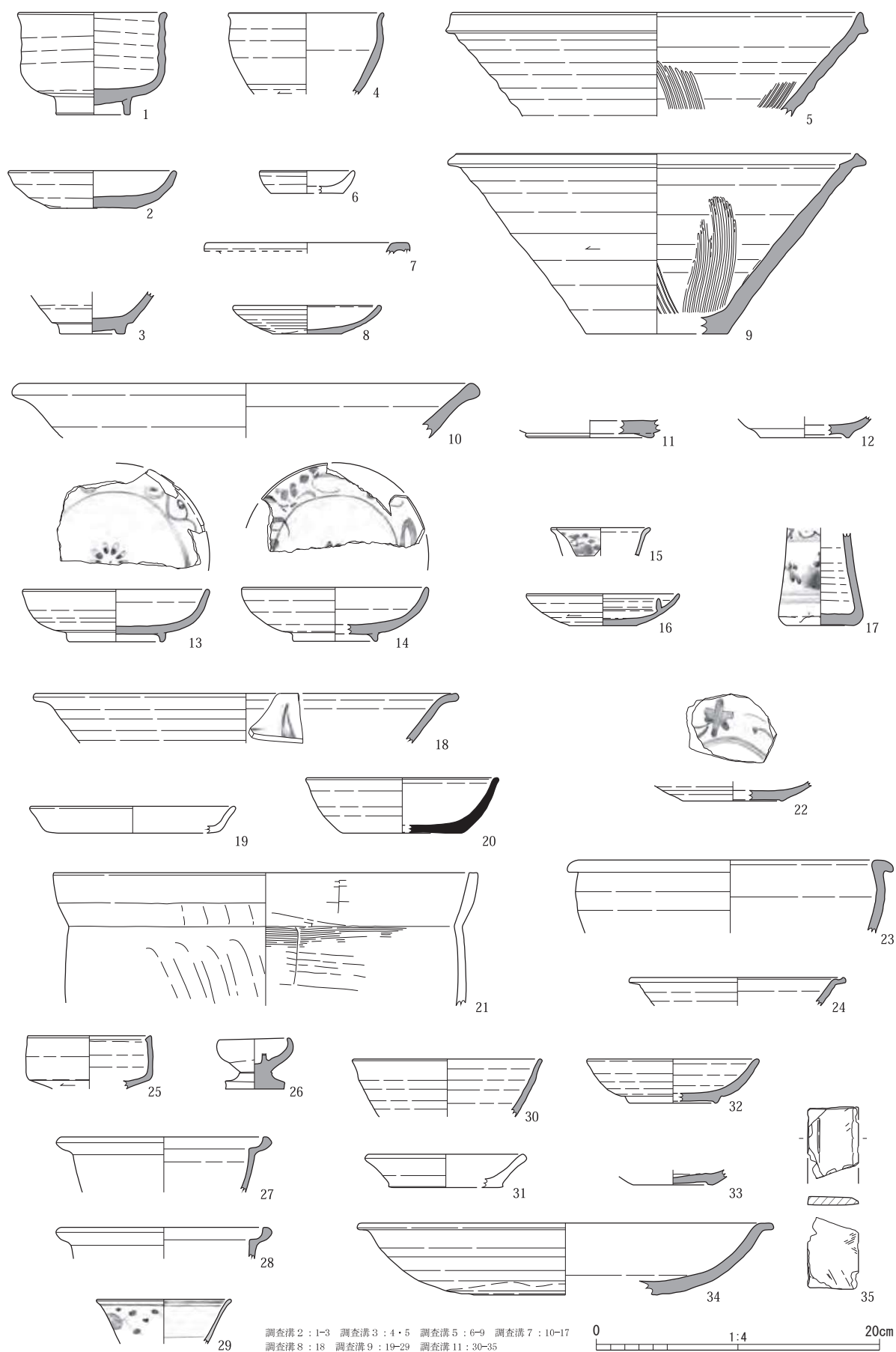
Fig.10 7次調査出土遺物 (1)
