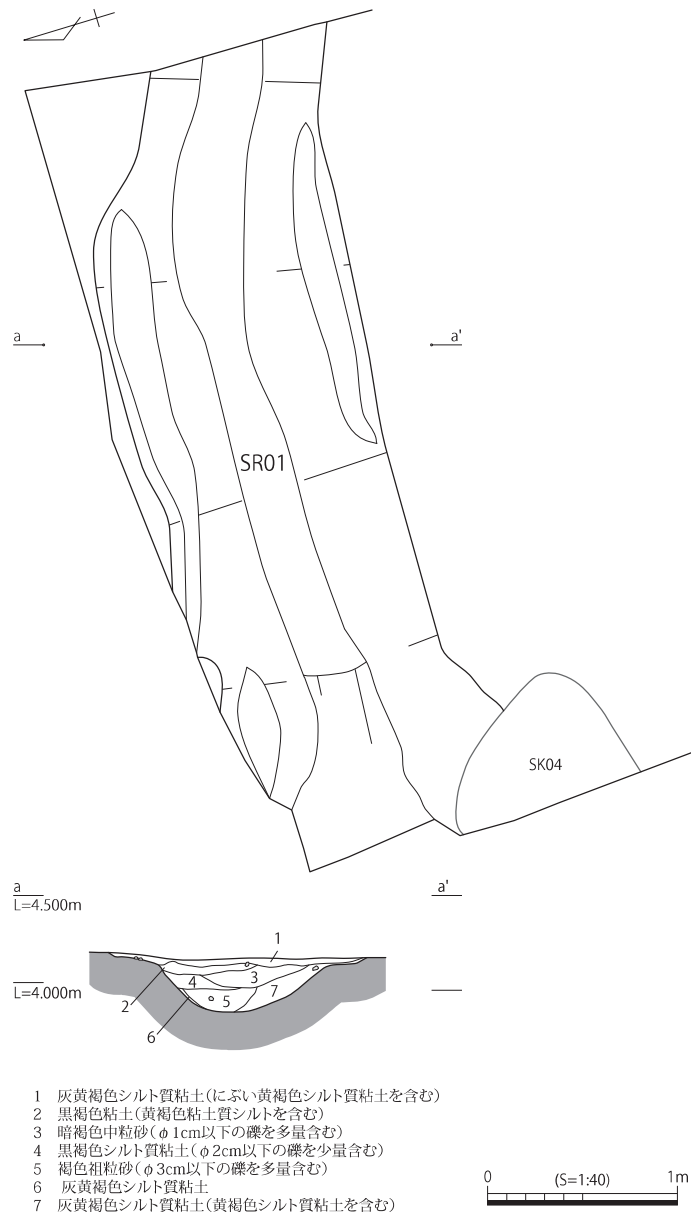
Fig.74 IV区 SR01 遺構図
