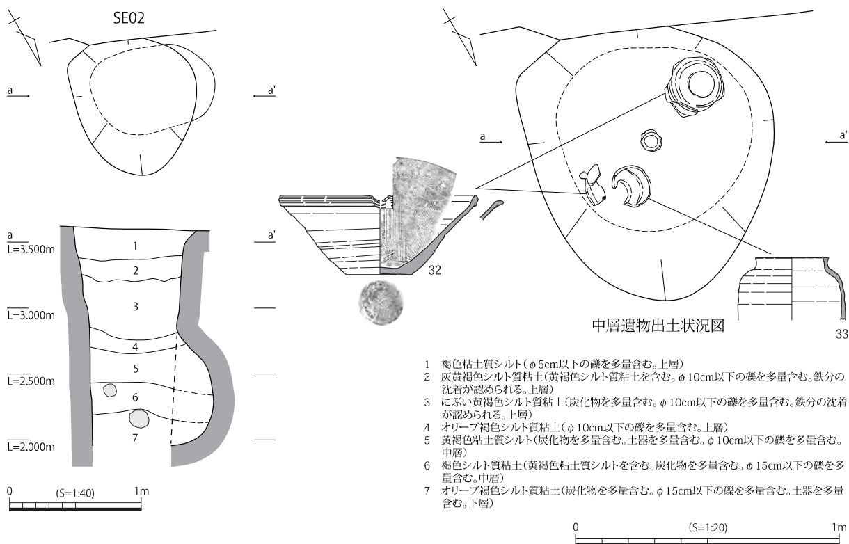
Fig.22 I区 SE02 遺構図
