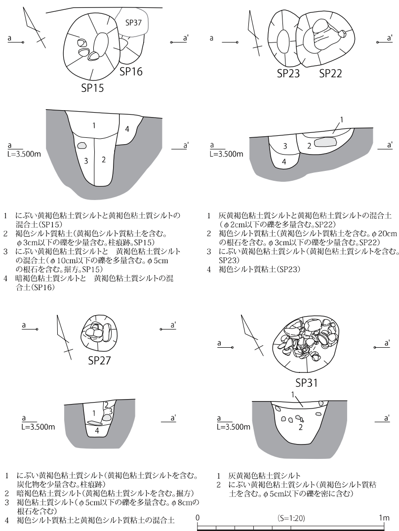
Fig.25 I 区 遺構図 (3)
