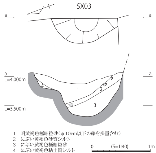
Fig.55 II d 区 SX03 遺構図
