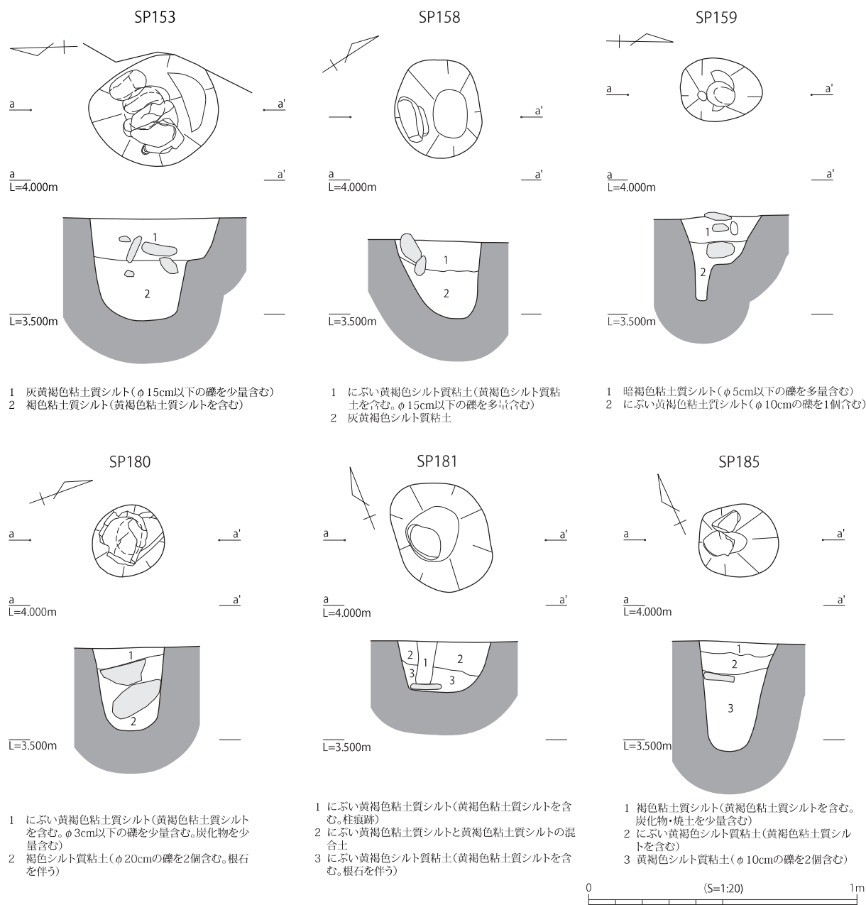
Fig.51 II c 区南部 遺構図(2)
