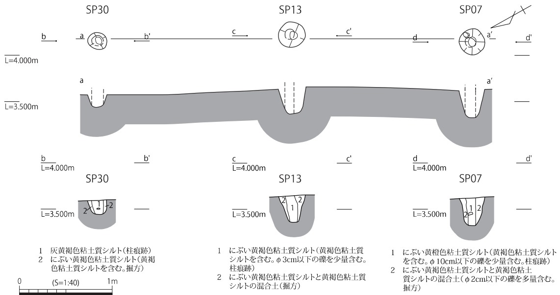
Fig.26 I区 SA01 遺構図
