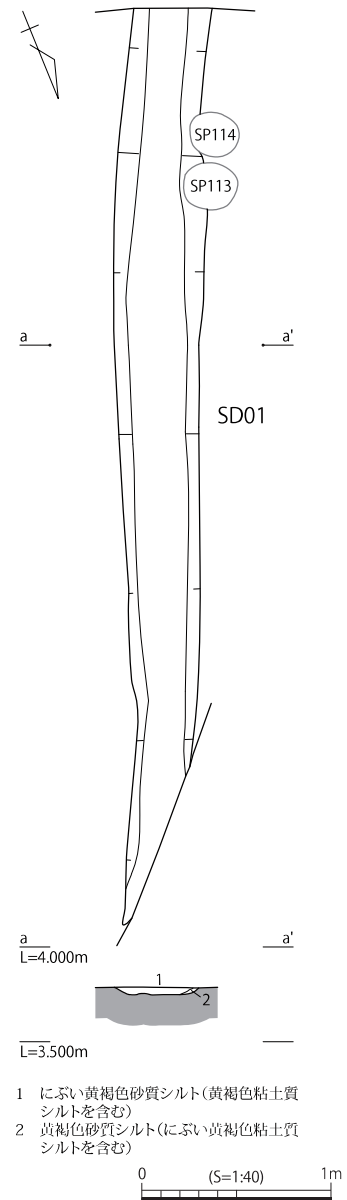
Fig. 40 Ⅱ b 区 SD01 遺構図
