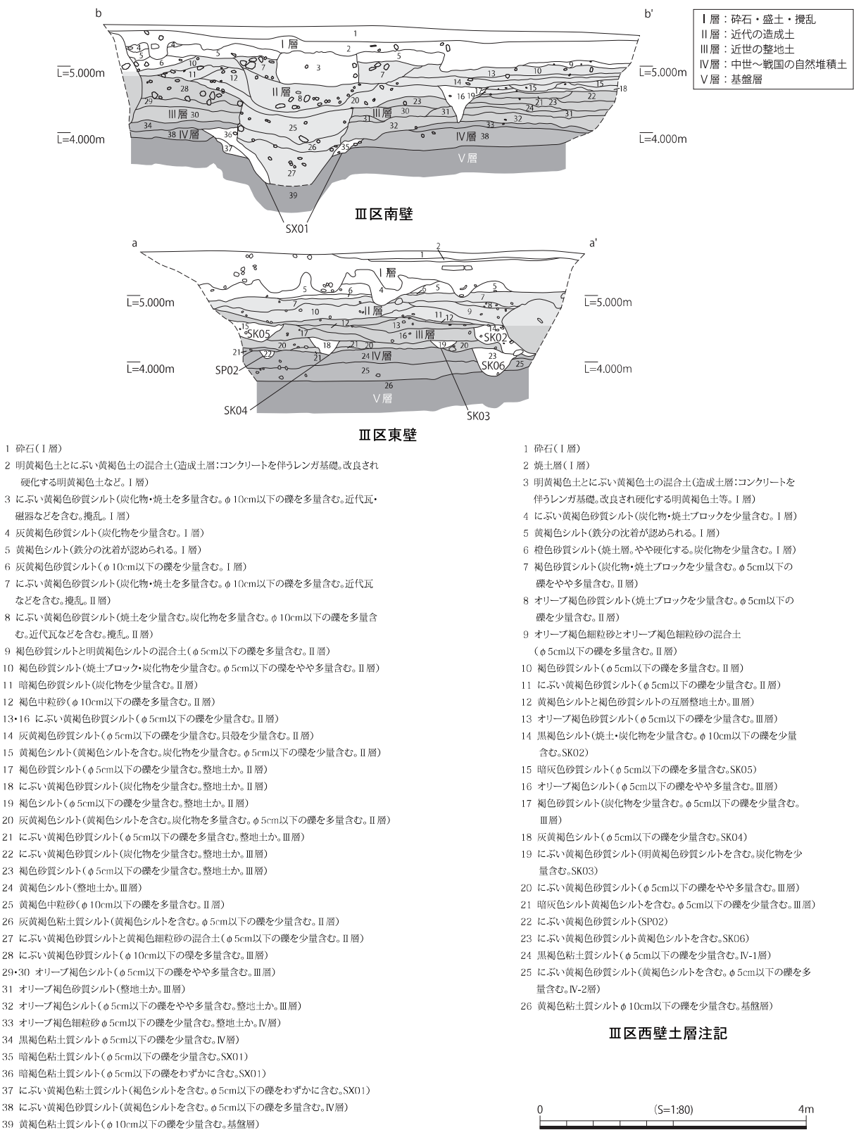
Fig.66 III区 壁面図
