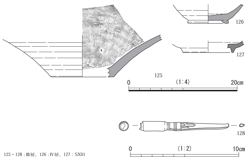
Fig.68 III区 出土遺物
