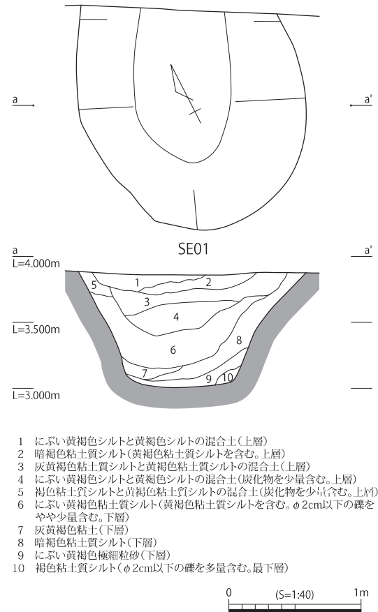
Fig.44 II c 区北部 SE01 遺構図
