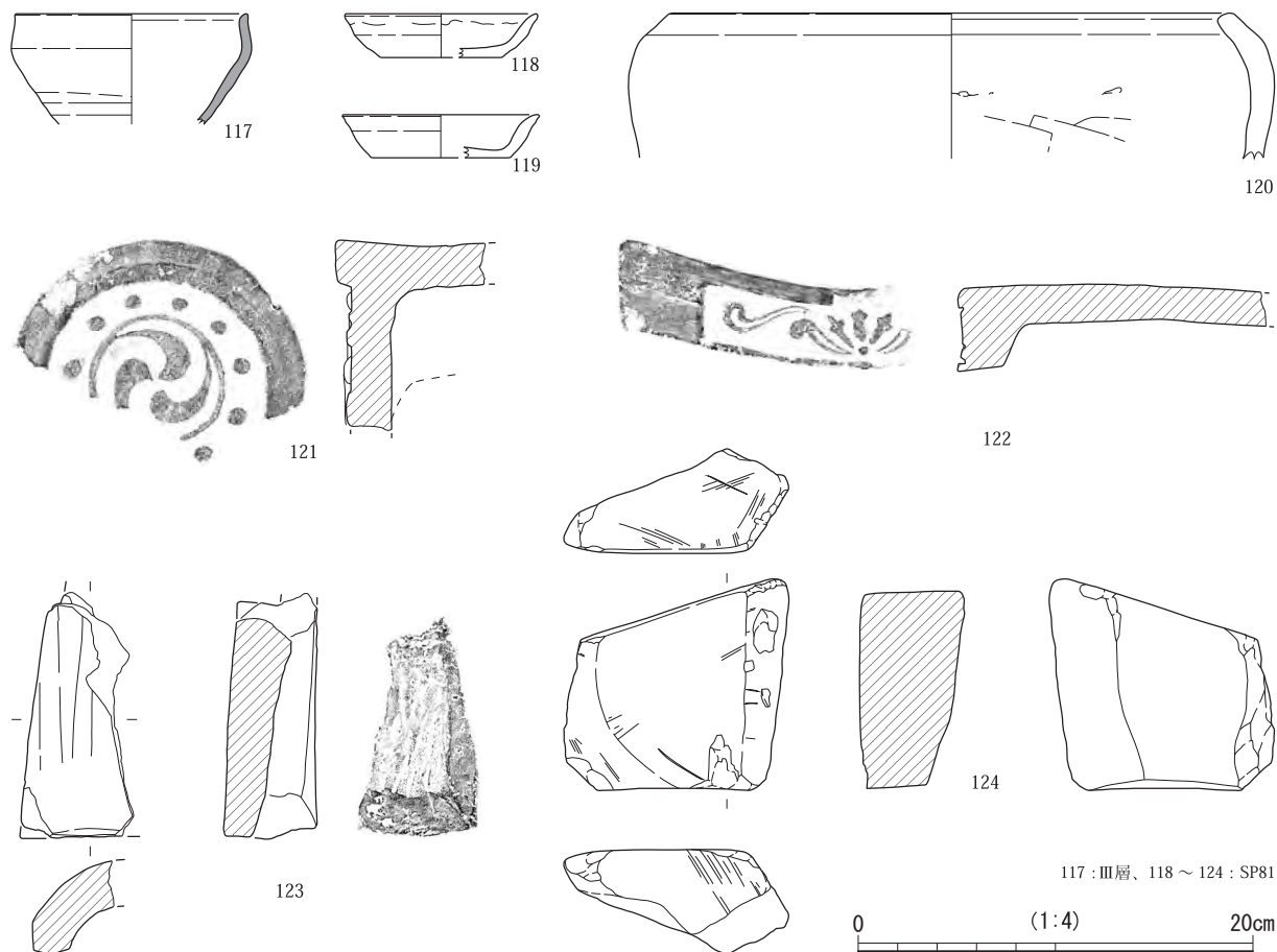
Fig.64 II e 区 出土遺物 (2)
