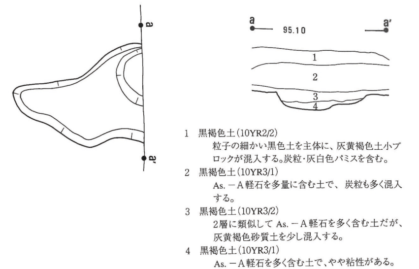
図18 SK33全体図
