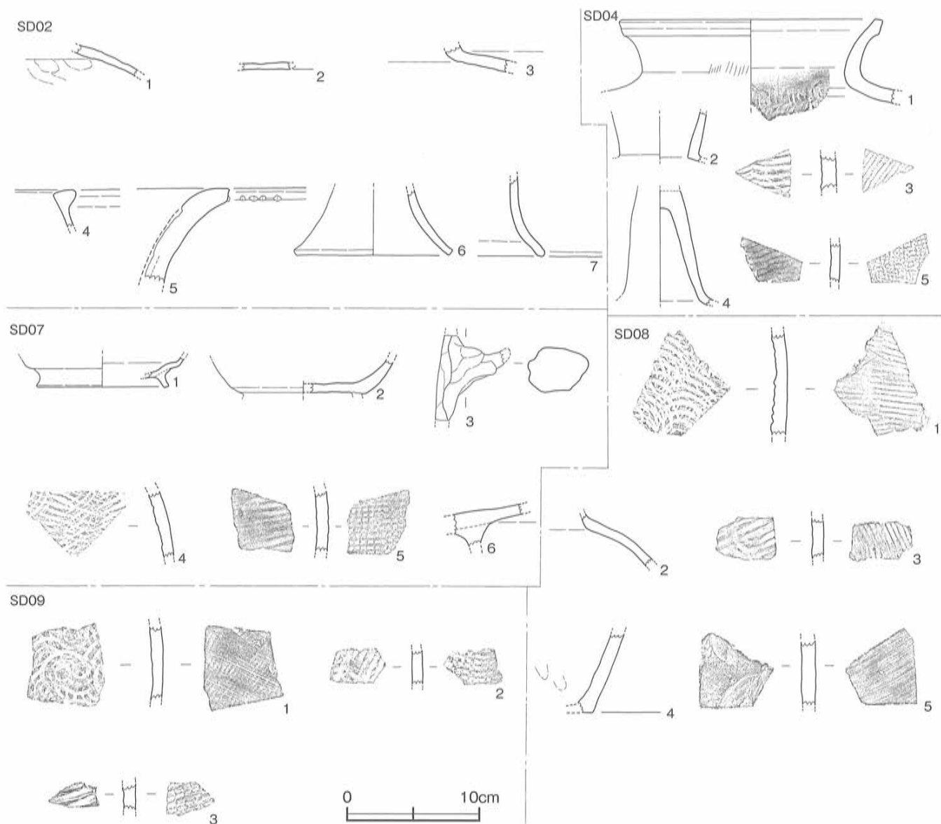
第69図 船底遺跡 溝 (SD02.04.07.08.09) 出土土器実測図 [1/4]
