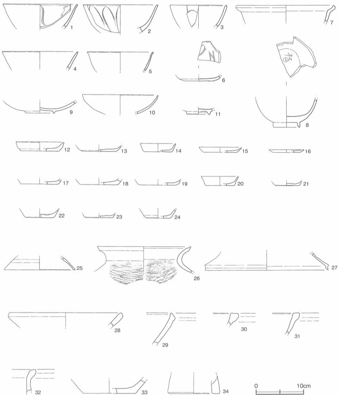
第37図 亀ノ甲・植初遺跡3次 出土土器実測図 [1/4]
