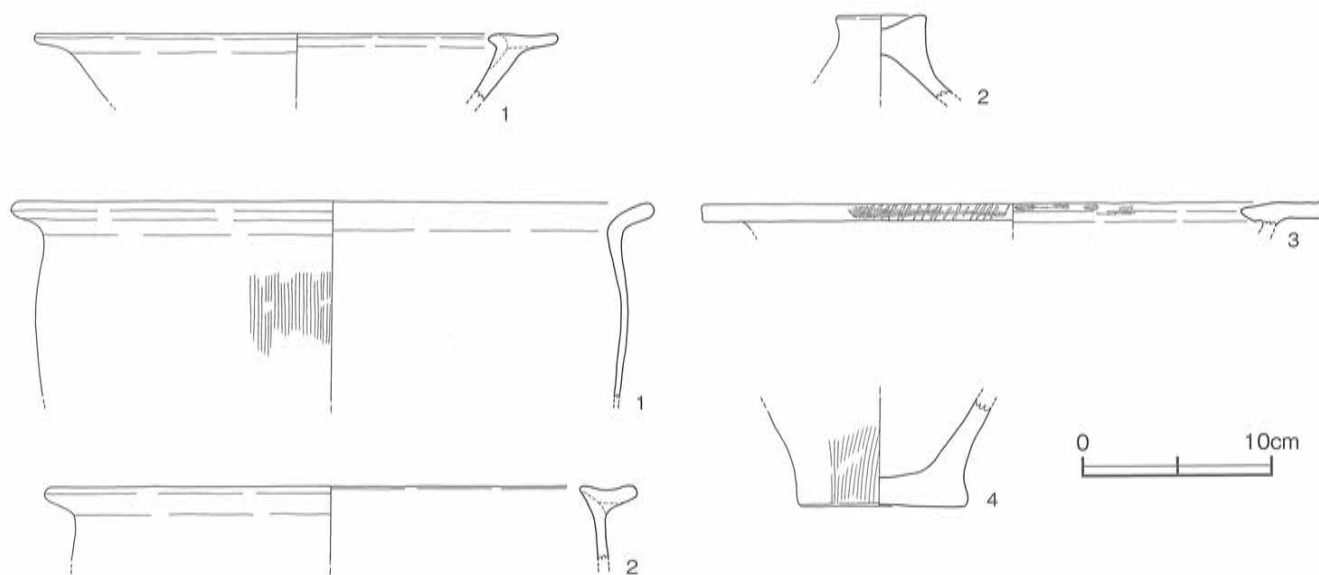
第22図 柳遺跡3次 竪穴住居 (SB) 土坑 (SK) 出土土器実測図 [1/ 4]
