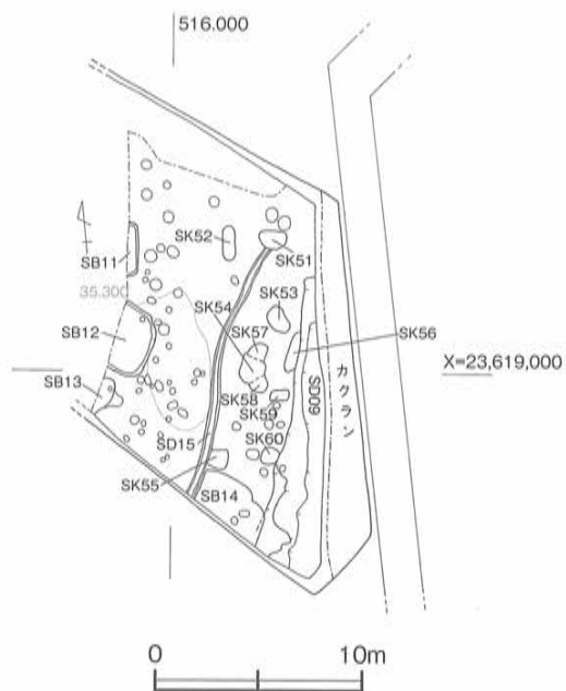
第19図 柳遺跡3次調査 遺構配置図 [1/ 400]
