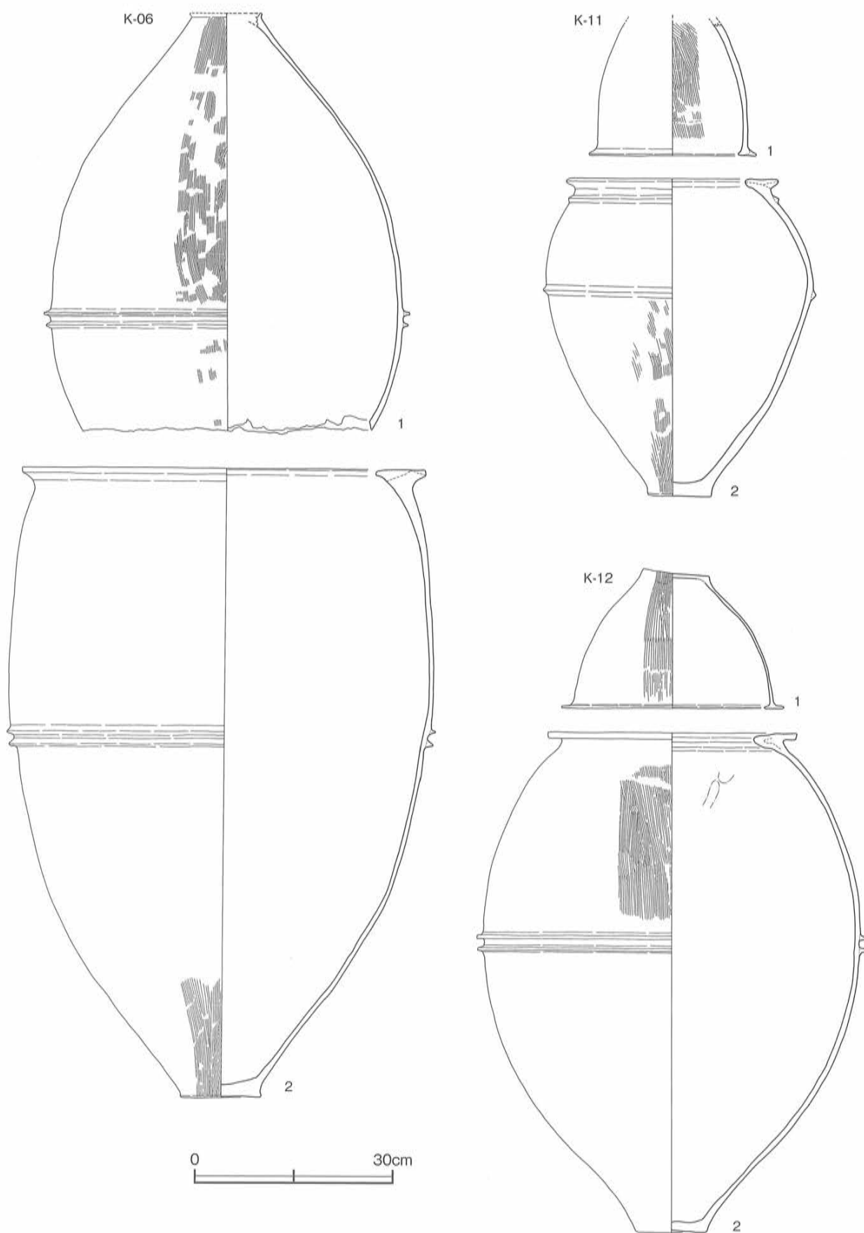
第3図 楠町遺跡2次 甕棺墓 (6. 11. 12号墓) 出土土器実測図 [1/8]
