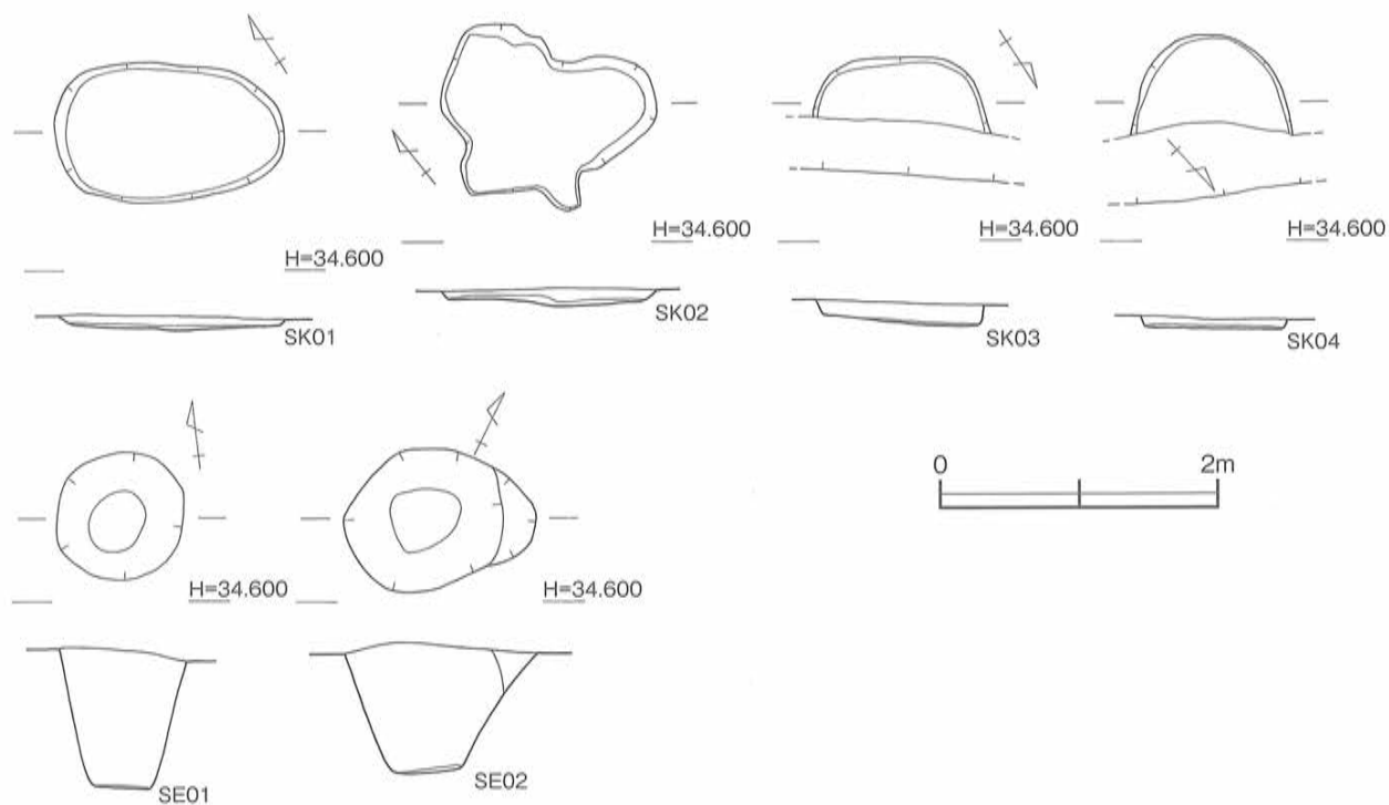
第54図 船底遺跡 土壇 (SK01~04) (SE01.02) 実測図 [1/60]
