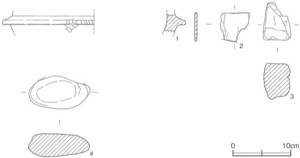
第40図 亀ノ甲・植初遺跡3次 出土石製品実測図〔1/4〕
