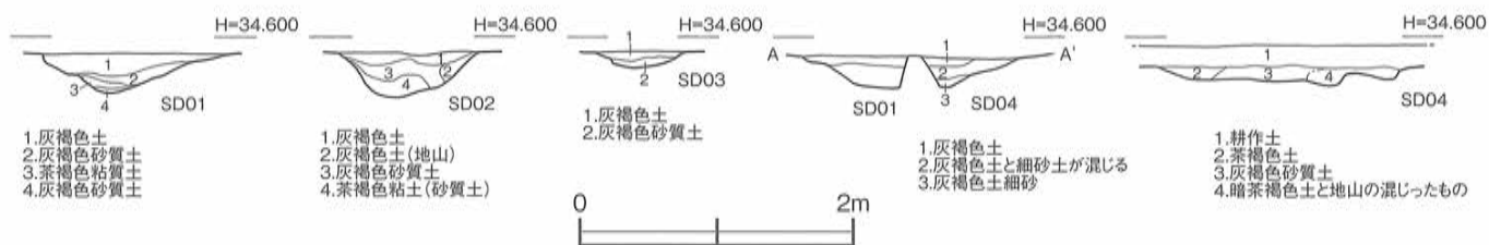
第15図 牟田田遺跡 溝 (SD01~04) 土層実測図 [1/60]
