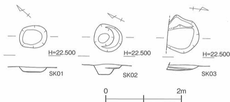
第43図 僧都遺跡2地点 土坑 (SK01~03) 実測図 [1/60]
