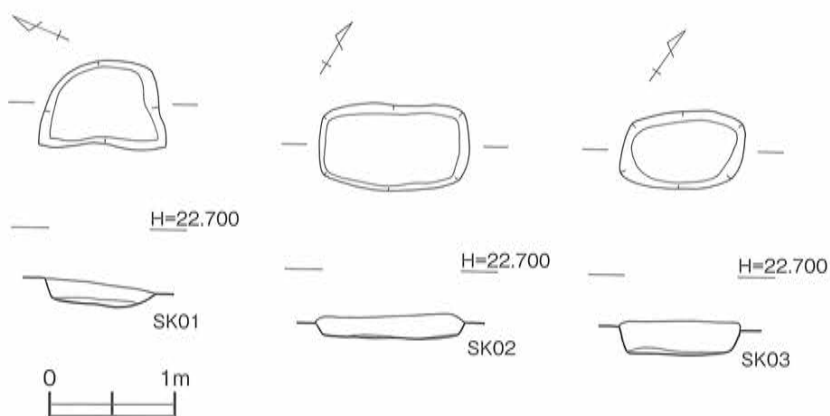
第49図 後田遺跡6次 土壌 (SK01~03) 実測図〔1/60〕
