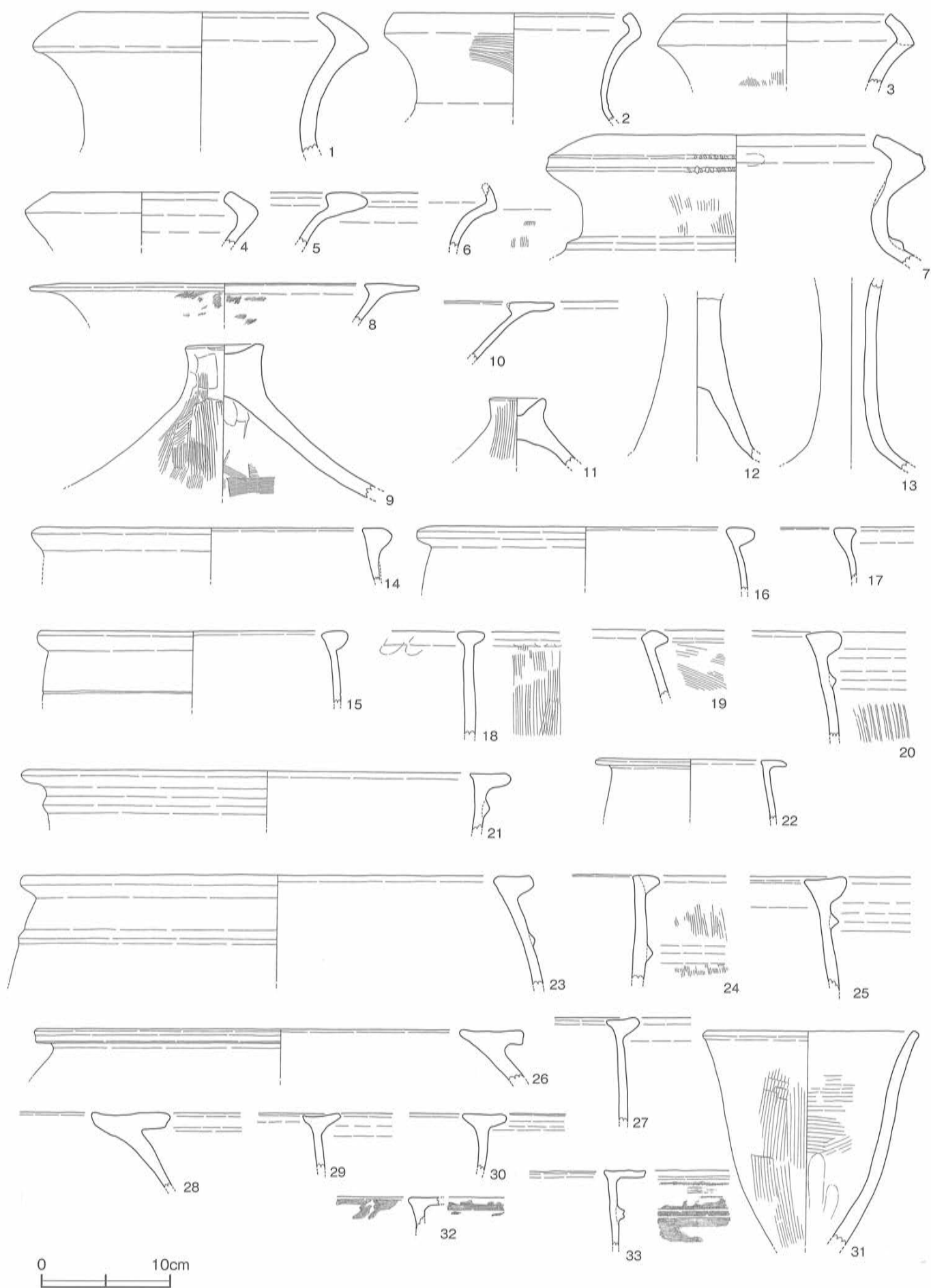
第59図 船底遺跡 溝 (SD01) 出土土器実測図 [1/4]
