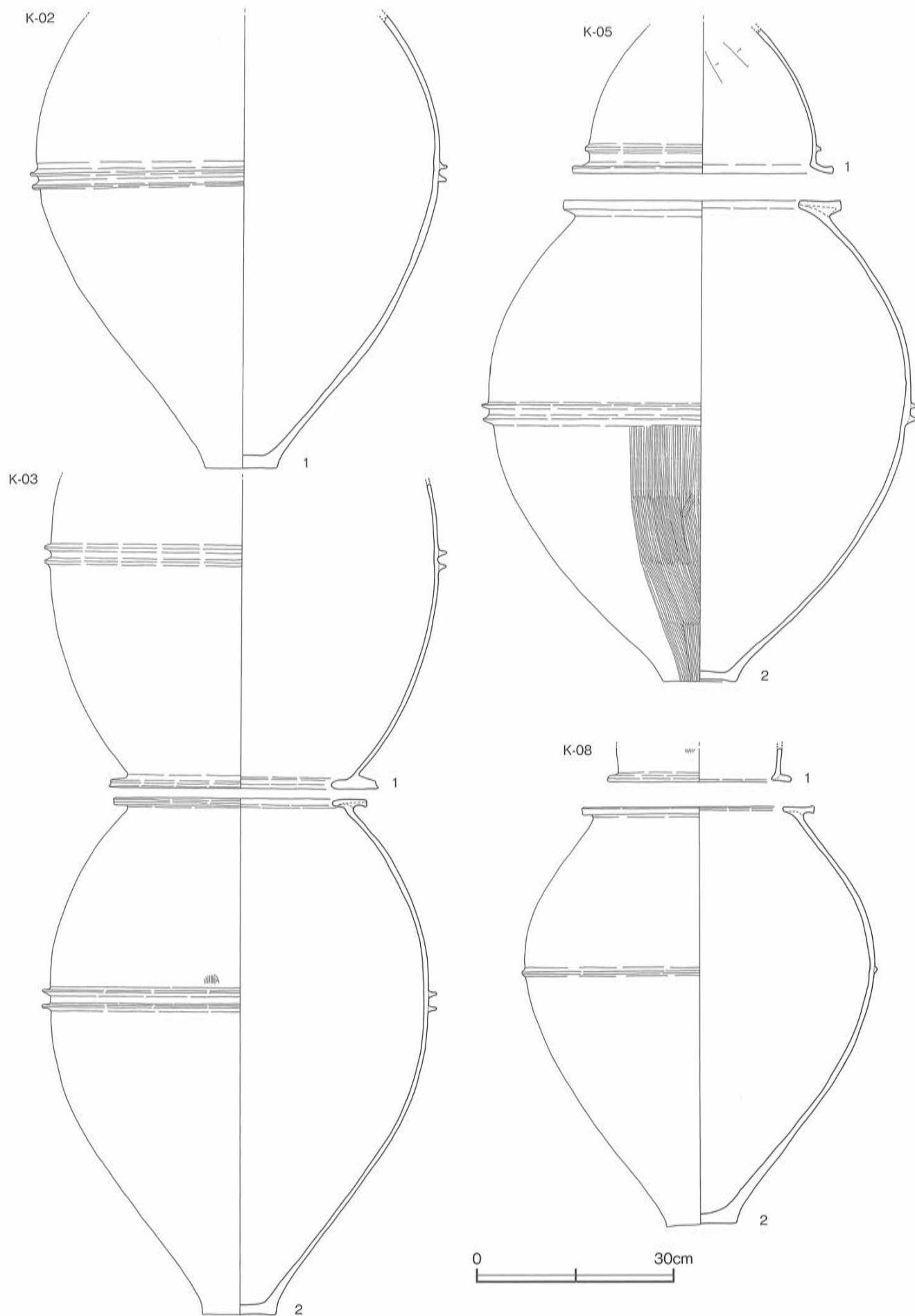
第2図 楠町遺跡2次 甕棺墓（2.3.5.8号墓）出土土器実測図〔1/8〕
