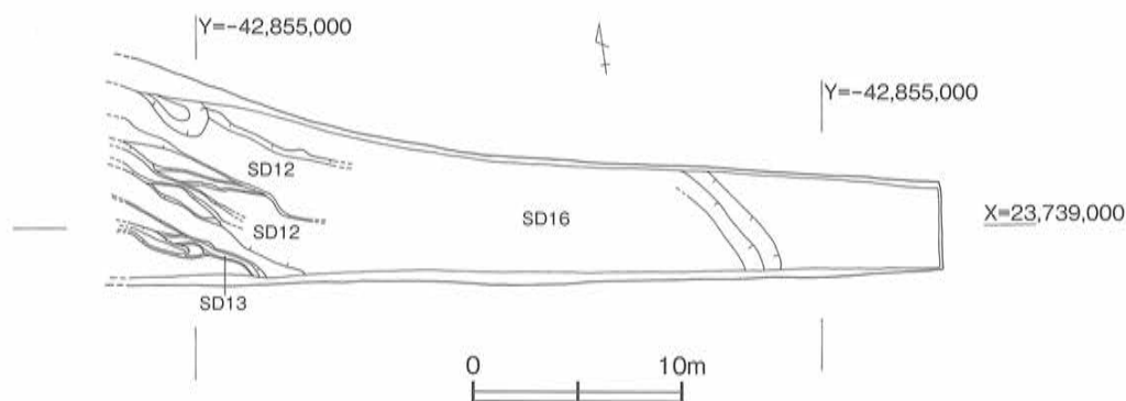
第45図 蒲原・植初遺跡3次 遺構配置図 [1/400]
