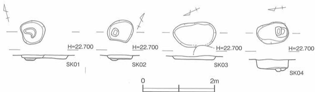
第34図 亀ノ甲・植初遺跡3次5地点 土壌 (SK01~04) 実測図 [1/ 60]
