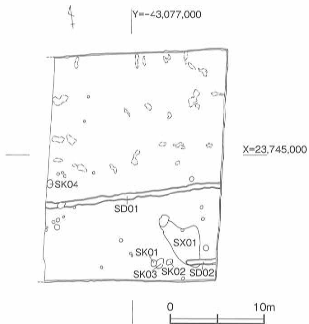
第33図 亀ノ甲・植初遺跡3次5地点 遺構配置図 [1/ 400]
