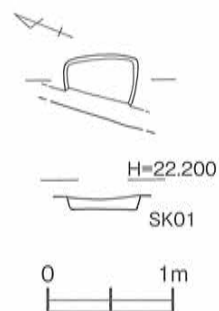
第27図 亀ノ甲・植初遺跡3次1地点 土壙 (SK01) 実測図 [1/ 60]
