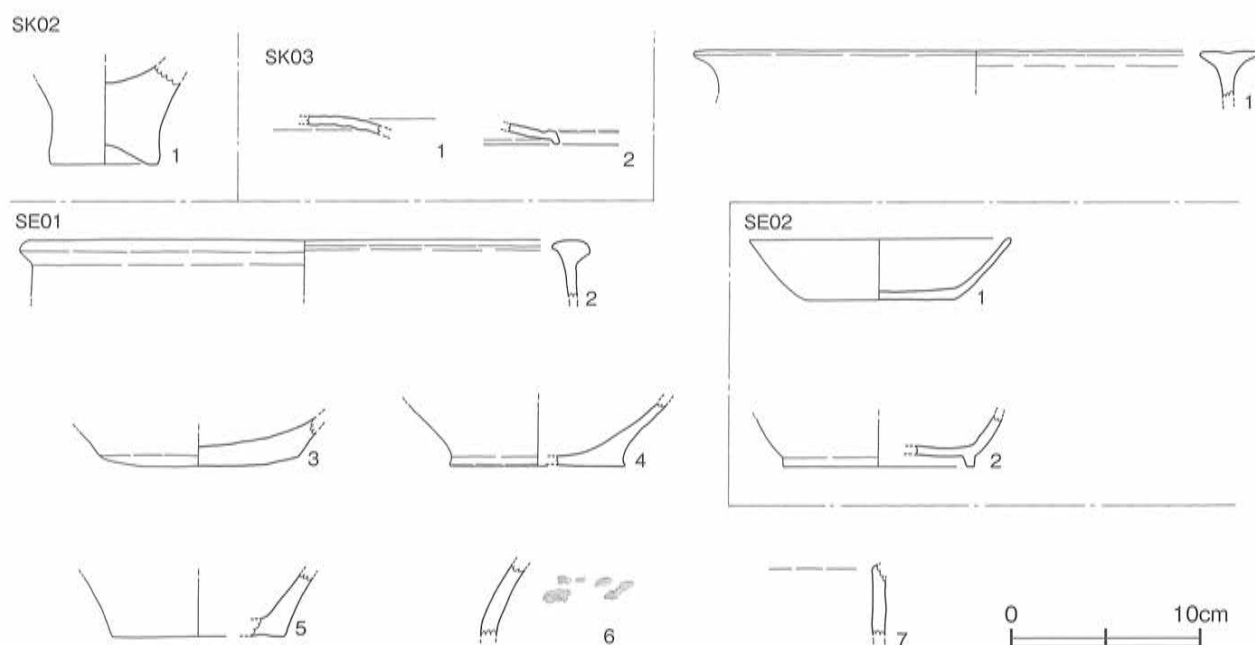
第58図 船底遺跡 土壙 (SK) 井戸 (SE) 出土土器実測図 [1/4]
