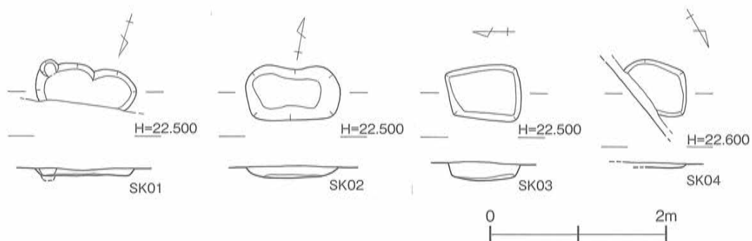
第29図 亀ノ甲・植初遺跡3次2地点 土壙 (SK01~04) 実測図 [1/ 60]
