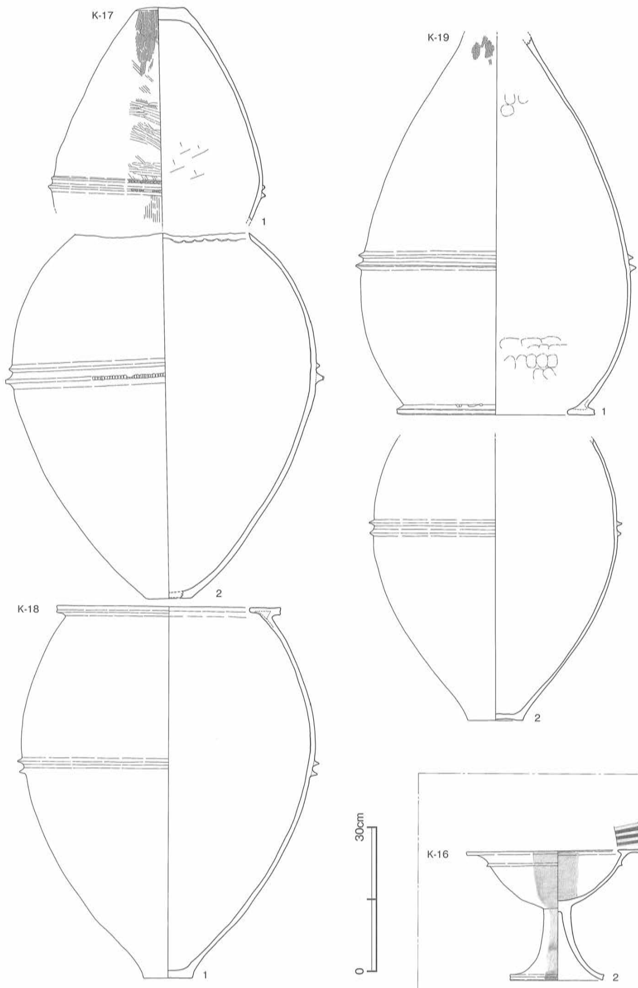
第5図 楠町遺跡2次 甕棺墓（16～19号墓）出土土器実測図〔1/8〕
