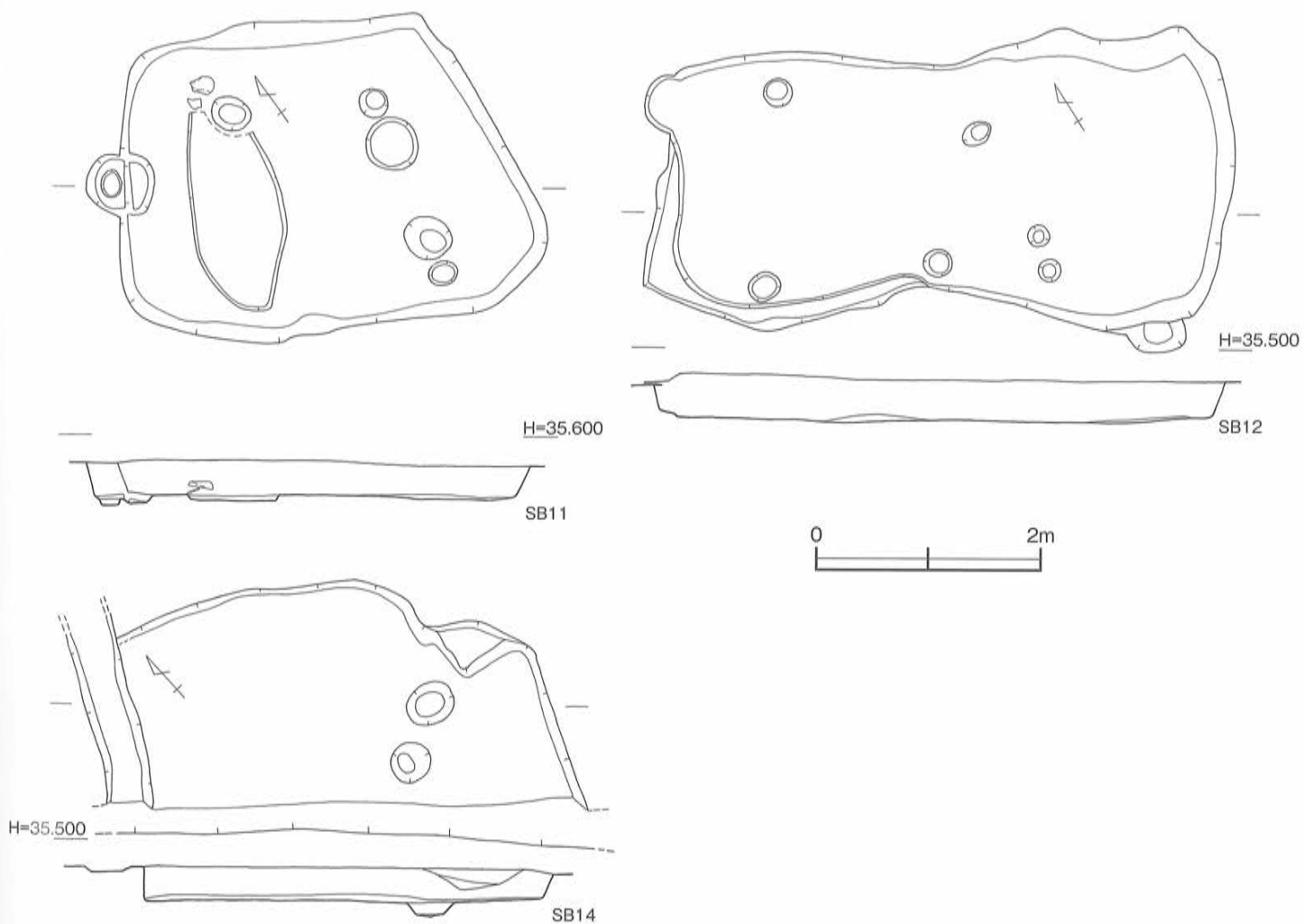
第20図 柳遺跡3次 竪穴住居 (SB11.12.14) 実測図 [1/ 60]
