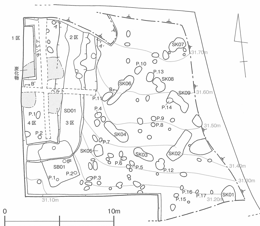
第6図 坂田遺跡 遺構配置図 [1/200]
