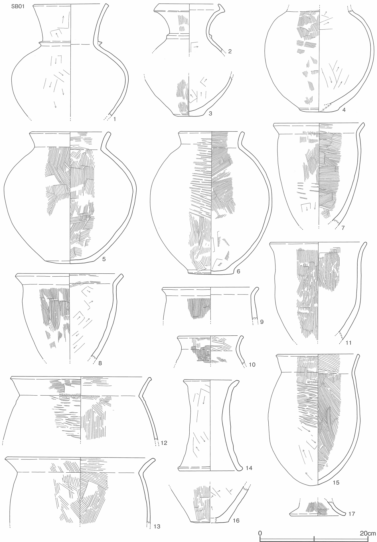
第 11 図 坂田遺跡 竪穴住居 (SB01) 出土土器実測図 [1/4]
