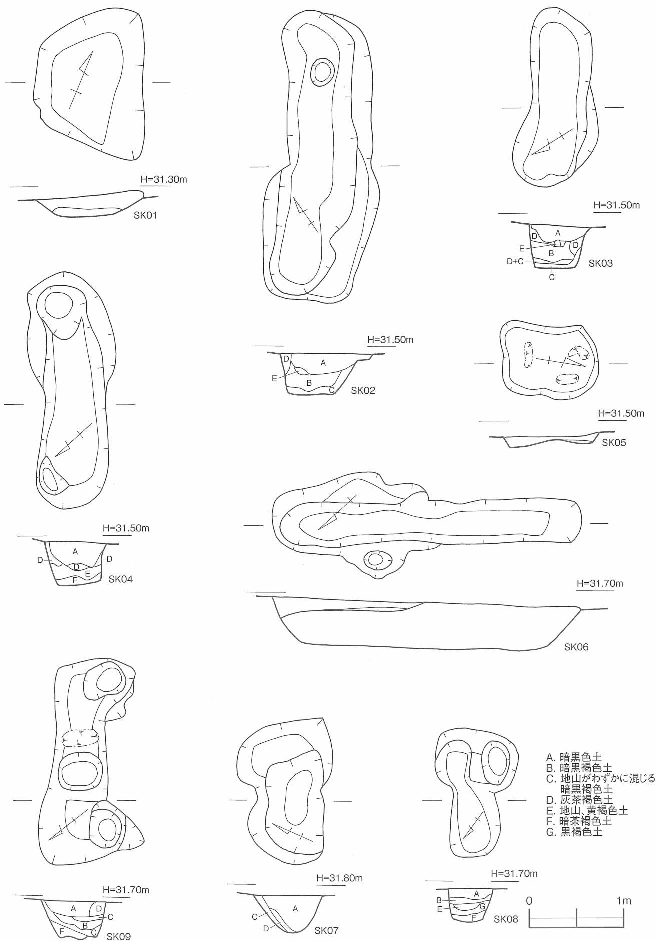
第 12 図 坂田遺跡 土壌 (SK01 ~ 09) 実測図 [1/40]
