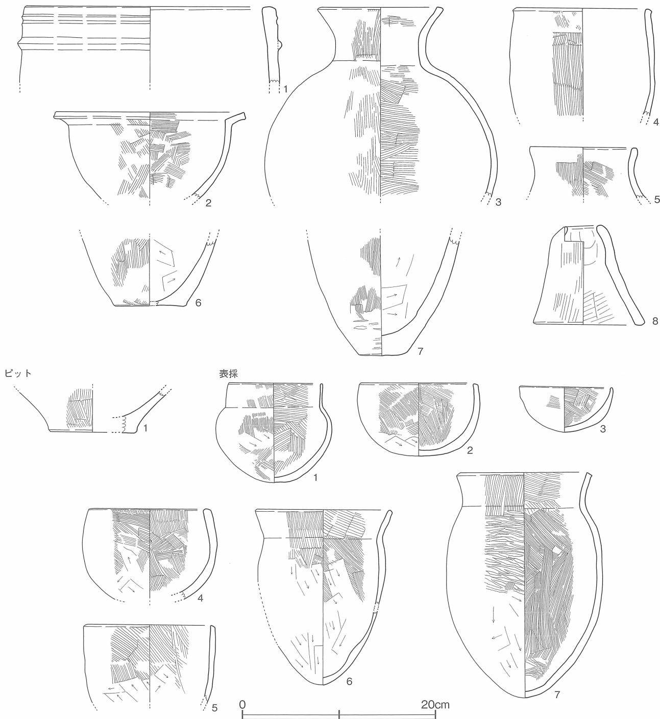
第28図 坂田遺跡 溝(SD01)ピット 表採 出土土器実測図 [1/4]
