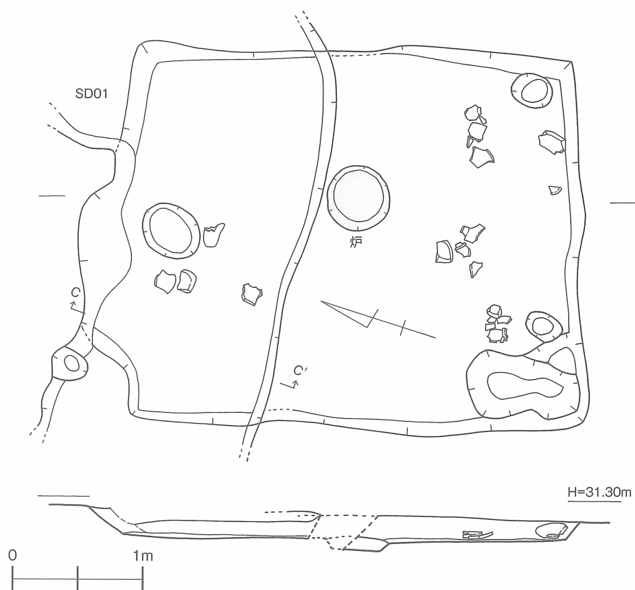
第10図 坂田遺跡 竪穴住居（SB01）実測図 [1/40]
