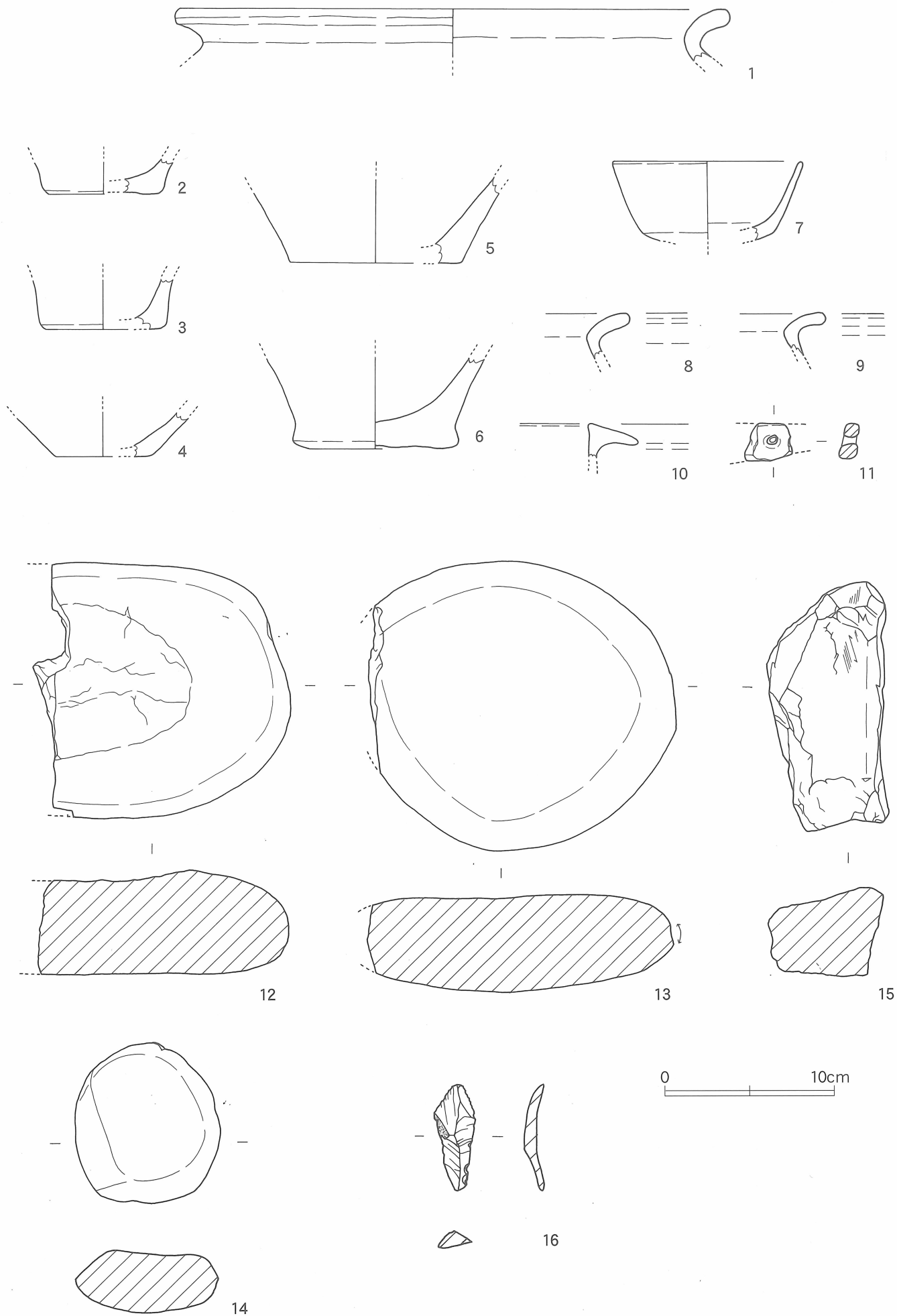
第7図 SD-03・05 出土遺物 実測図 [1/3]
