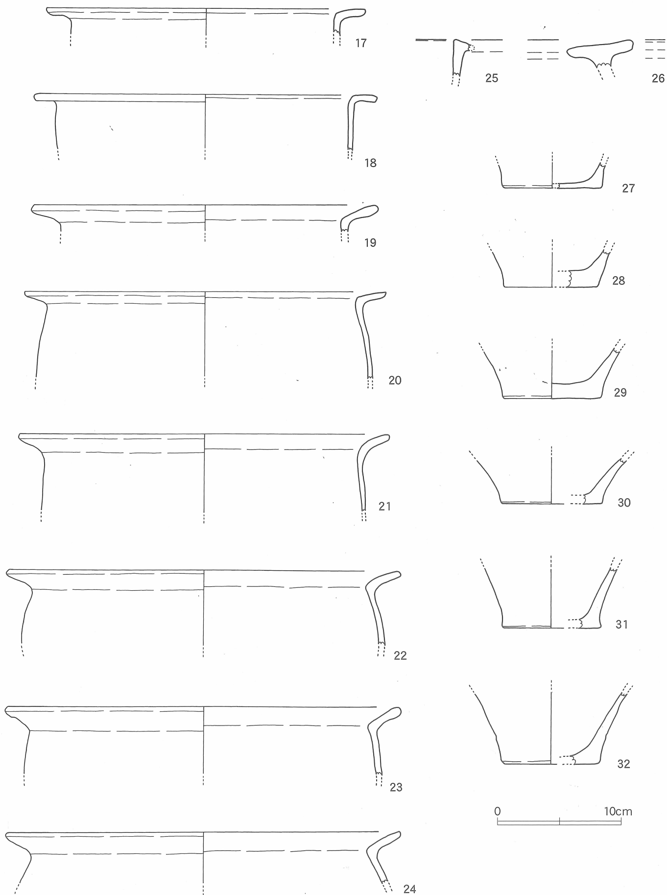
第10図 SX-01 出土遺物 実測図 [1/3]
