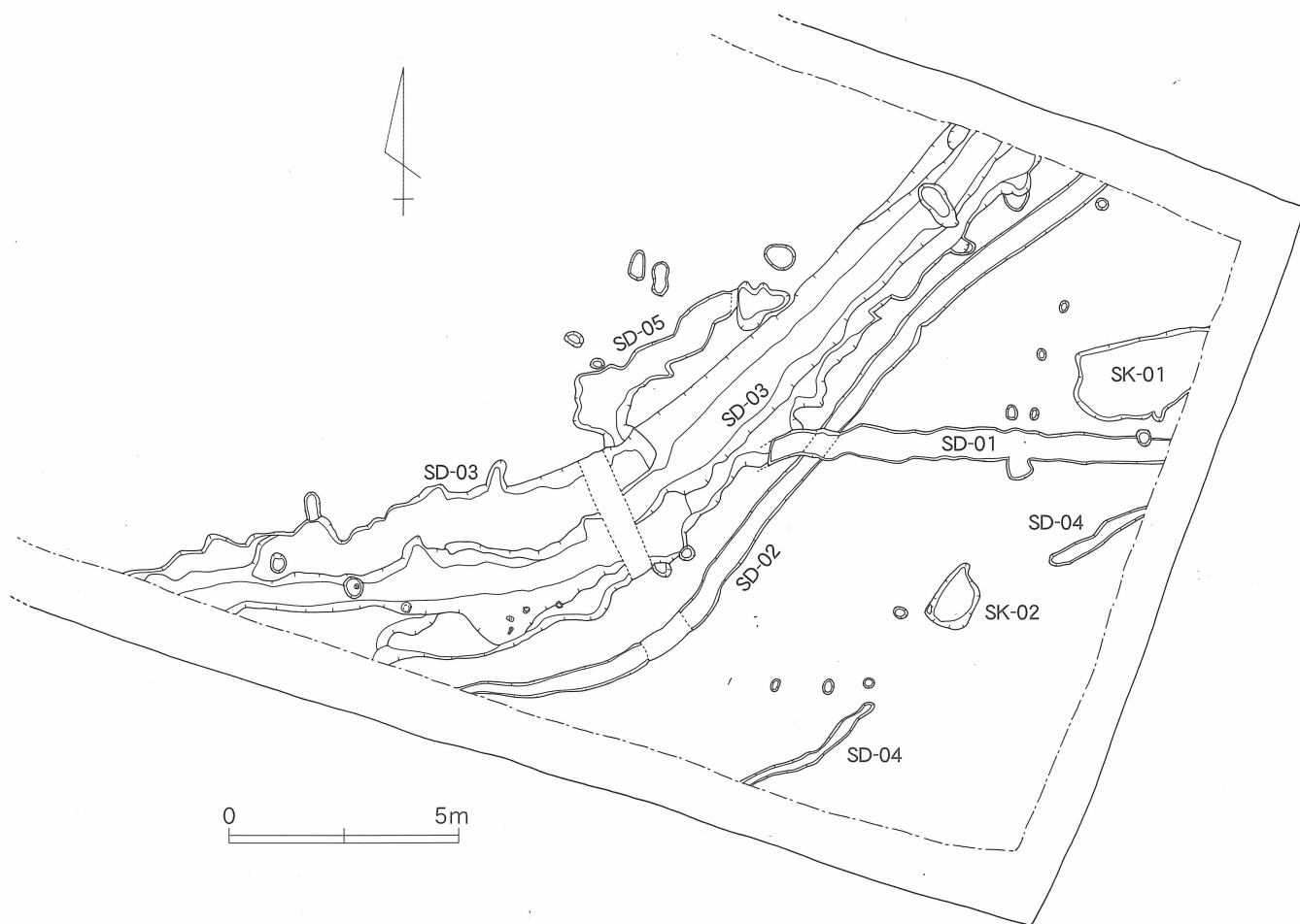
第4図 調査区東側検出遺構群 実測図 [1/160]
