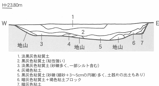
第6図 SD-03 B土層 断面実測図 [1/40]
