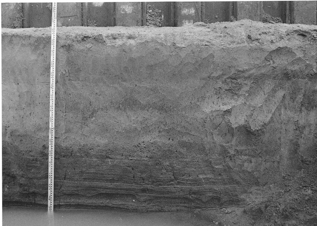
1. En-a 下基本土層(A地区0ライン)
