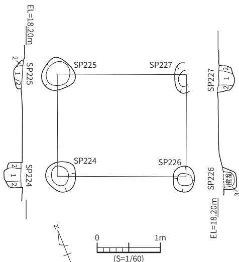
図102 SB29 遺構平面・土層断面図
