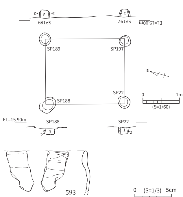
図132 SB17 遺構平面・土層断面図、出土遺物
