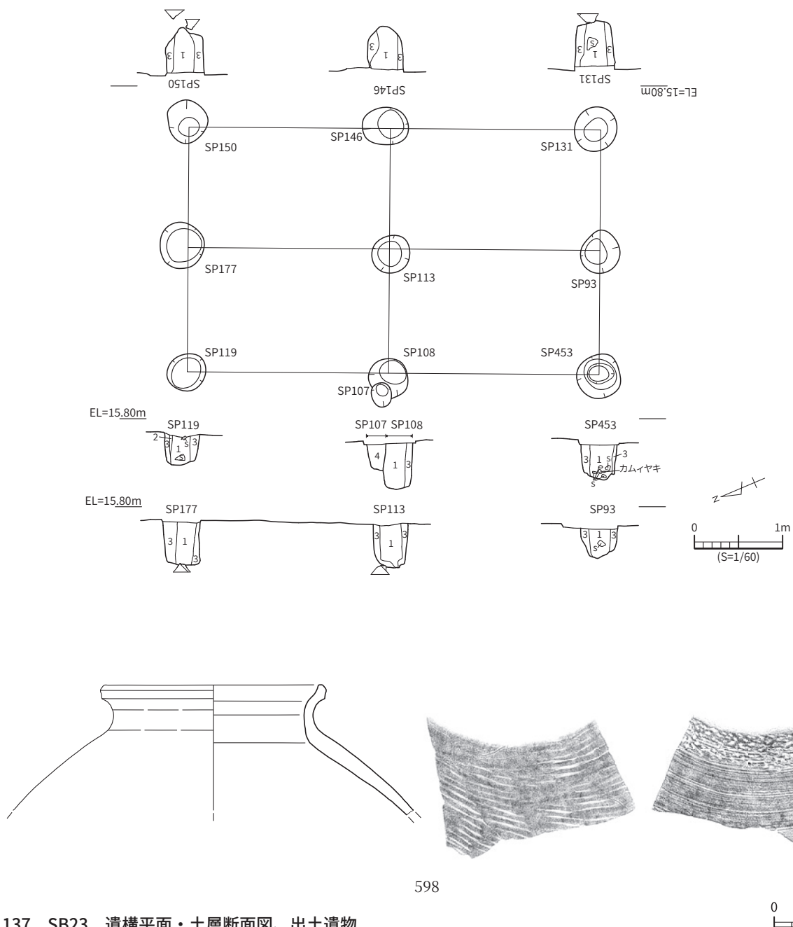
図 137 SB23 遺構平面・土層断面図、出土遺物
