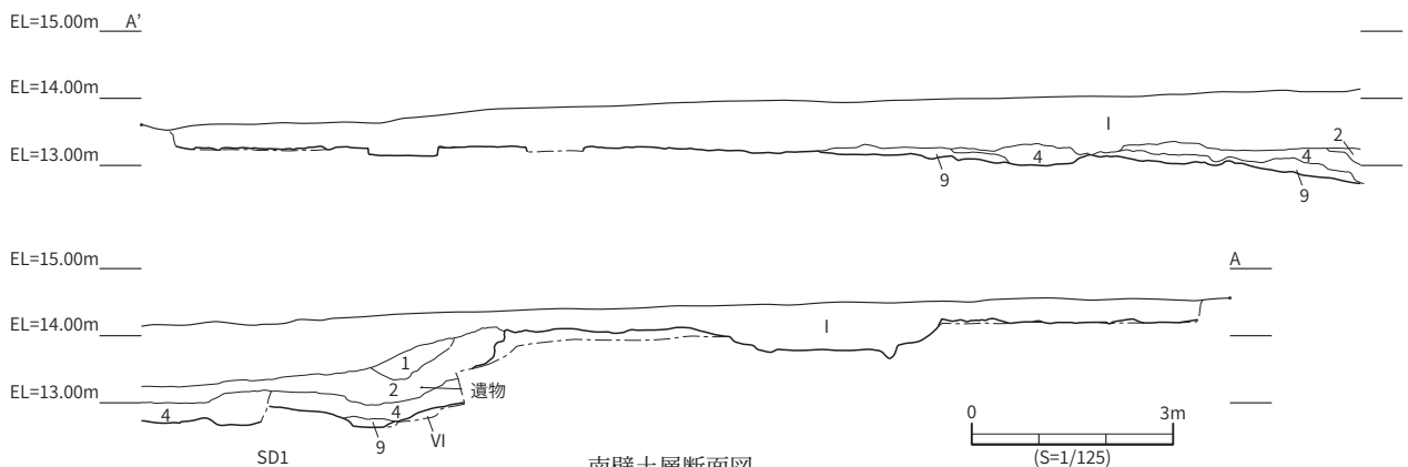
図 61 楚辺親見原遺跡 G 区 土層断面図
