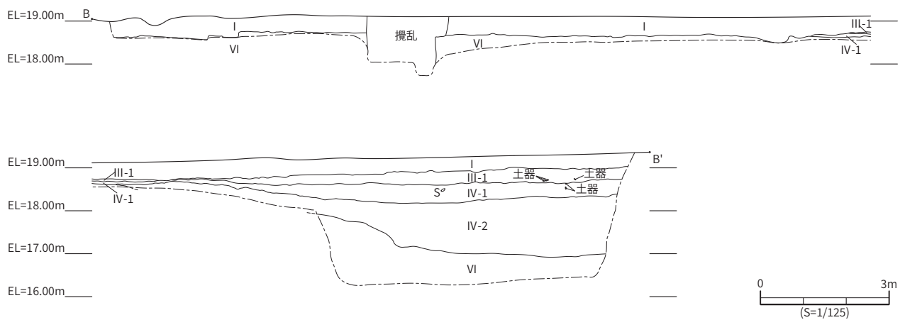
北壁土層断面図
