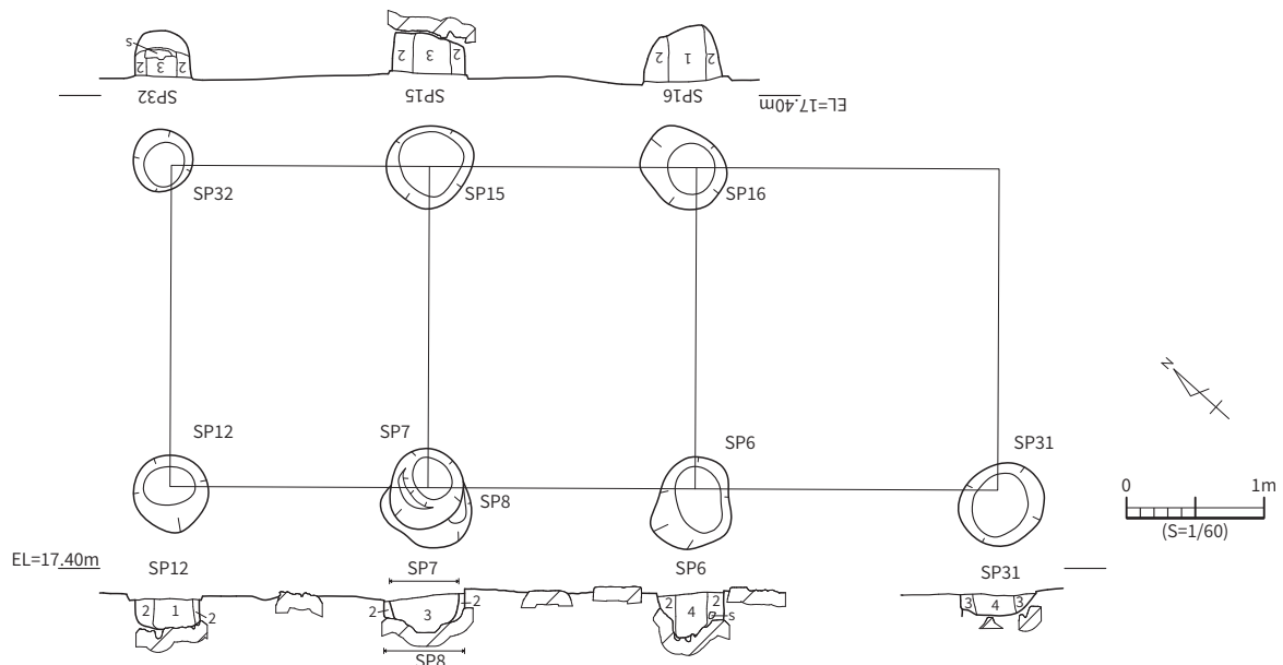
図 152 SB10 遺構平面・土層断面図
