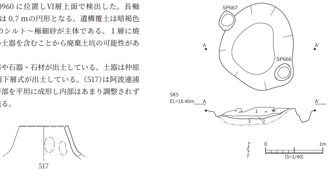
図 70 SK5 遺構平面・土層断面図、出土遺物
