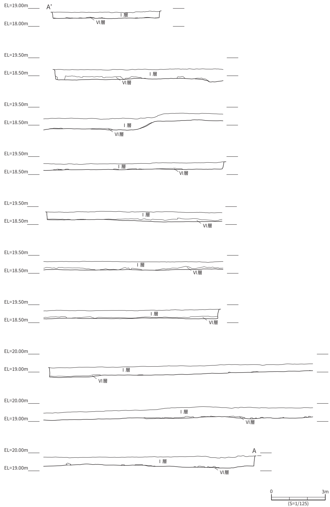
北壁土層断面図
