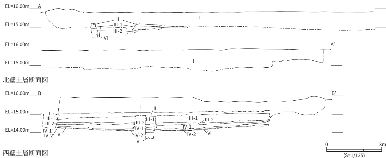
図 56 B 区 土層断面図
