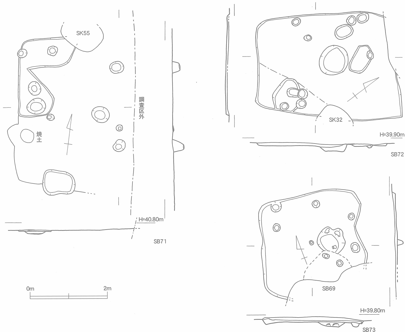
第8図 竪穴住居 (SB71・72・73) 実測図 [1/60]
