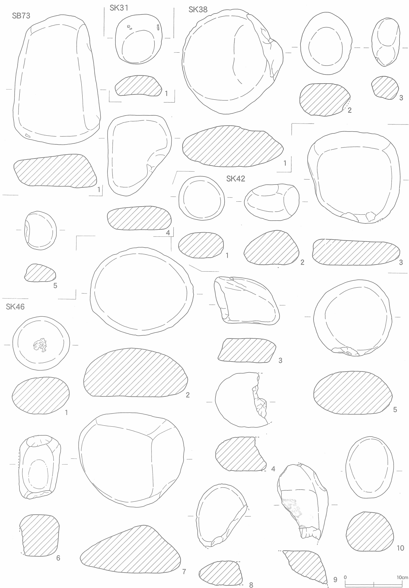
第33図 竪穴住居（SB73）、土坑（SK31・38・42・46）出土石器実測図 [1/4]
