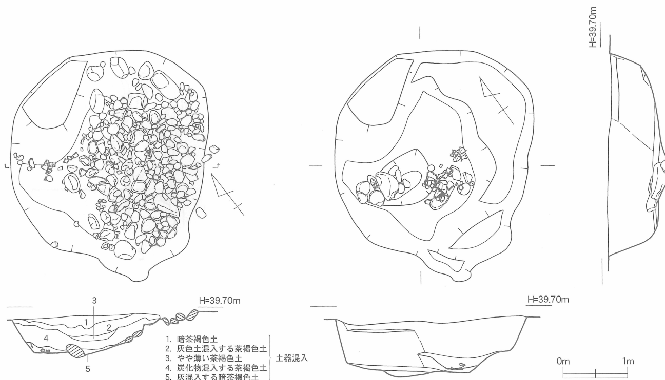
第12図 土坑（SK50）実測図 [1/60]
