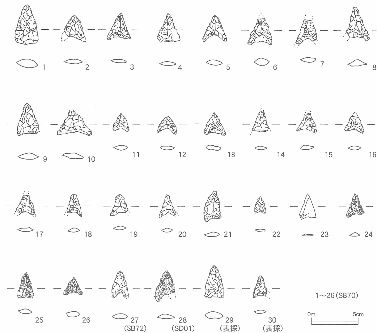
第30図 竪穴住居(SB70・72)、溝(SD01)、表採出土石器実測図 [1/2]
