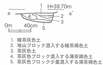
第14図 溝 (SD01) 土層実測図 [1/40]
