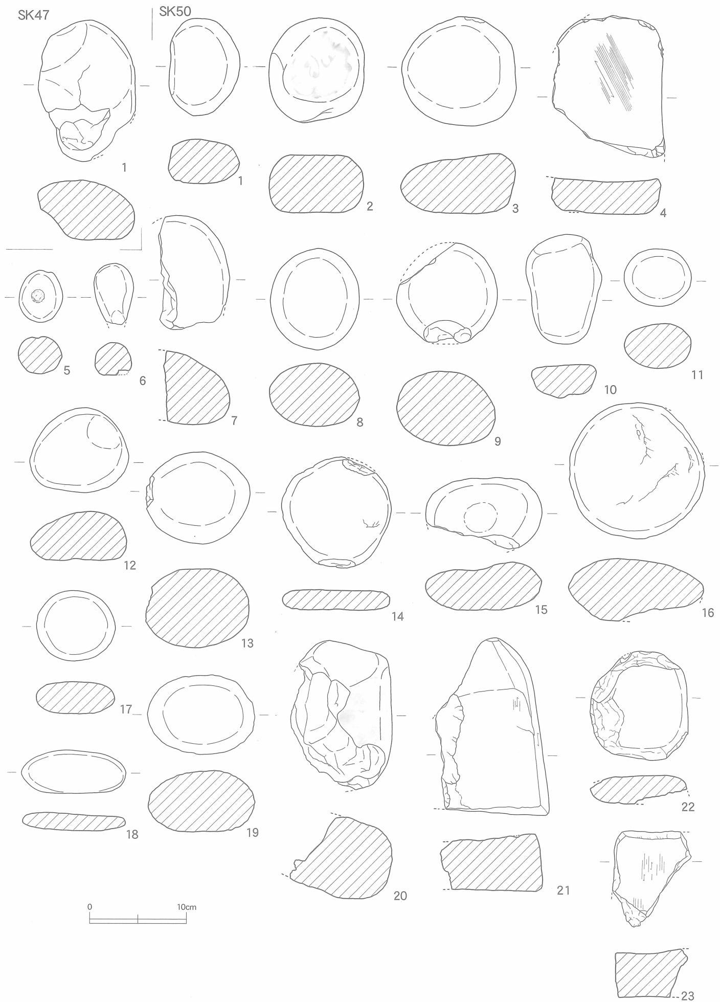
第34図 土墳（SK47・50）出土石器実測図 [1/4]
