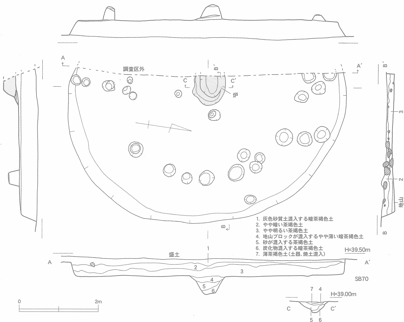
第7図 竪穴住居 (SB68・69・70) 実測図 [1/60]
