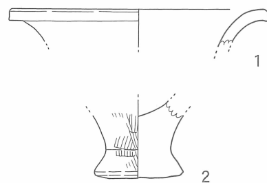
第17図 竪穴住居（SB70その2・73）出土土器実測図 [1/4]
