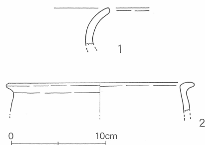
第25図 溝(SD01)出土 土器実測図 [1/4]
