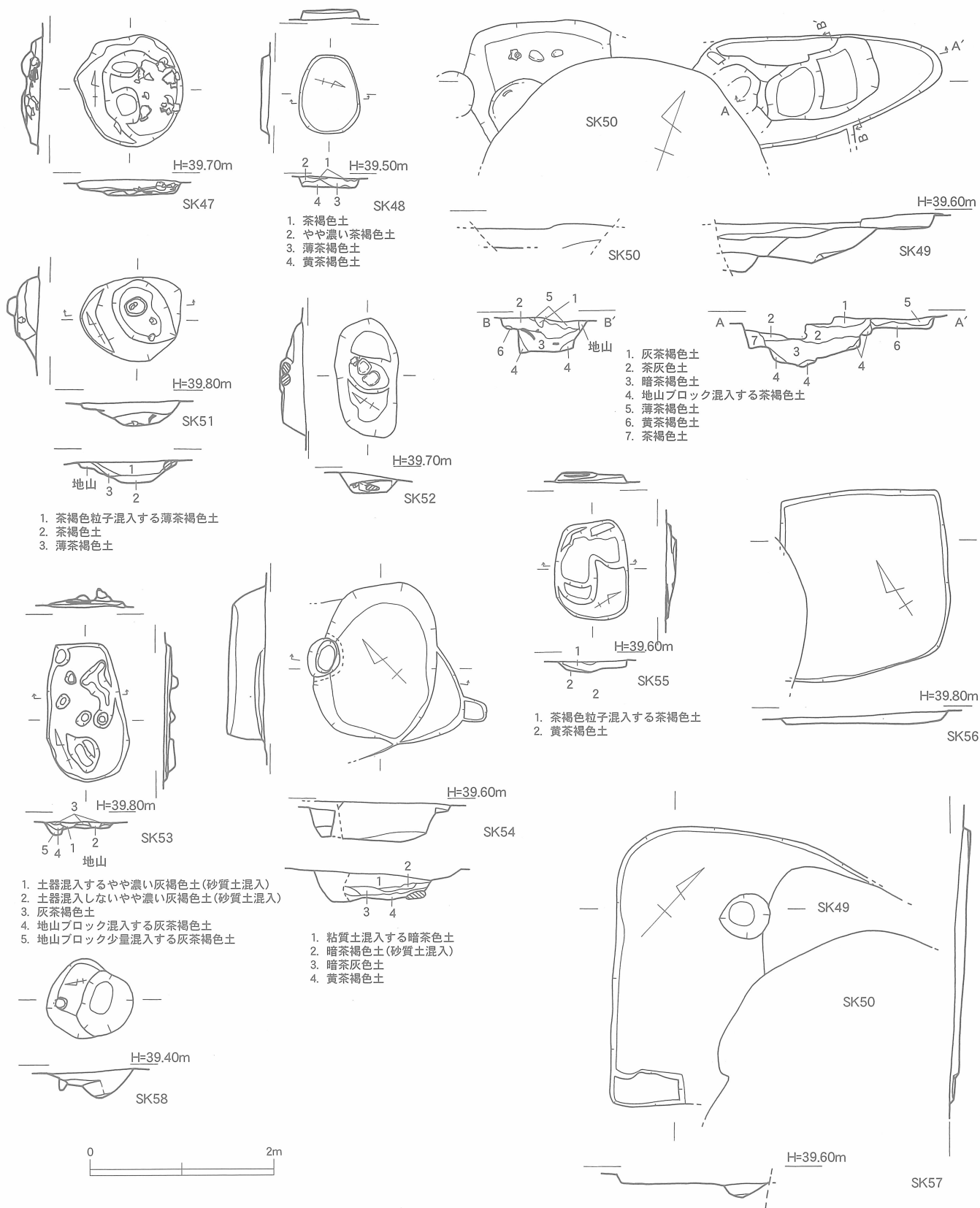
第11図 土壌 (SK47~49・51~58) 実測図 [1/60]
