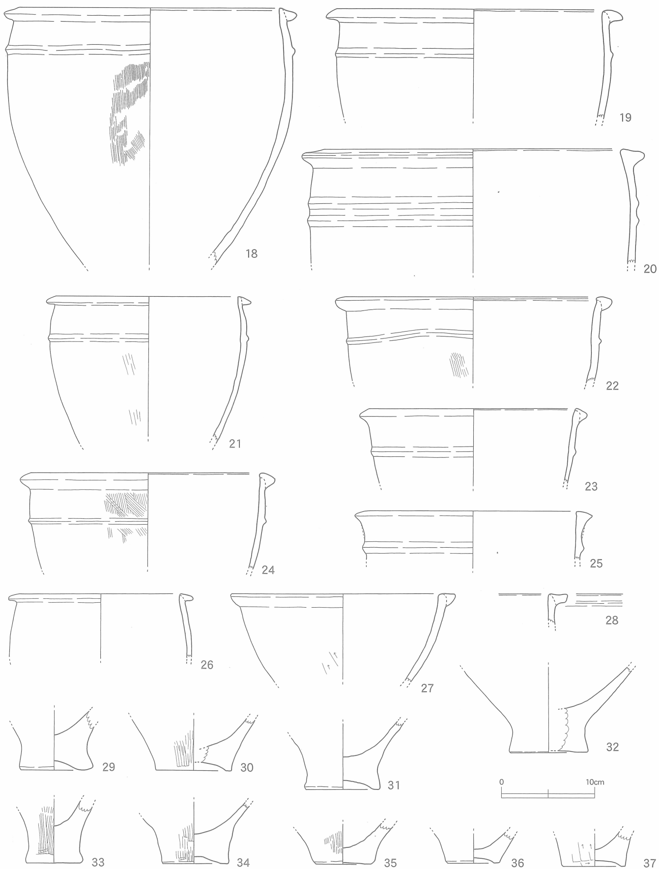
第 2 2 図 土墳（SK50その2）出土土器実測図 [1/4]
