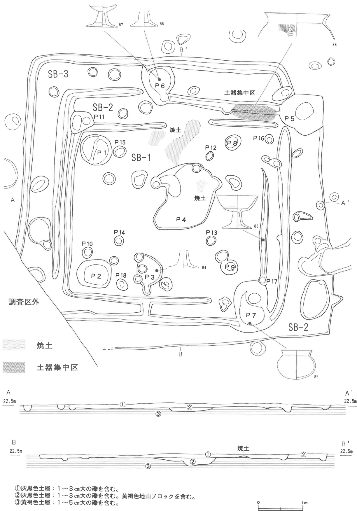
SB-1・2・3実測図 (1/50)
