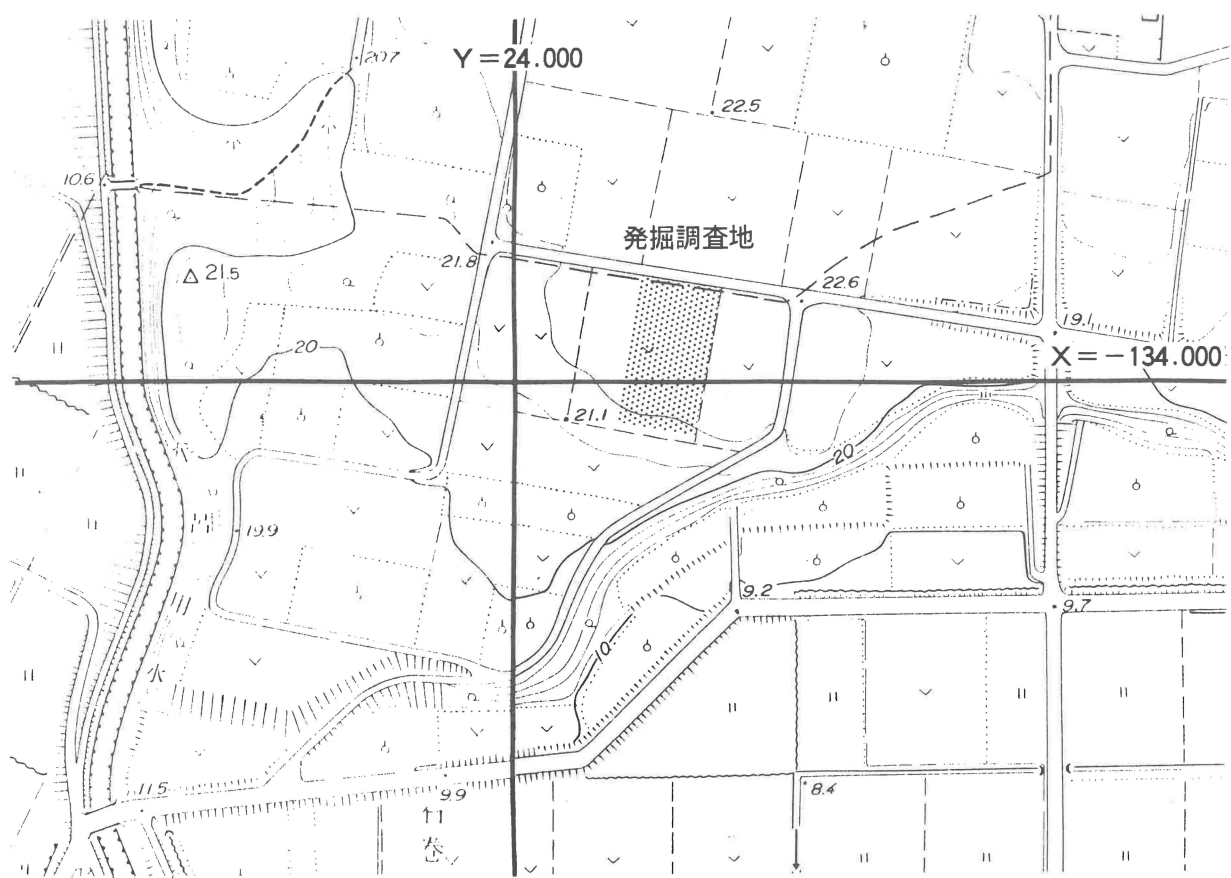
第3図 高井遺跡周辺地形図-3 (1/2,500 1980年 豊橋市都市計画基本図)
