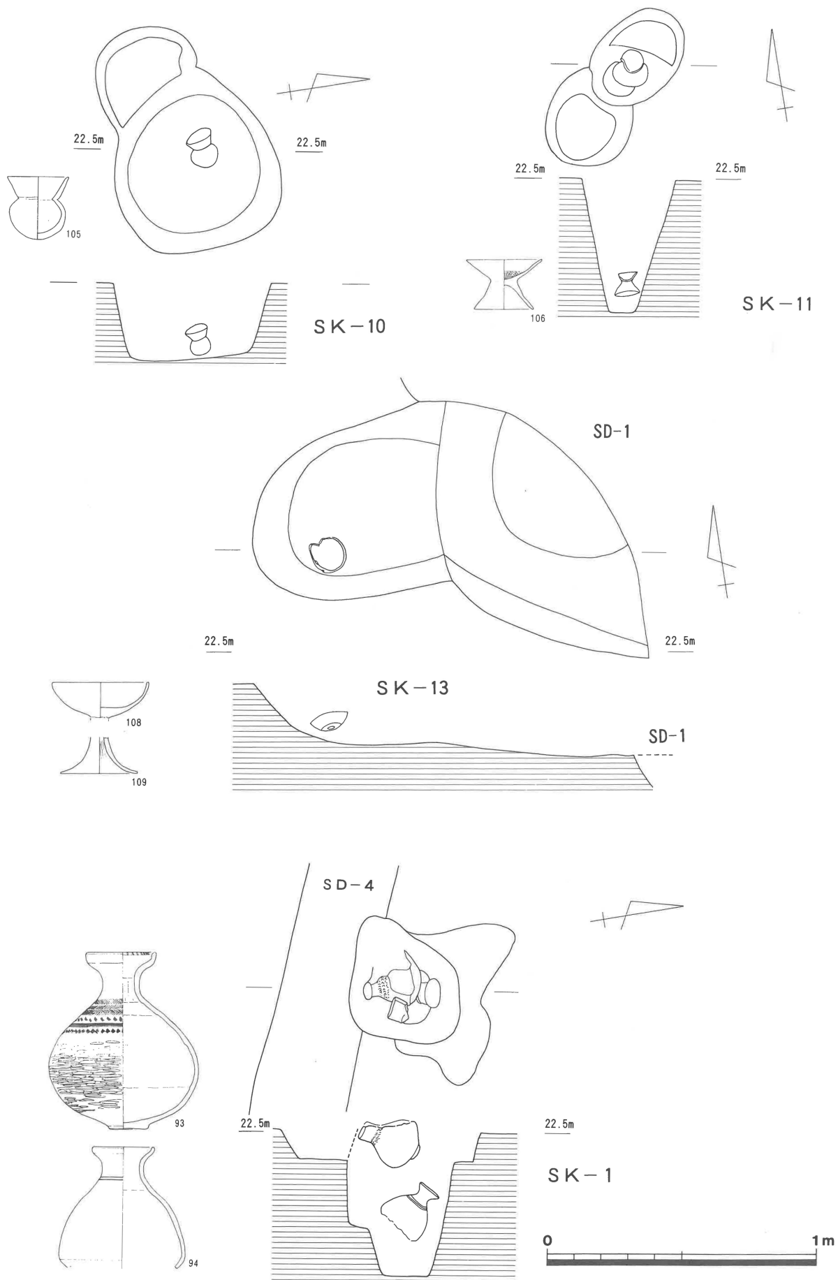
SK-1・10・11・13遺物出土状況図 (1/20)
