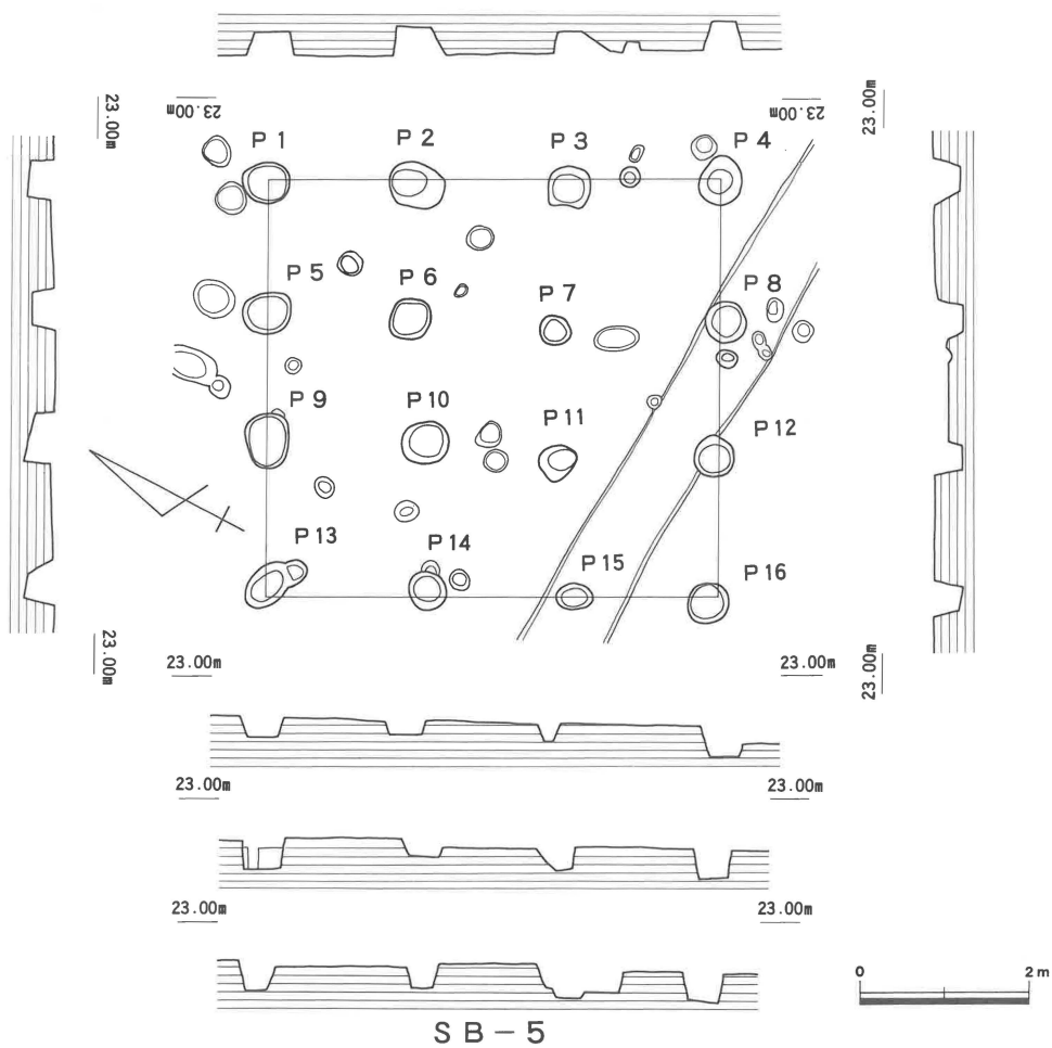
S B - 4 ・ 5 実測図 ( 1 / 100 )
