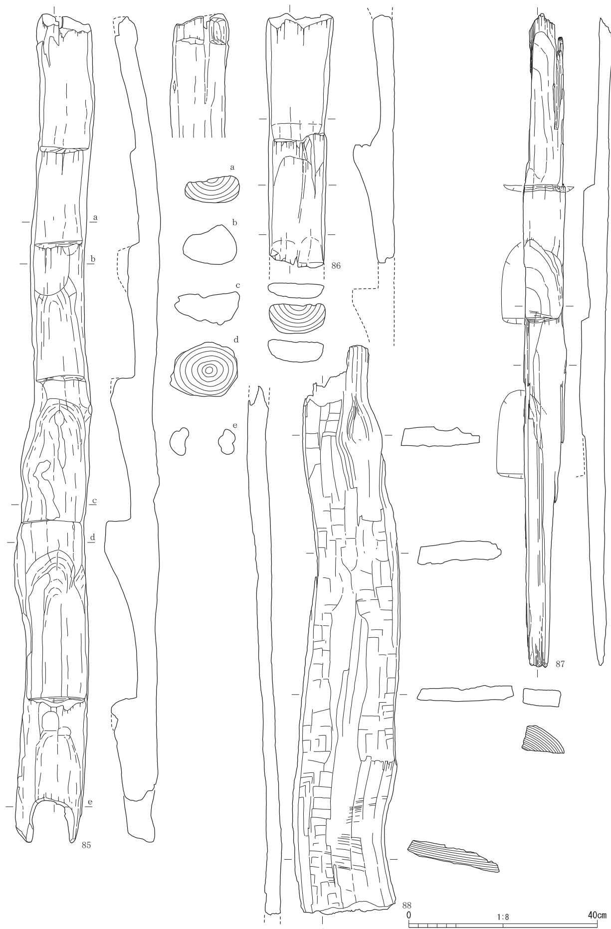
図 58 D層出土木製品 (14) 〈梯子〉
