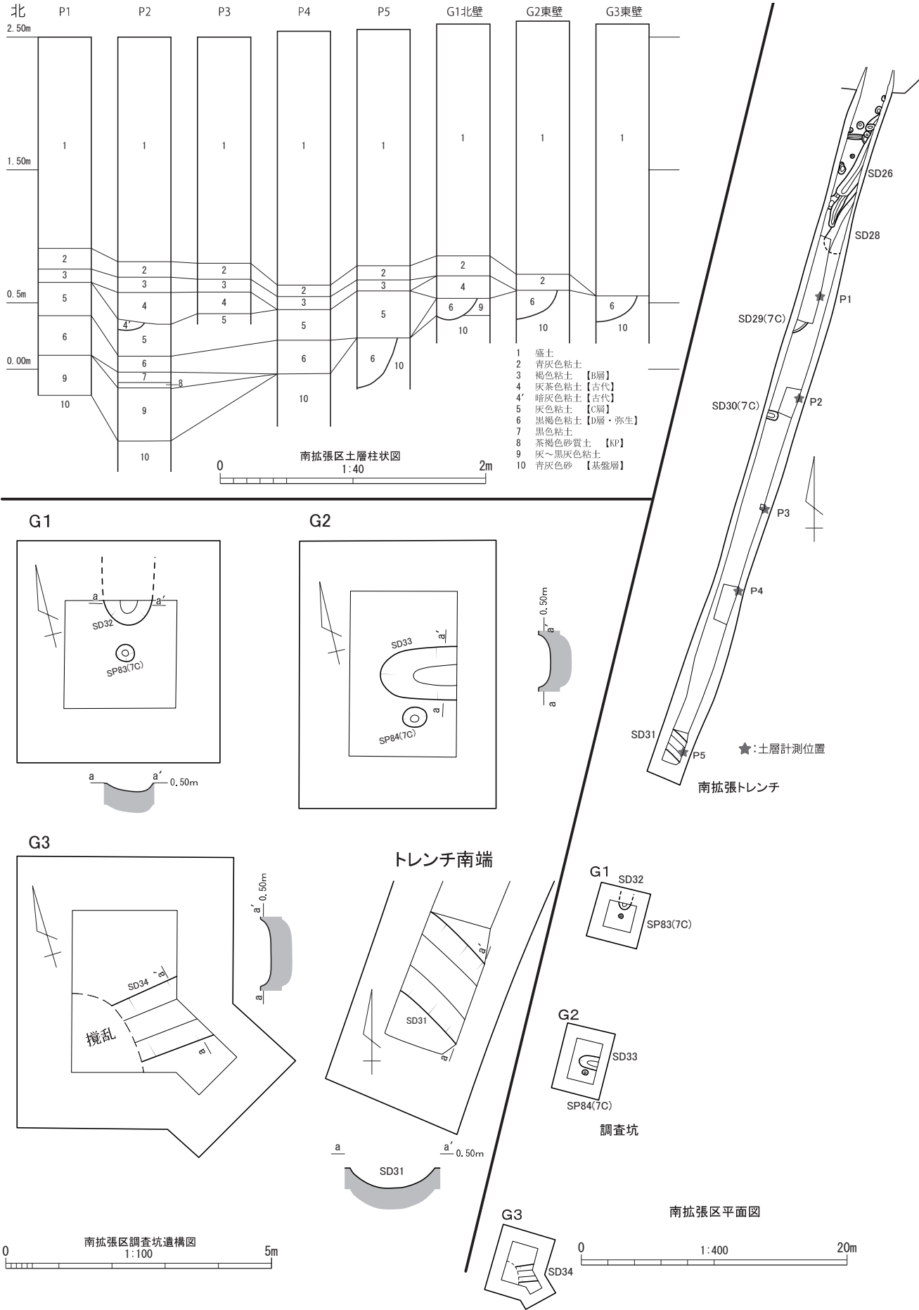
図 23 南拡張区遺構全体図・土層柱状図
