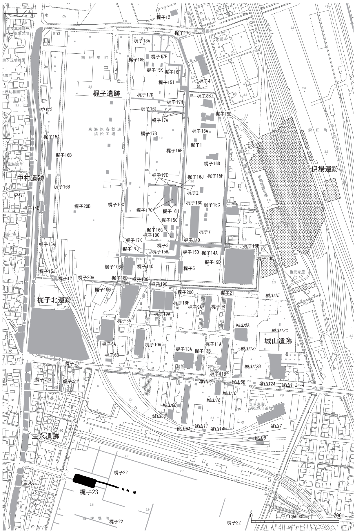
図5 櫓子遺跡 23次調査区位置図
