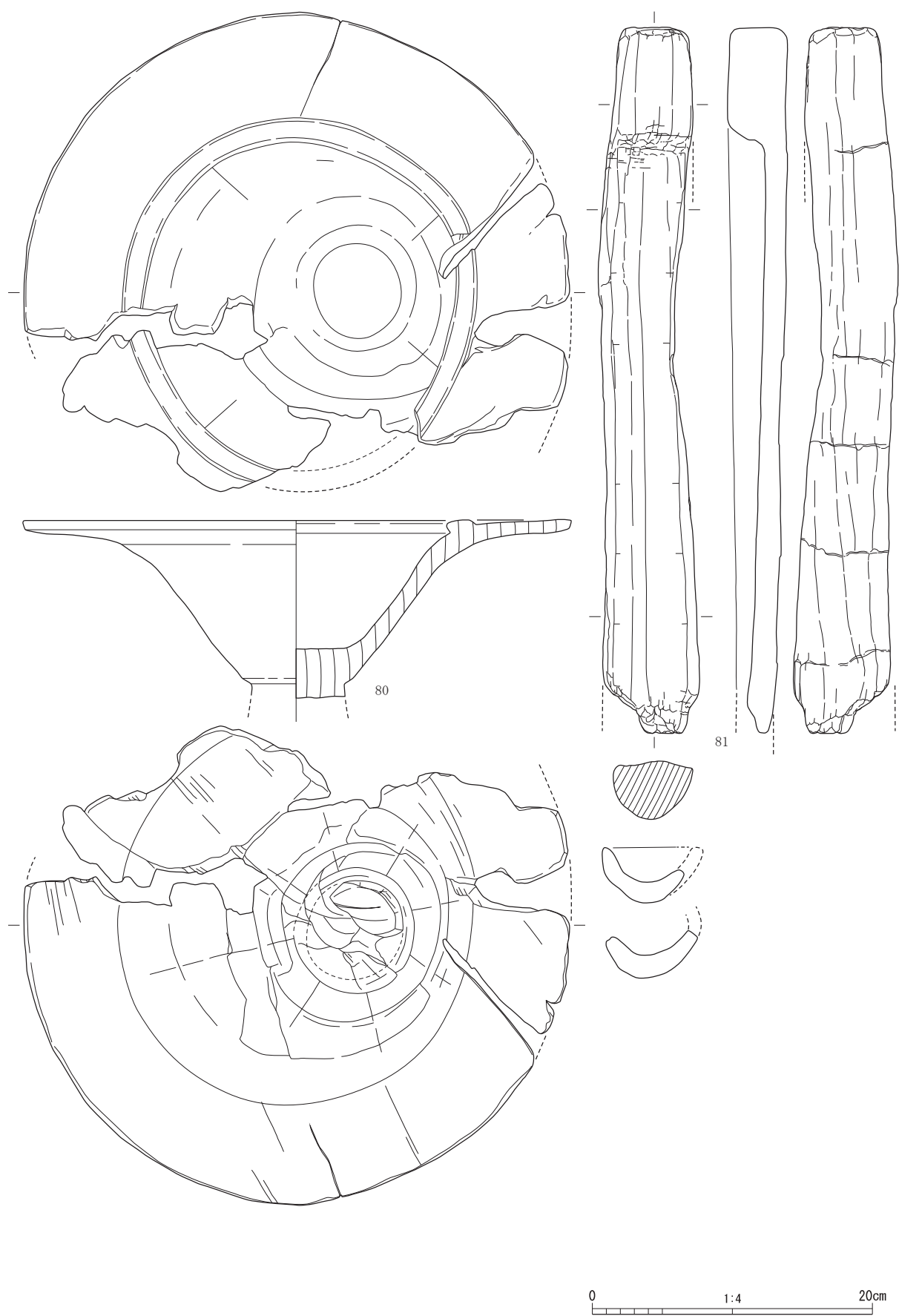
图 56 D層出土木製品 (12) 〈高杯・槽〉
