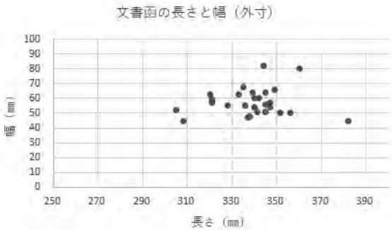
図 69-1 文書函の長さと幅の関係（外寸）
