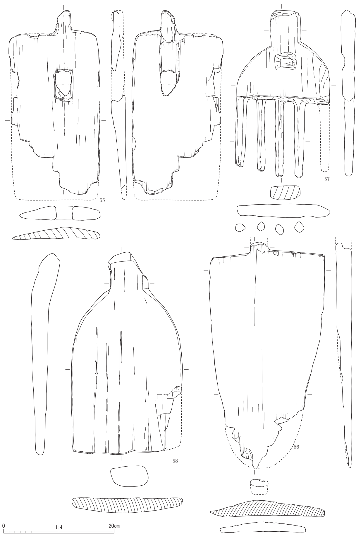
図 51 D層出土木製品(7)〈鍬・鋤〉
