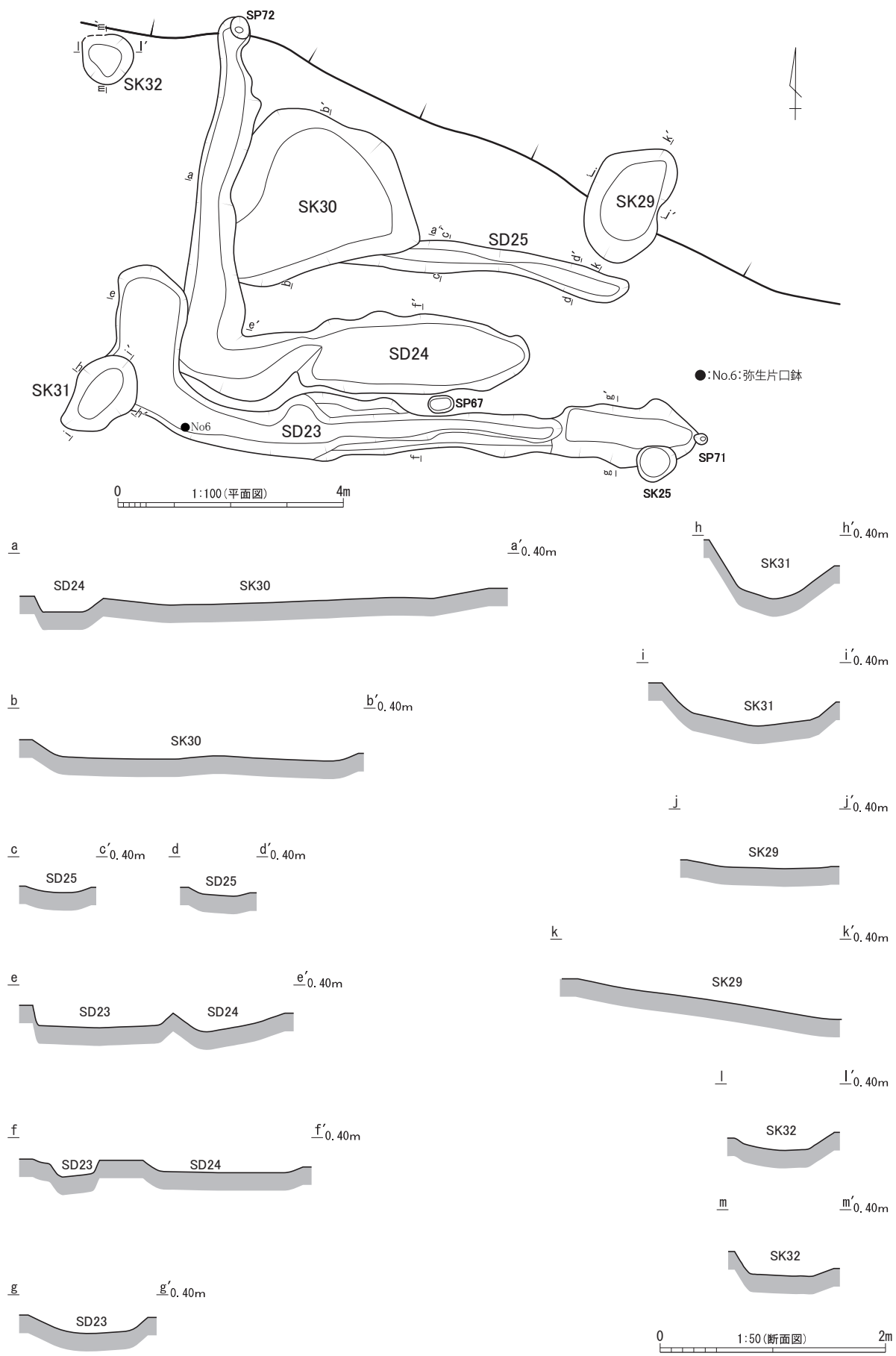
図 18 南微高地弥生時代遺構図（土坑・溝）
