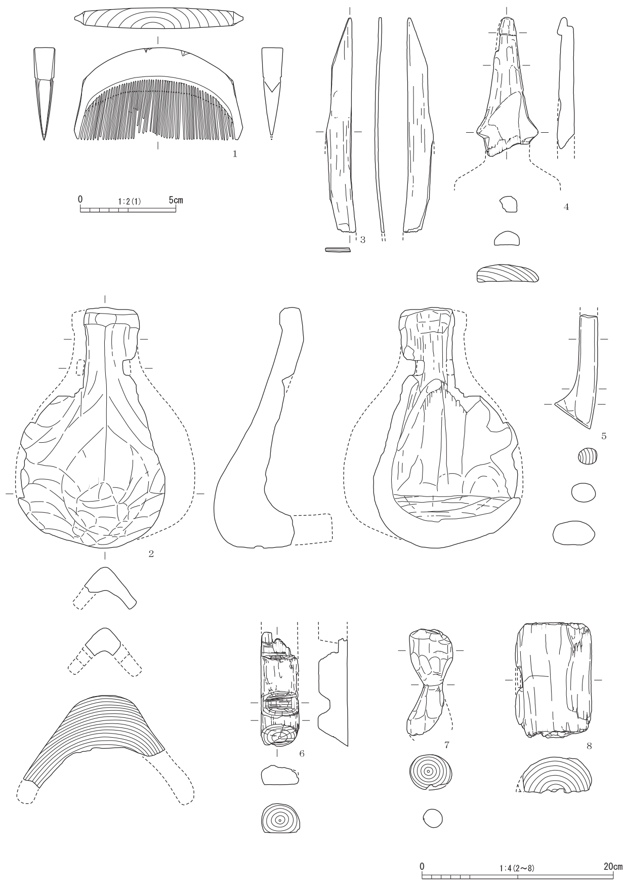
図 45 大溝出土木製品（1）〈Ⅶ層①〉
