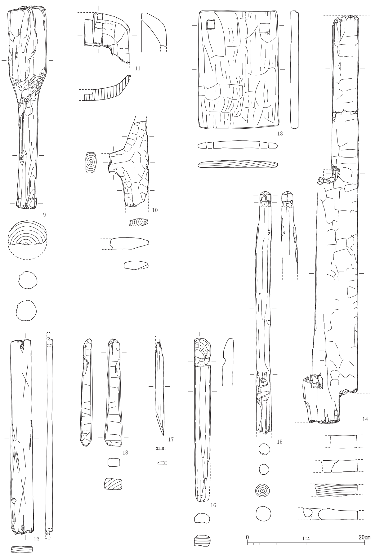
図 46 大溝出土木製品（2）〈Ⅶ層②〉
