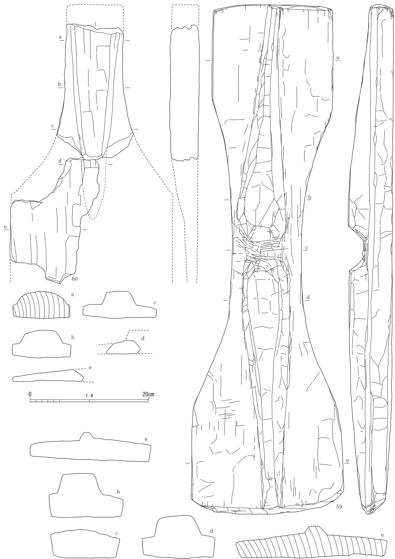
图 52 D層出土木製品（8）〈鍬未成品〉
