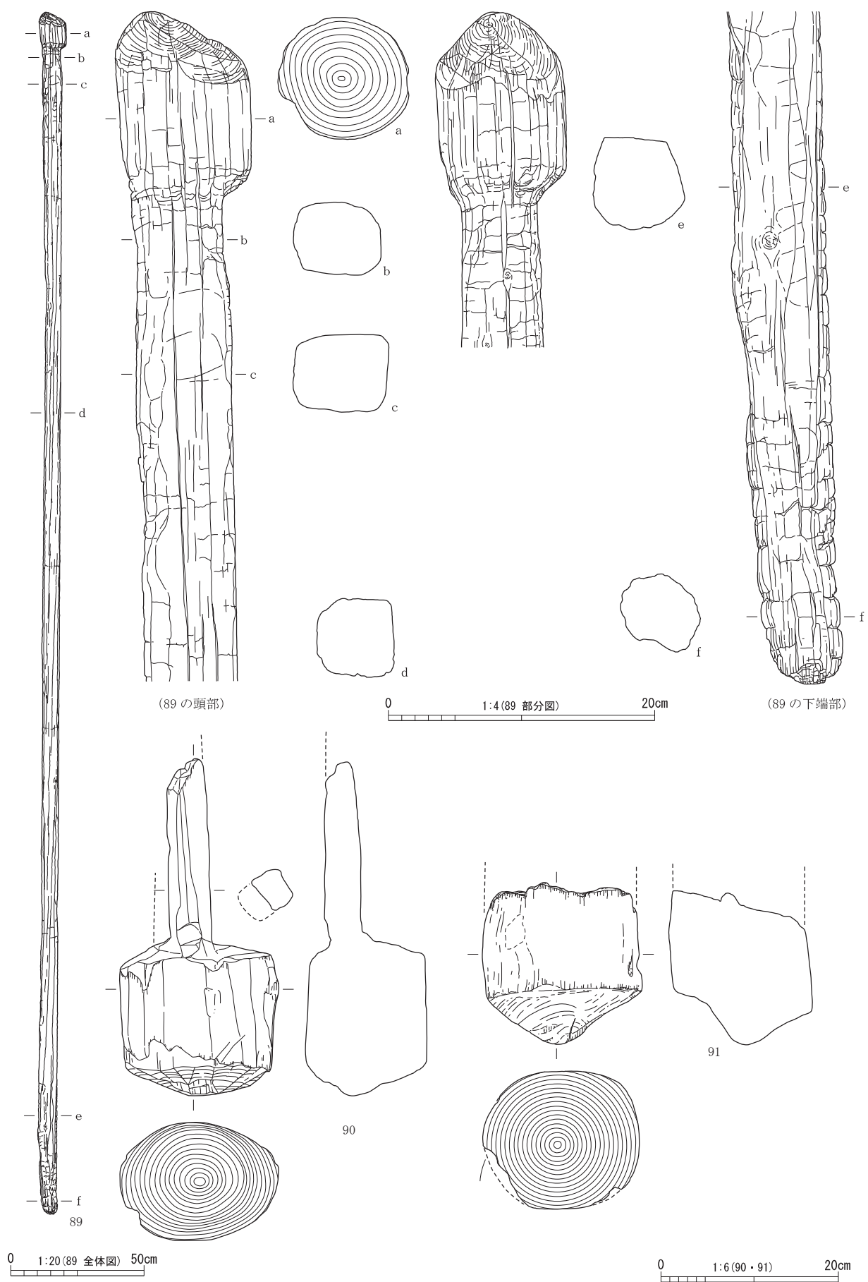
図 59 D層出土木製品 (15) 〈垂木・柱根〉
