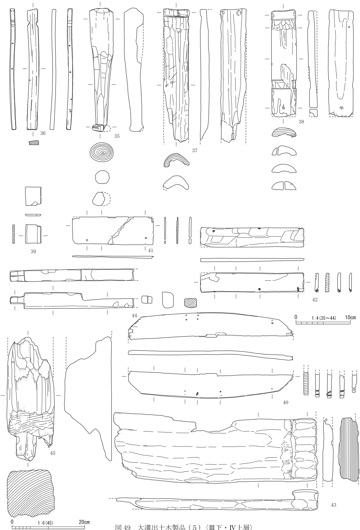
图 49 大溝出土木製品 (5) 〈Ⅲ下・Ⅳ上層〉
