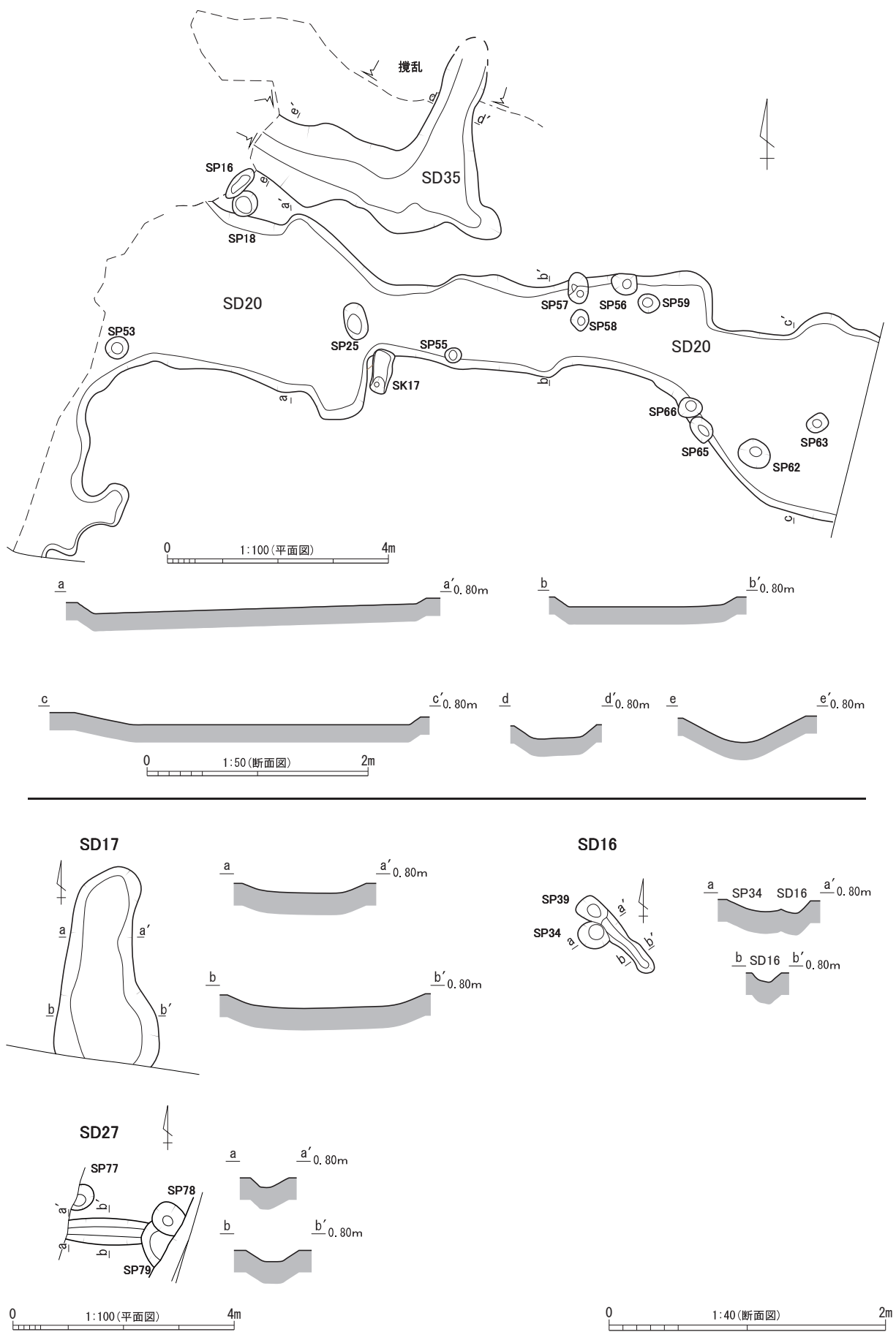
図 19 南微高地弥生時代遺構図（溝）
