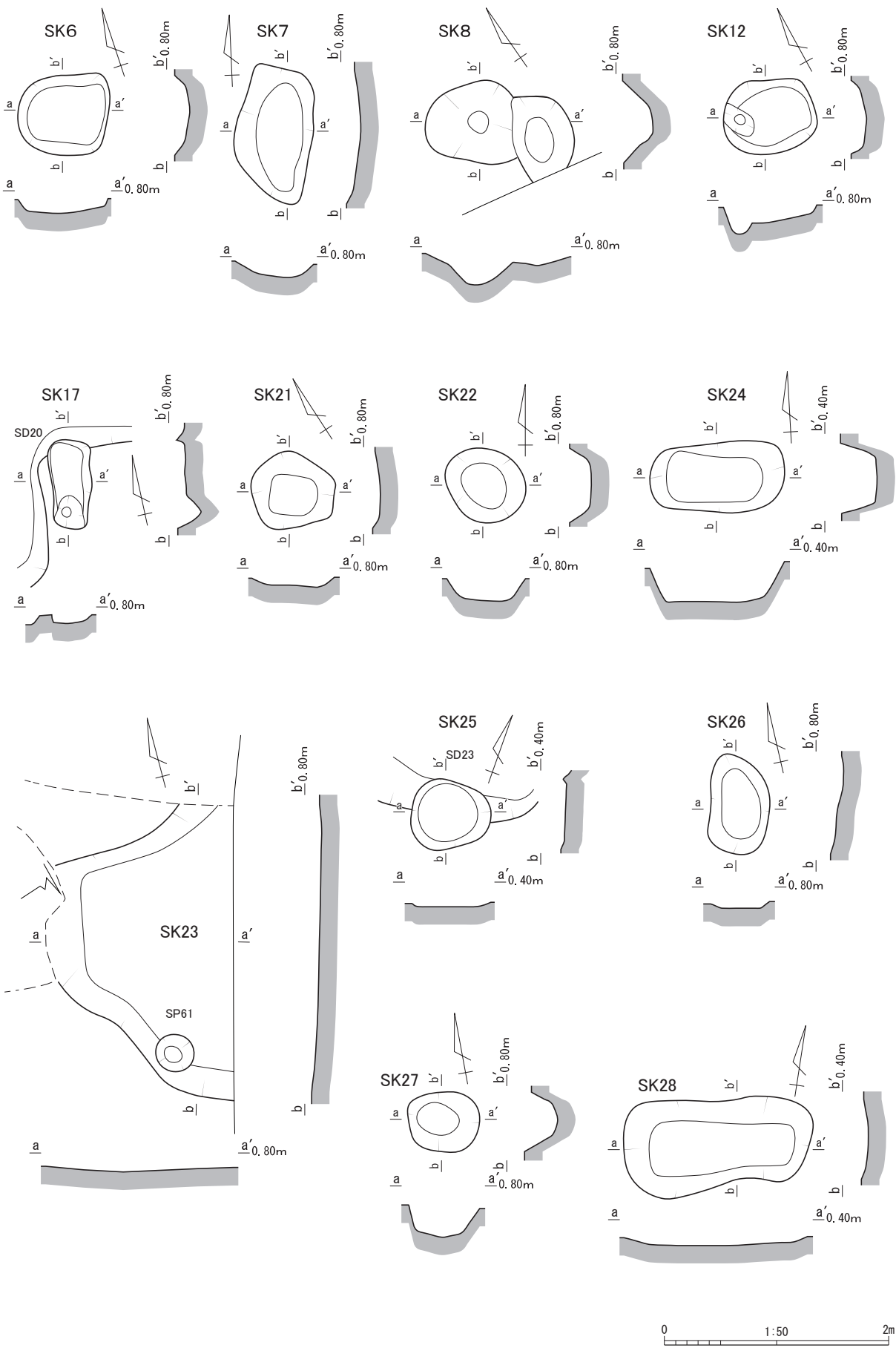
図 20 南微高地弥生時代遺構図（土坑）
