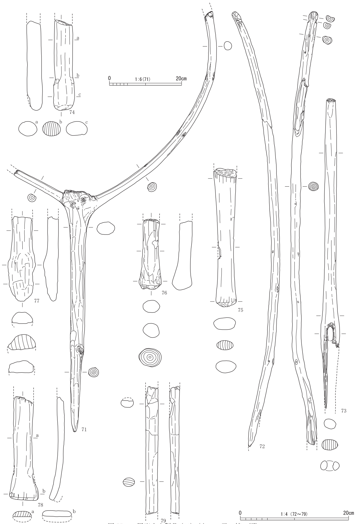
図 55 D層出土木製品 (11) 〈タモ・弓・柶・柄〉
