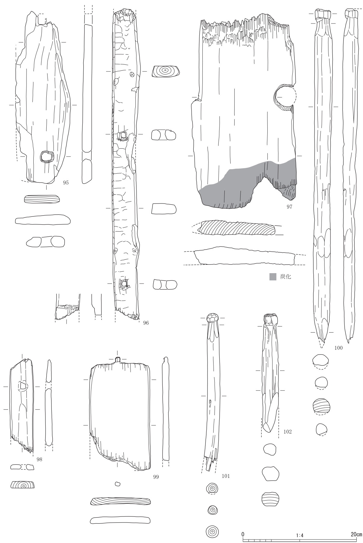
図 61 D層出土木製品 (17) 〈有孔板・出柄板・有頭棒〉
