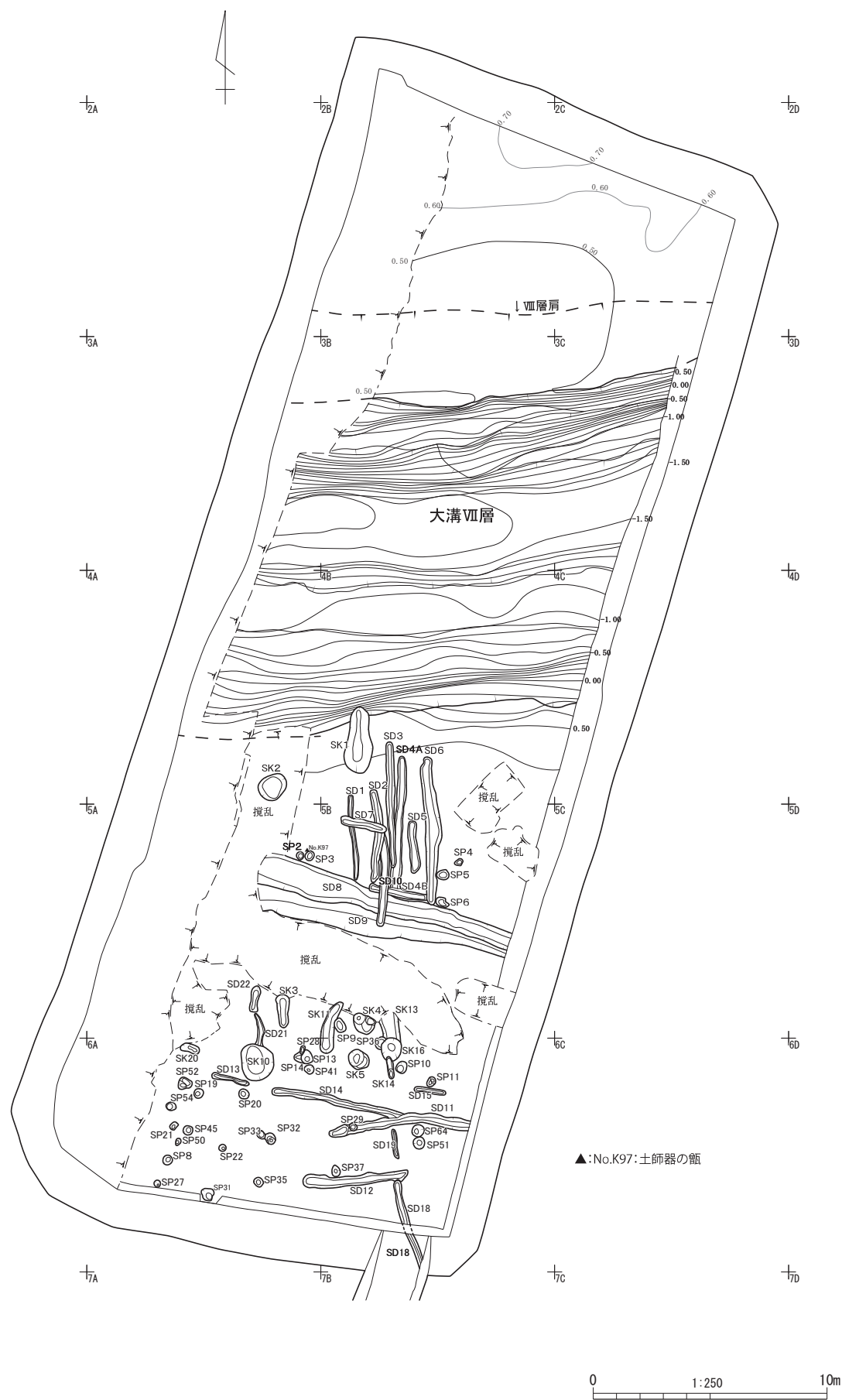
図8 大溝Ⅶ層・南区古代面（飛鳥時代）全体図
