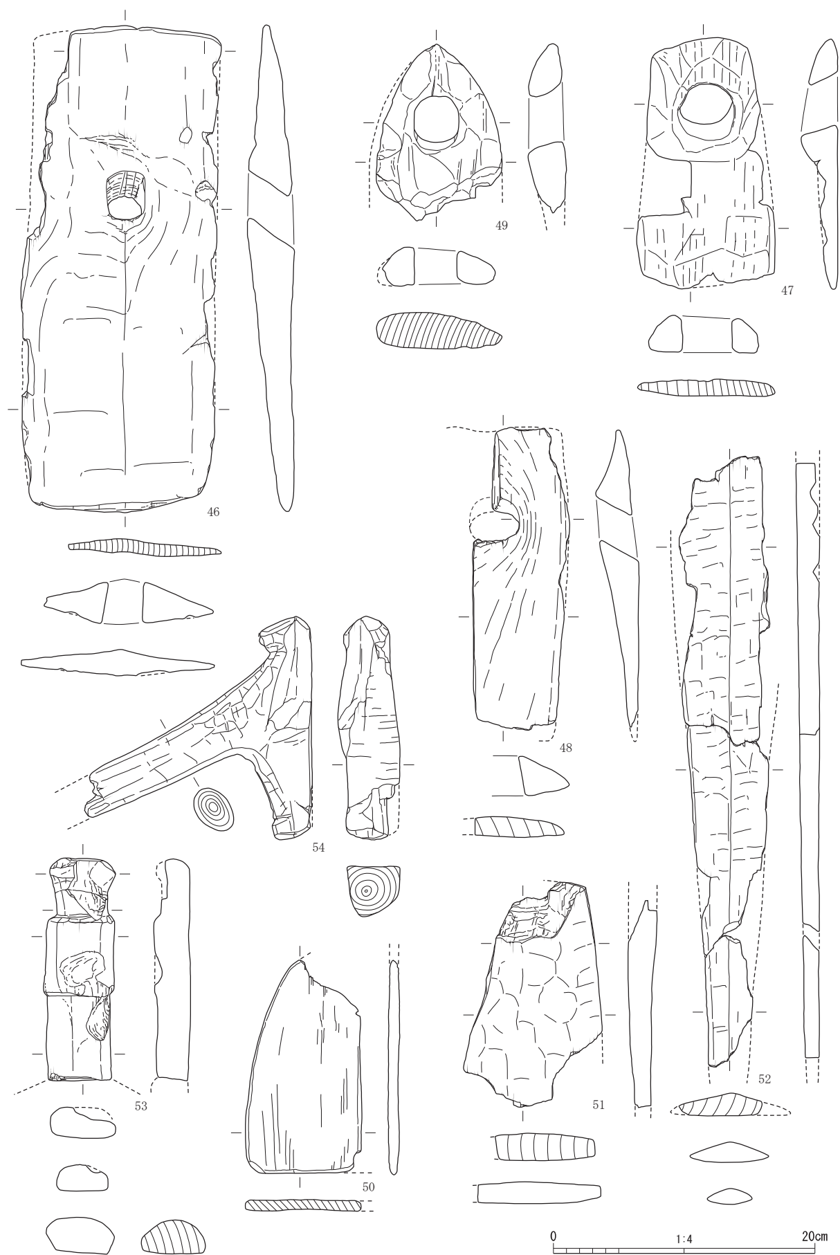
図 50 D層出土木製品（6）〈鍬〉
