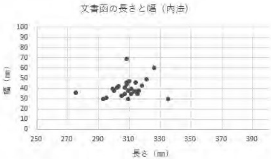
図 69-2 文書函の長さと幅の関係（内法）
