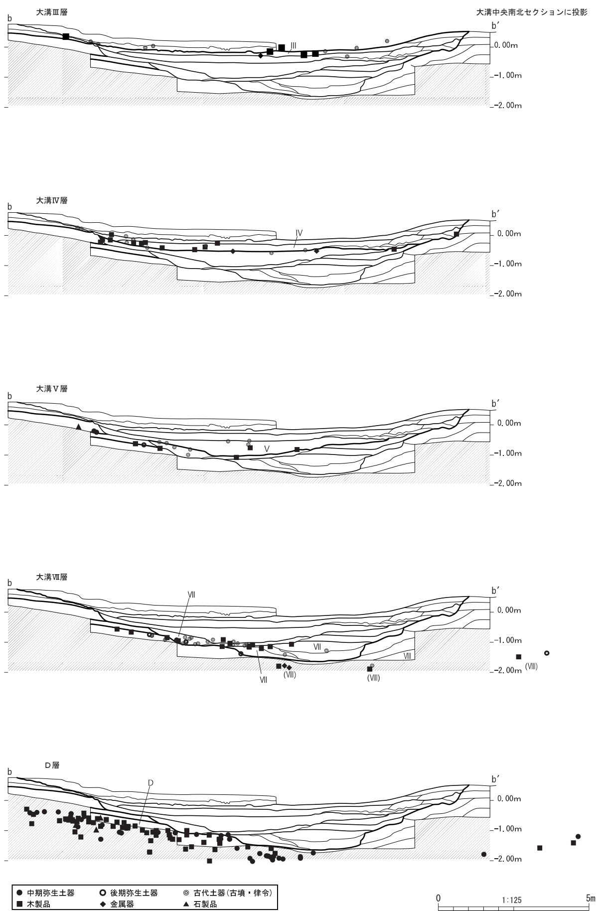
図 17 大溝・D層出土遺物の層位別垂直分布図
