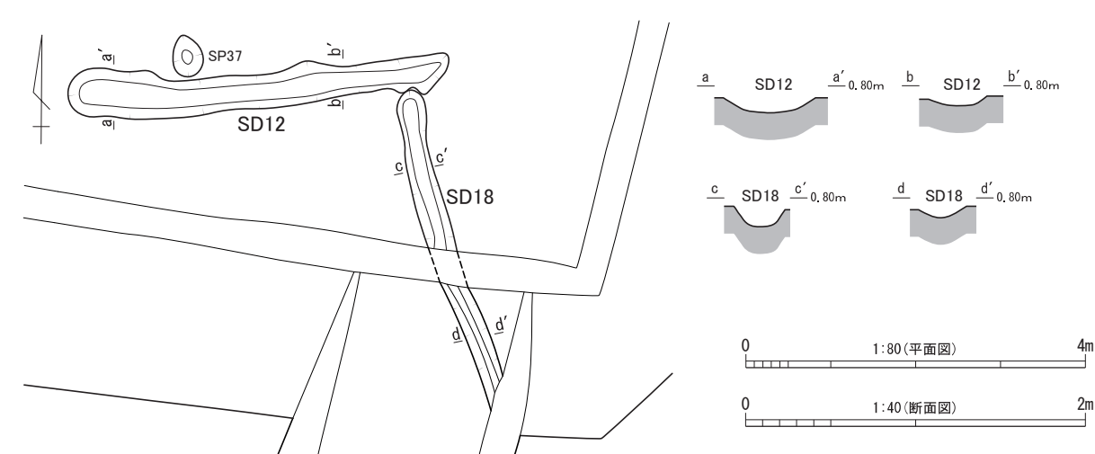
図 21 南微高地古代遺構図（溝）
