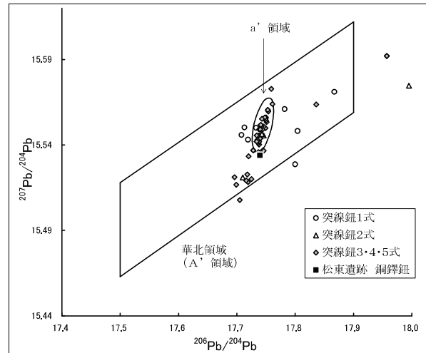
Fig.120 松東遺跡出土銅鐸と突線鈕式銅鐸の鉛同位体比分布 (B式図)
