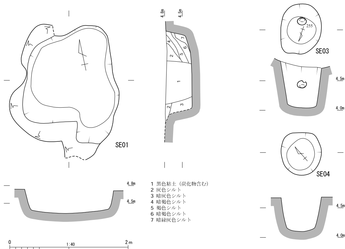
Fig.106 SE01・SE03・SE04 実測図
