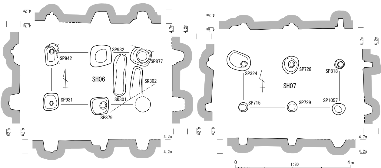
Fig.81 SH06・SH07 実測図
