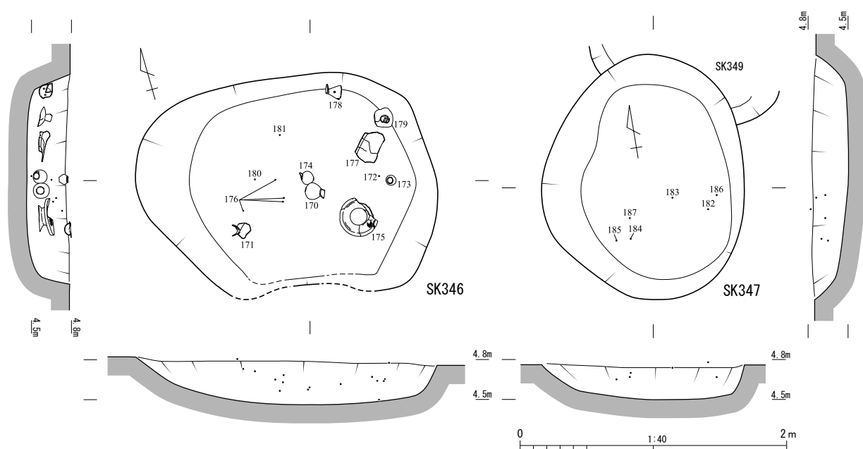
Fig.36 SK346・SK347 実測図
