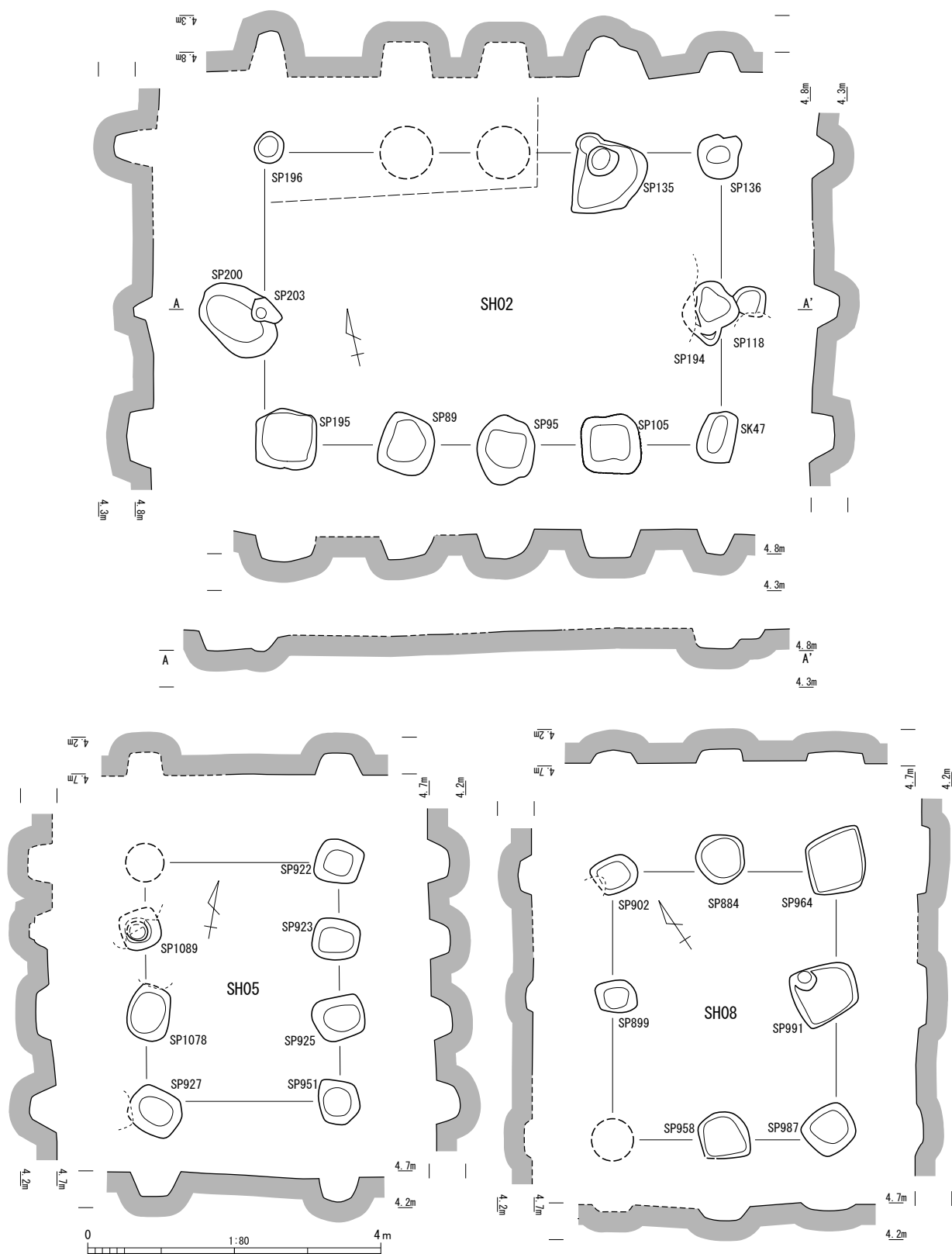
Fig.77 SH02・SH05・SH08 実測図
