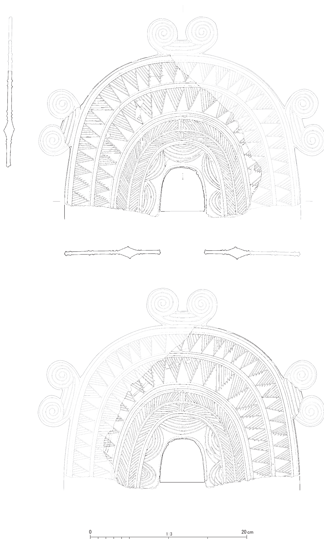
Fig.29 SK06 出土銅鐸復元図
