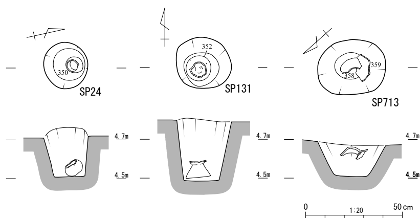
Fig.67 SP24・SP131・SP713 実測図
