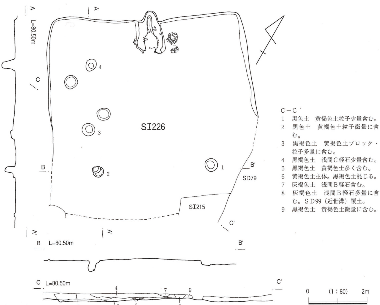
第154図 9区西226号住居
