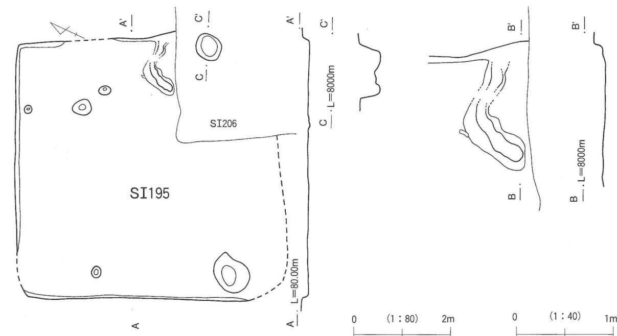
第175図 9区東195号住居・カマド
