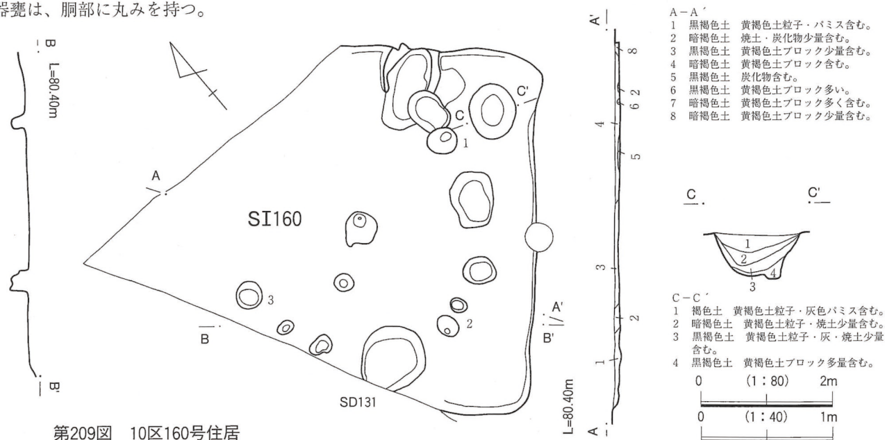
第209図 10区160号住居
