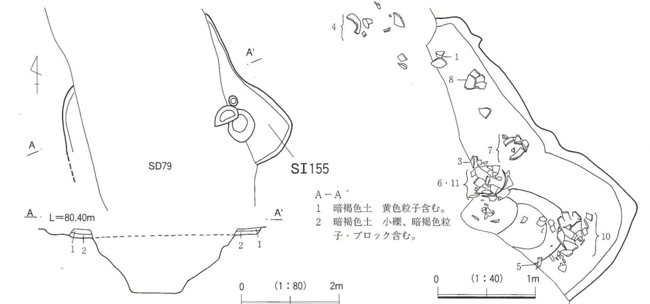
第238図 11区155号住居
