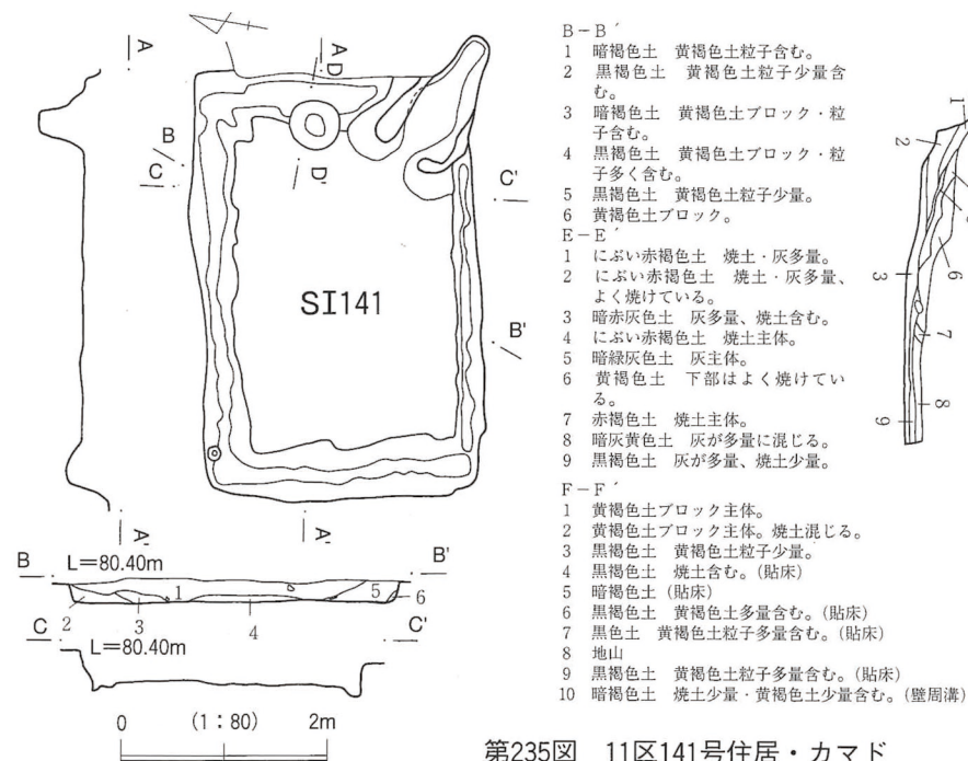
第235図 11区141号住居・カマド
