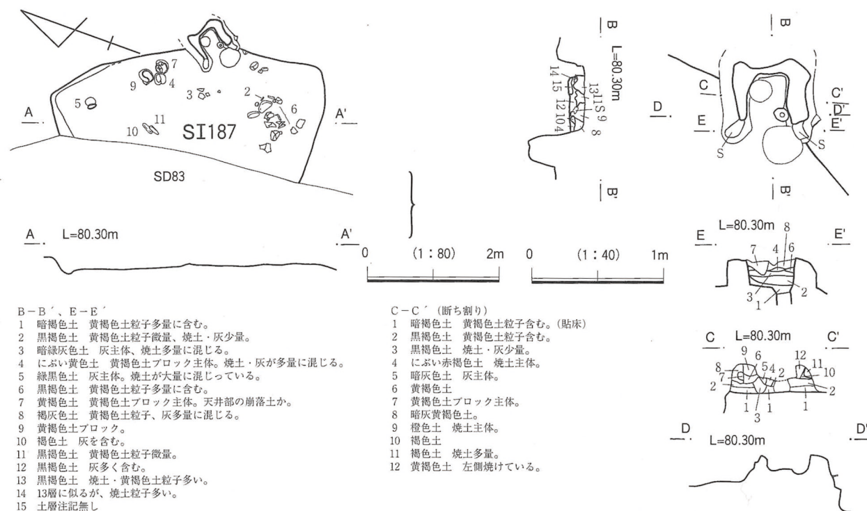
第167図 9区東187号住居遺物出土状況・カマド
