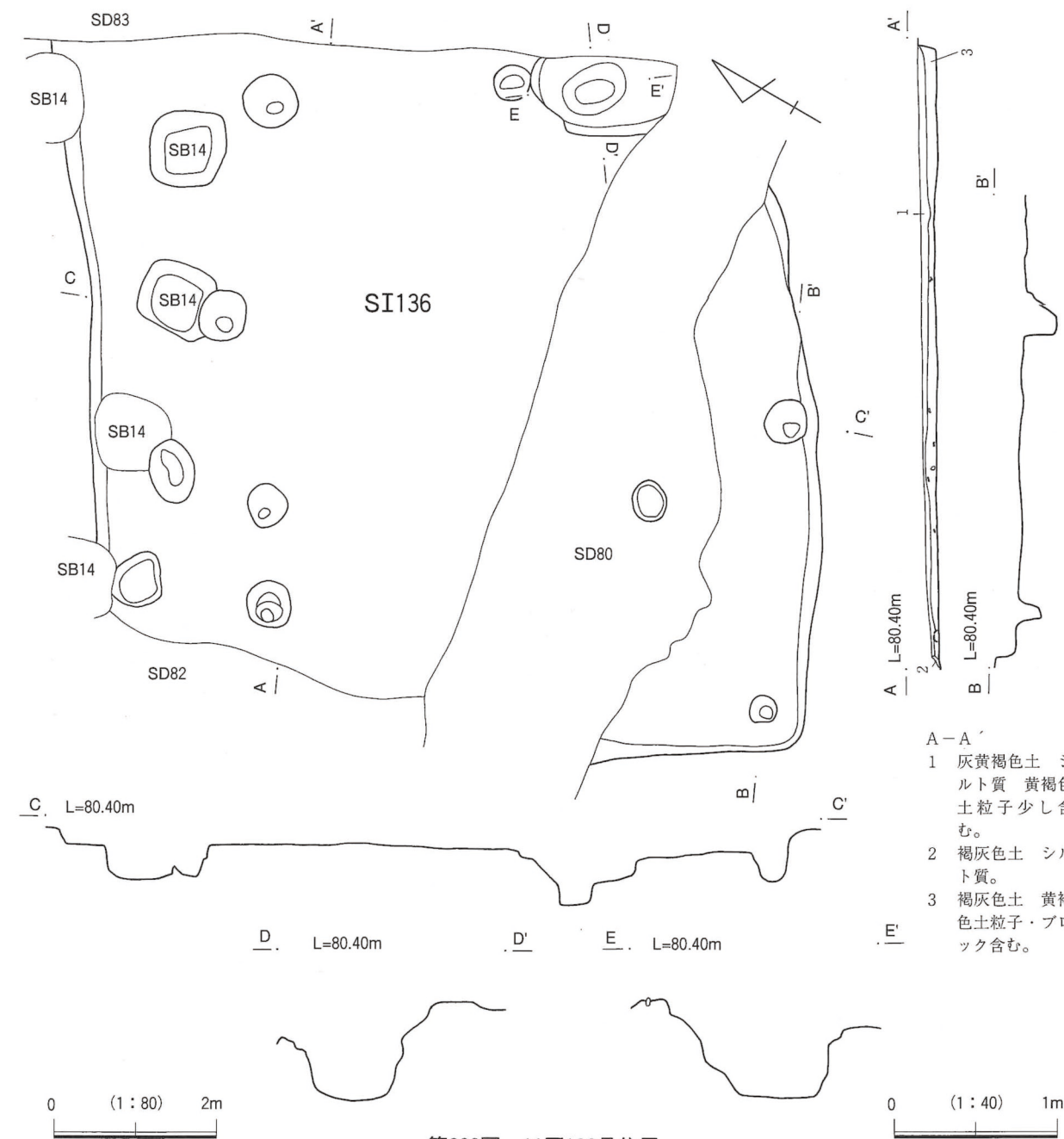
第223図 11区136号住居
