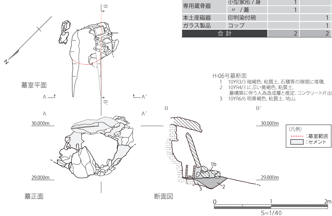
図 4.11 H-06 号墓 (平面図・断面図)
