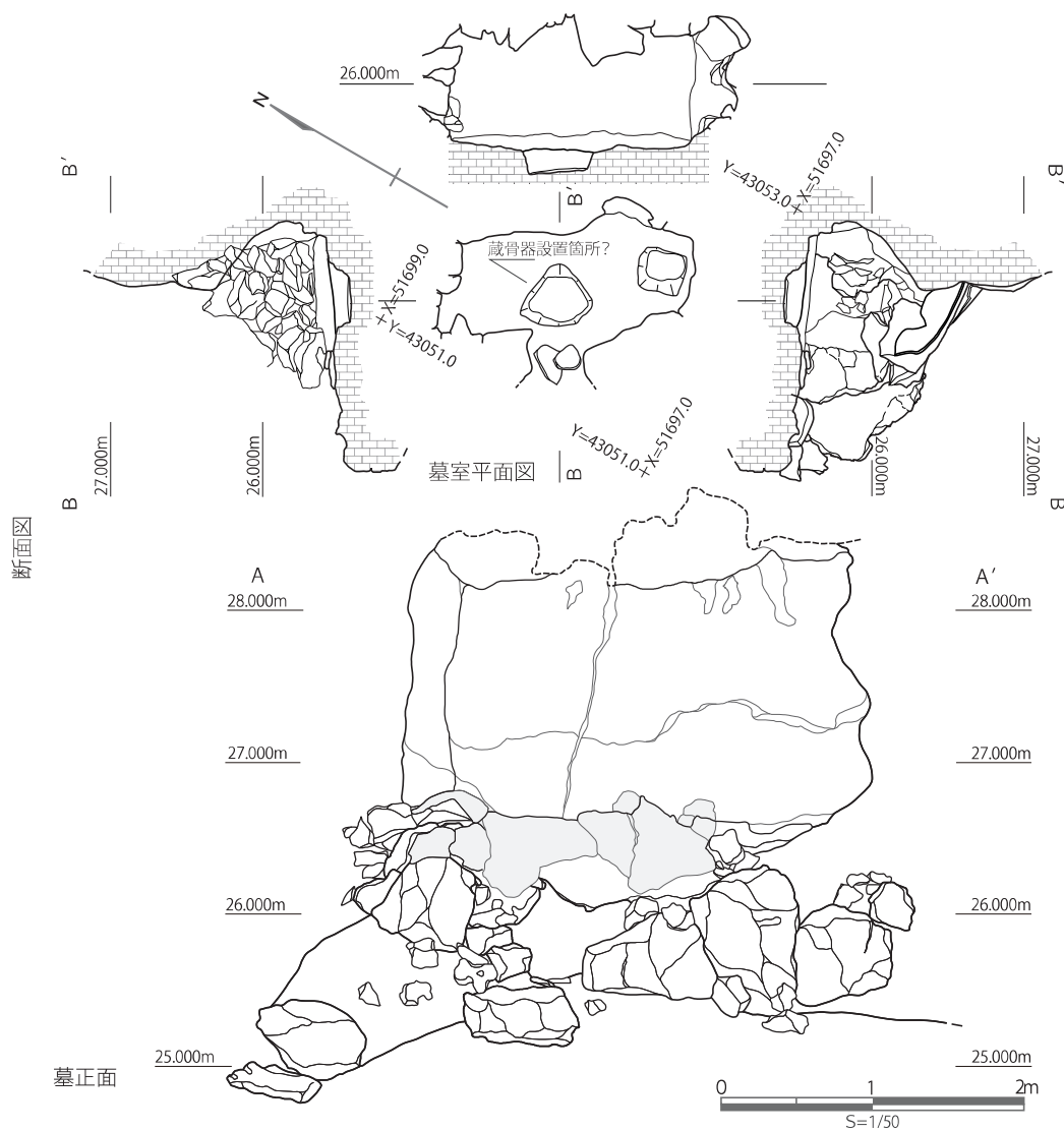
図 4.2 H-01 号墓 (平面図・断面図)
