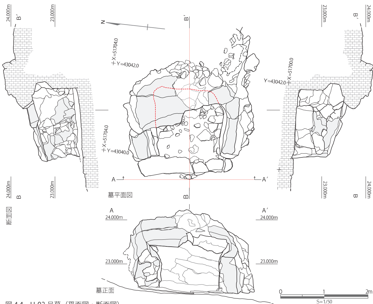
図 4.4 H-02 号墓（平面図・断面図）
