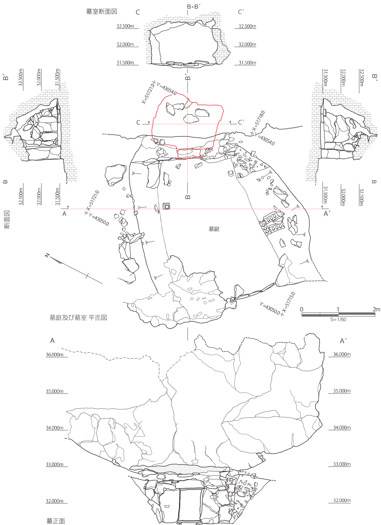
図 4.6 H-03 号墓 (平面図・断面図)
