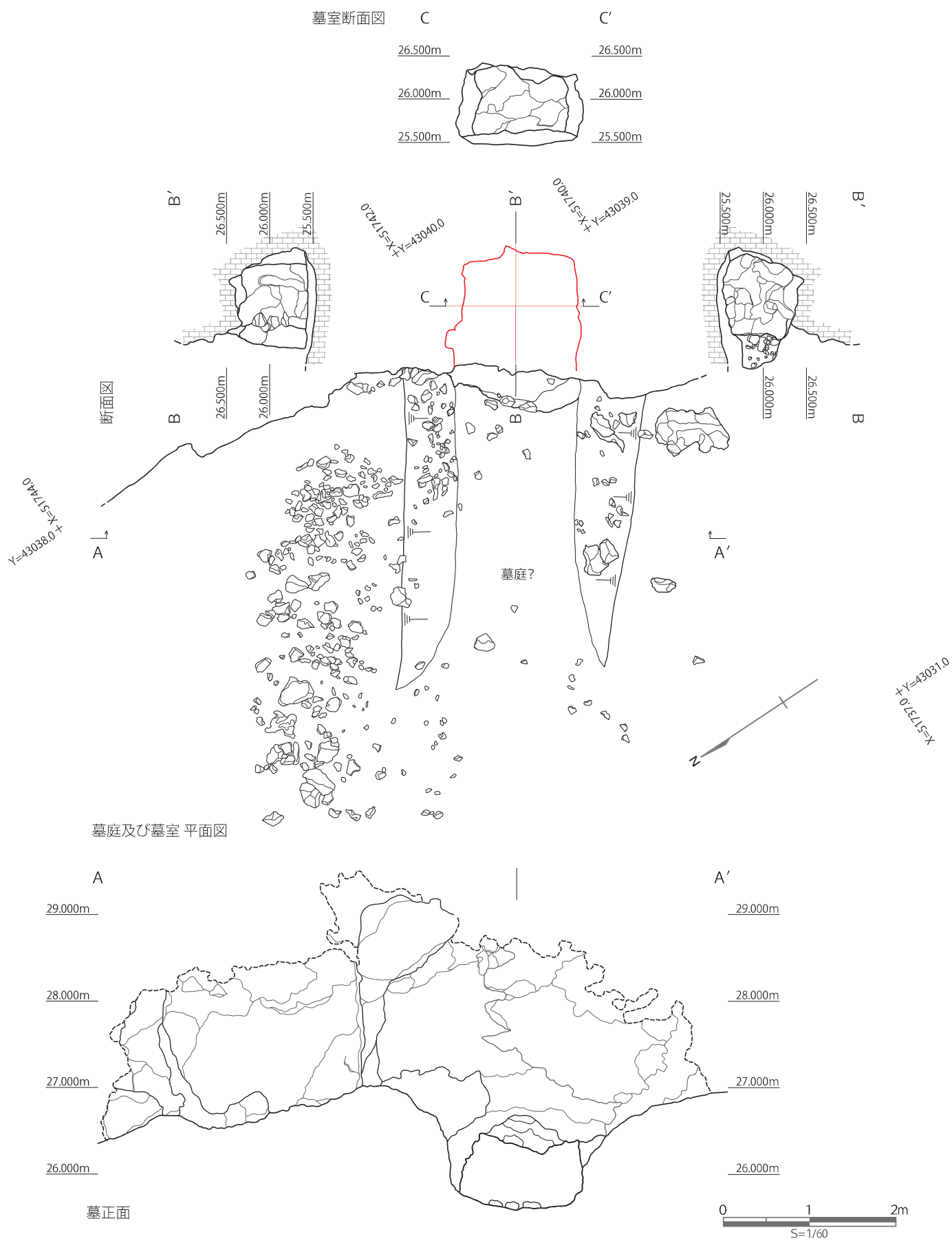
図 4.7 H-04 号墓 (平面図・断面図)
