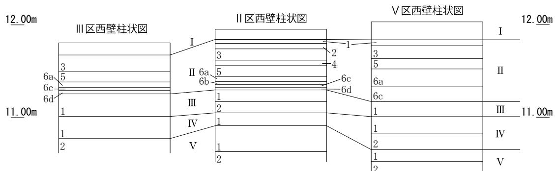
Fig. 9 基本層序柱状図 (S=1/40)
