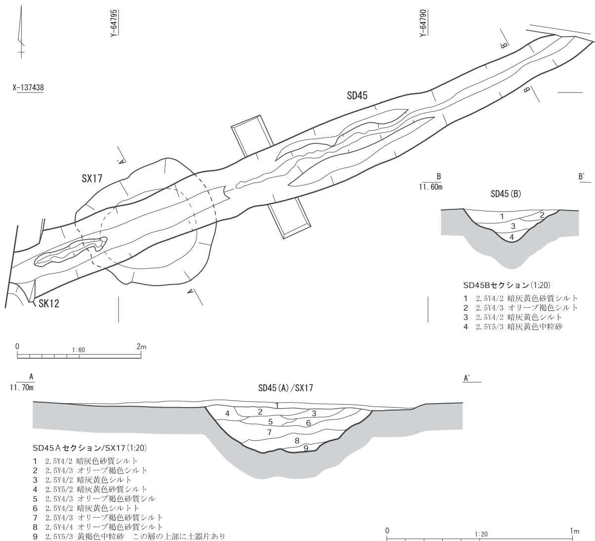
Fig. 35 SD45 平面 (S=1/60)・断面図 (S=1/20)
