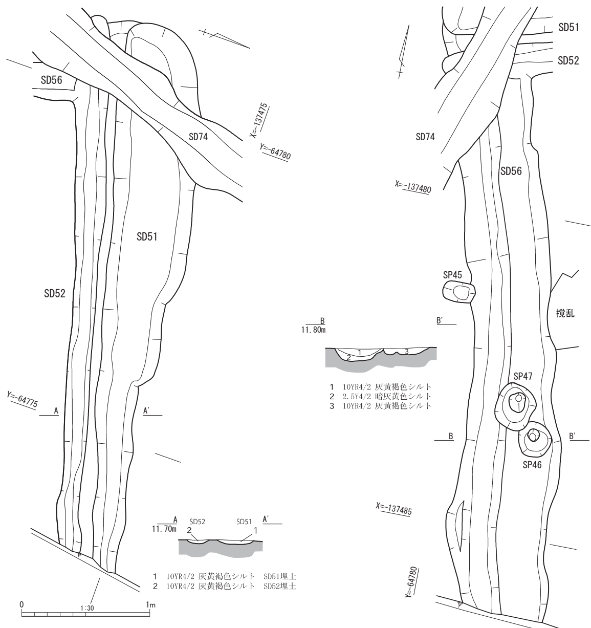
Fig. 37 SD51・52・56 平面・断面図 (S=1/30)
