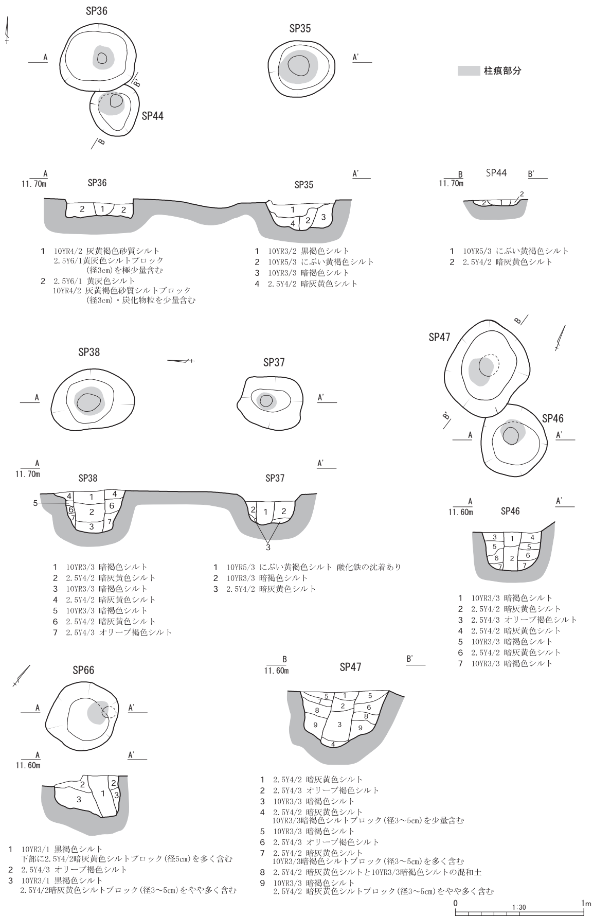
Fig. 33 小穴群各遺構平面・断面図 (S=1/30)
