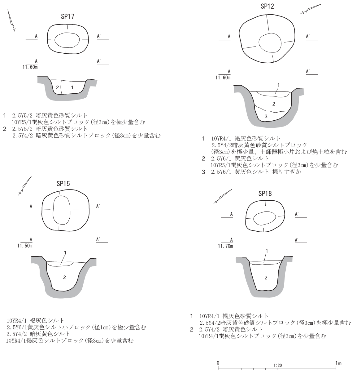
Fig. 24 SP17・12・15・18 平面・断面図 (S=1/20)
