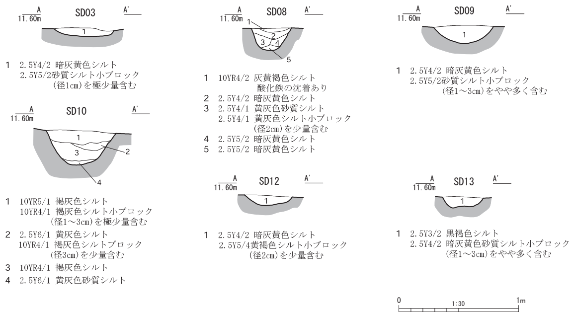
Fig. 27 SD03・08・09・10・12・13 断面図 (S=1/30)
