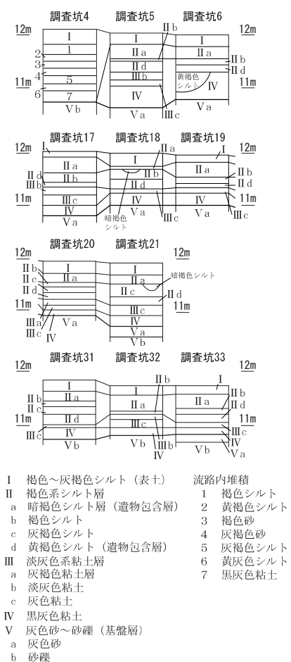
Fig. 8 土層柱状図 (S=1/100)
