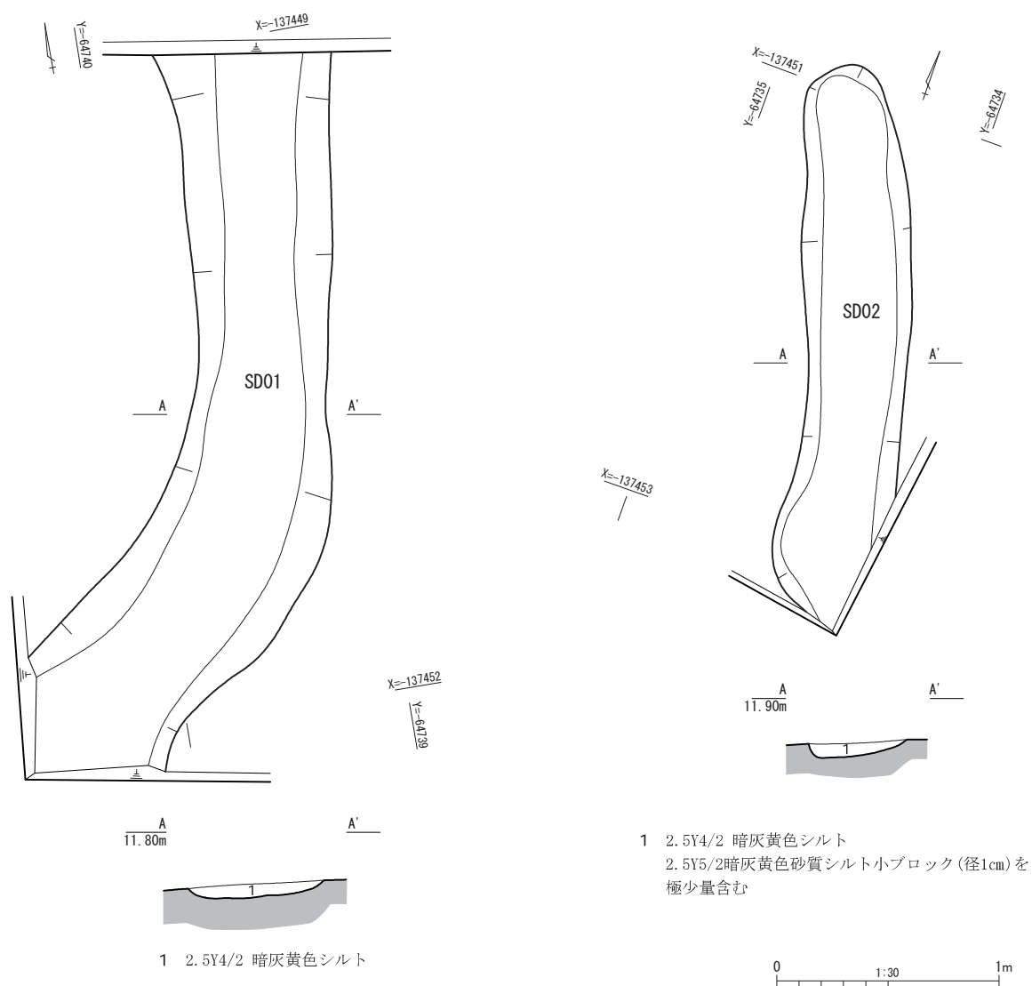
Fig.19 SD01・SD02 平面図 (S=1/30)
