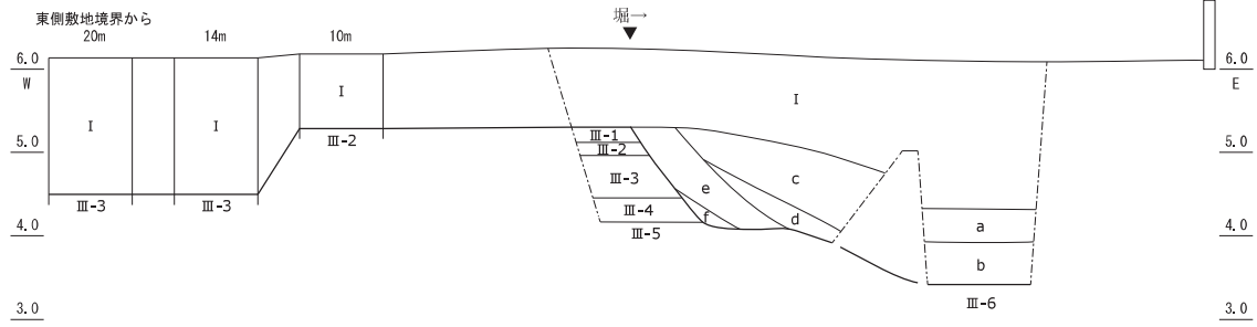
調査溝 2 土層断面図
