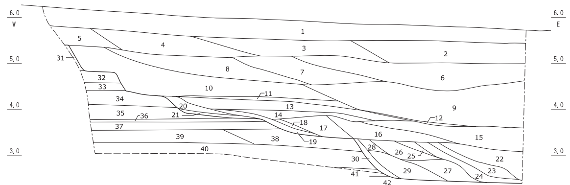
調査区2 南壁土層断面図（反転）
