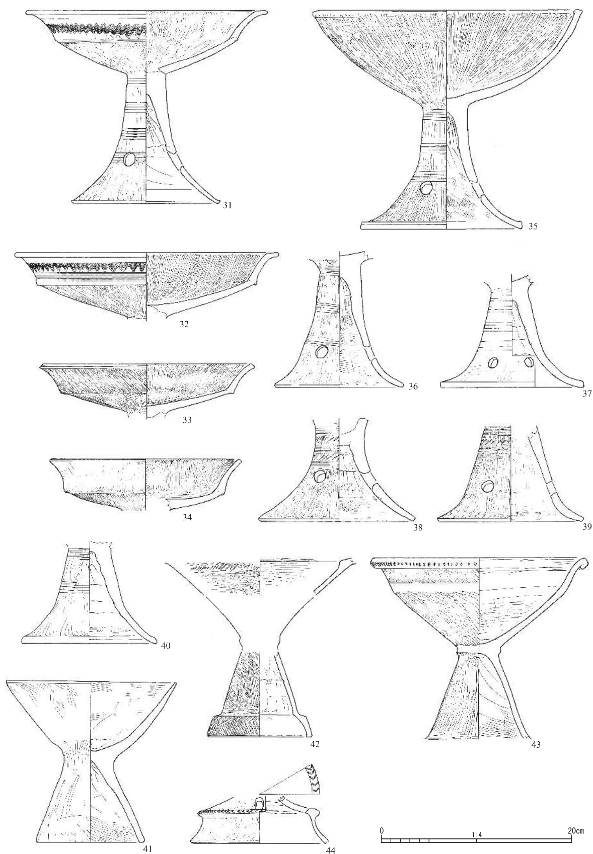
Fig.9 SD01 出土遺物 (3)
