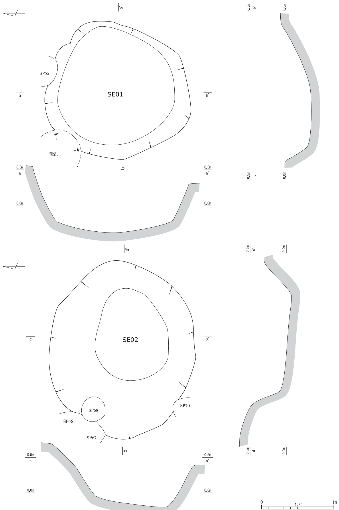
Fig.13 SE01・02 実測図
