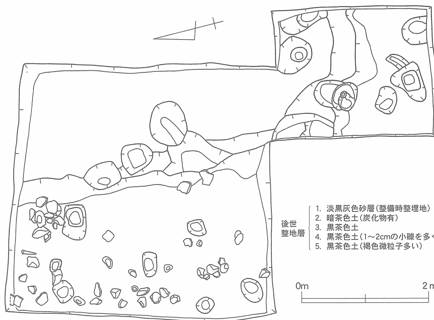
第12図 5トレンチ平面実測図〔1/60〕
