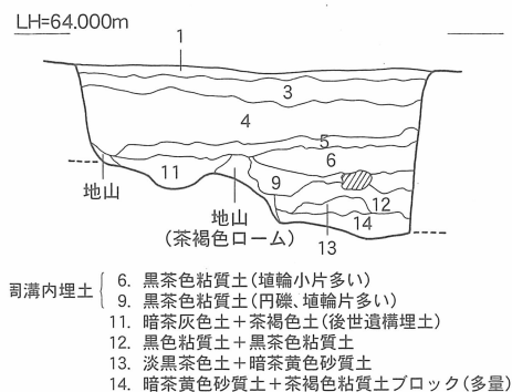
第13図 5トレンチ東壁土層 実測図〔1/60〕
