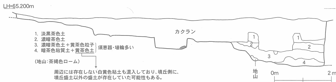
第10図 4トレンチ東壁土層実測図〔1／80〕
