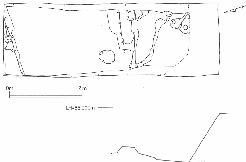
第9図 3トレンチ平面実測図〔1/60〕
