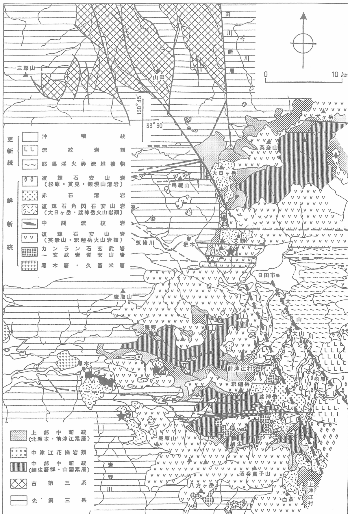
第2図 福岡・大分・熊本県付近の地質図 鶴見山古墳石室の石材産地を■で、それに類似する岩体を★印で示した。 番号は本文と一致する。
