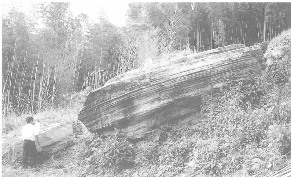
写真1 流理構造が発達しきれいな平面で割れる角閃石安山岩溶岩 斜面を矢部川に向かって崩落しつつある。黒木町女郎岳。
