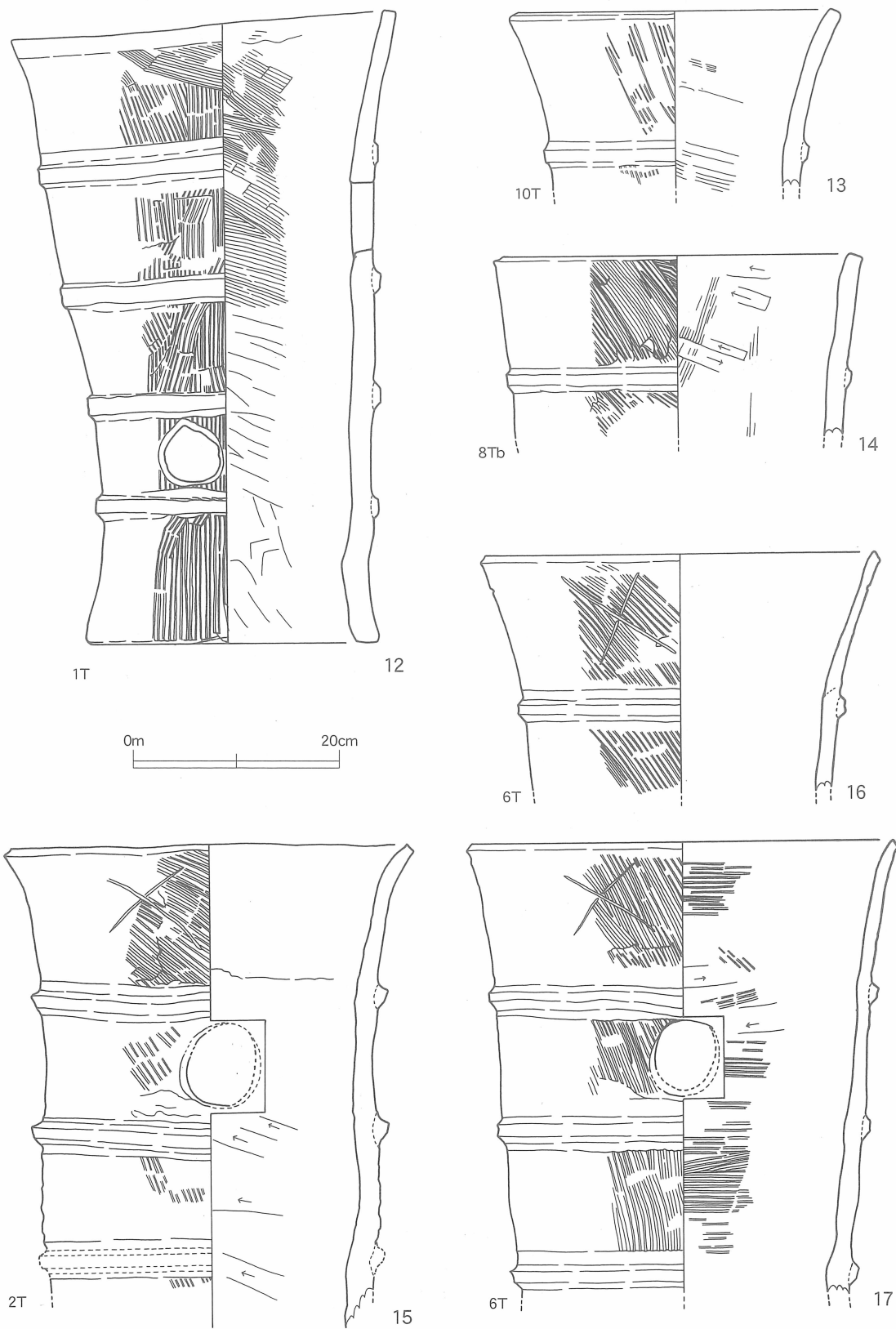
第28図 出土遺物実測図〔1／6〕
