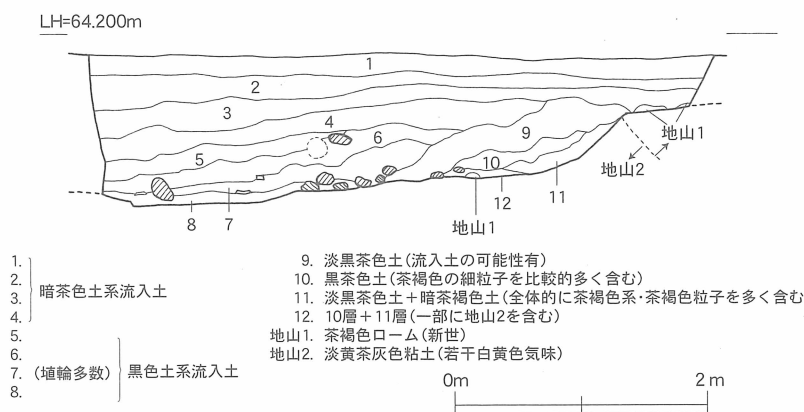
第25図 10トレンチ北壁土層実測図〔1/60〕
