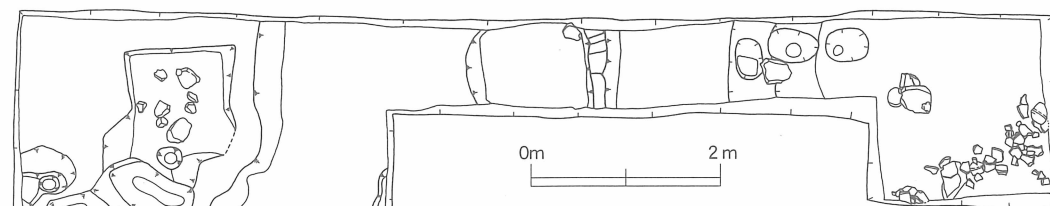
第11図 4トレンチ平面実測図〔1／80〕
