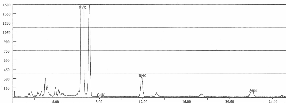
NO.19 帶金具 銀頭 蛍光X線分析結果-①
