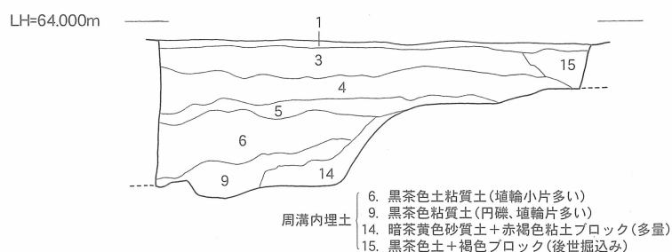
第15図 5トレンチ北壁土層実測図〔1/60〕
