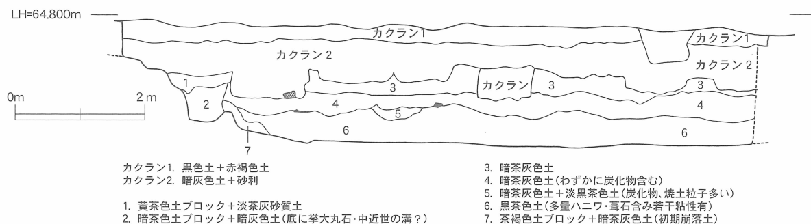
第17図 6トレンチ東壁土層実測図〔1/80〕
