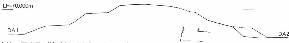
第37図 鶴見山古墳 石室及び墳丘断面図〔1/400〕
