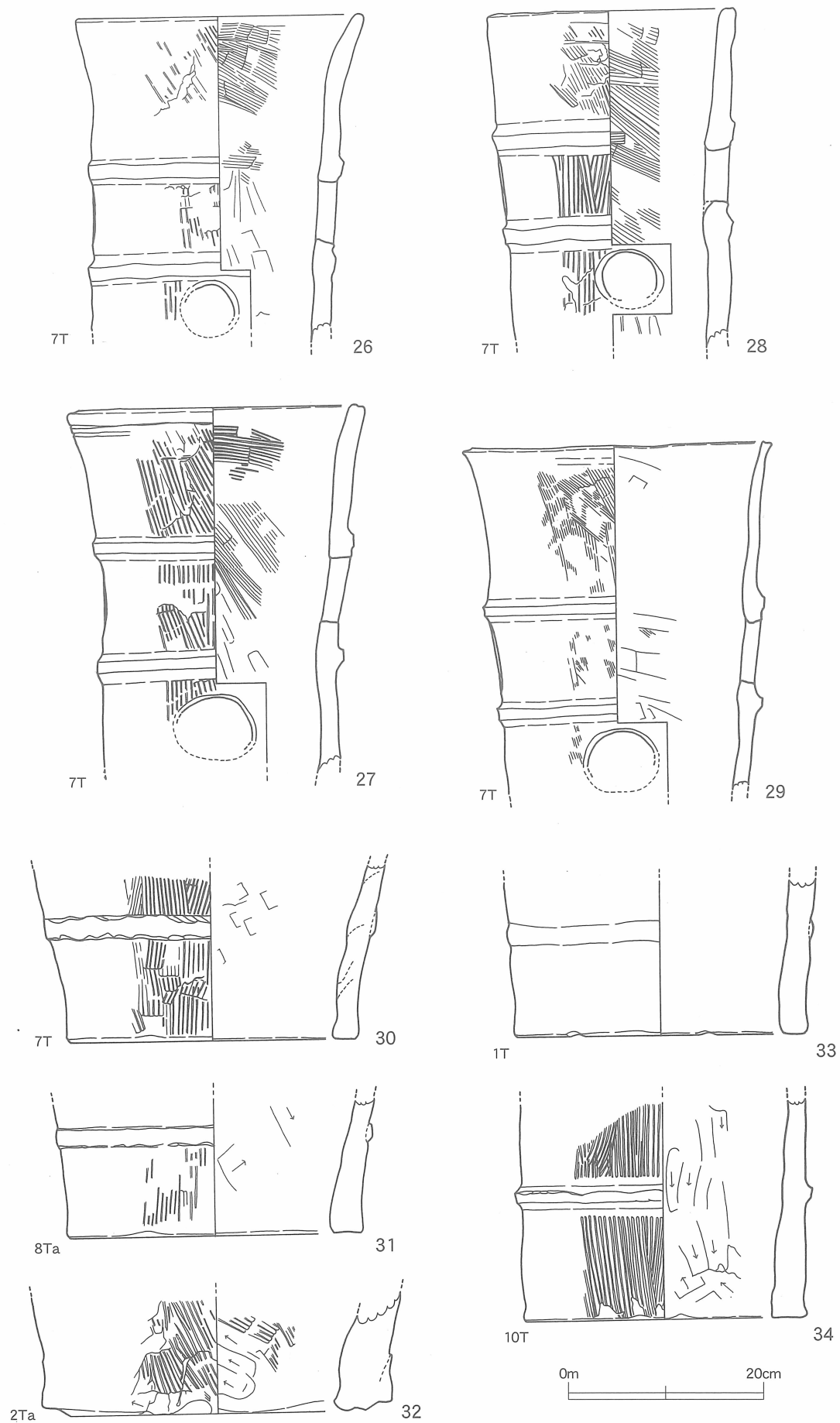
第30図 出土遺物実測図〔1／6〕
