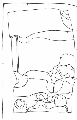
第6図 2トレンチ a 北壁土層実測図〔1/60〕
