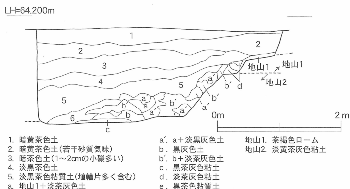
第23図 9トレンチ北壁土層実測図〔1/60〕
