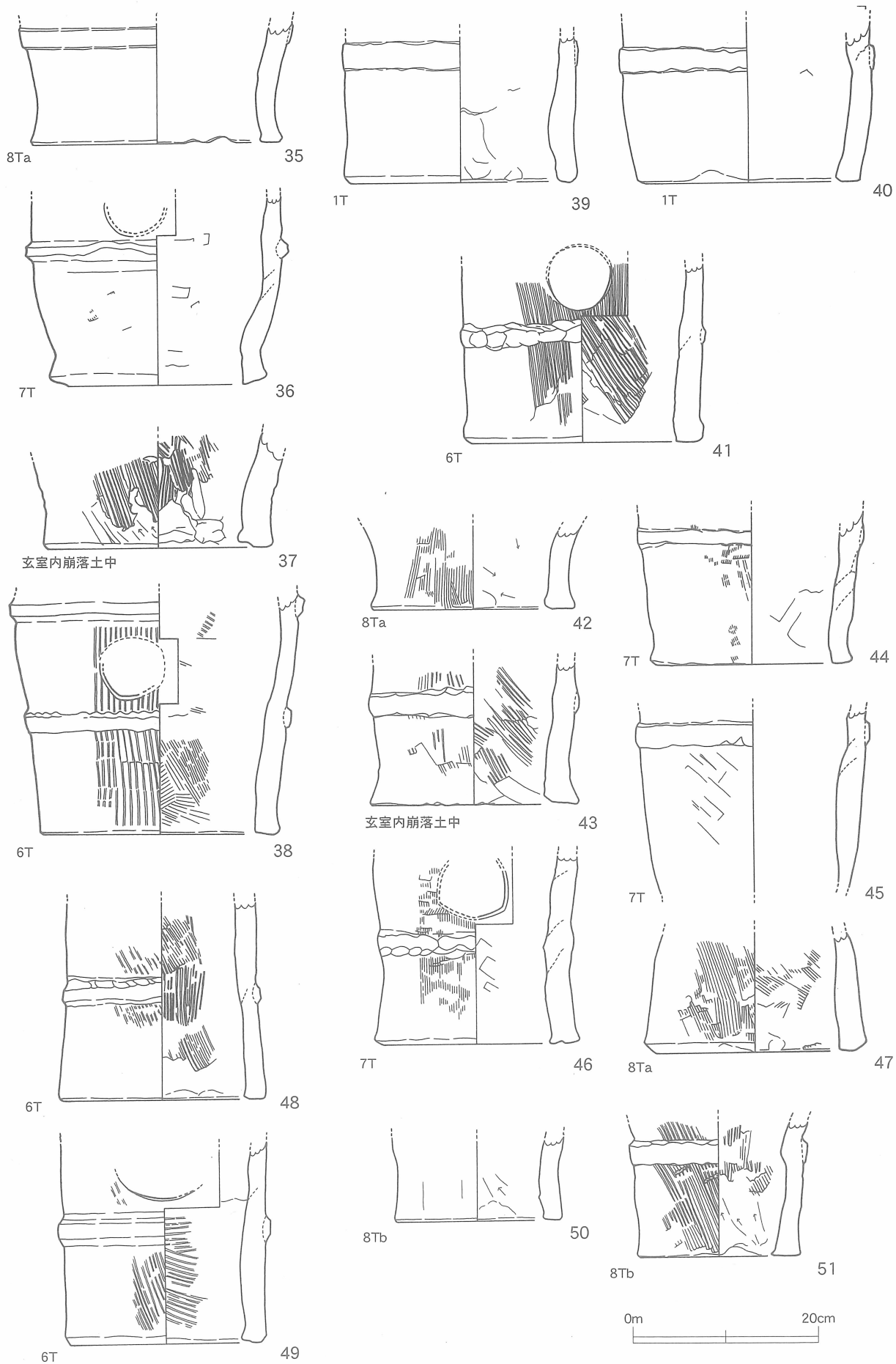
第31図 出土遺物実測図〔1／6〕
