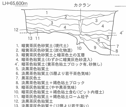
第8図 2トレンチ b 南壁土層実測図〔1/60〕
