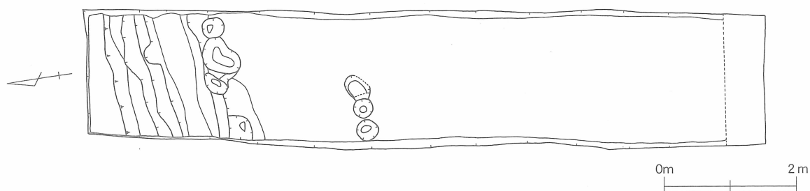
第16図 6トレンチ 平面実測図〔1/80〕
