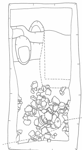
第22図 9トレンチ 平面実測図〔1/60〕
