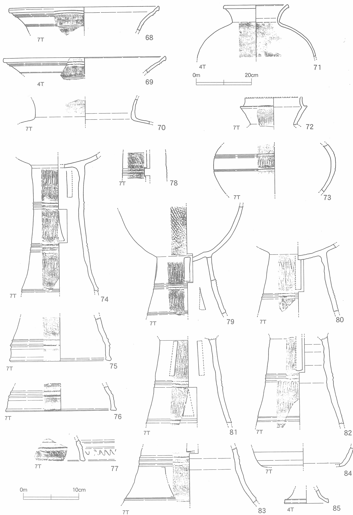
第33図 出土遺物実測図〔1/4・1/8(68~71)〕
