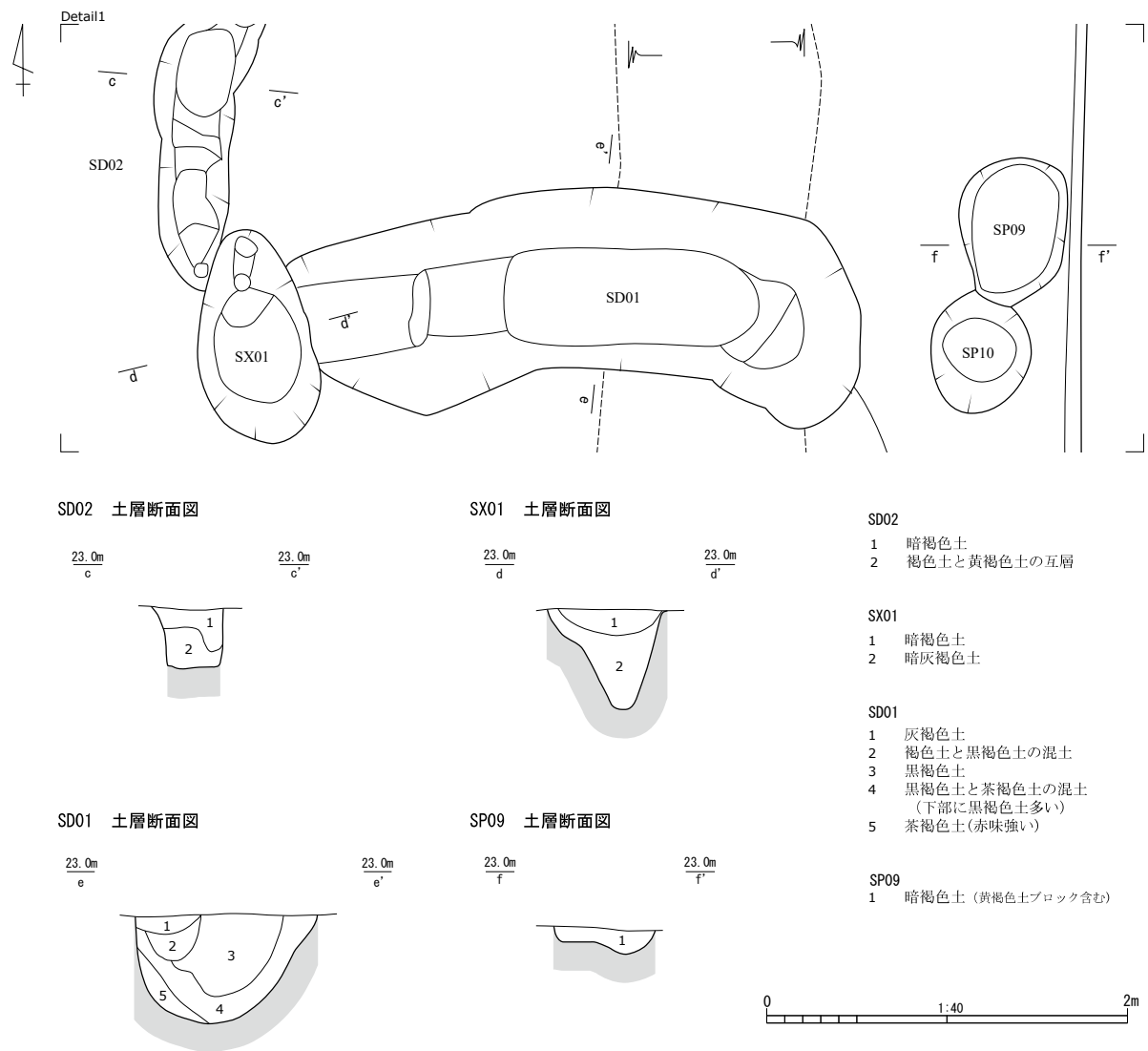
第8図 遺構実測図(1)
