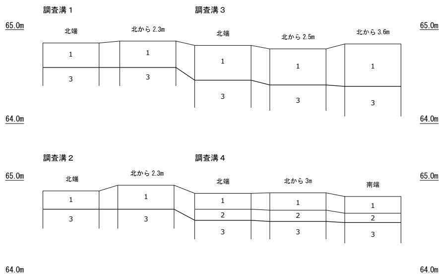
土層柱状図 (S=1/40)
