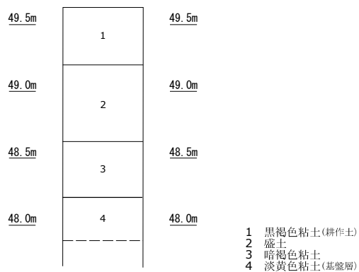
土層柱状図 (S=1/40)
