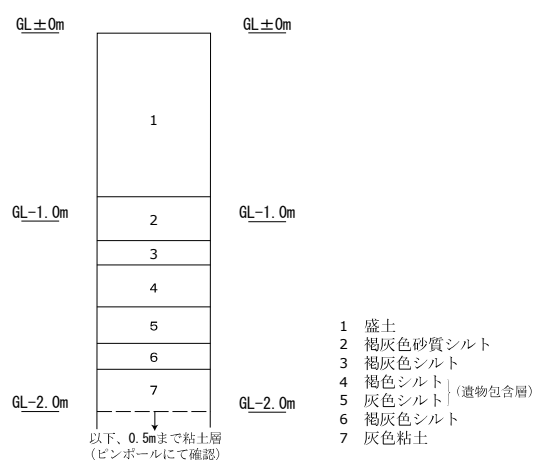
土層柱状図 (S=1/40)
