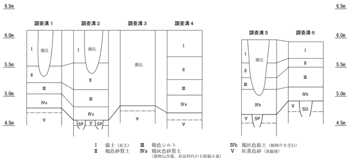
第2図 14次調査土層柱状図
