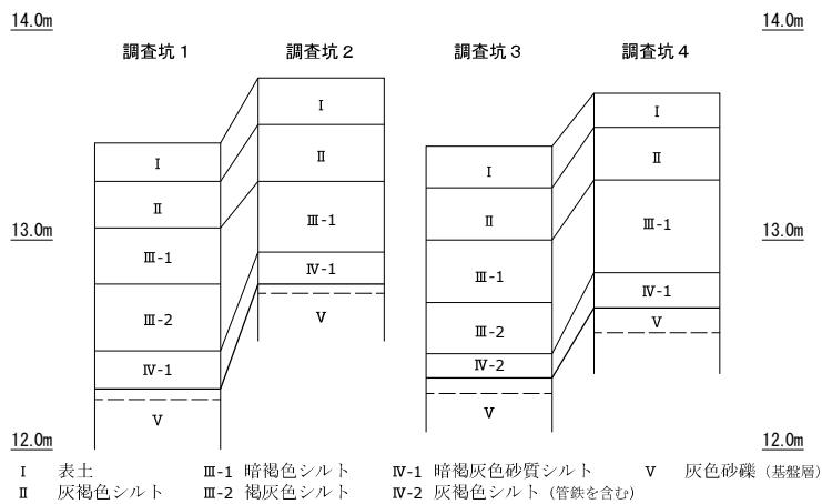
土層柱状図 (S=1/40)
