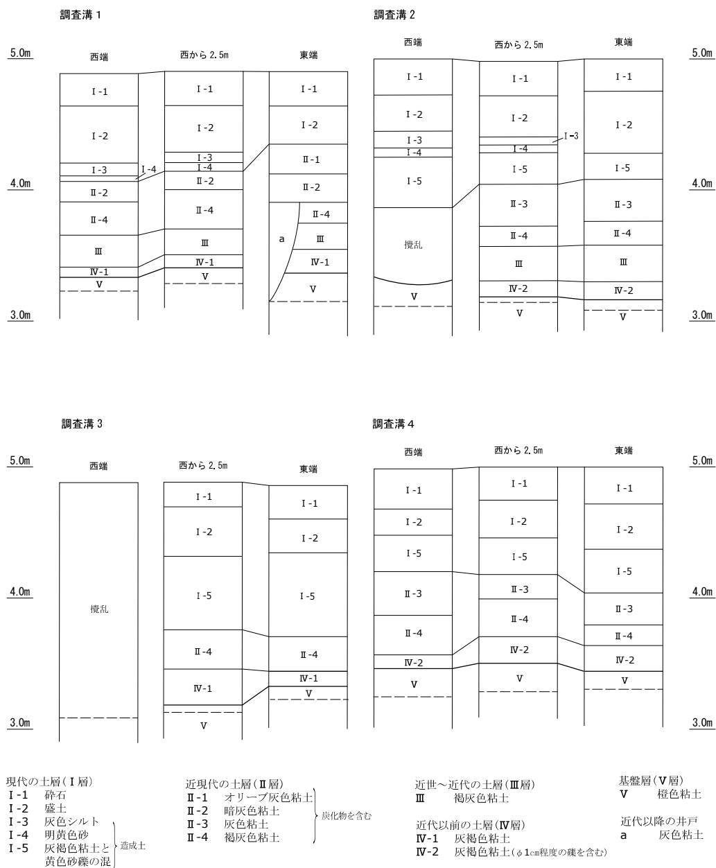
土層柱状図 (S=1/40)
