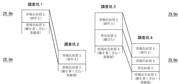
土層柱状図 (S=1/40)
