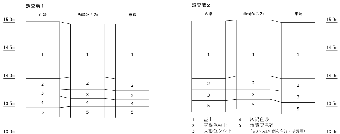
土層柱状図 (S=1/40)
