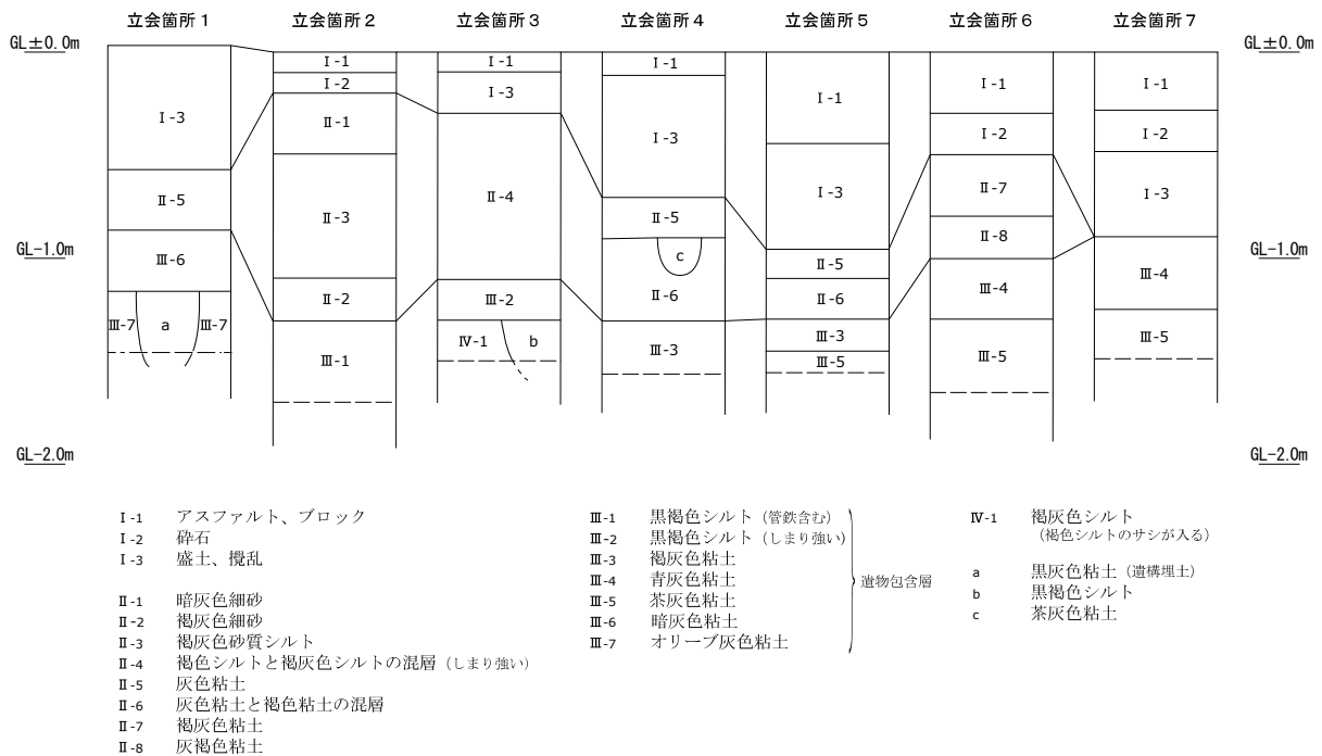
土層柱状図 (S=1/40)
