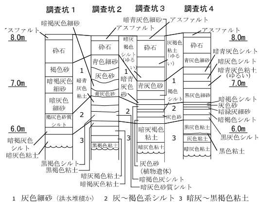
土層柱状図 (S=1/80)
