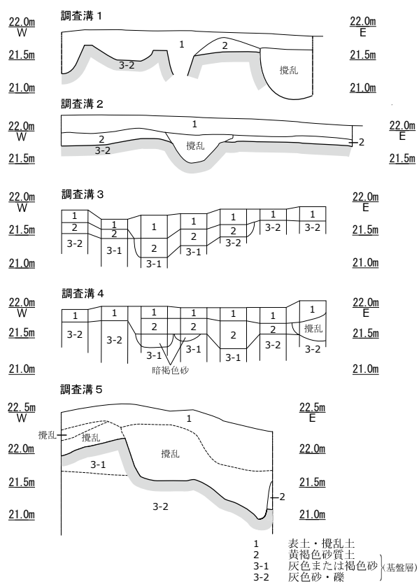
土層柱状図 (S=1/80)
