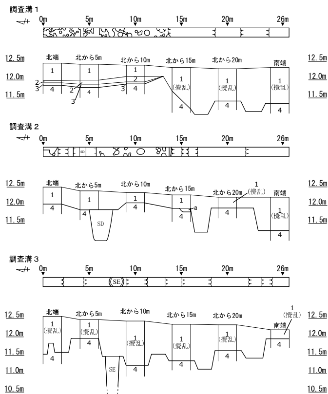
土層柱状図 (S=1/100) 及び平面図 (S=1/400)
