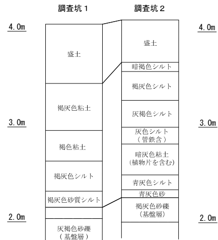
土層柱状図 (S=1/40)
