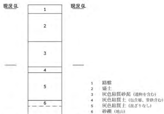
土層柱状図 (S= 1/40)
