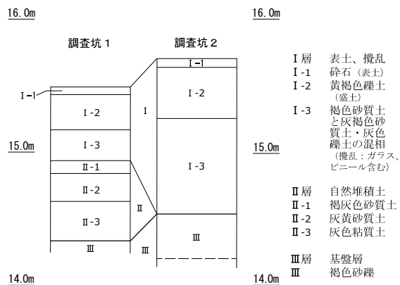
土層柱状図 (S=1/40)
