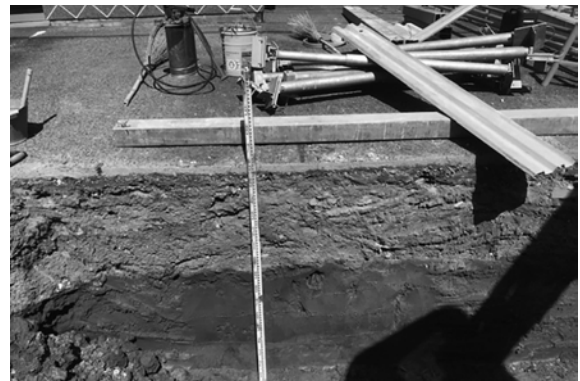
立会箇所 3 土層堆積状況
