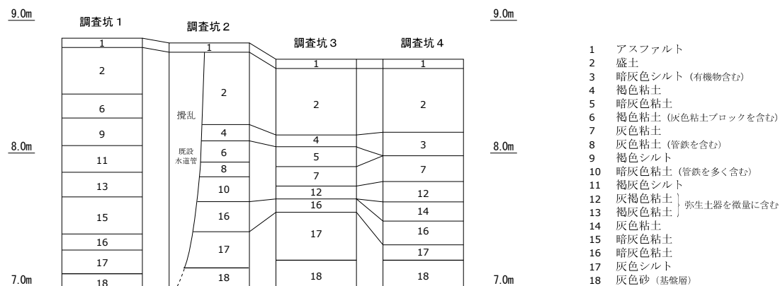
土層柱状図 (S=1/40)
