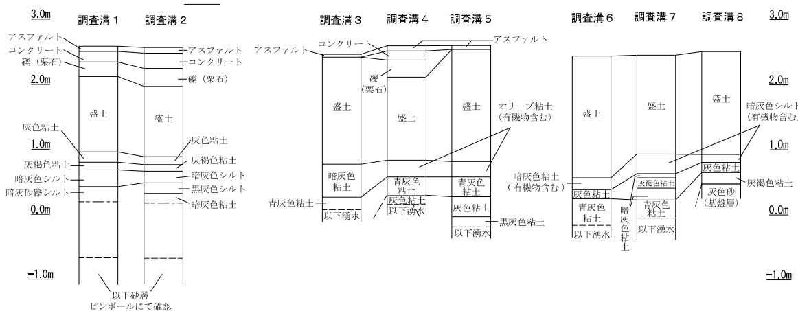
土層柱状図 (S=1/80)
