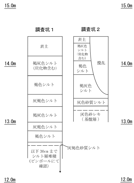
土層柱状図 (S=1/40)
