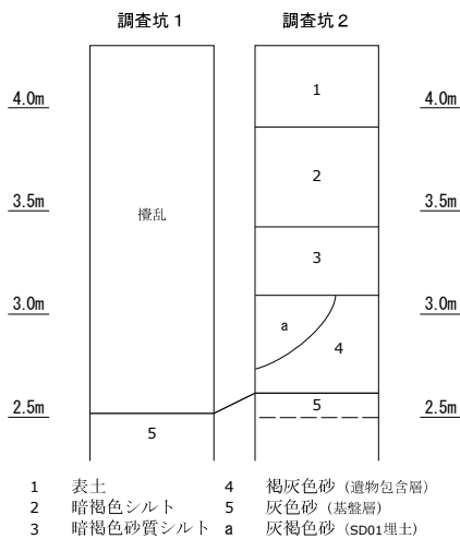
土層柱状図 (S=1/40)
