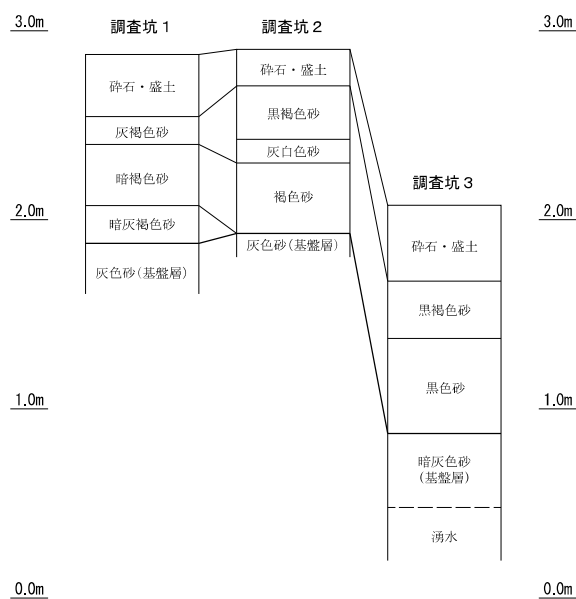
土層柱状図 (S=1/40)
