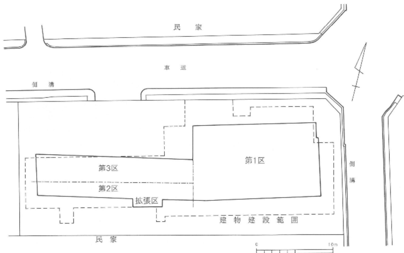
第169図 発掘調査区配置図 1 / 300
