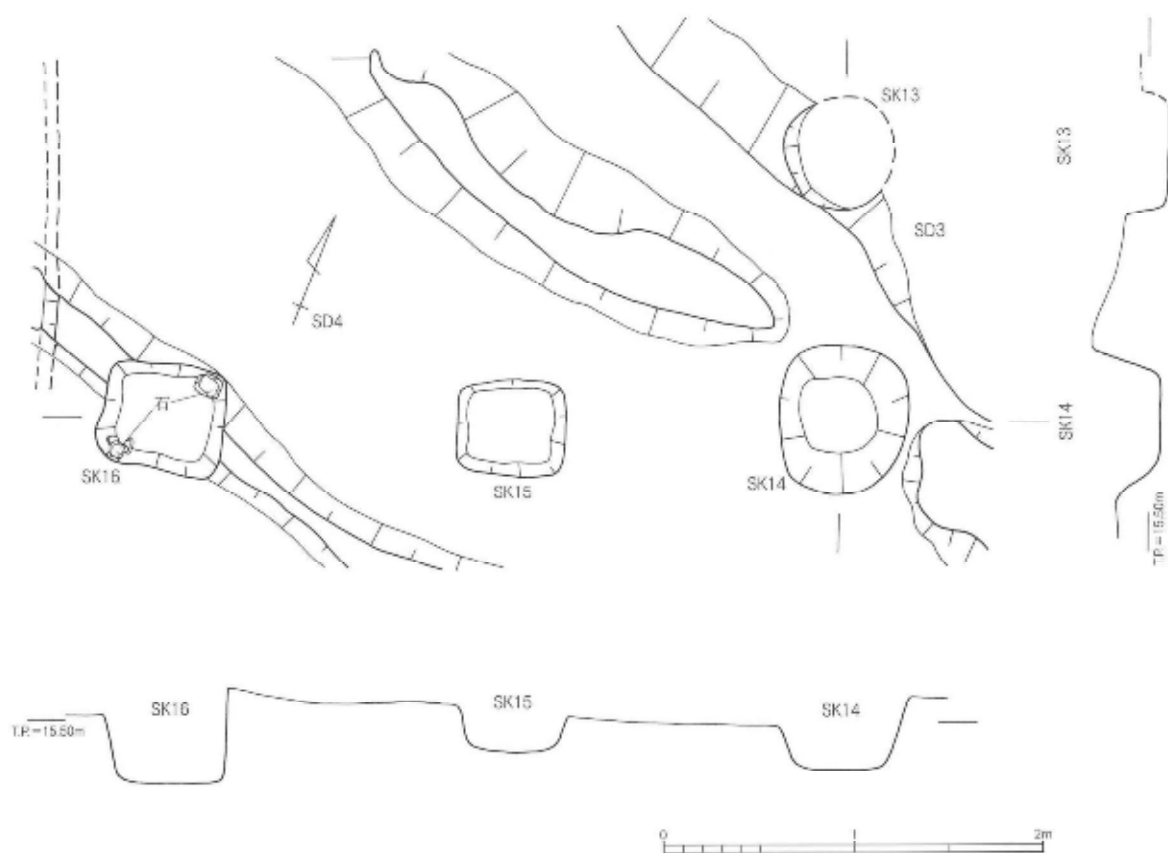
第 178 図 SD4・SK13 ~ 16 平面・断面実測図 1 / 40
