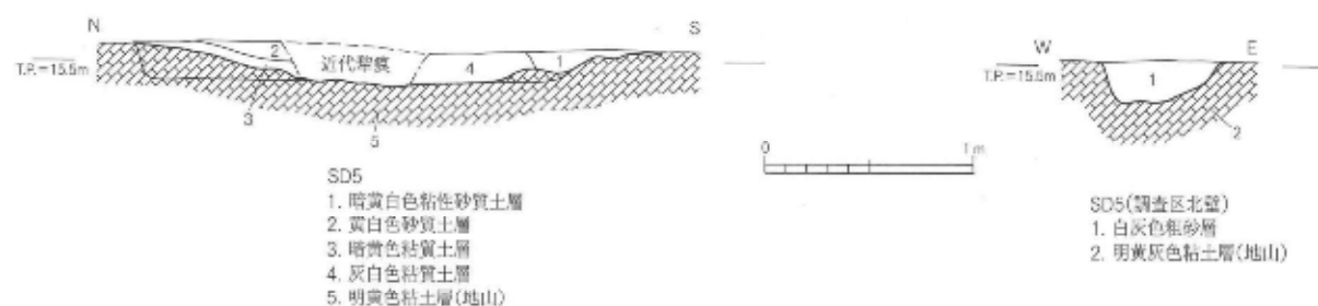
第 176 図 SD5 断面実測図 1 / 40
