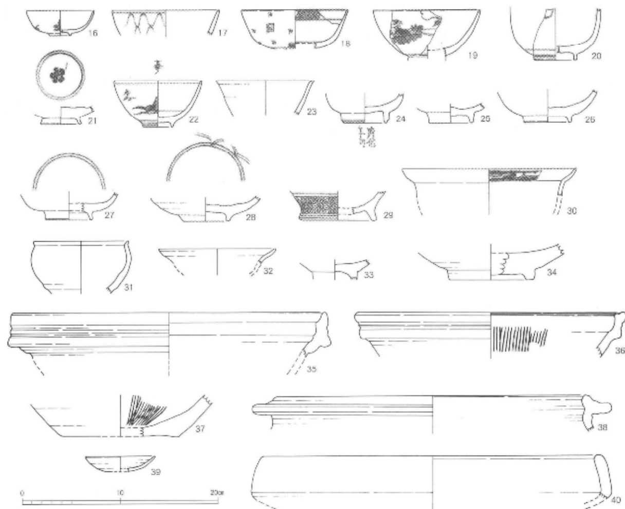
第183図 出土遺物実測図(2) 1/4
