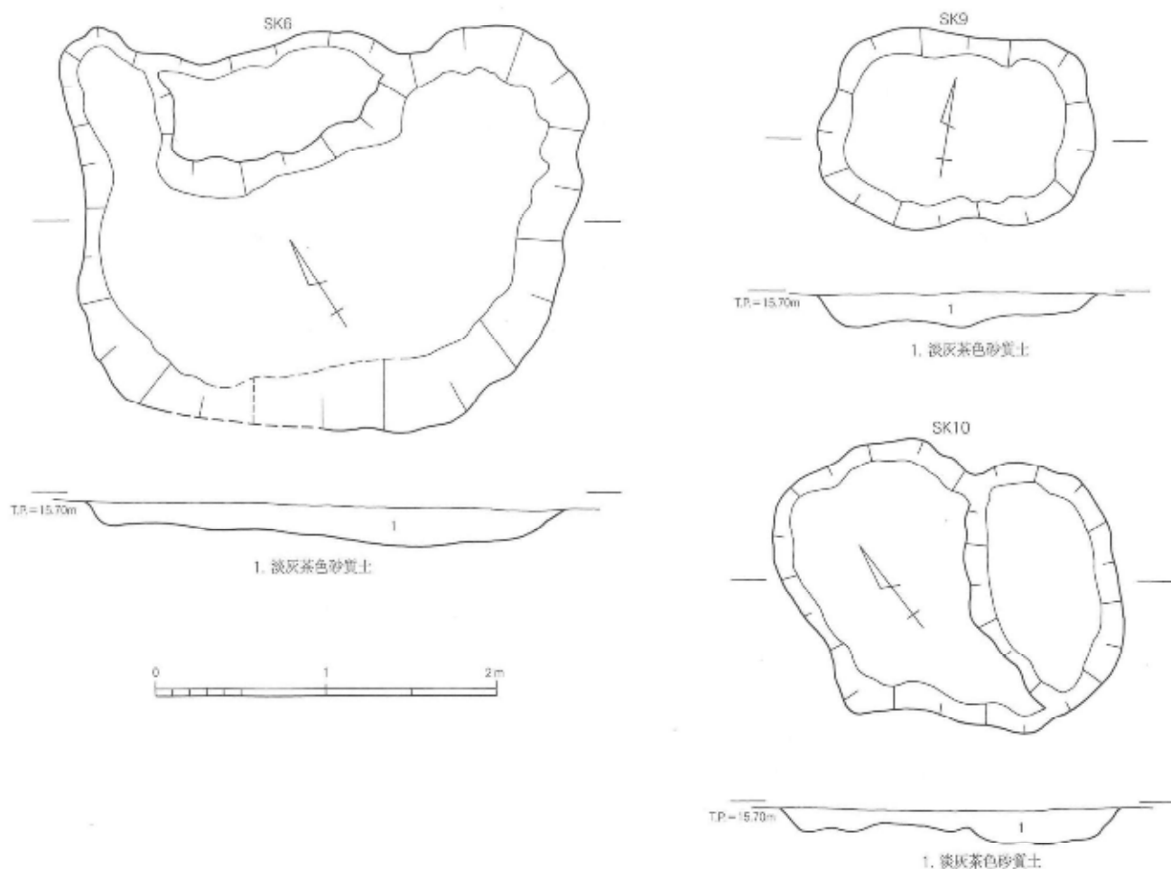
第 179 図 SK6・9・10 平面・断面実測図 1 / 40
