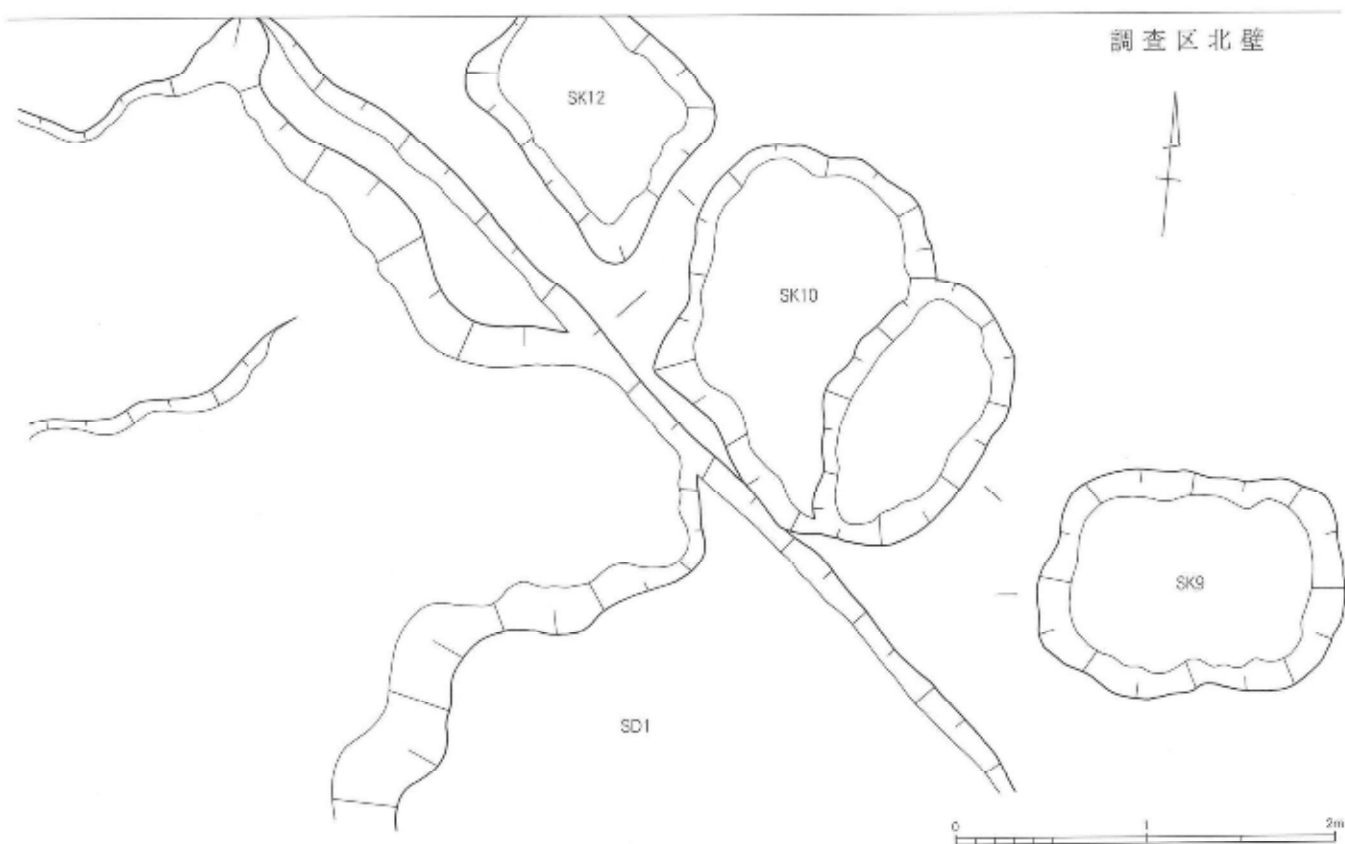
第174図 SD1・SK9・10・12平面実測図 1 / 40
