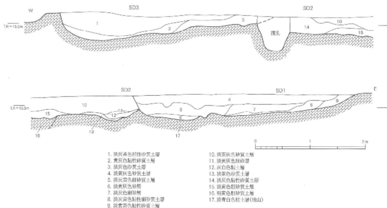
第 175 図 SD1 ～ 3 断面実測図 1 / 40
