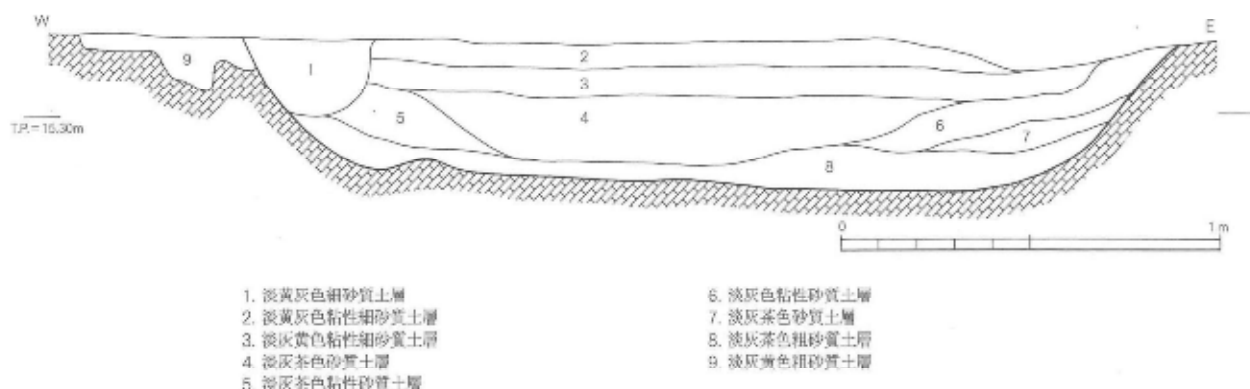
第 181 図 SK18 断面実測図 1 / 20
