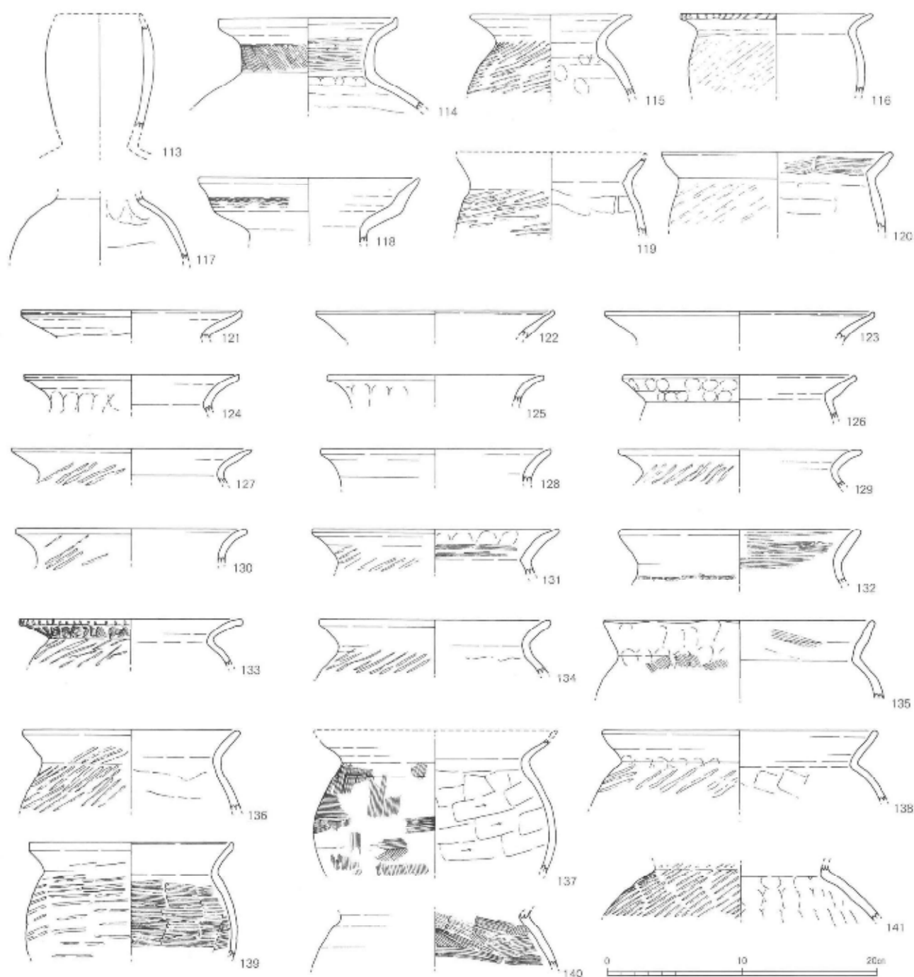
第 157 図 出土遺物実測図 (8) 1 / 4 3 号河道①
