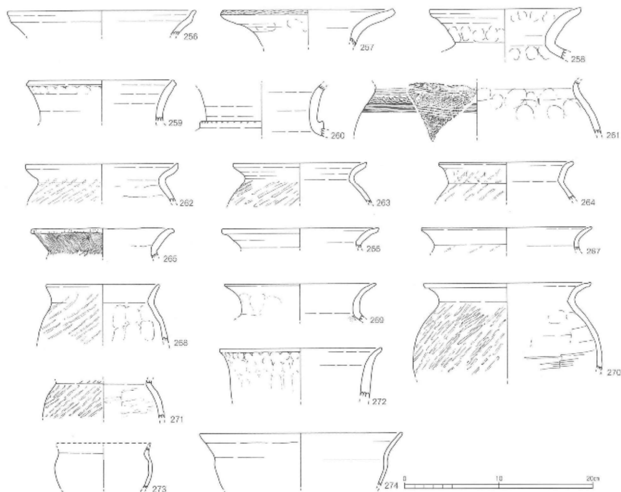
第 162 図 出土遺物実測図・拓影 (13) 1 / 4 3 号河道⑥ (塚状遺構)
