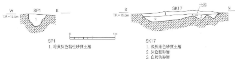
第 180 図 SP1・SK17 断面実測図 1 / 40
