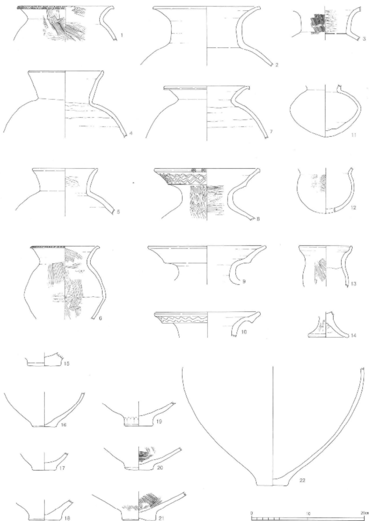
第150圖 出土遺物実測図(1) 1/4
