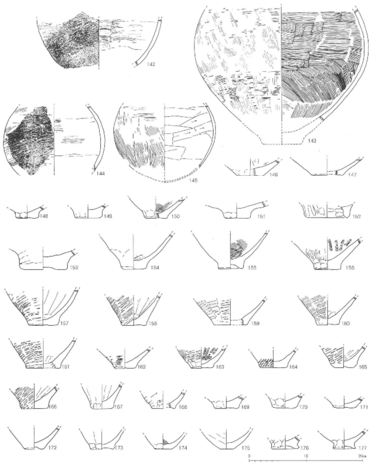
第158図 出土遺物実測図(9) 1/4 3号河道②
