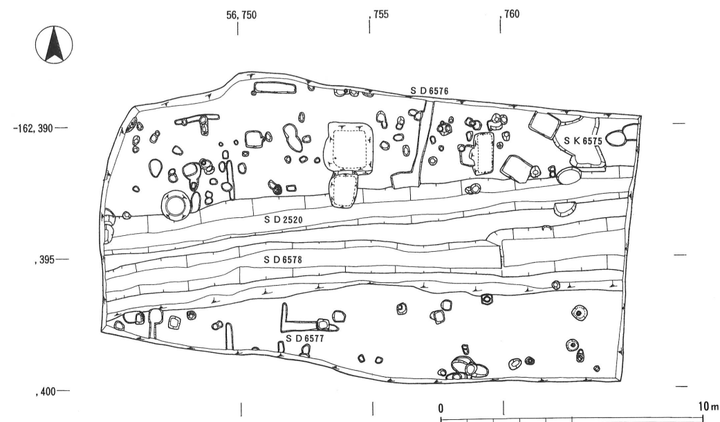
第3図 遺構実測図(1/200)
