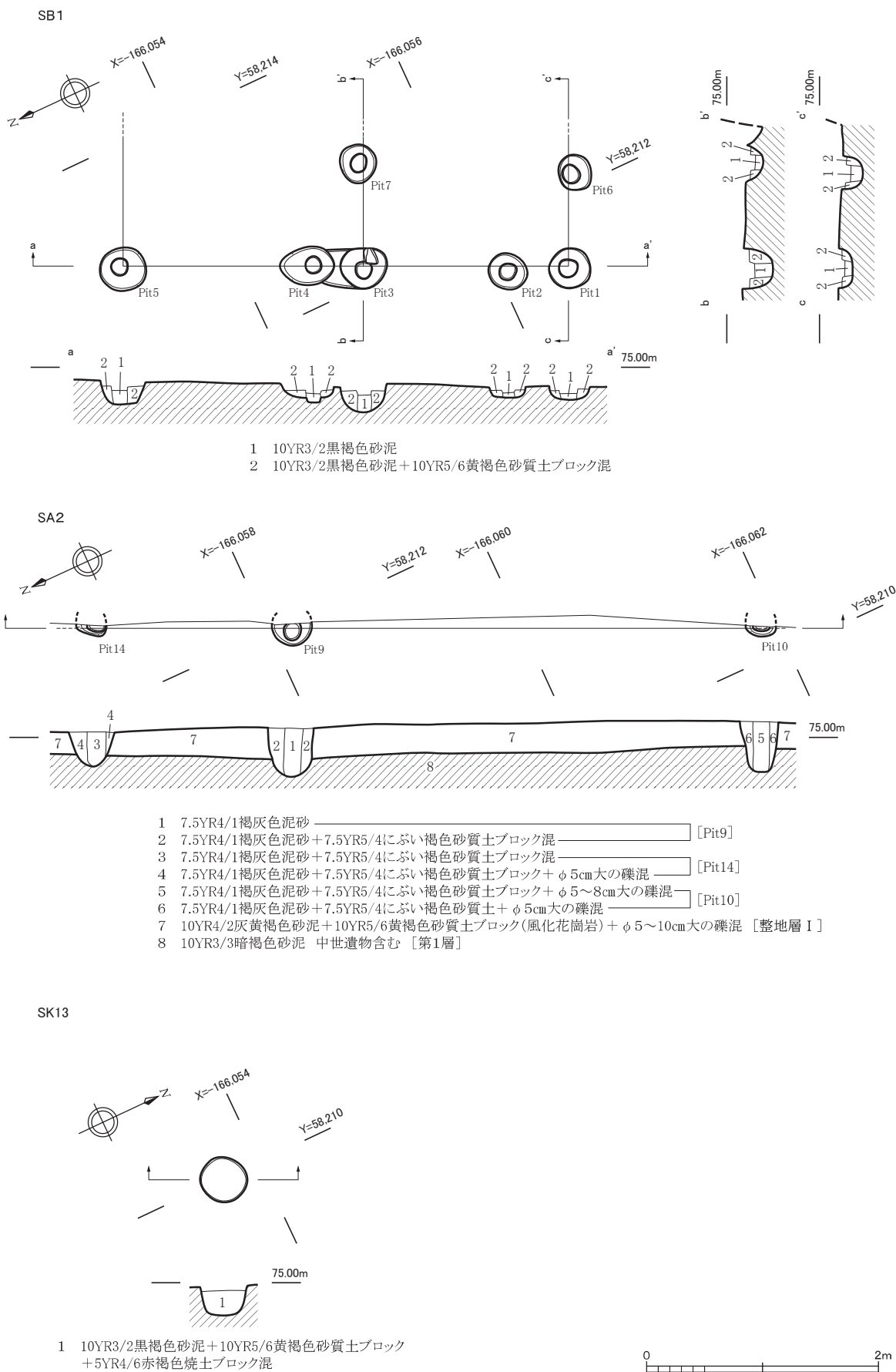
第5次調査区（2トレンチ）SB1、SA2、SK13平・断面図（1：50）
