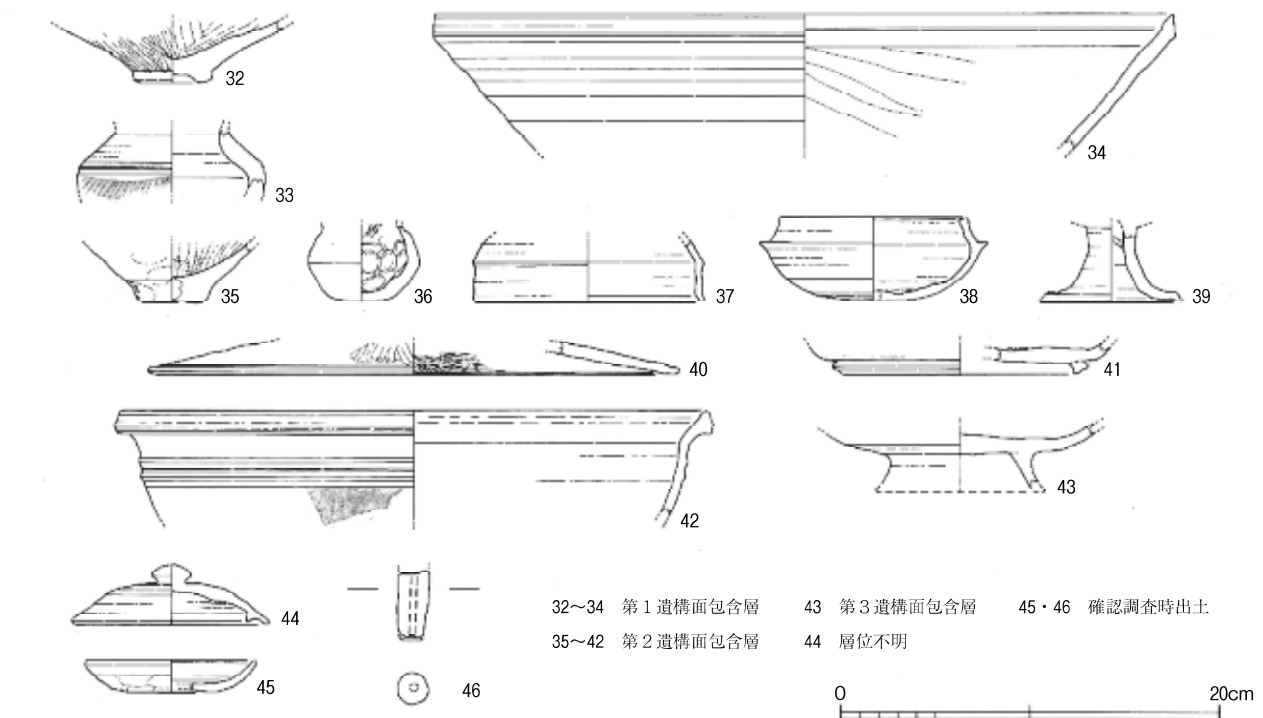
第13図 出土遺物実測図(3) 1/4
