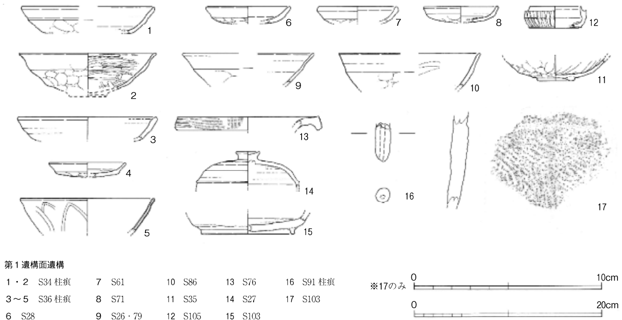
第11図 出土遺物実測図(1) 1/2・1/4
