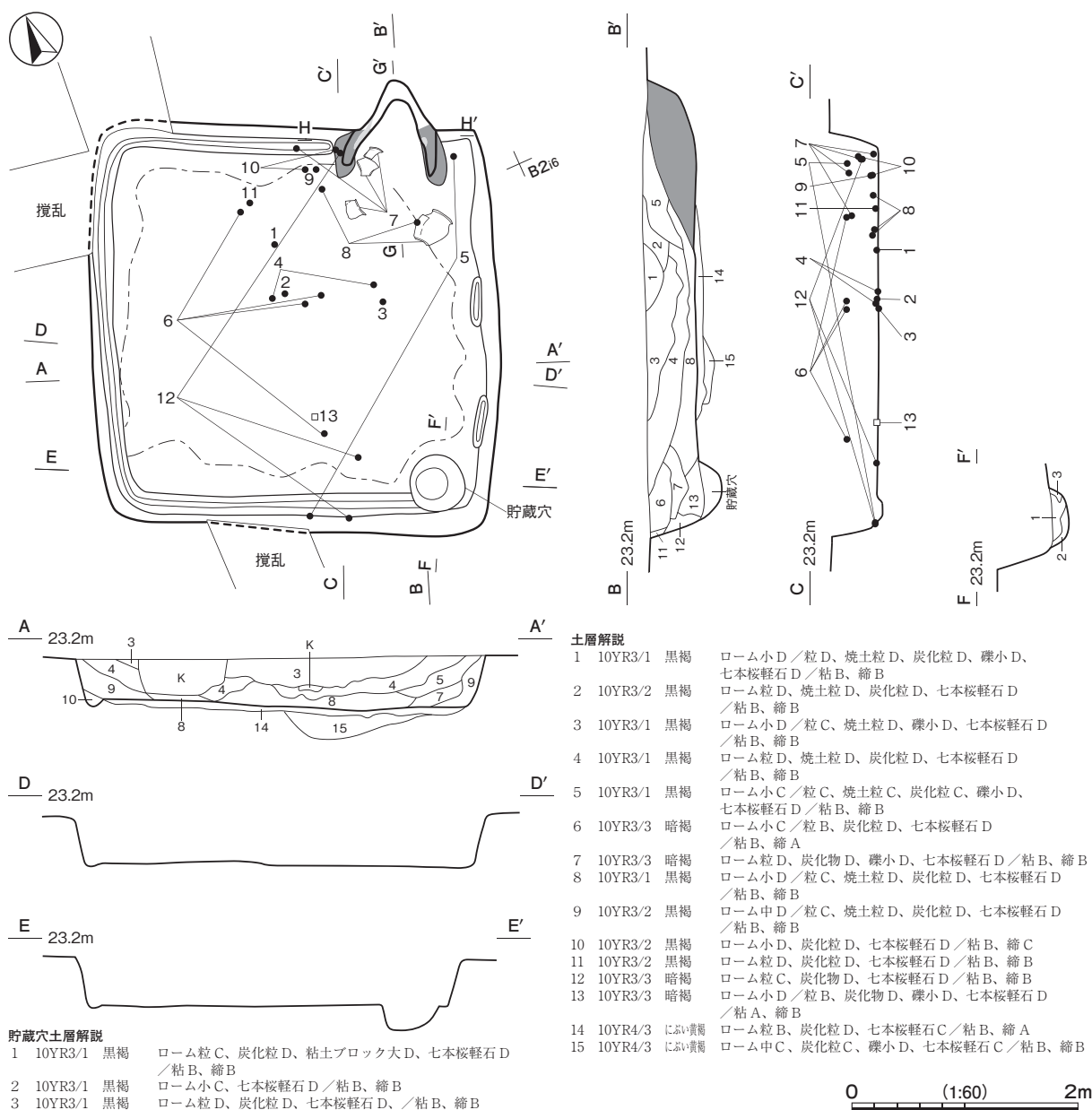
第5図 第1号竪穴建物跡実測図(1)
