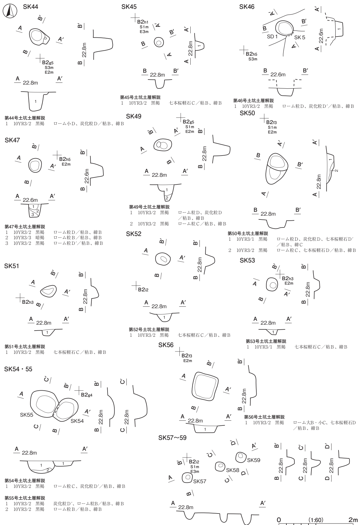
第 38 図 その他の土坑実測図 (4)
