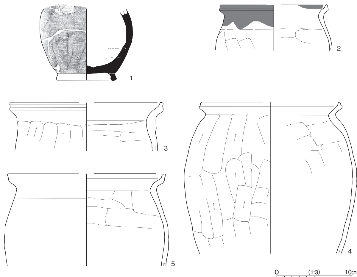
第12図 第3号竪穴建物跡出土遺物実測図(1)
