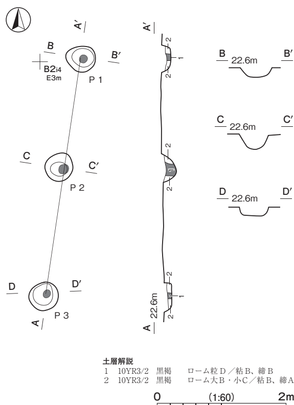
第 41 図 第 1 号柱穴列実測図
