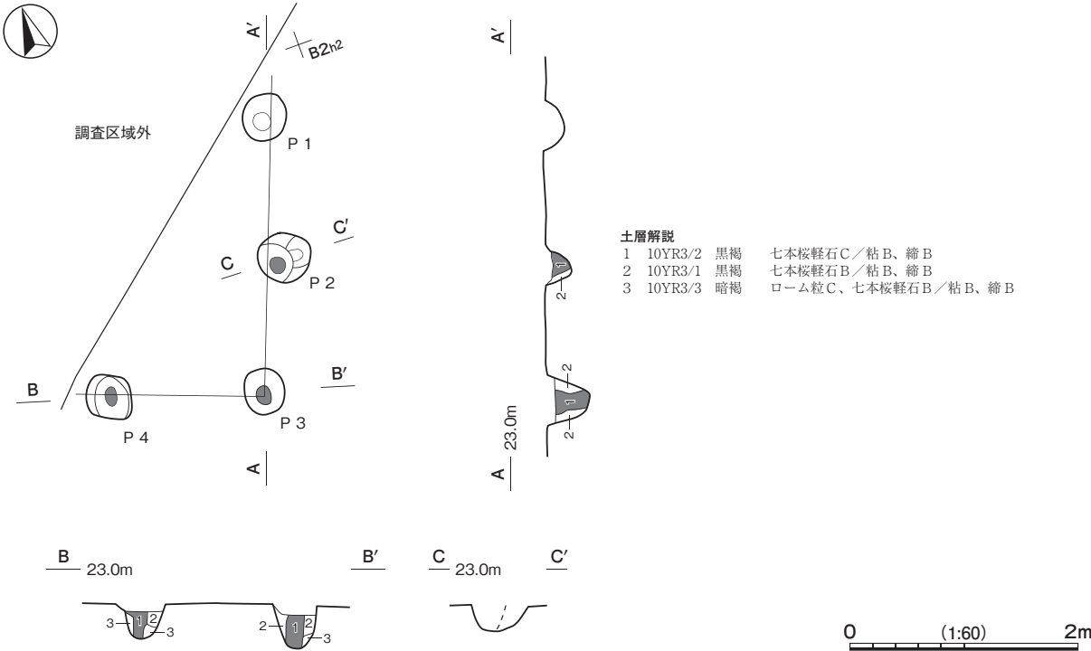
第 27 図 第 1 号掘立柱建物跡実測図
