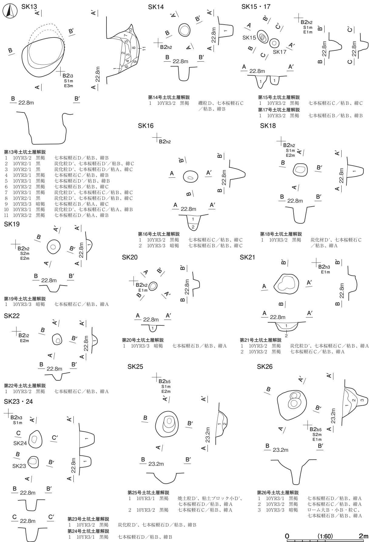
第 36 図 その他の土坑実測図 (2)
