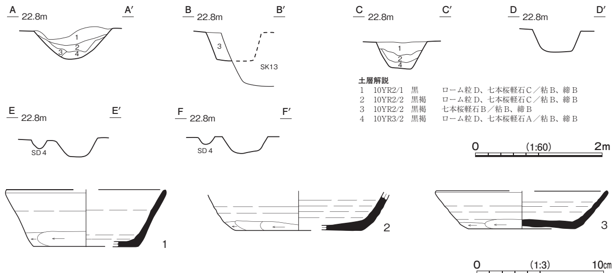
第15図 第1号溝跡・出土遺物実測図
