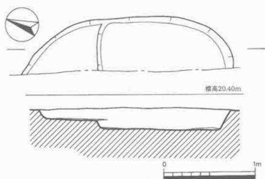
第21図 SK50実測図 (1/40)
