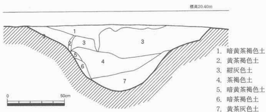
第19図 SD96土層断面図 (1/20)
