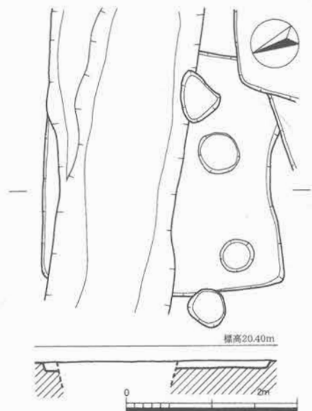
第15図 SI 100実測図 (1/60)
