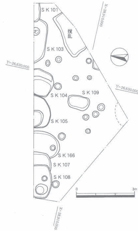
第6図 調査2区遺構配置図 (1/100)
