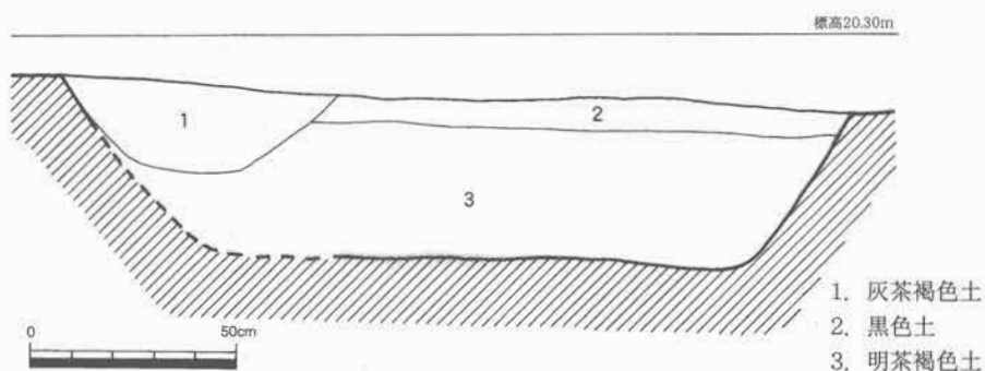
第17図 SD14土層断面図 (1/20)
