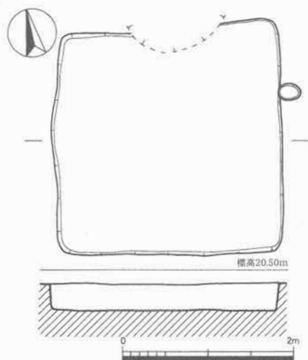
第8図 S I 2実測図 (1/60)
