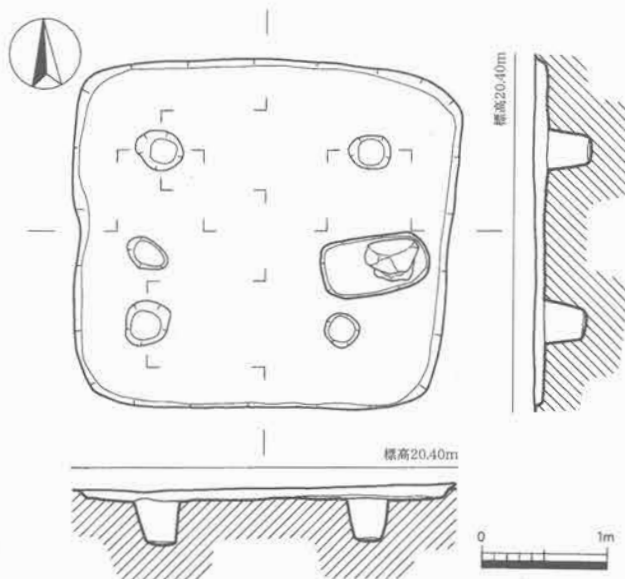
第11図 S I 34実測図 (1/60)
