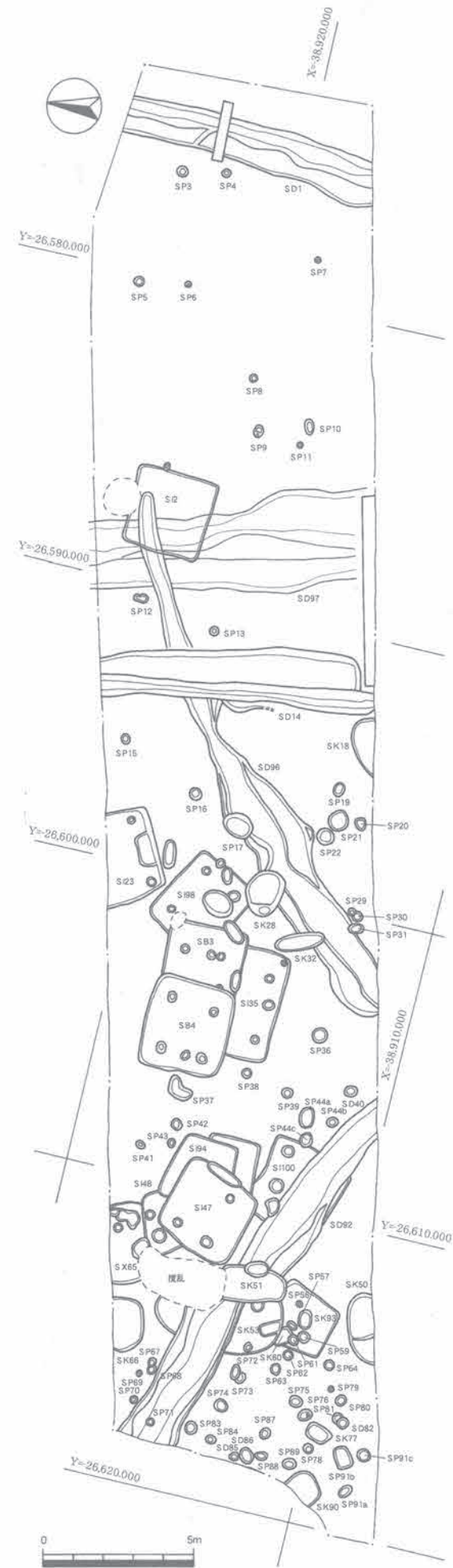
第5図 調査1区遺構配置図 (1/200)
