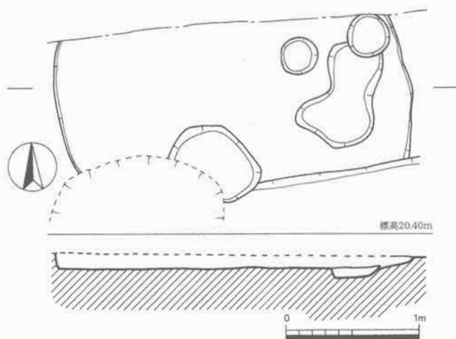
第24図 SK65実測図 (1/40)
