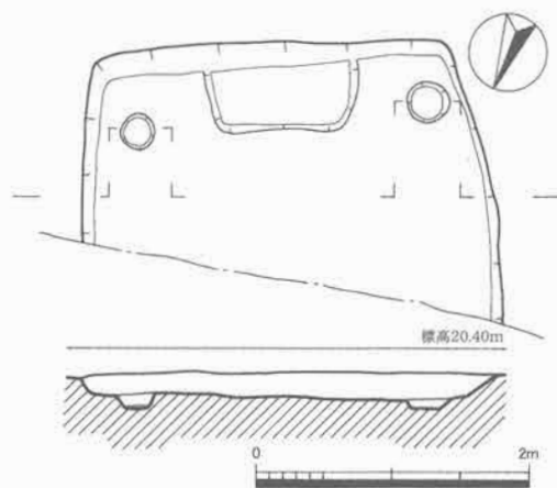
第9図 S I 23実測図 (1/60)
