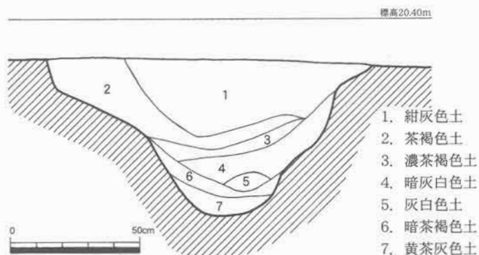
第18図 SD92土層断面図 (1/20)
