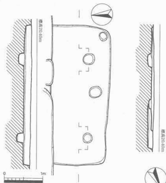
第12図 S I 35実測図 (1/60)
