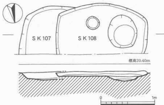
第31図 S K 107・108実測図 (1/40)
