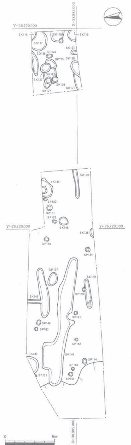
第7図 調査3区遺構配置図 (1/200)
