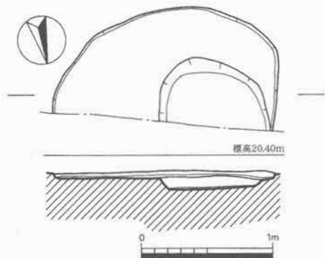
第29図 S K 105実測図 (1/40)
