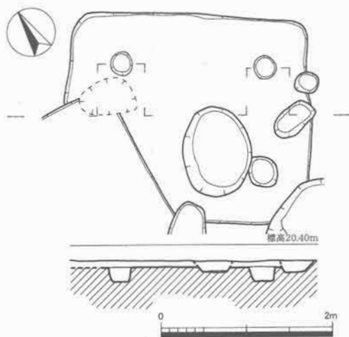
第14図 SI 98実測図 (1/60)
