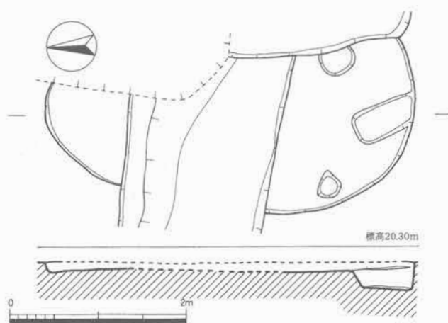
第23図 SK53実測図 (1/60)
