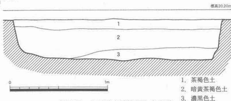
第20図 SD97土層断面図 (1/20)
