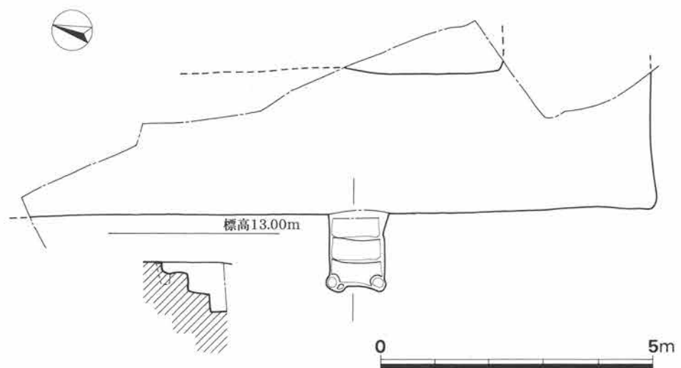
第16図 S X 6 防空壕実測図（1/100）
