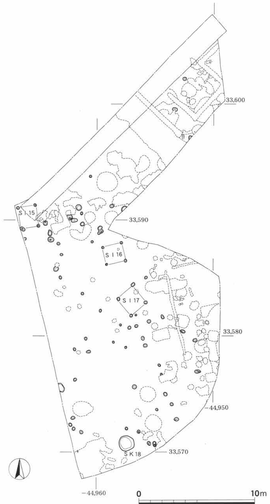
第24図 E区遺構配置図 (1/200)
