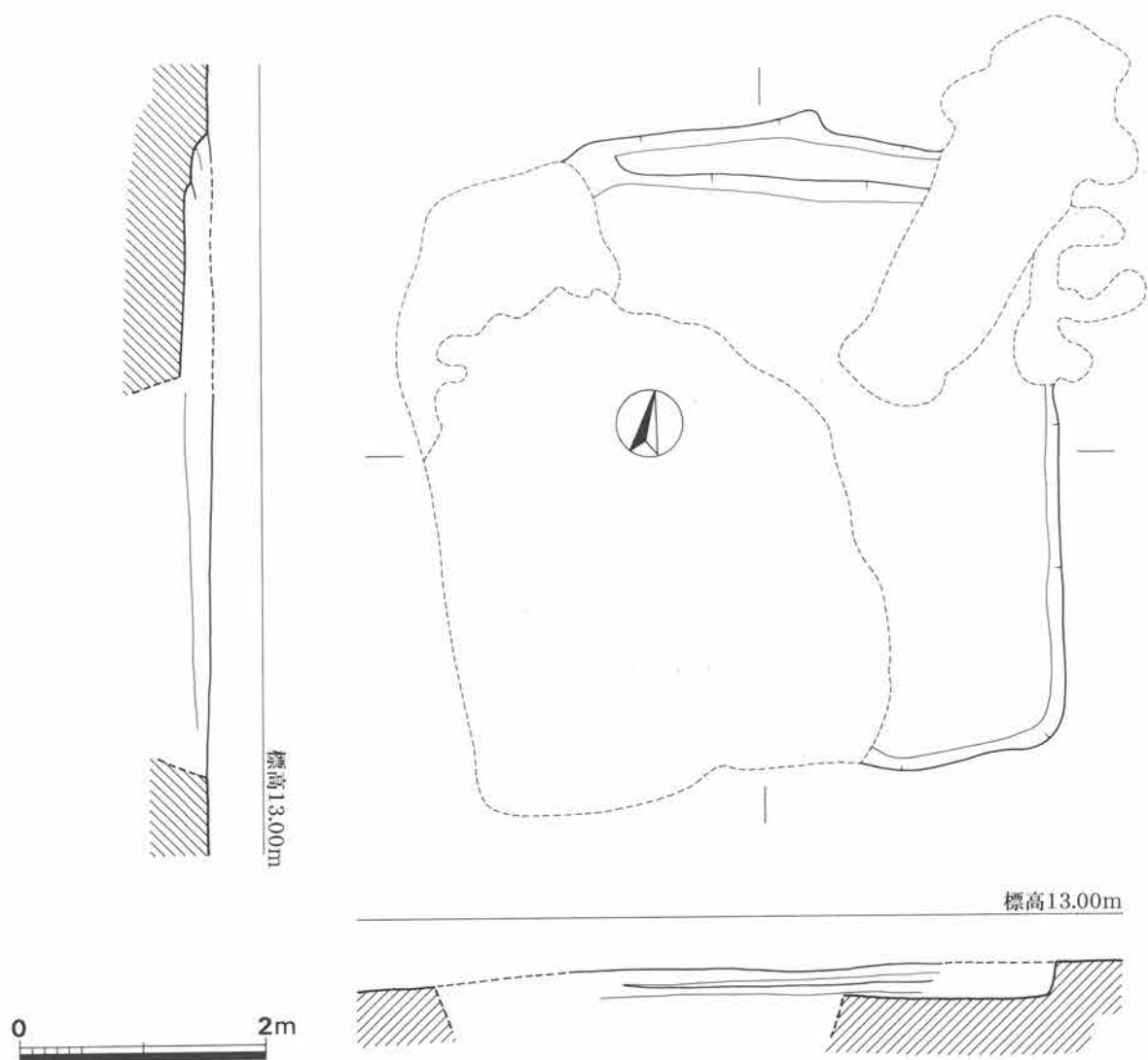
第13図 S I 5 実測図 (1/60)
