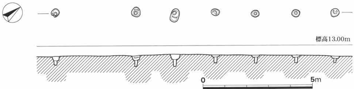
第19図 SA 7 実測図 (1/100)
