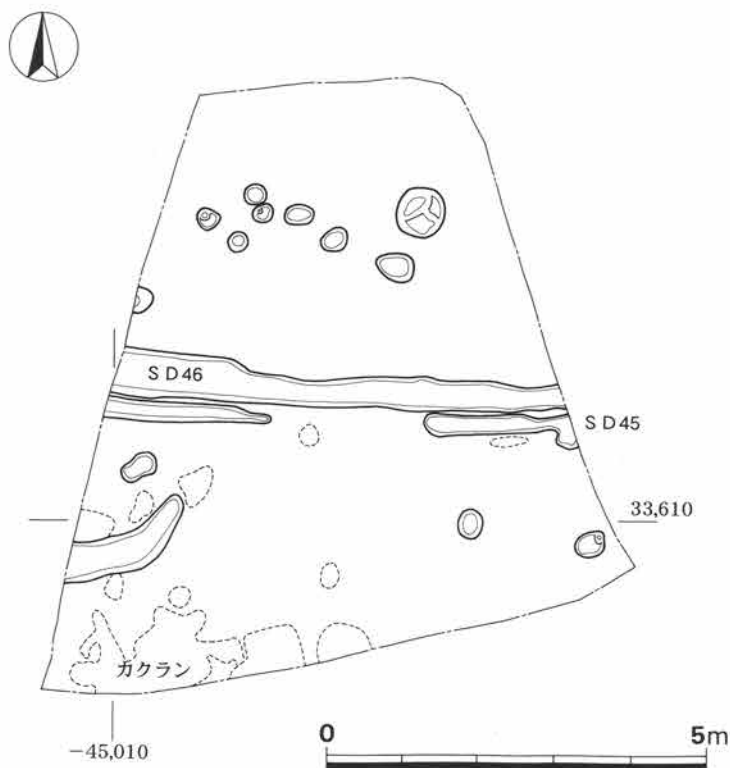
第37図 G-1区遺構配置図（1/100）
