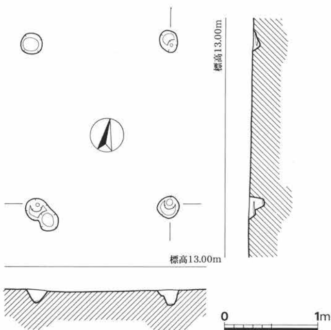
第28図 S I 15実測図 (1/40)
