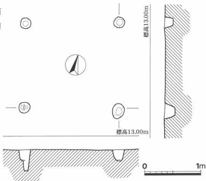
第30図 S I 16実測図（1/40）
