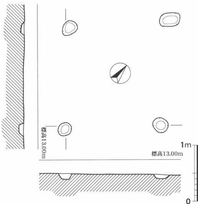
第32図 S I 17実測図（1/40）
