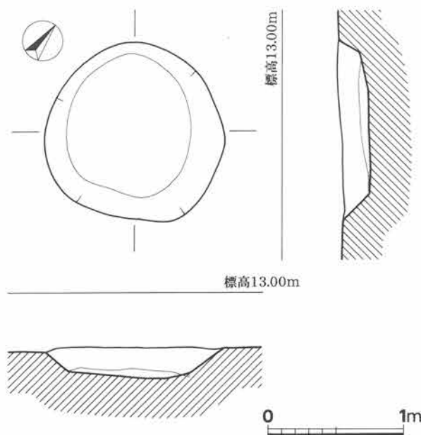
第34図 S K 18実測図 (1/40)
