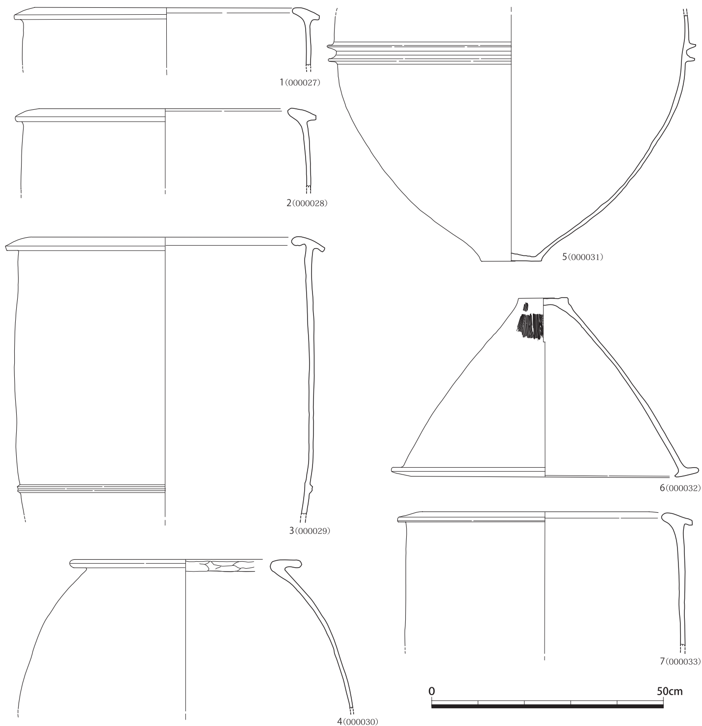
図15 SD 1 出土遺物実測図① (1/8)
