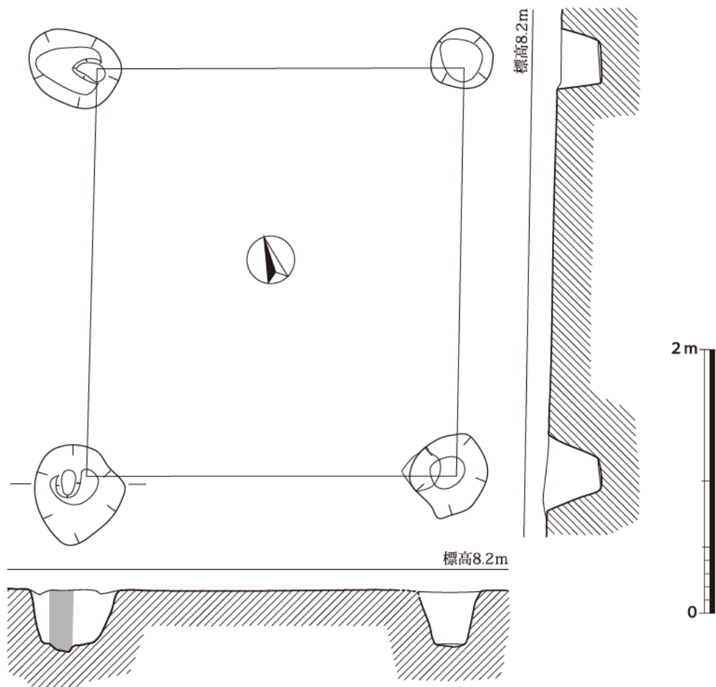
図6 S I 100 平面・断面見通し図 (1/40)
