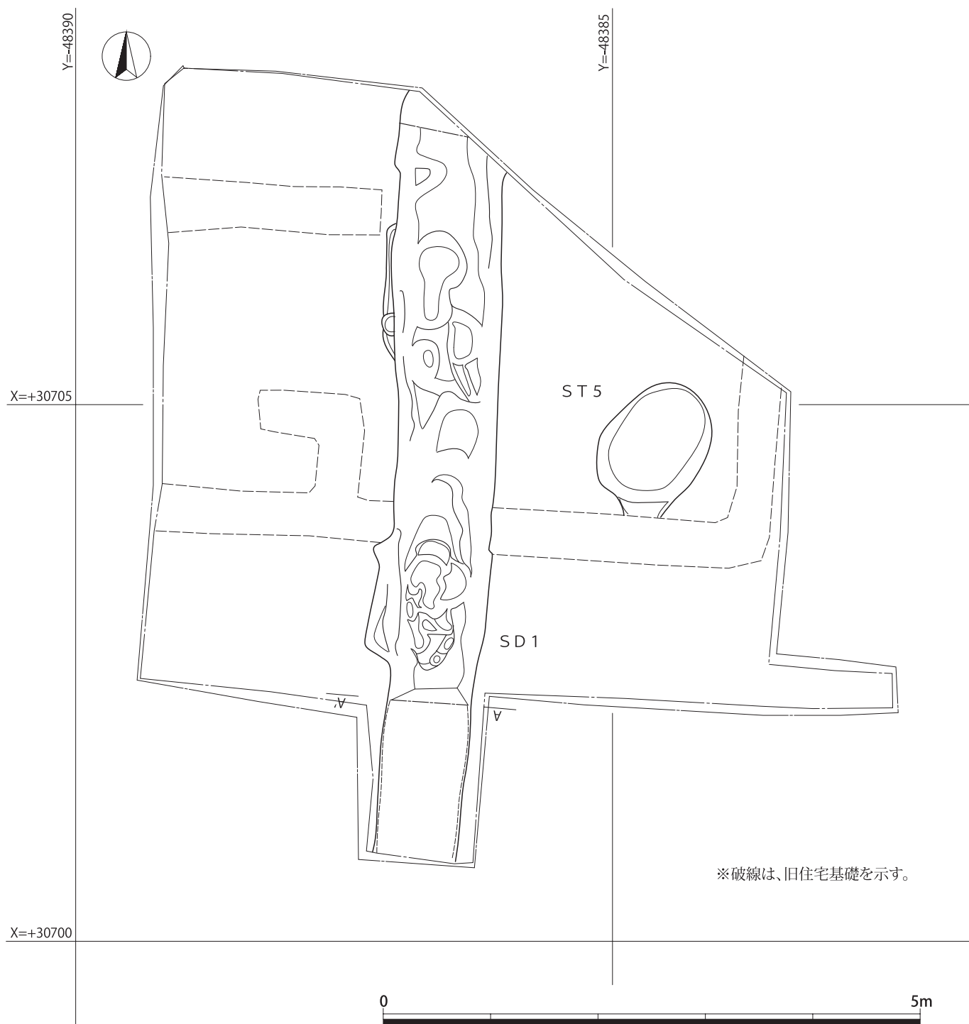
図11 第2次調査区平面図 (1/50)
