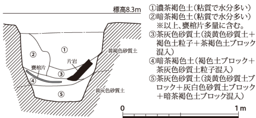
図13 SD1土層断面図 (1/20)
