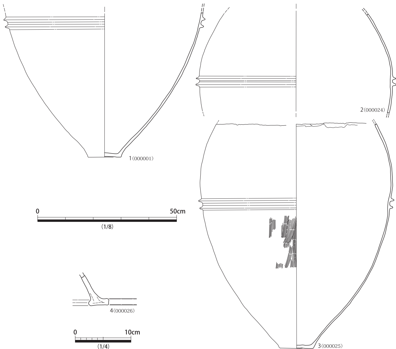
図9 S T 10・70・80 出土遺物実測図 (1/4・1/8)
