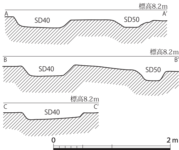
図8 SD40・50 断面図 (1/40)
