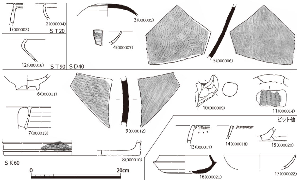
図10 ST 20・SD 40・SK 60・ST 90 ピット出土遺物実測図 (1/4)
