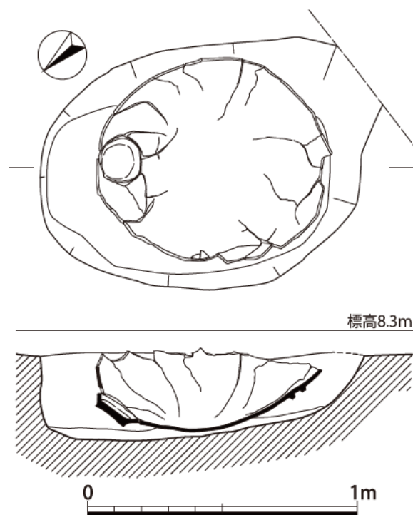
図12 ST5平面・断面見通し図 (1/20)
