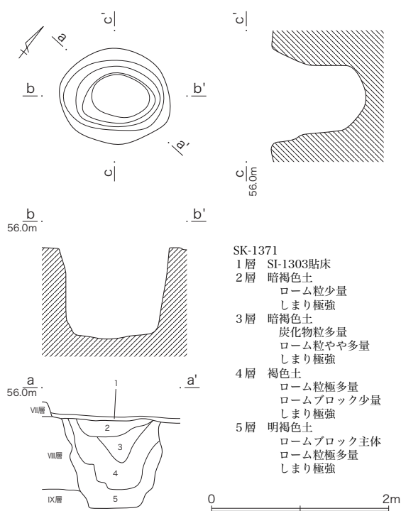
第387図 SK-1371 陥穴状遺構
