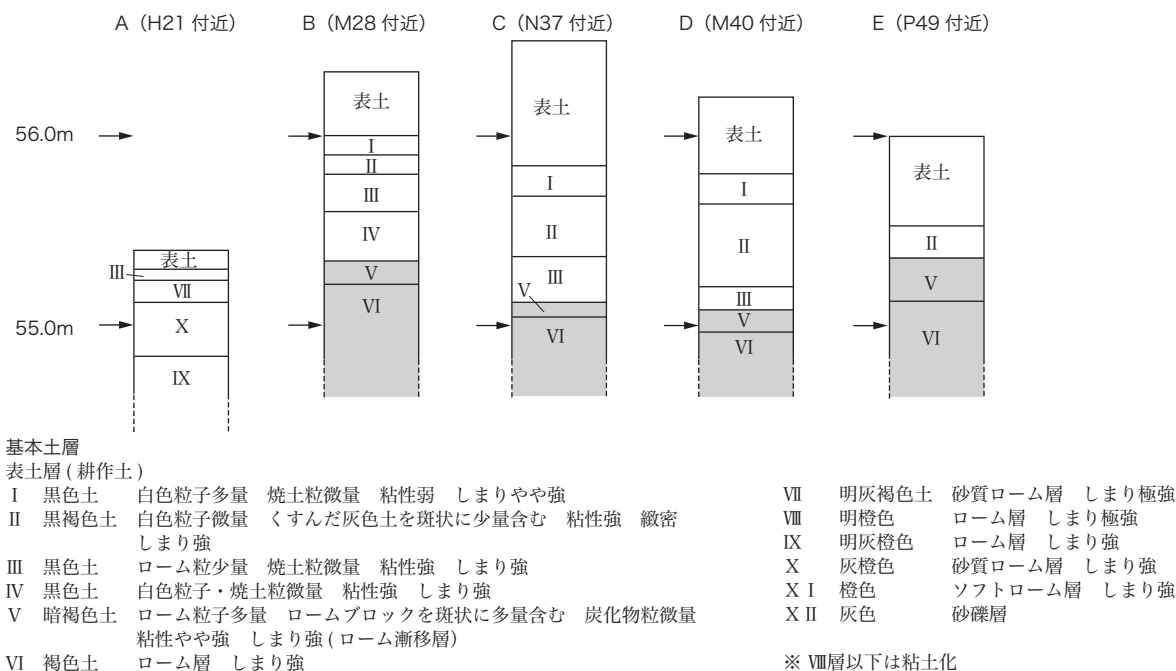
第 371 図 低地の基本土層
