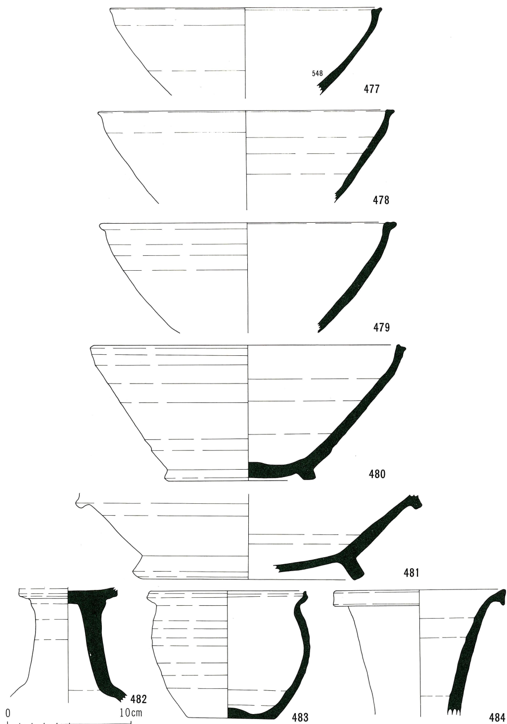
第33図 鉢伏3号窯址出土遺物実測図
