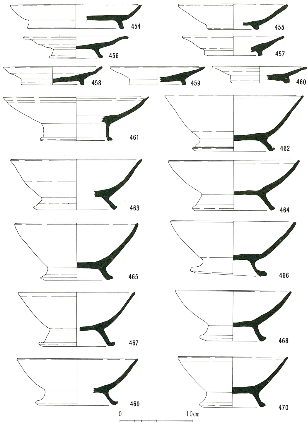
第31図 鉢伏3号窯址出土遺物実測図
