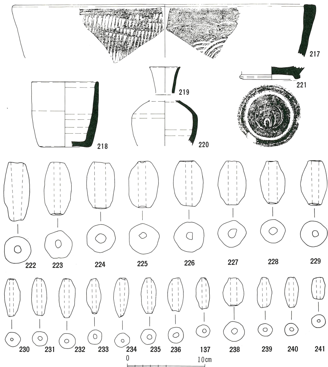
第22図 鉢伏2号窯址出土遺物実測図
