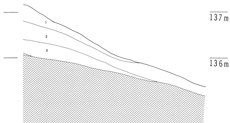
第10図 2号窯址灰原セクション図
