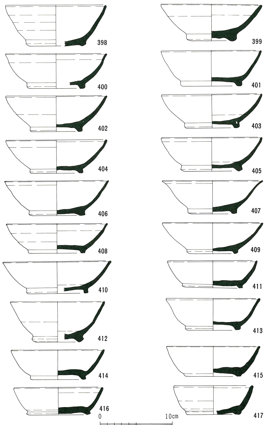
第29図 鉢伏3号窯址出土遺物実測図
