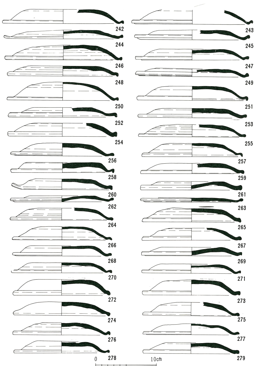
第24图 鉢伏3号窯址出土遺物実測図
