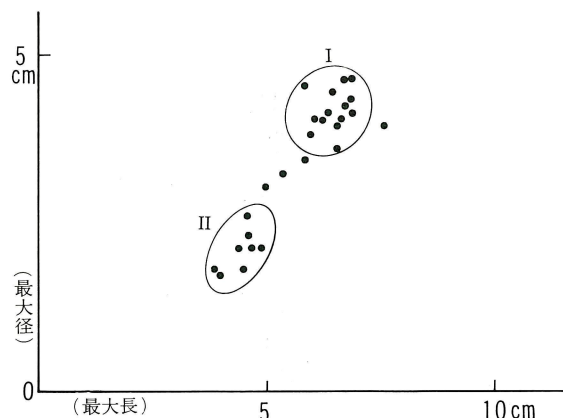
第52図 鉢伏3号窯址出土陶鍾法量図
