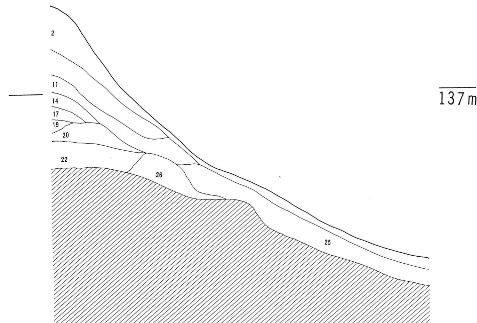
第23図 3号窯址灰原セクション図
