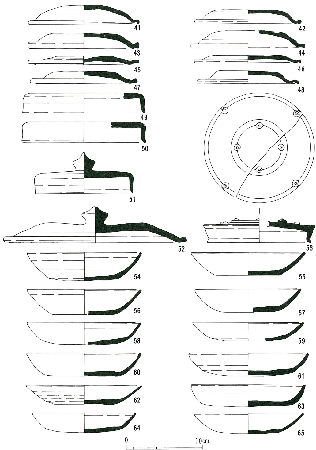
第12図 鉢伏2号窯址出土遺物実測図
