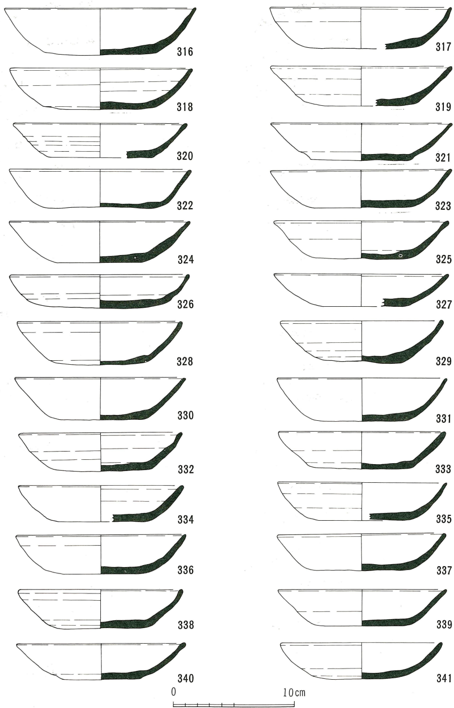
第26図 鉢伏3号窯址出土遺物実測図
