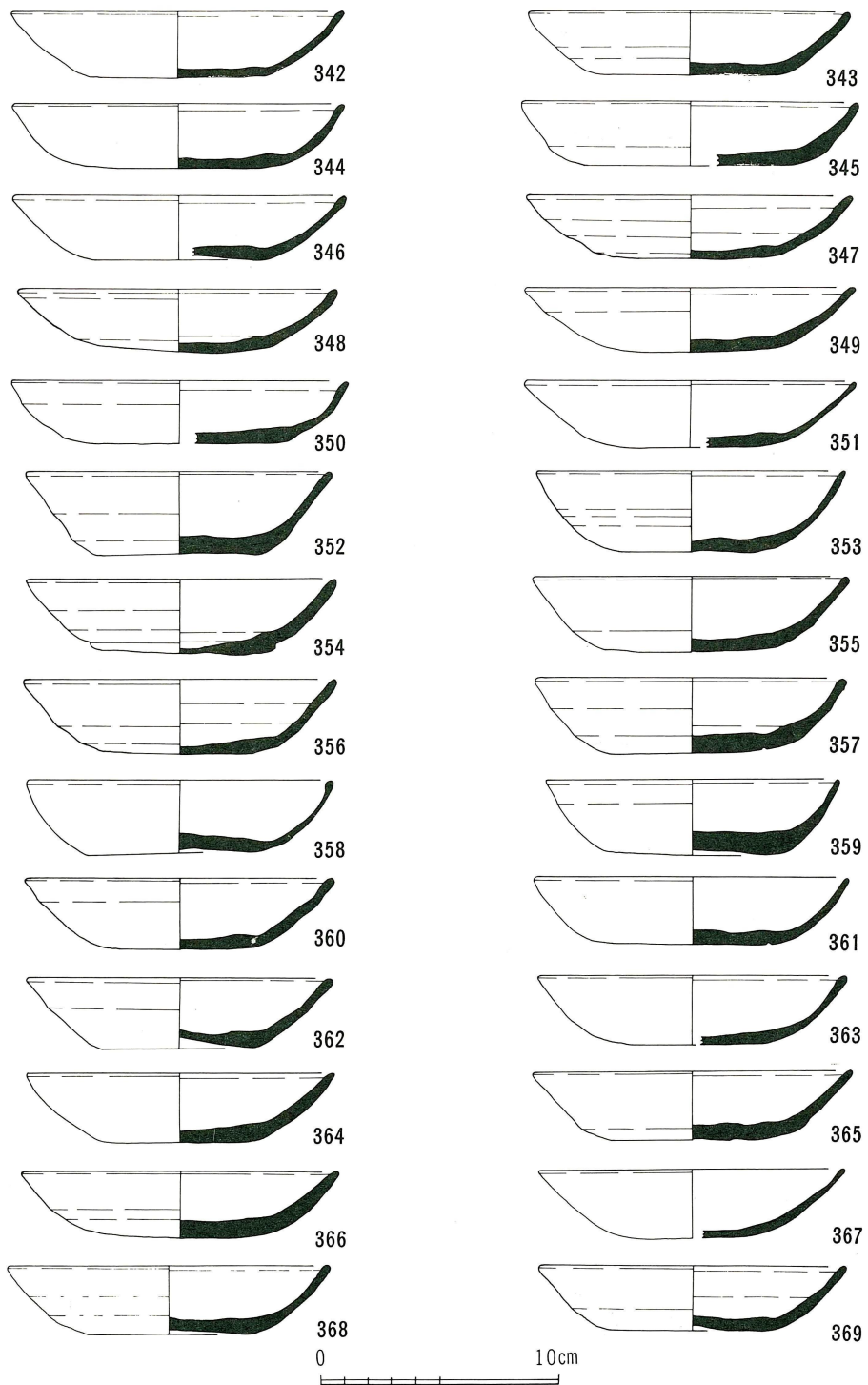
第27図 鉢伏3号窯址出土遺物実測図
