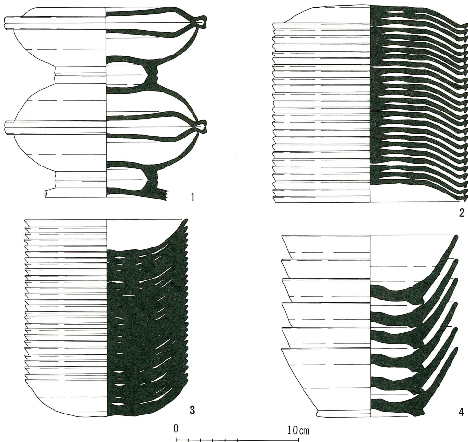
第53図 鉢伏2，3号窯址重ね焼き模式図
