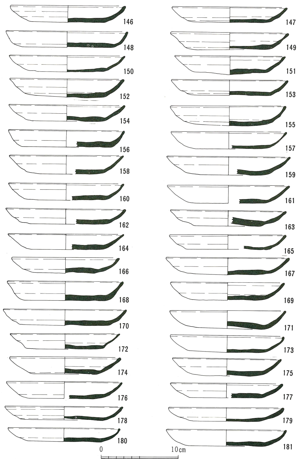
第16図 鉢伏2号窯址出土遺物実測図
