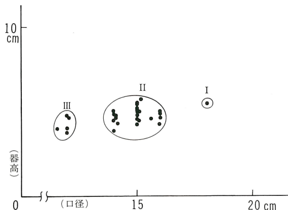
第43図 鉢伏2号窯址出土坏B法量図
