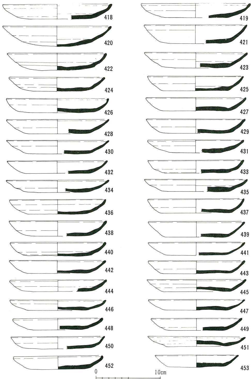
第30図 鉢伏3号窯址出土遺物実測図
