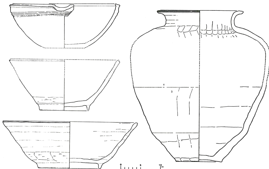
第7図 江波経塚群出土遺物実測図
