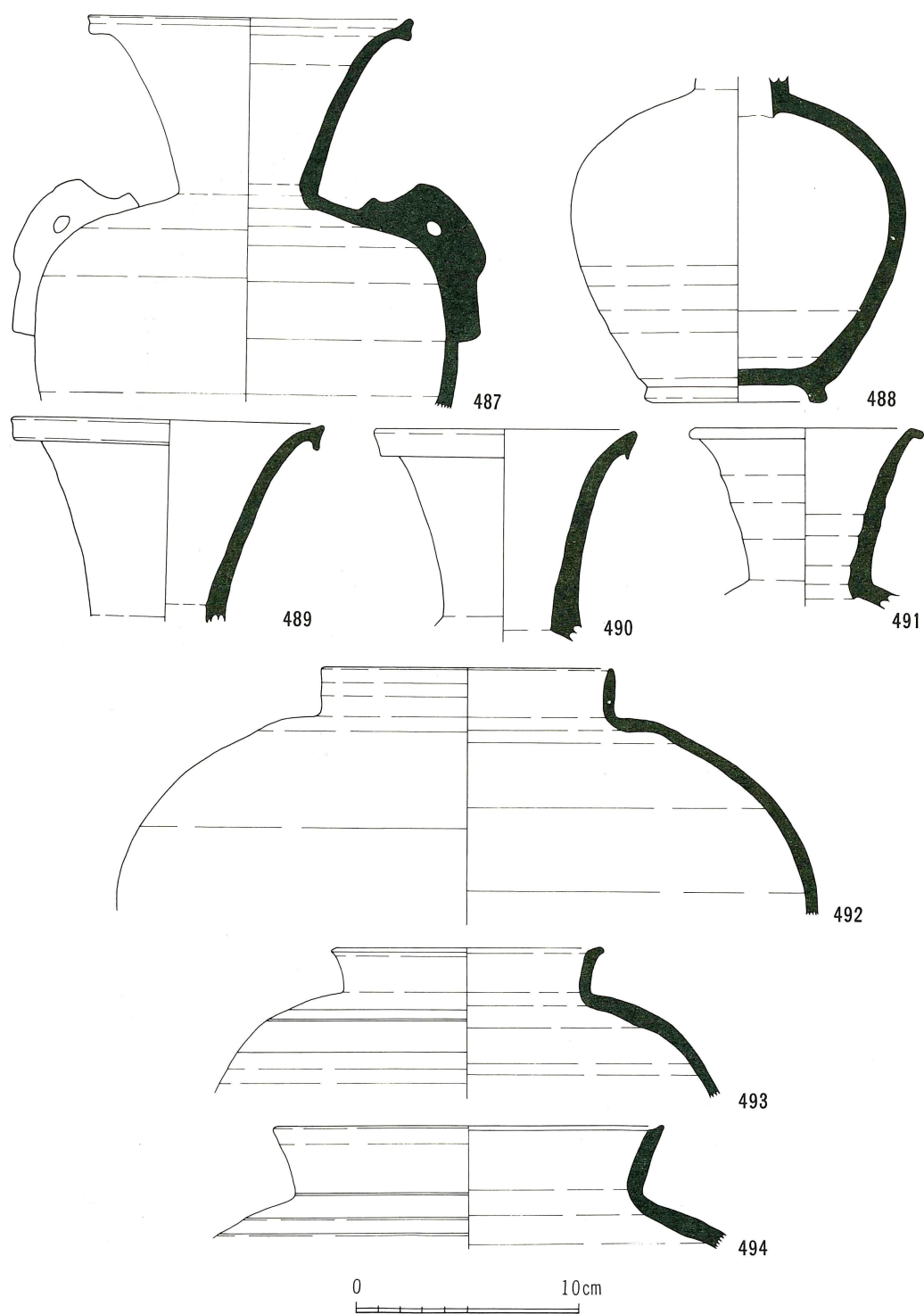
第35図 鉢伏3号窯址出土遺物実測図
