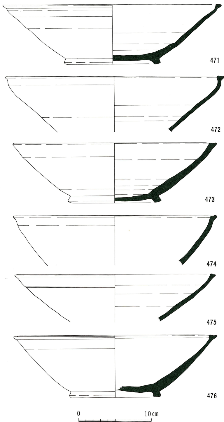
第32図 鉢伏3号窯址出土遺物実測図
