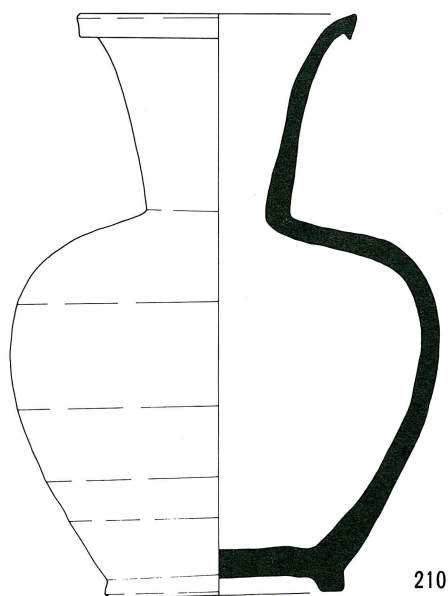
第20図 鉢伏2号窯址出土遺物実測図
