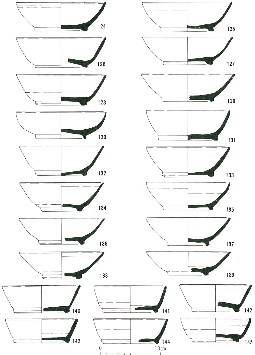
第15図 鉢伏2号窯址出土遺物実測図
