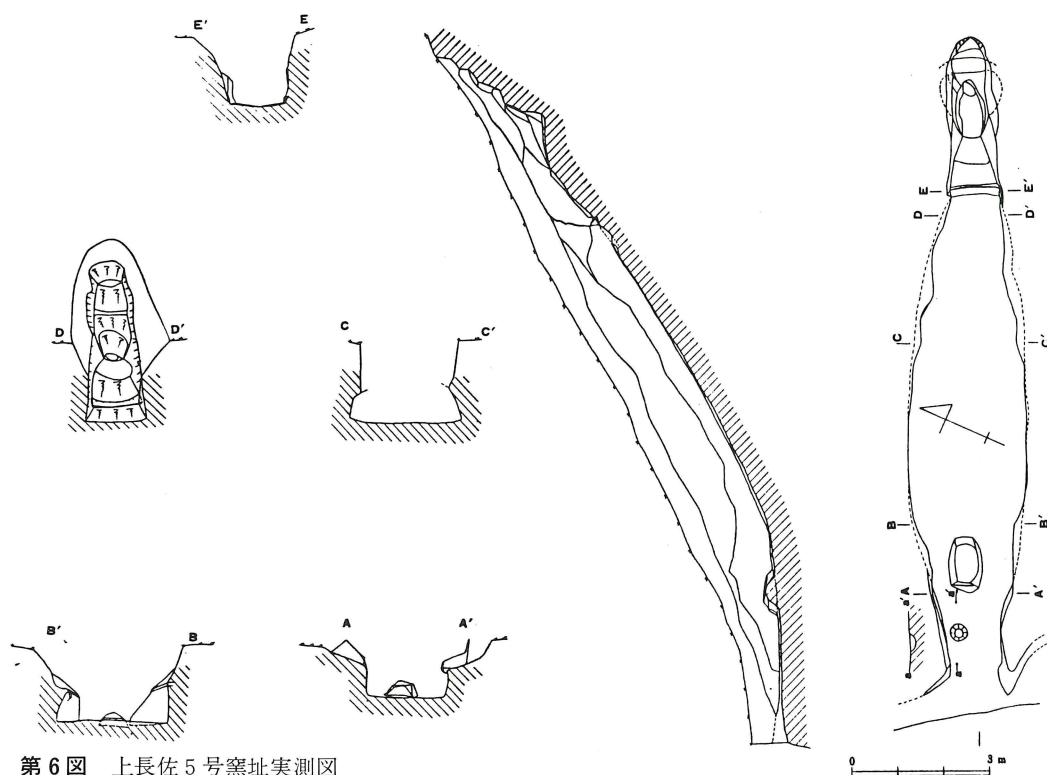
第6図 上長佐5号窯址実測図
