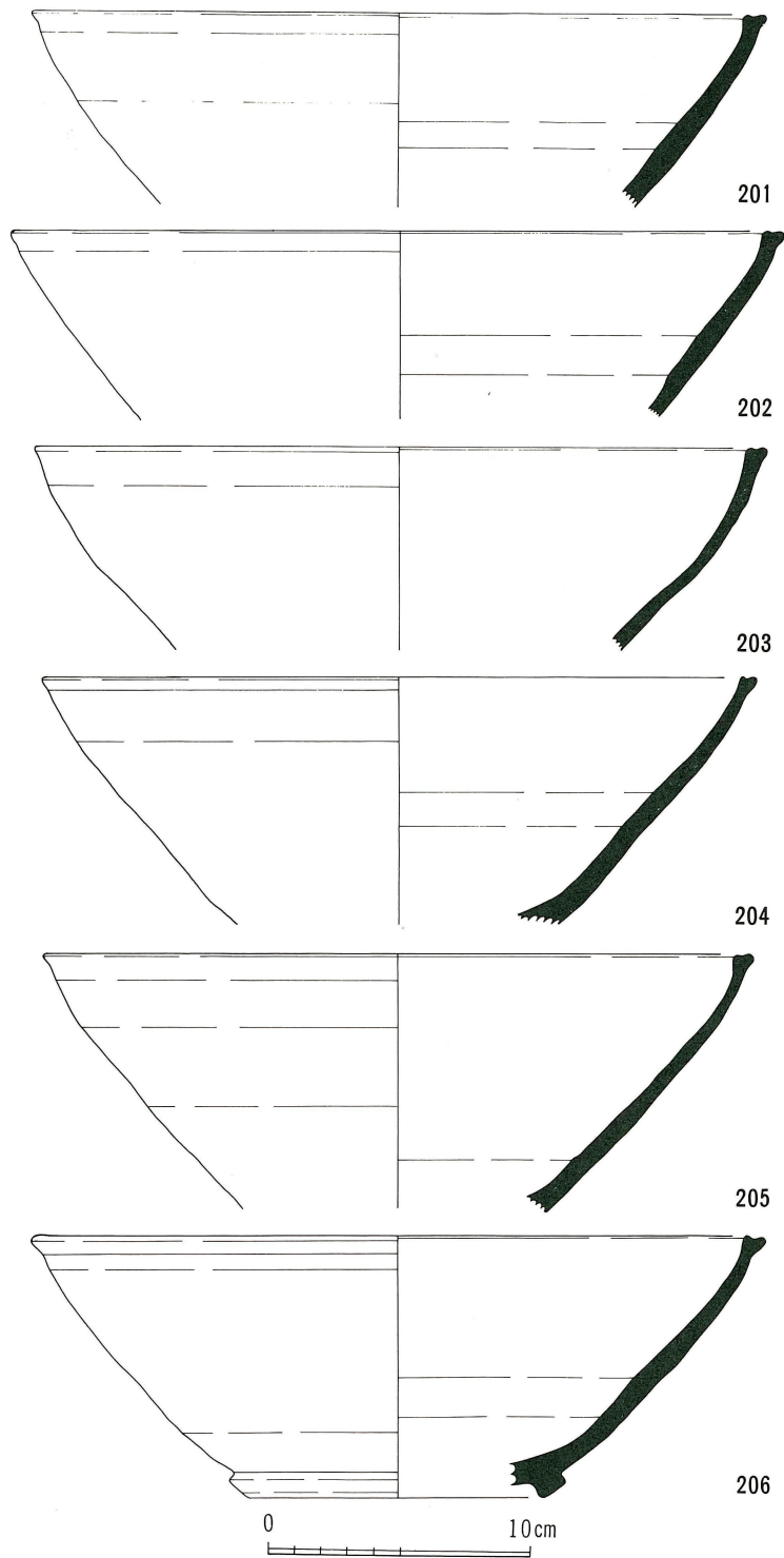
第19図 鉢伏2号窯址出土遺物実測図
