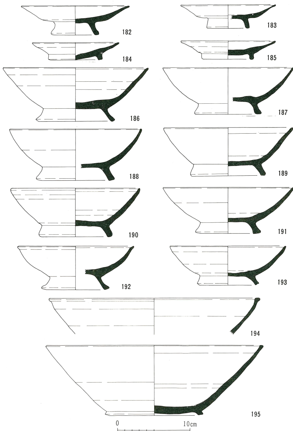
第17図 鉢伏2号窯址出土遺物実測図
