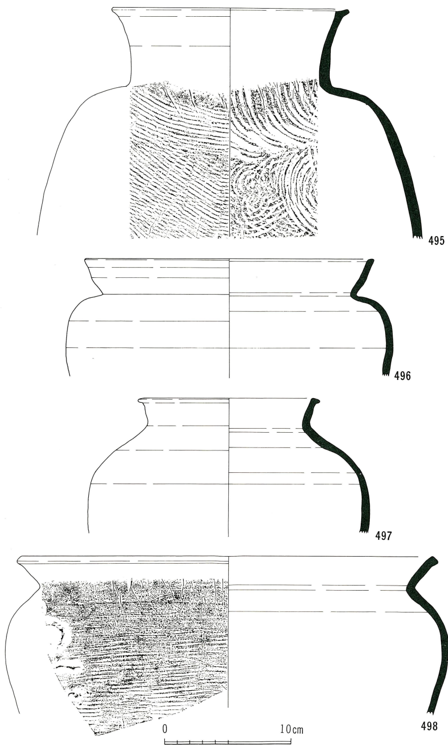
第36図 鉢伏3号窯址出土遺物実測図
