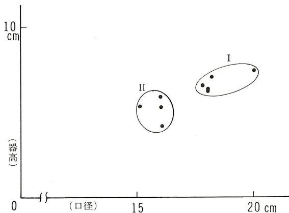
第49図 鉢伏2号窯址出土椀B法量図
