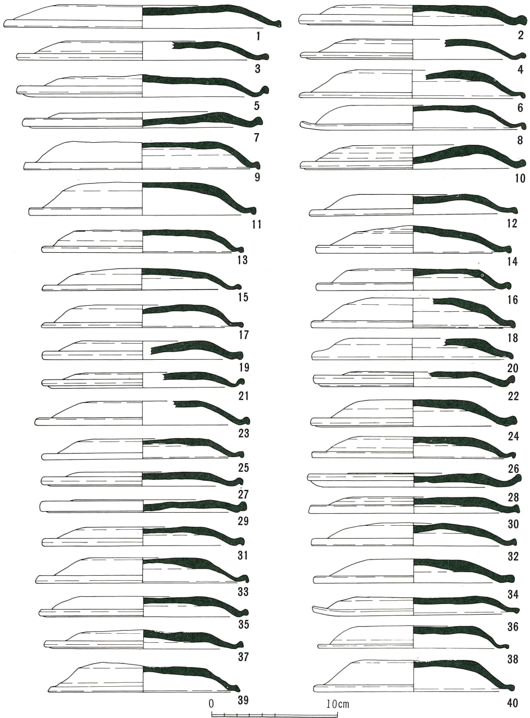
第11図 鉢伏2号窯址出土遺物実測図
