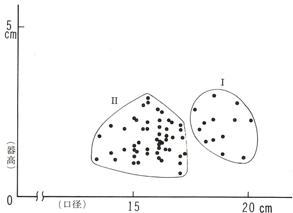
第40図 鉢伏3号窯址出土蓋法量図
