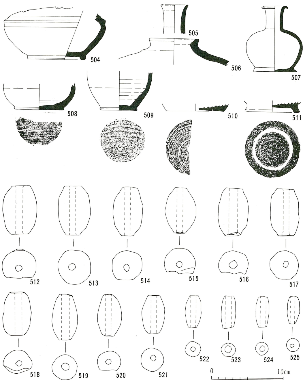
第38図 鉢伏3号窯址出土遺物実測図
