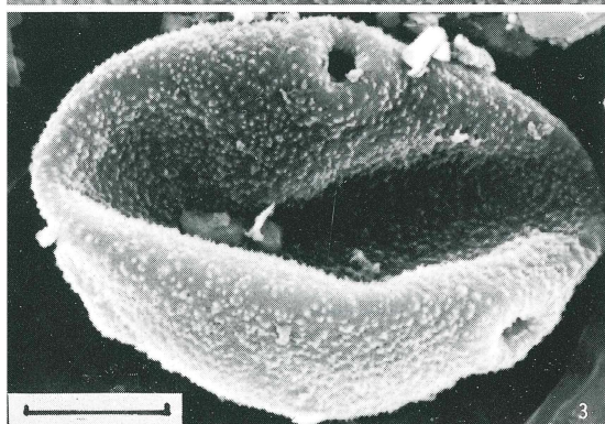
1 イネ属型 (棒5ミクロン)、2 イネ属型 (棒5ミクロン)、 3 クワ科 (カナムグラ型) (棒5ミクロン)、 4～5 クワ科 (×750倍)、6～7 イネ科 (×750倍)
