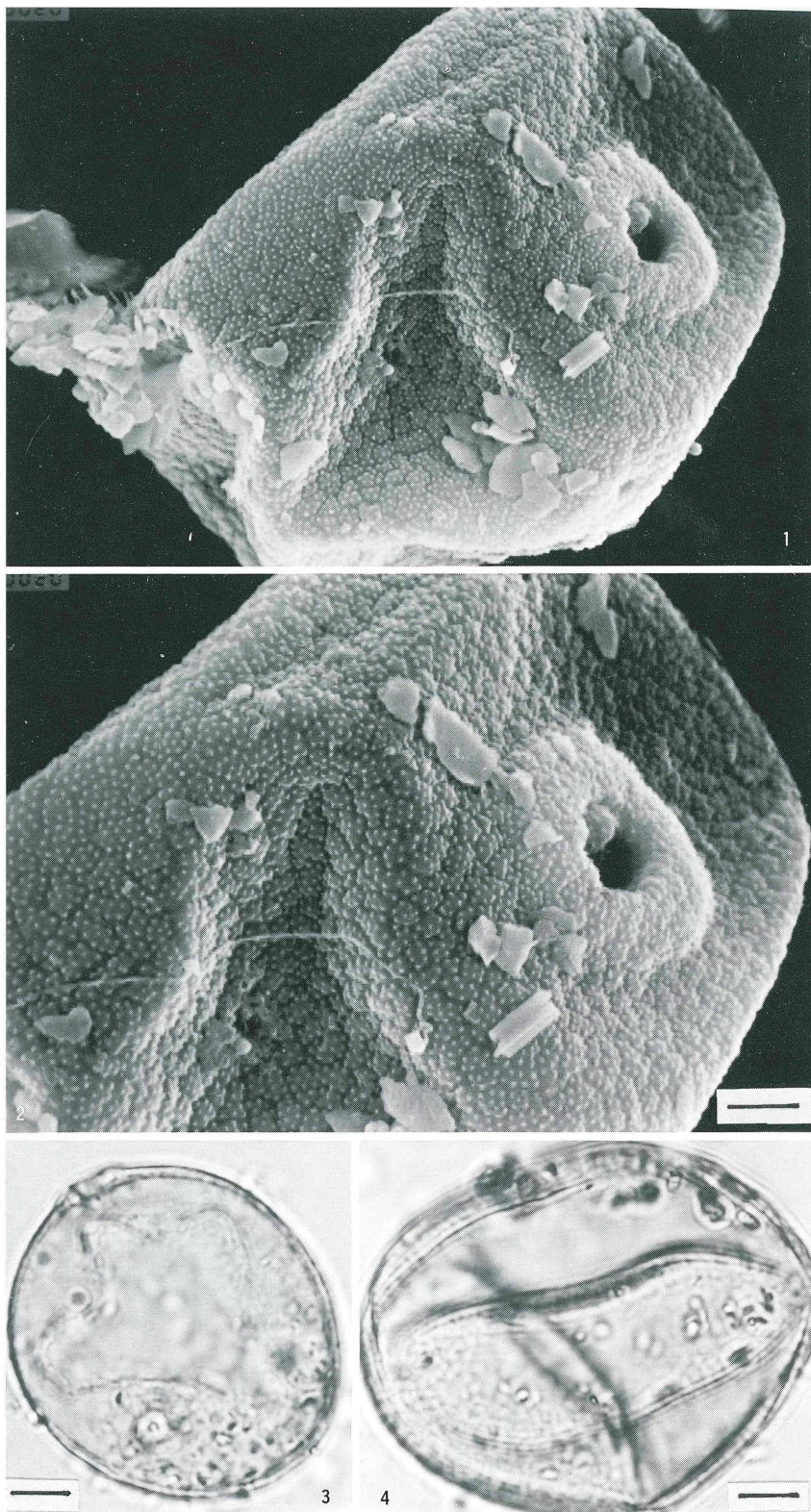
1 イネ科 (棒5ミクロン)、2 イネ科 (棒2ミクロン)、3 イネ科 (棒5ミクロン)、 4 イネ科 (棒5ミクロン)
