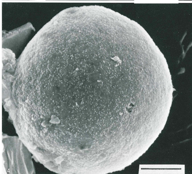
1 アサダ属(?) (棒5ミクロン)、2~3 ヨモギ属 (棒5ミクロン)、4 エノキ属 (棒5ミクロン)、 5 ニレ属 (×750倍)、6 エノキ属 (×750倍)
