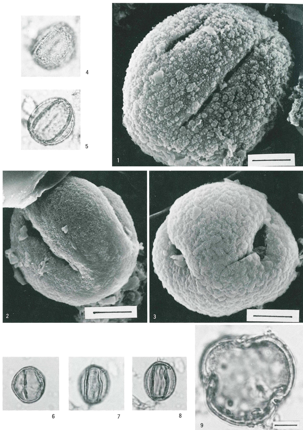
1 カシワ型 (棒5 ミクロン)、2 イチイガシ—シラカシ—ツクバネガシ型 (棒5 ミクロン)、 3 ウラジログシ型 (棒5 ミクロン)、4～5 コナラ亜属 (×750倍)、 6～8 アカガシ亜属 (×750倍)、9 アカガシ亜属 (棒5 ミクロン)
