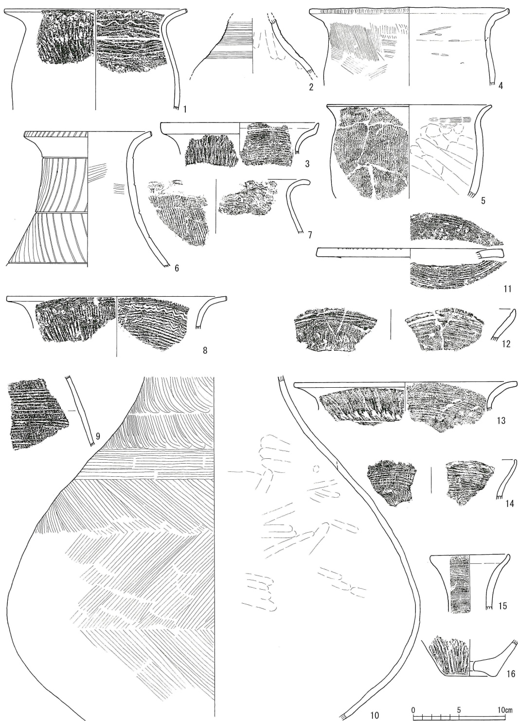
第 82 図 土壙出土土器実測図 7 (縮尺 1/4)
