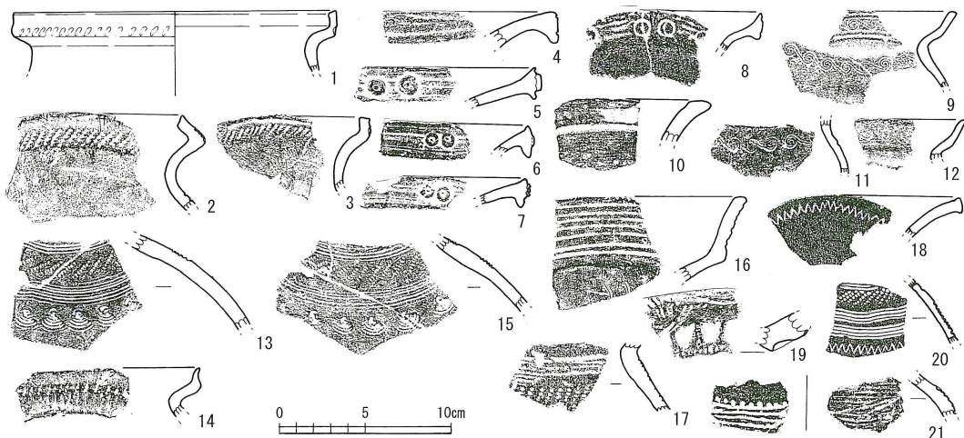
第118図 包含層出土土器実測図4（縮尺1/4）
