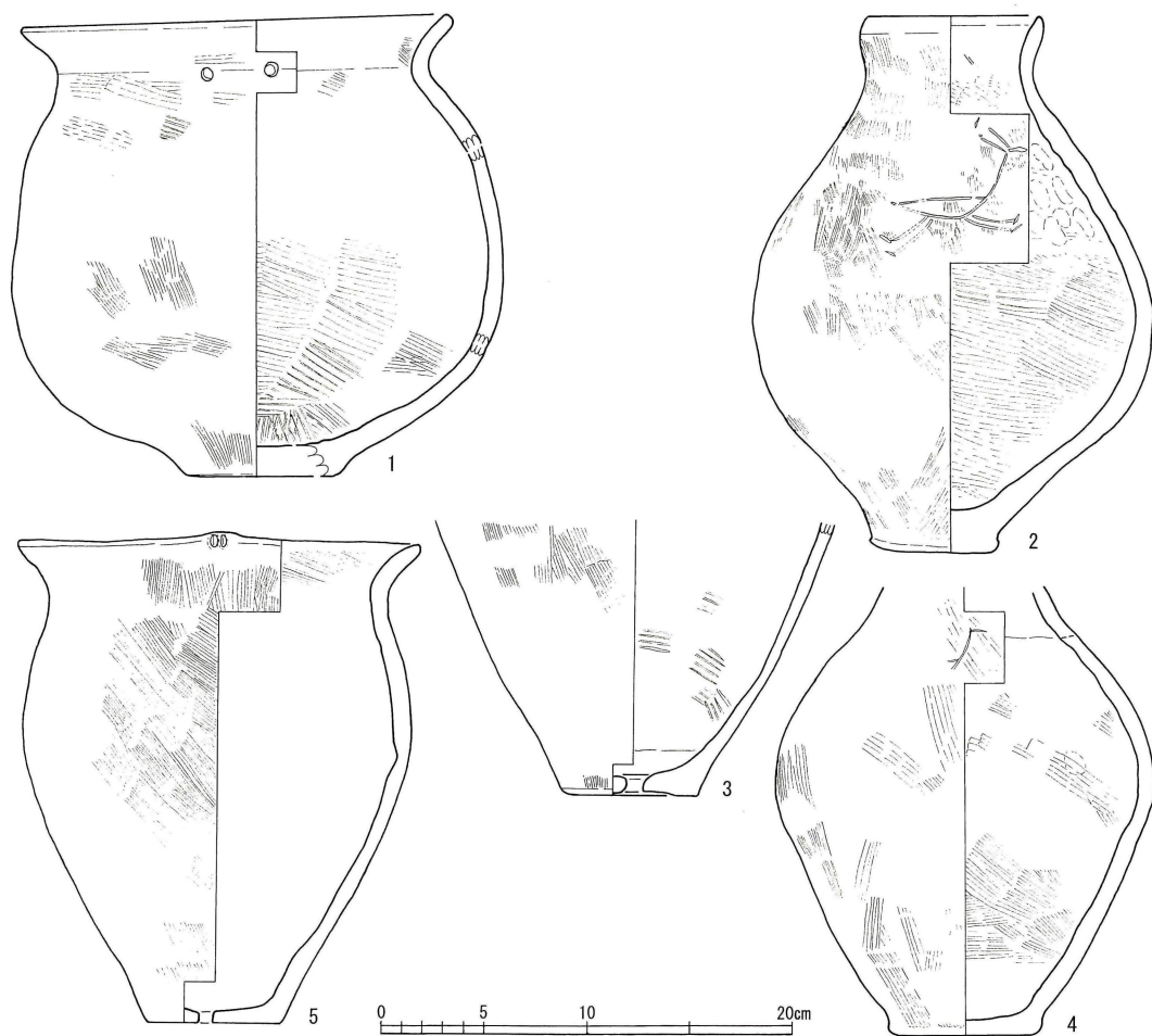
第 89 図 土壇出土土器実測図 14( 縮尺 1/4)
