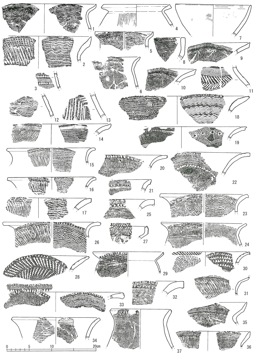
第 87 図 土壙出土土器実測図 12( 縮尺 1/4)
