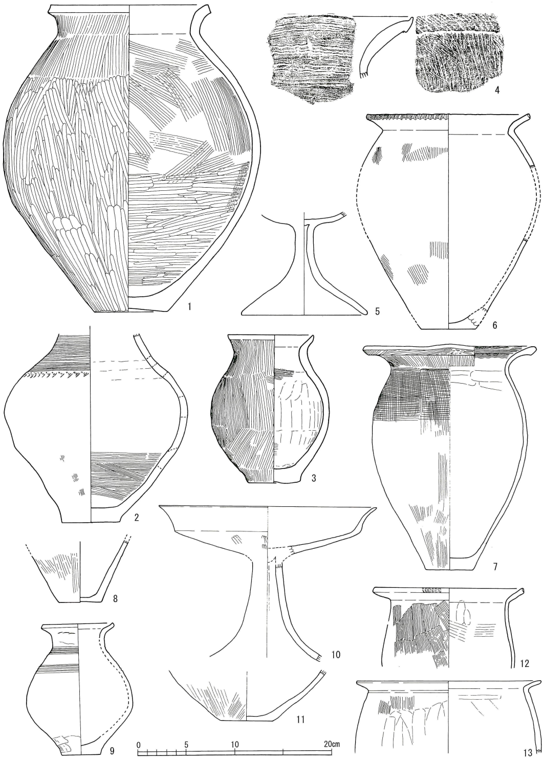
第107図 方形周溝墓出土土器実測図7(縮尺1/4)
