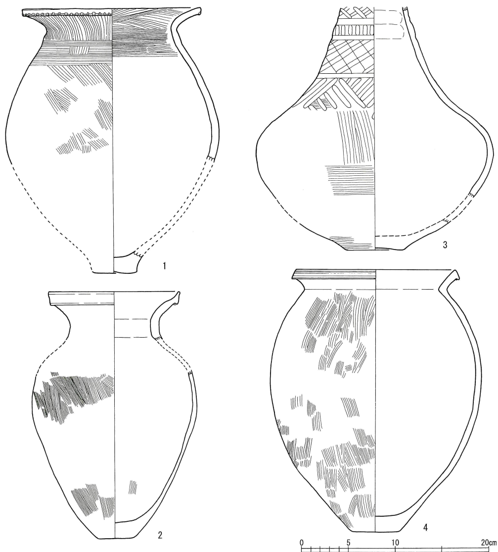
第96 図 溝出土土器実測図3(縮尺1/4)
