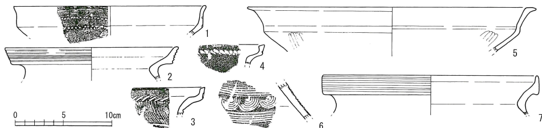
第83図 土壙出土土器実測図8（縮尺1/4）
