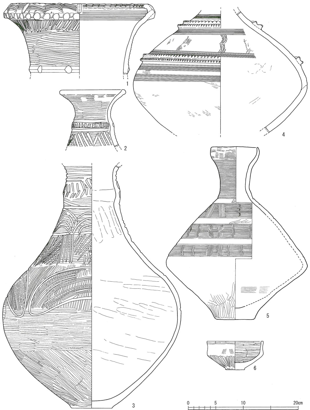
第94図 溝出土土器実測図1(縮尺1/4)
