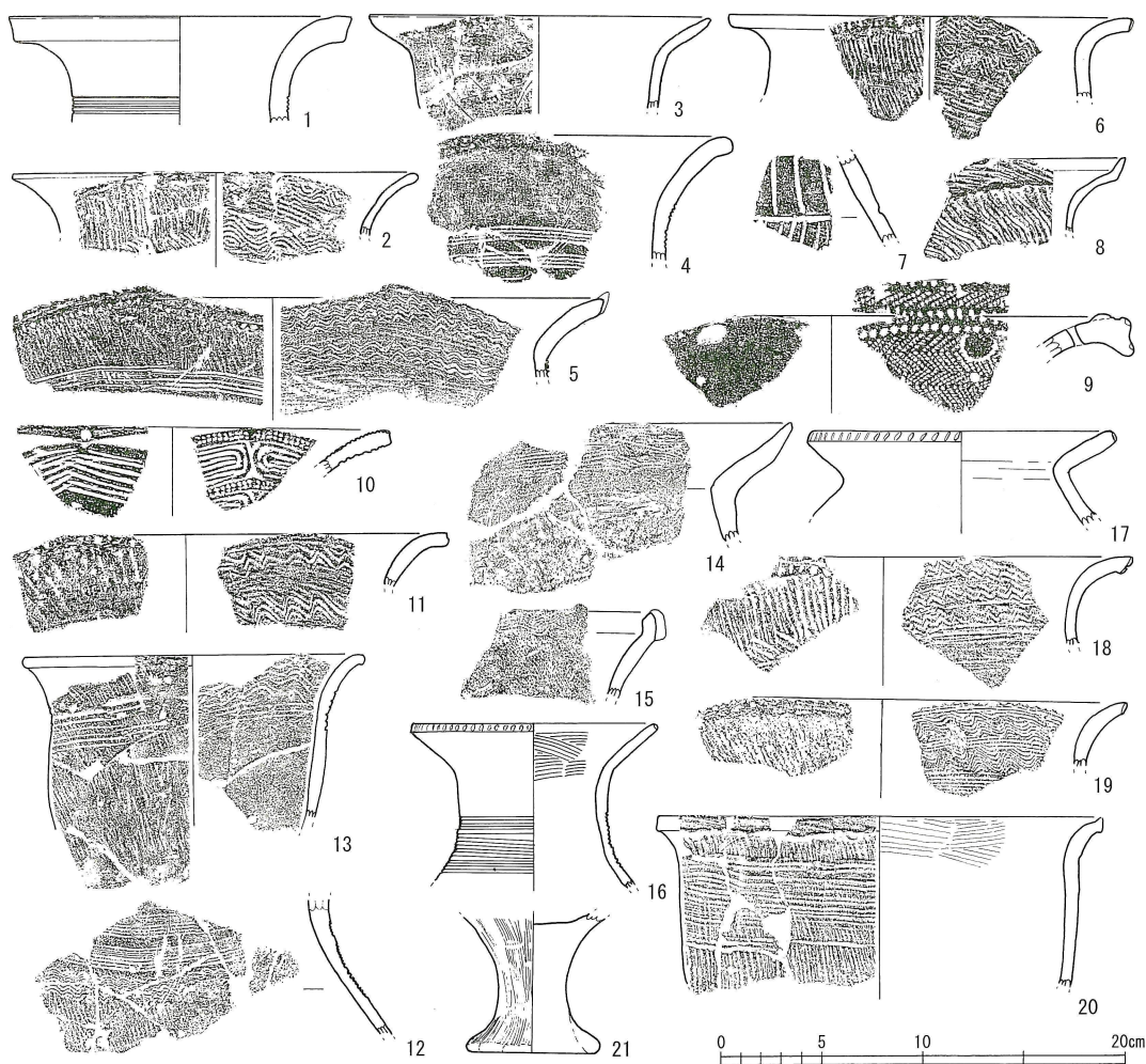
第92図 土壌出土土器実測図16(縮尺1/4)
