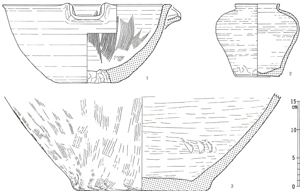
第88図 坂ノ下中世墓群出土蔵骨器実測図②（壺その他）（縮尺1/4）
