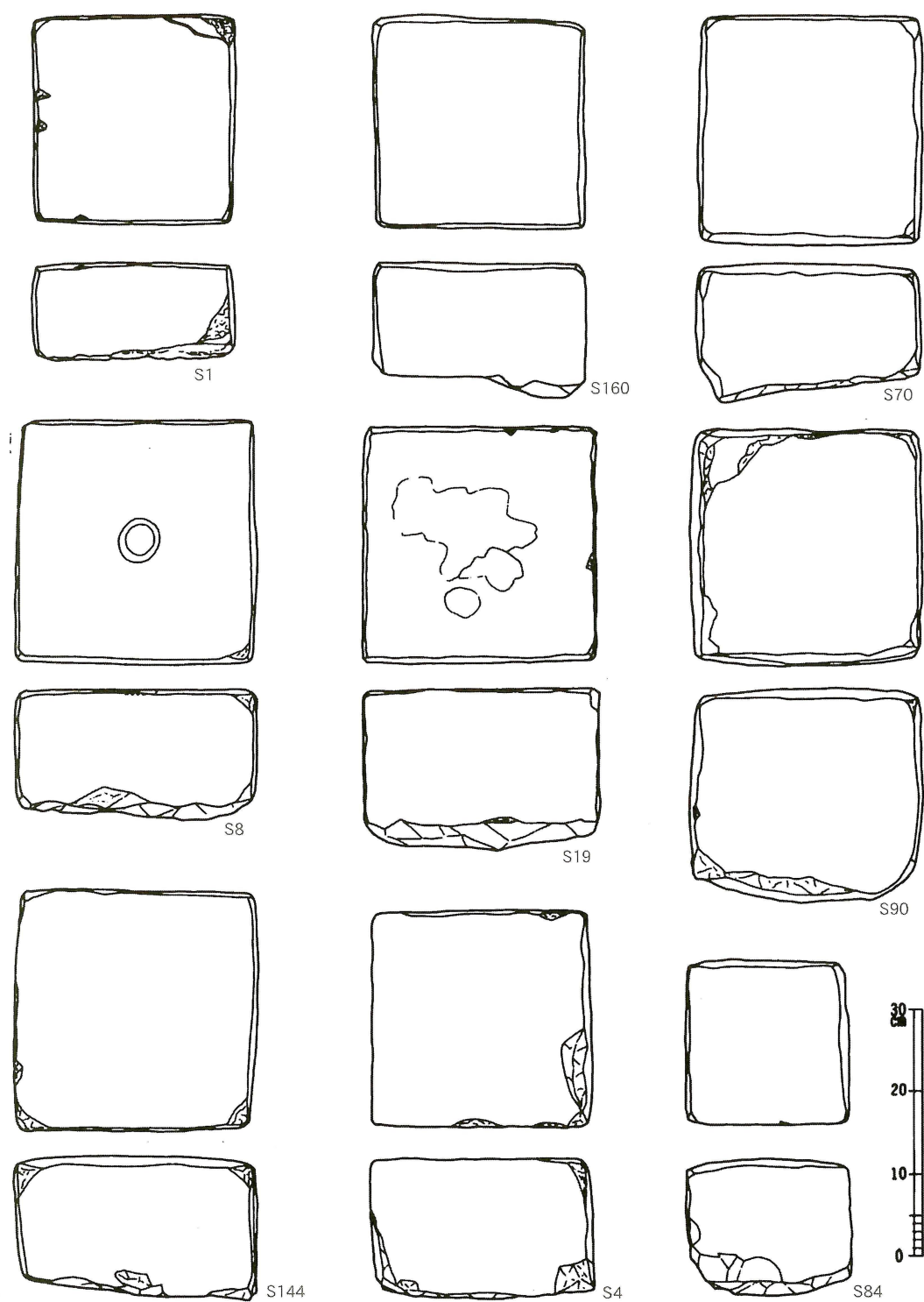
第109図 坂ノ下中世墓群出土地輪実測図④ (縮尺1/8)
