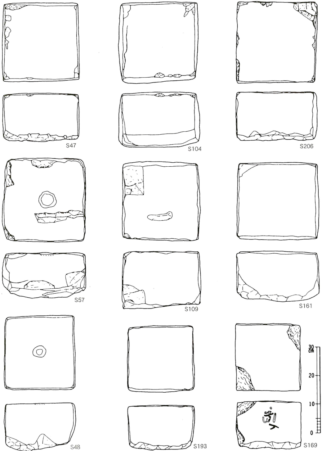
第107図 坂ノ下中世墓群出土地輪実測図② (縮尺1/8)
