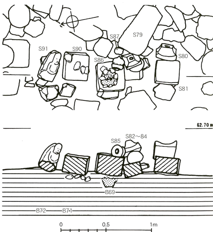
第76図 坂ノ下中世墓D群40・41・42・43・44号墓 実測図 (縮尺1/25)
