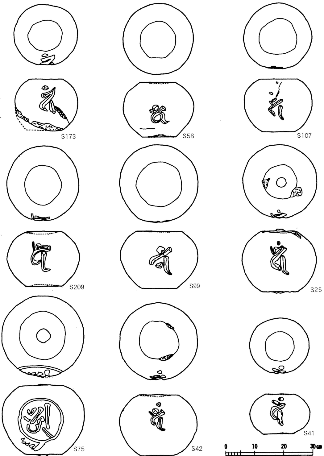
第103図 坂ノ下中世墓群出土水輪実測図① (縮尺1/8)
