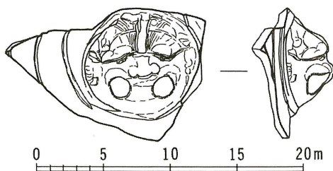
第93図 坂ノ下中世墓群出土土製品実測図（縮尺1/4）
