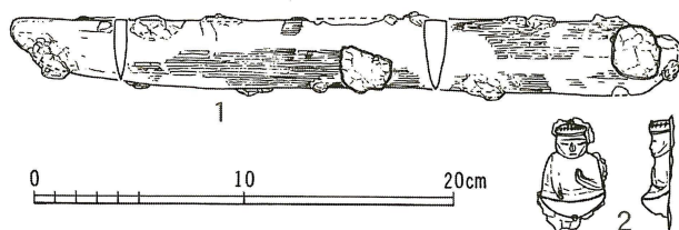
第96図 坂ノ下中世墓群出土短刀・拵（部分）実測図（縮尺1/4）
