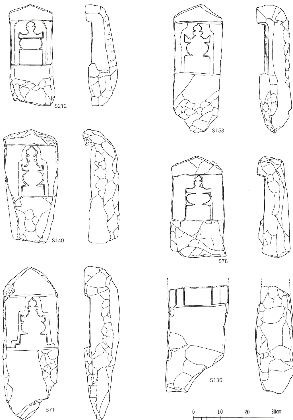
第118図 坂ノ下中世墓群出土板碑実測図⑥ (縮尺1/8)
