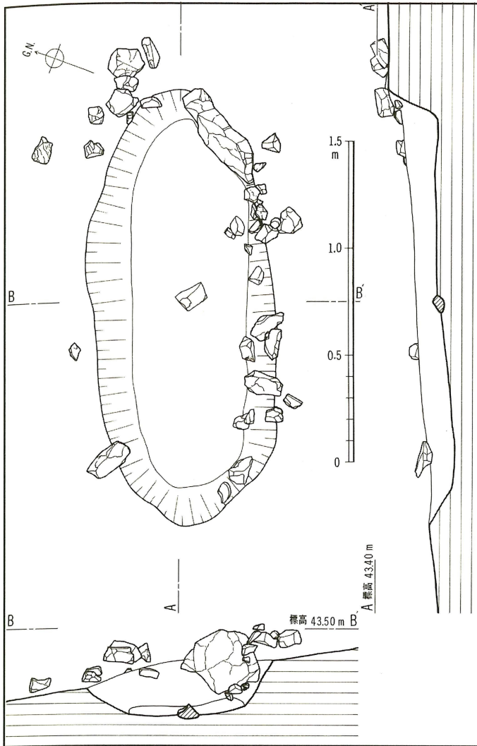
第31図 明神山18号墳墓壙実測図（縮尺1/25）
