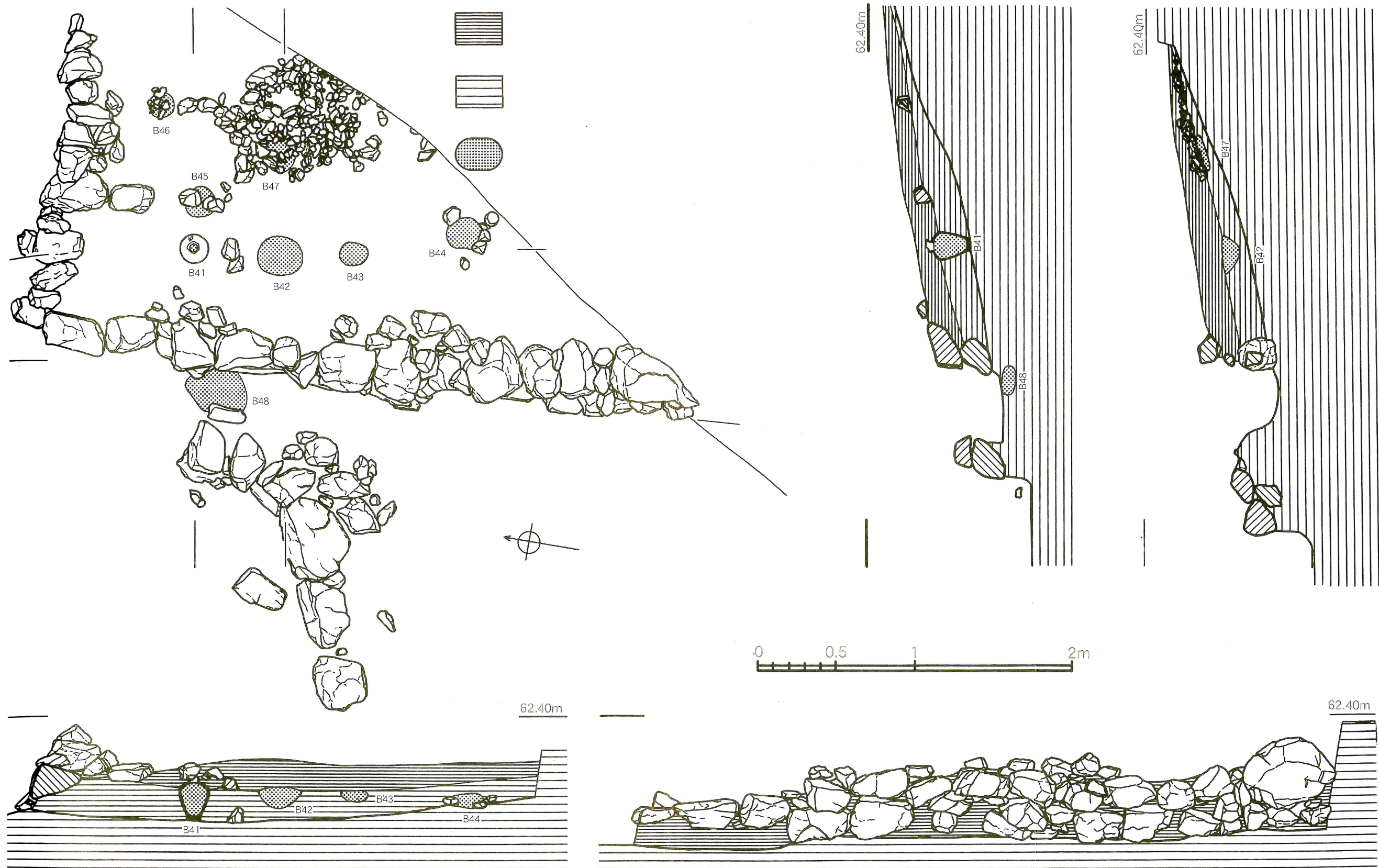
第70図 坂ノ下中世墓D群26号墓実測図（縮尺1/25）
