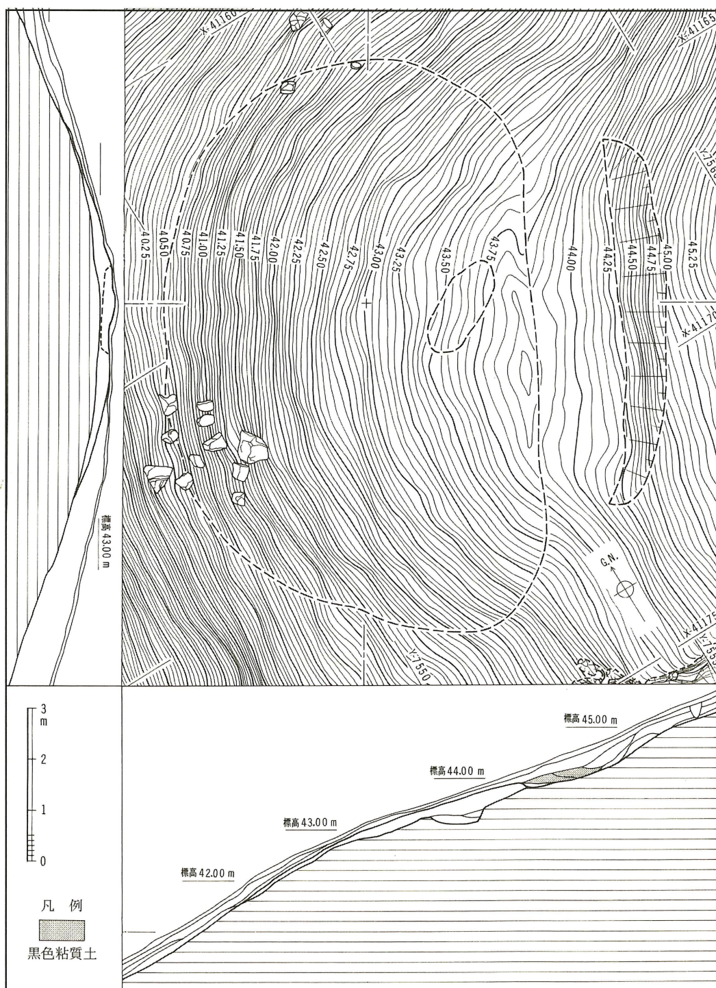
第30図 明神山18号墳墳丘測量図（縮尺1/100）
