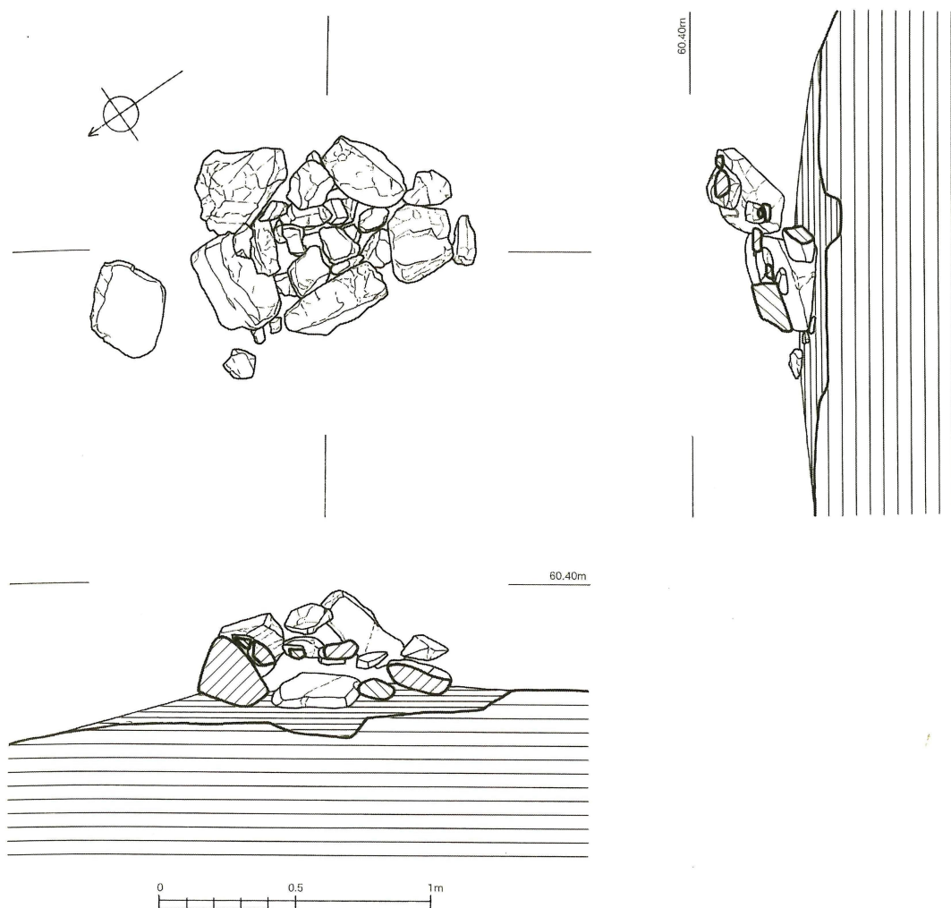
第40図 坂ノ下中世墓群2号経塚（縮尺1/25）
