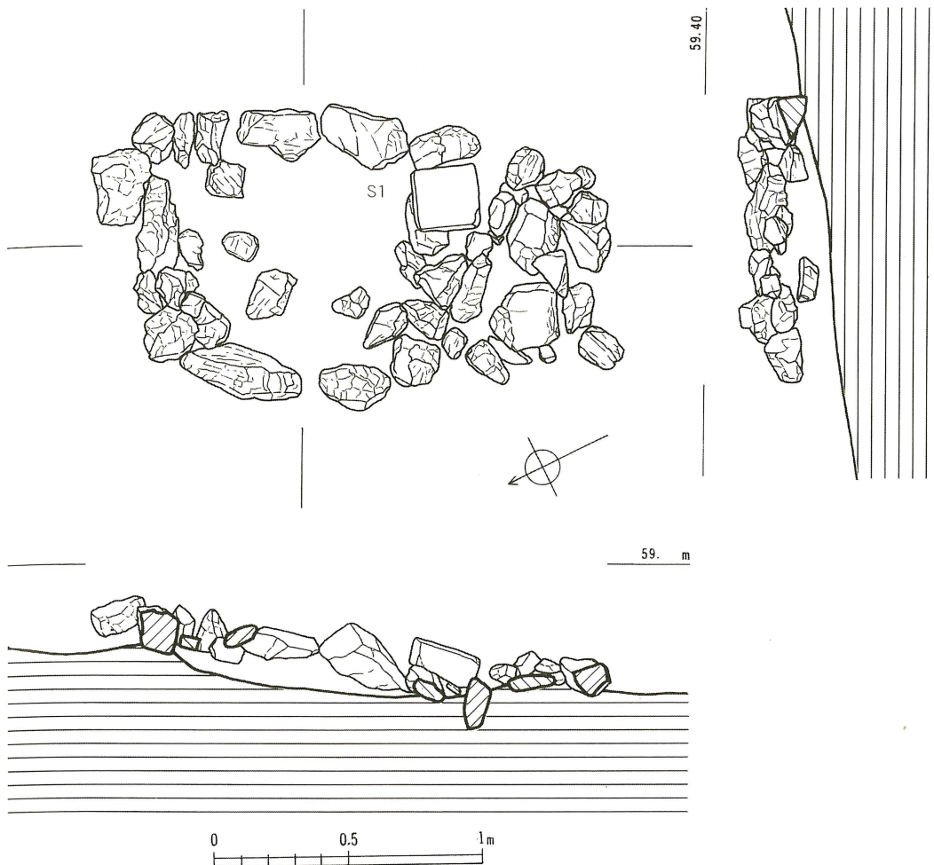
第46図 坂ノ下中世墓A群1号墓実測図（縮尺1/25）
