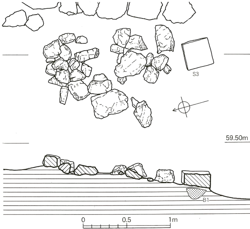
第47図 坂ノ下中世墓A群2号墓実測図（縮尺1/25）
