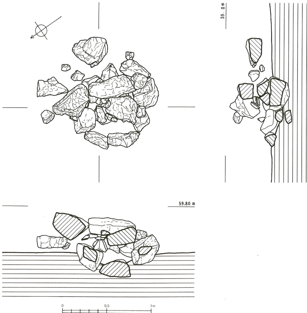
第39図 坂ノ下中世墓群1号経塚 (縮尺1/25)
