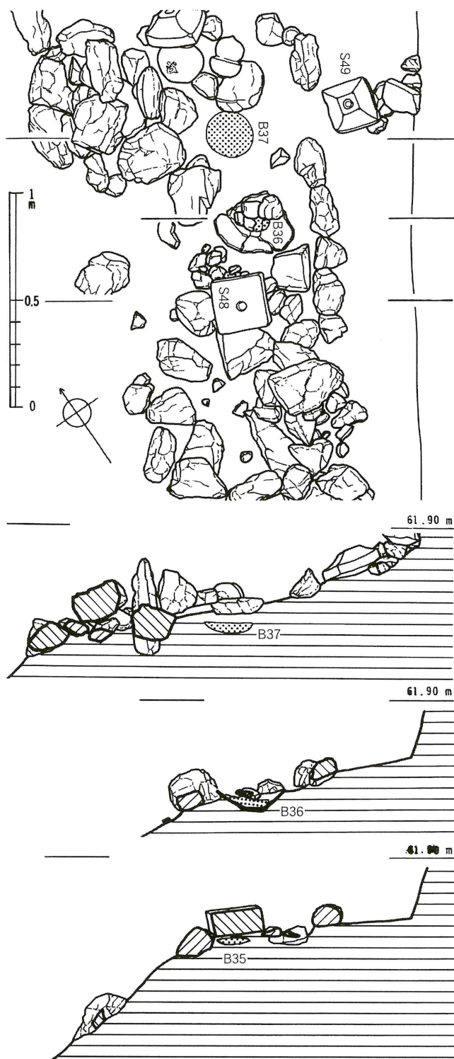
第68図 坂ノ下中世墓C群24号墓実測図（縮尺1/25）
