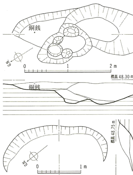
第32図 丑寅山遺跡1号土塋実測図（上）・ 2号土塋実測図（下）（縮尺1/50）
