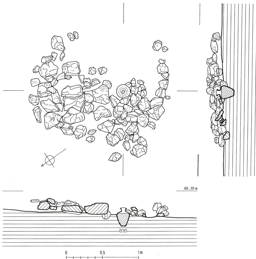
第64図 坂ノ下中世墓B群21号墓実測図（縮尺1/25）
