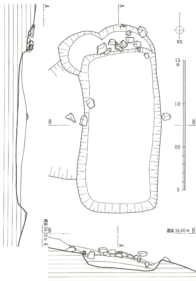
第13図 明神山12号墳墓墳実測図（縮尺1/25）
