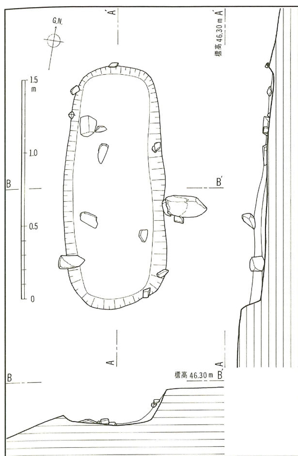
第15図 明神山13号墳墓墳実測図（縮尺1/25）
