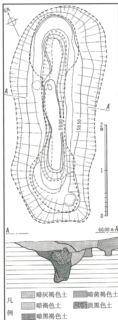
第21図 明神山15号墳墓壙実測図 (縮尺1/50)
