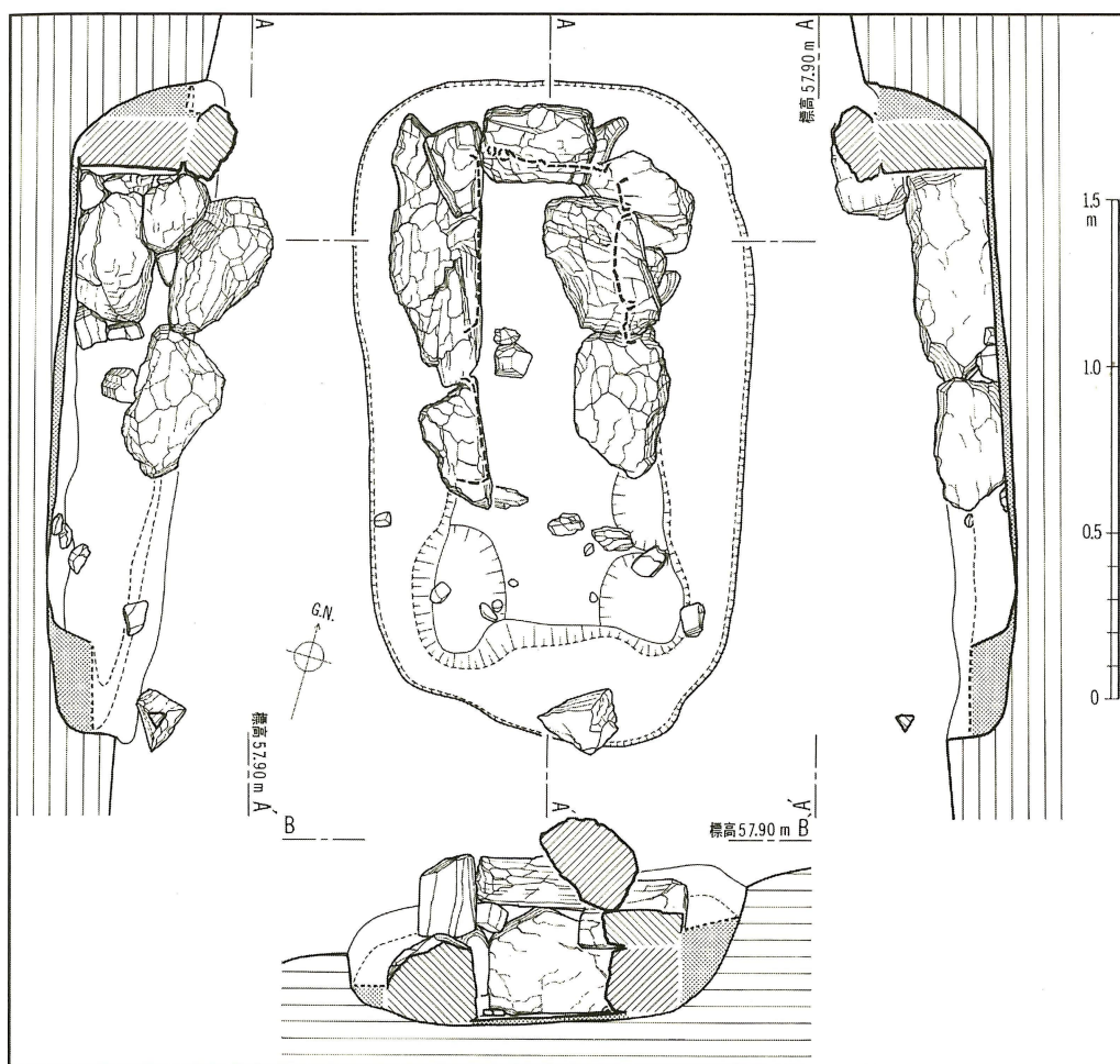
第27図 明神山古墳群縦穴式小石室実測図（縮尺1/25）
