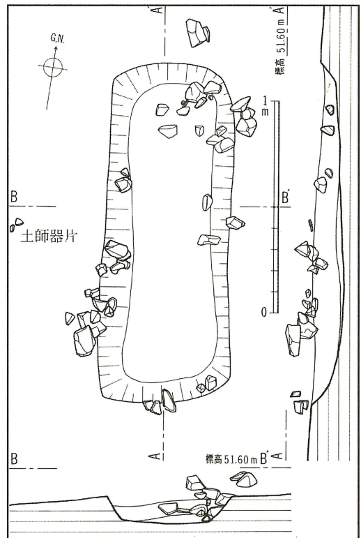
第18図 明神山14号墳墓壙実測図（縮尺1/25）
