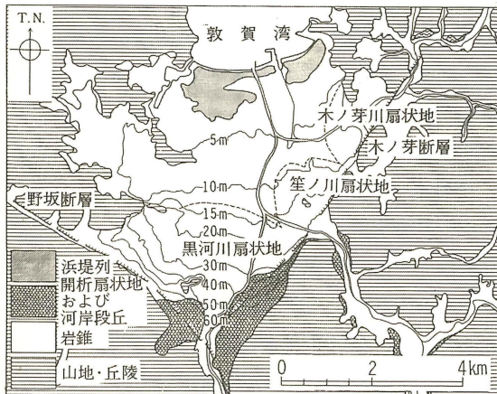
第3図 敦賀平野の地形分類図 (縮尺1/150,000)
