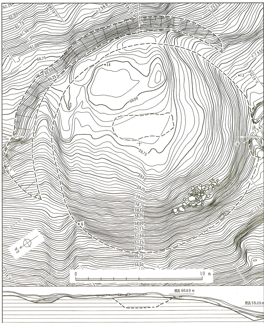
第19図 明神山15号墳墳丘測量図（縮尺1/150）
