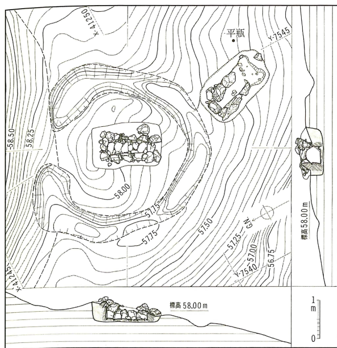
第24図 明神山17号墳墳丘・竪穴式小石室等 測量図（縮尺1/100）
