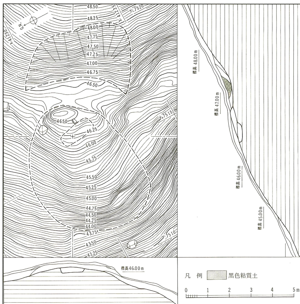
第14図 明神山13号墳墳丘測量図（縮尺1/100）
