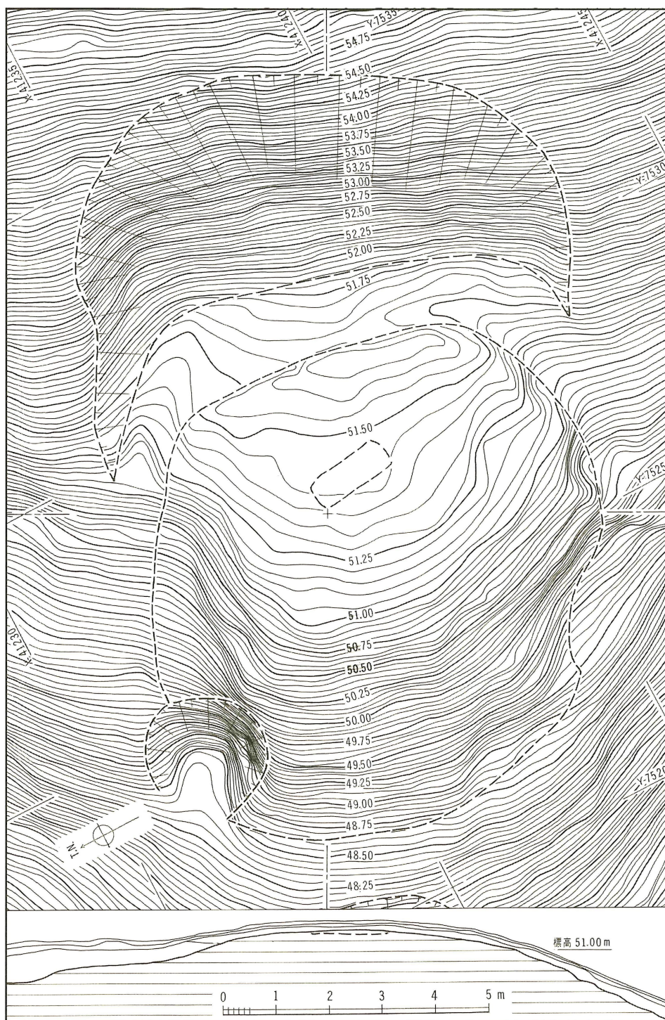
第16図 明神山14号墳墳丘測量図 (縮尺1/100)
