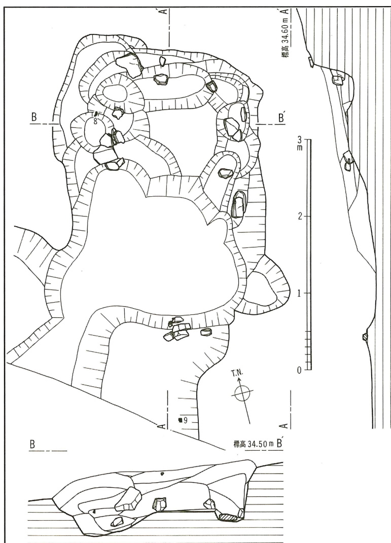
第23図 明神山16号墳横穴式石室墓壙実測図（縮尺1/50）
