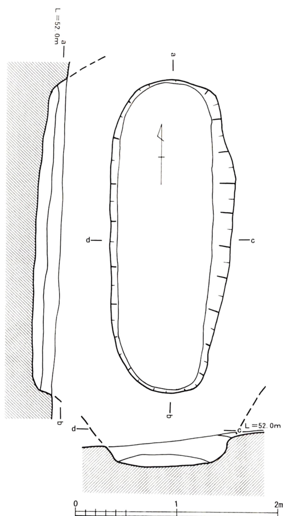
第46図 4号墳埋葬施設実測図
