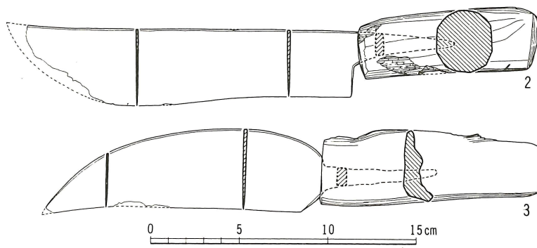
第117図 各土壇出土金属器実測図（縮尺1/3） 庖丁（2・3）
