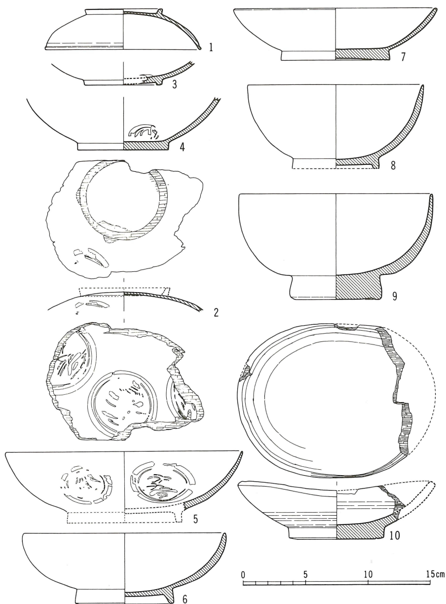
第110図 各土壙出土木器実測図1 (縮尺 1/3) 漆器蓋 (1・2) 同碗 (3～9) 木碗 (10)
