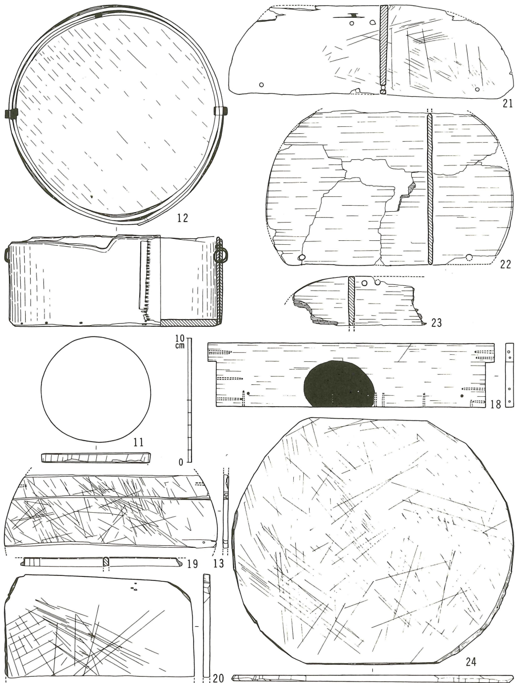
第111図 各土壙出土木器実測図2 (縮尺1/3) 曲物 (11～13) 箱 (18) 折敷 (19～21) 不明板材 (22～24)
