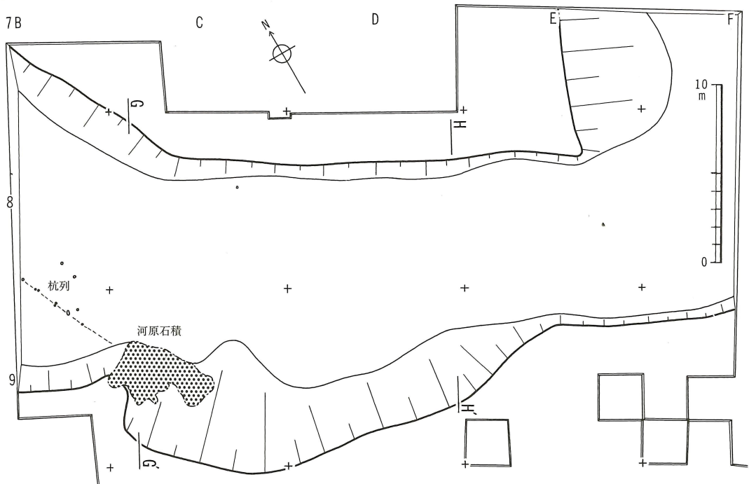
第22図 河道実測図（縮尺1/300）
