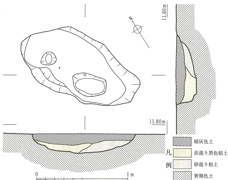
第14図 3号遺構実測図（縮尺 1/25）
