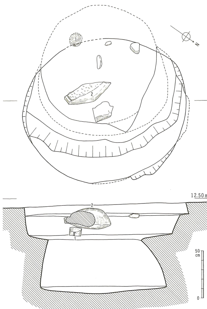
第51図 16号土壙実測図（縮尺1/25）
