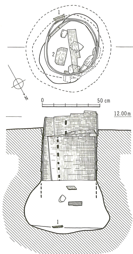
第43図 9号土壙実測図(縮尺1/20)
