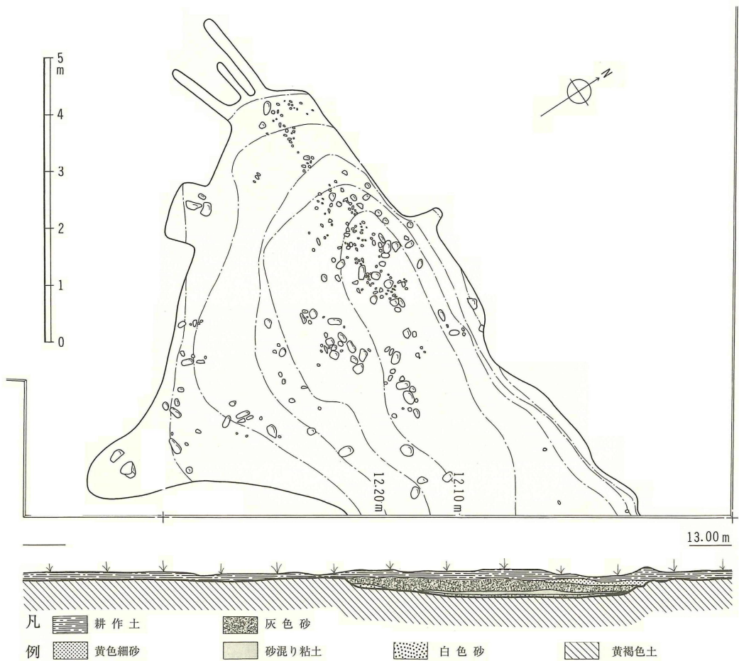
第 27 図 窪地実測図
