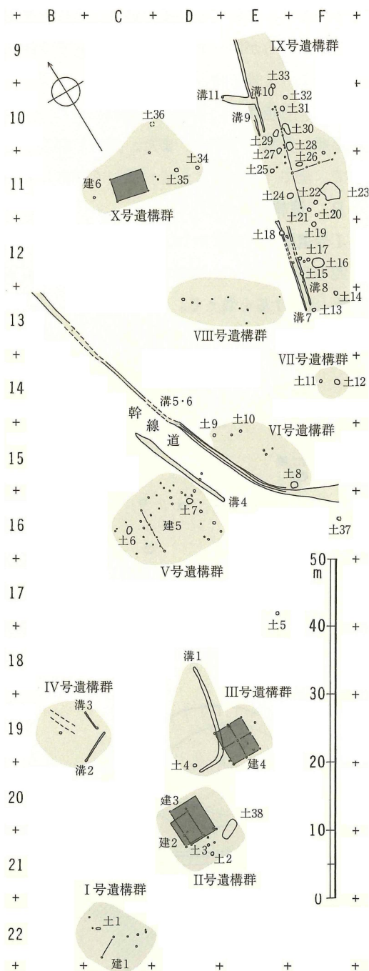
第29図 室町時代遺構分布図 (縮尺 1/800)
