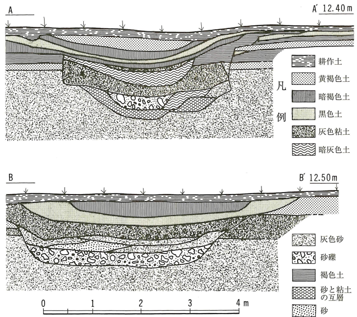
第21図 大溝断面実測図（縮尺1/75）
