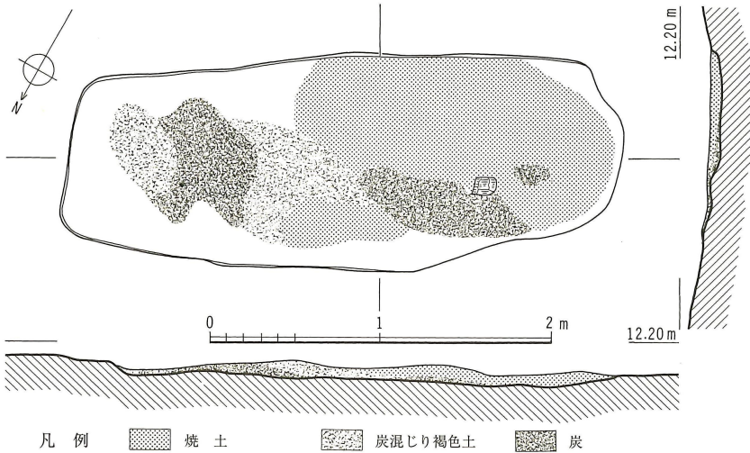
第34図 38号土壙実測図（縮尺1/40）
