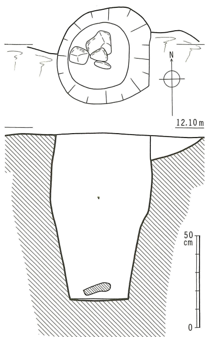
第 48 図 13 号土壙実測図（縮尺 1/20）
