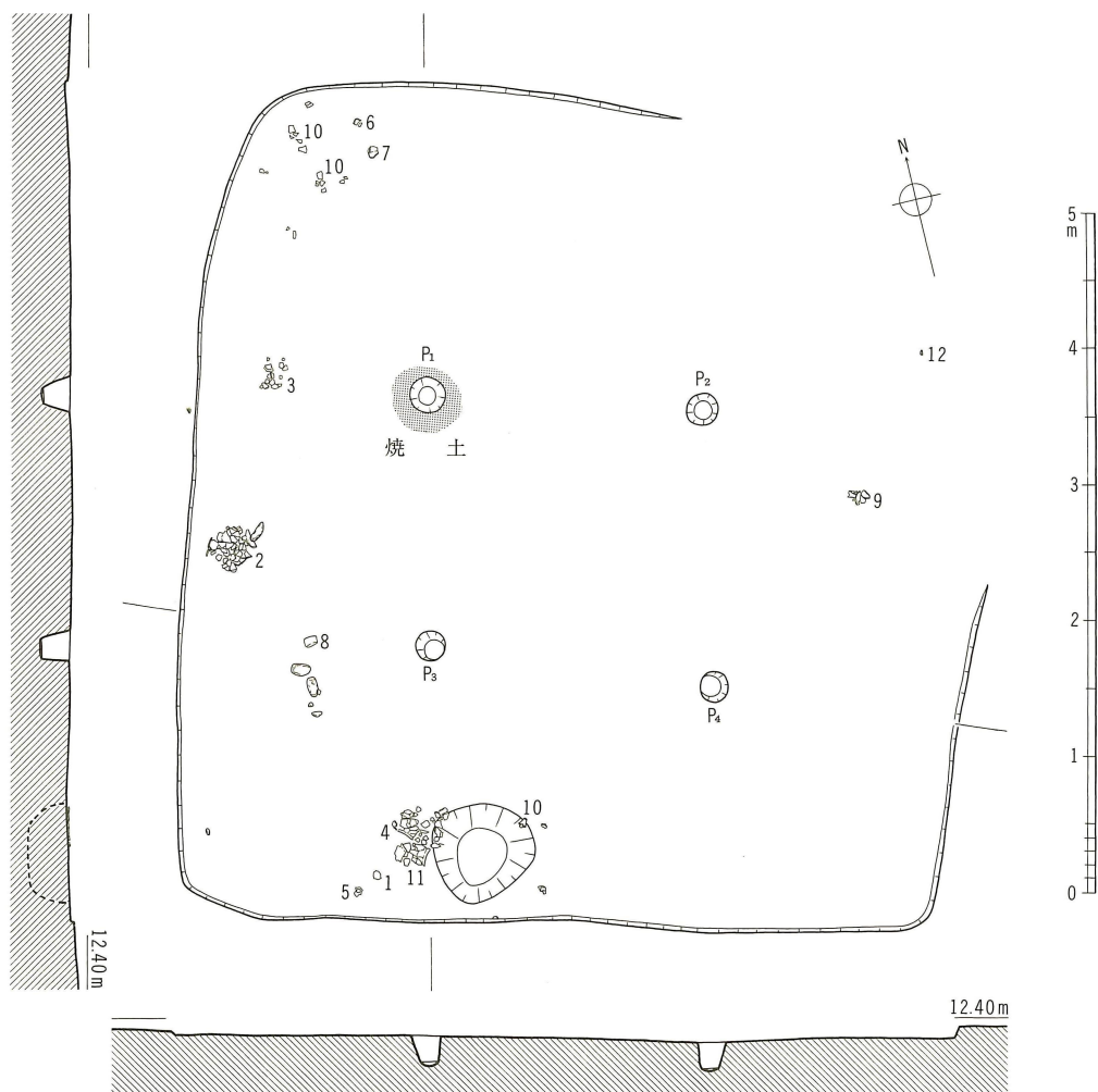
第18図 竪穴住居実測図（縮尺 1/60）
