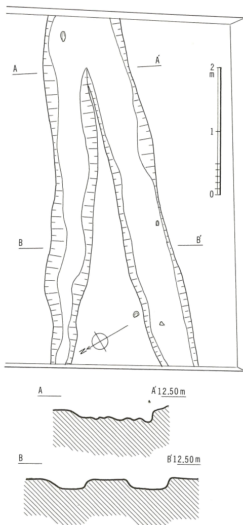
第28図 1・2号溝実測図（縮尺1/60）
