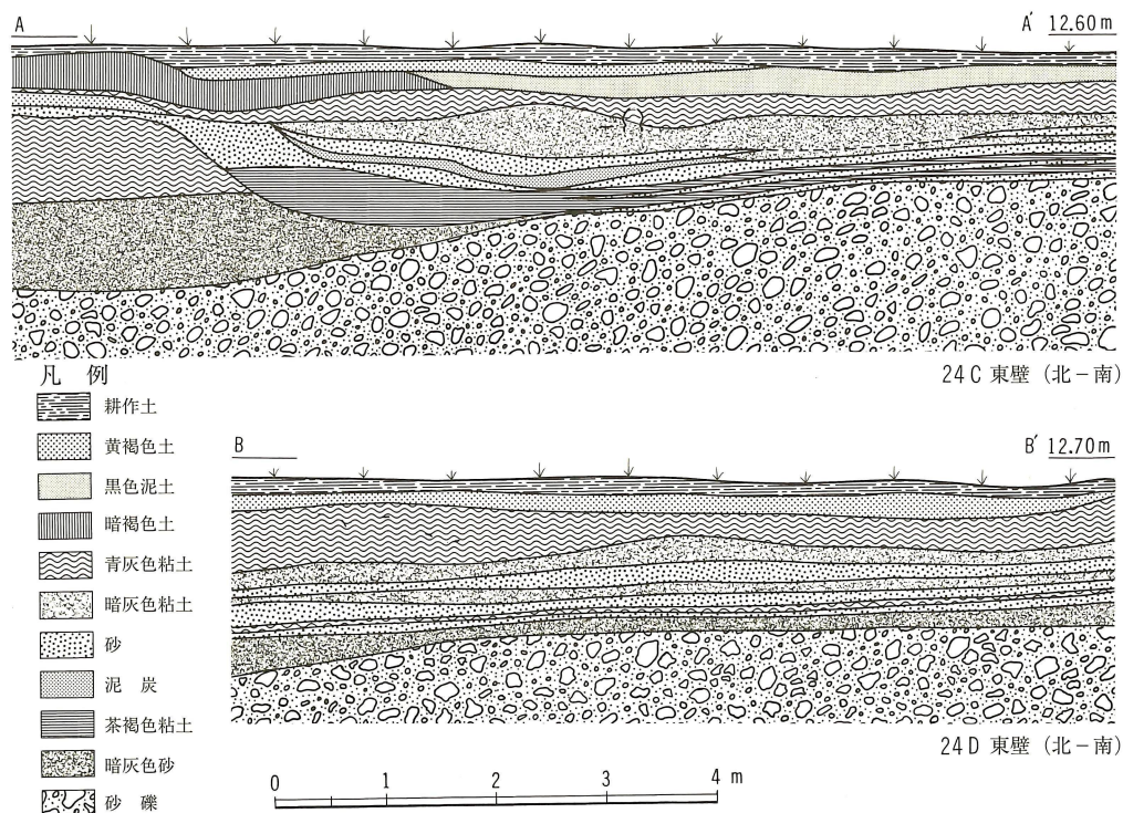
第26図 低湿地断面実測図 (縮尺 1/75)
