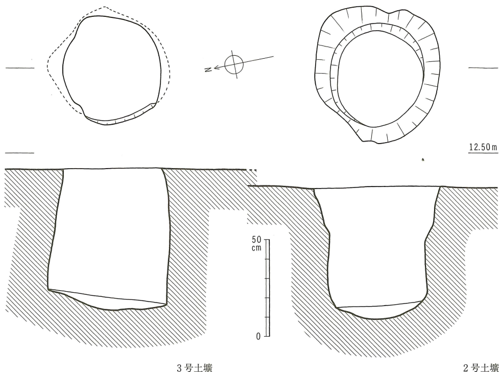
第33図 2・3号土塋実測図（縮尺 1/20）
