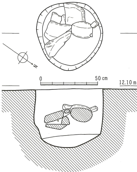
第 52 図 17 号土坑実測図 (縮尺 1/20)
