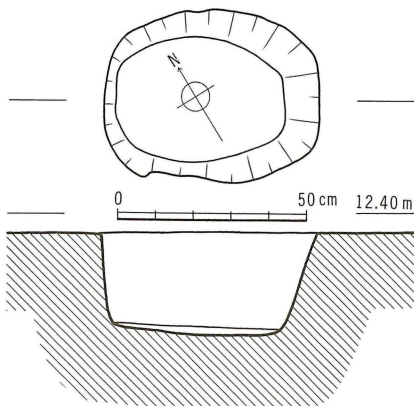
第31図 Ⅰ号土塋実測図（縮尺1/20）
