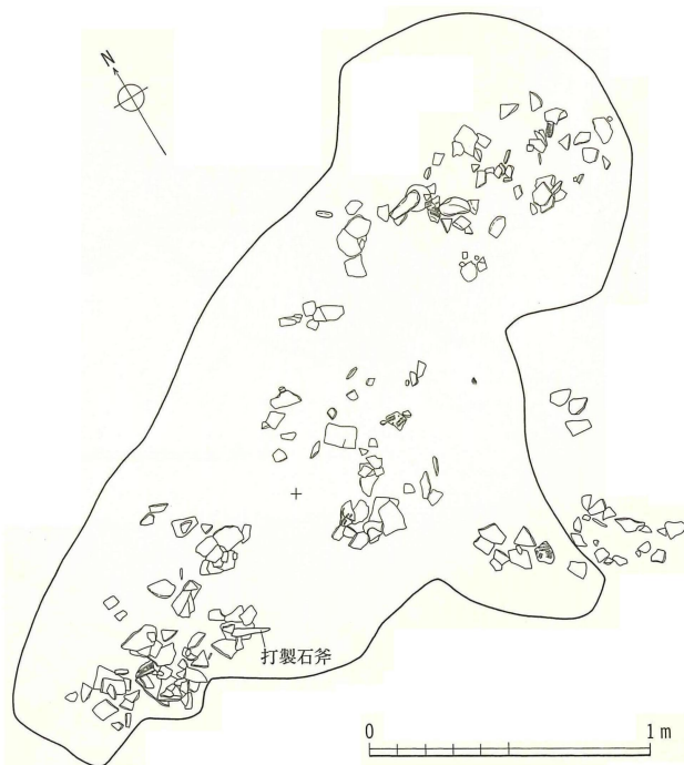
第10図 1号遺構上面遺物出土状態実測図(縮尺 1/30)
