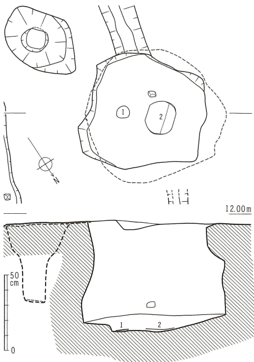
第 53 図 18 号土坑実測図 (縮尺 1/25)
