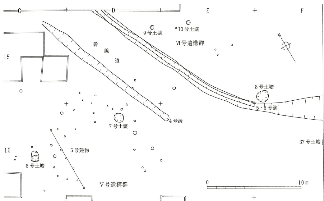
第 39 図 V・VI号遺構群実測図 (縮尺 1/250)
