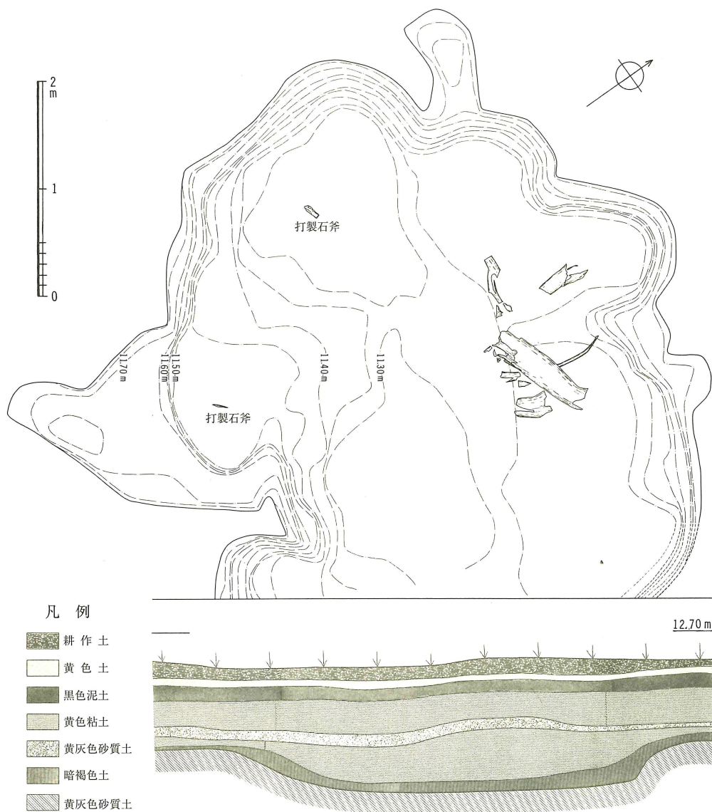
第16図 6号遺構実測図（縮尺1/50）
