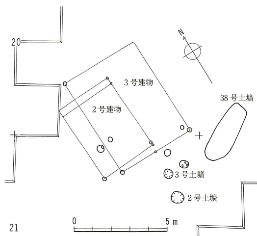
第32図 Ⅱ号遺構群実測図（縮尺 1/200）
