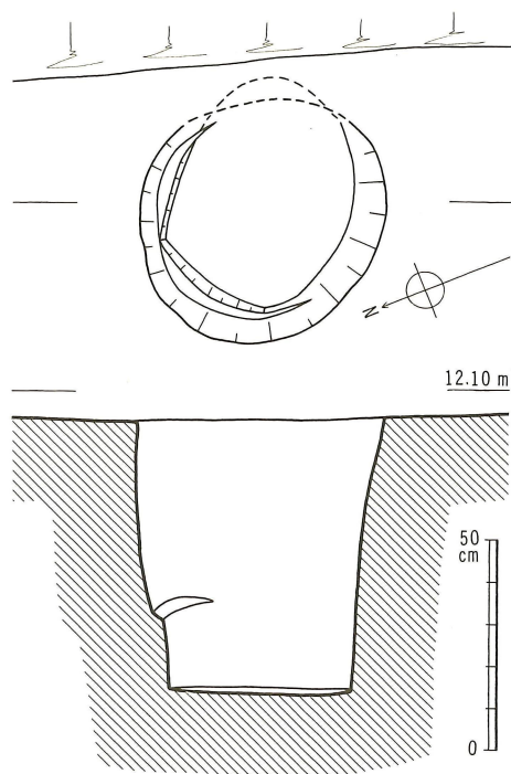
第 49 図 14 号土壙実測図（縮尺 1/20）
