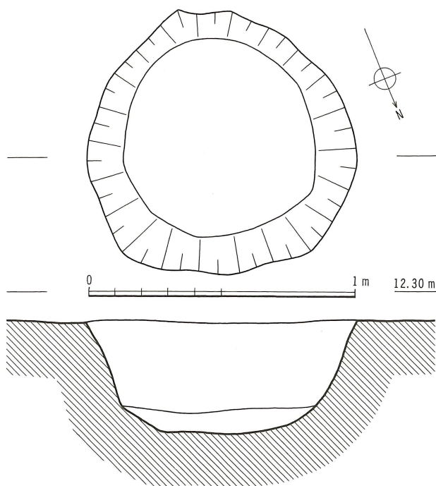
第41図 7号土壌実測図（縮尺1/20）
