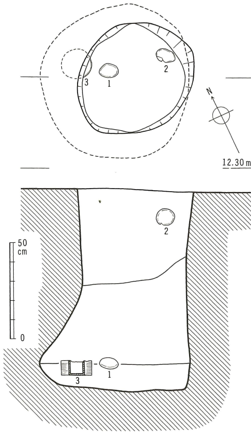
第 46 図 11 号土壙実測図 (縮尺 1/20)
