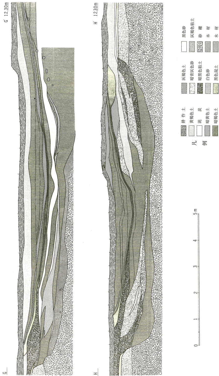
第23图 河道断面实测图 (縮尺 1/70)
