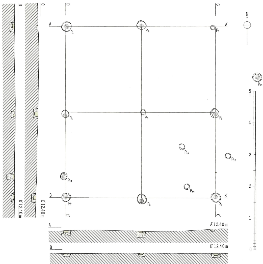
第36図 4号掘立柱建物実測図（縮尺1/60）
