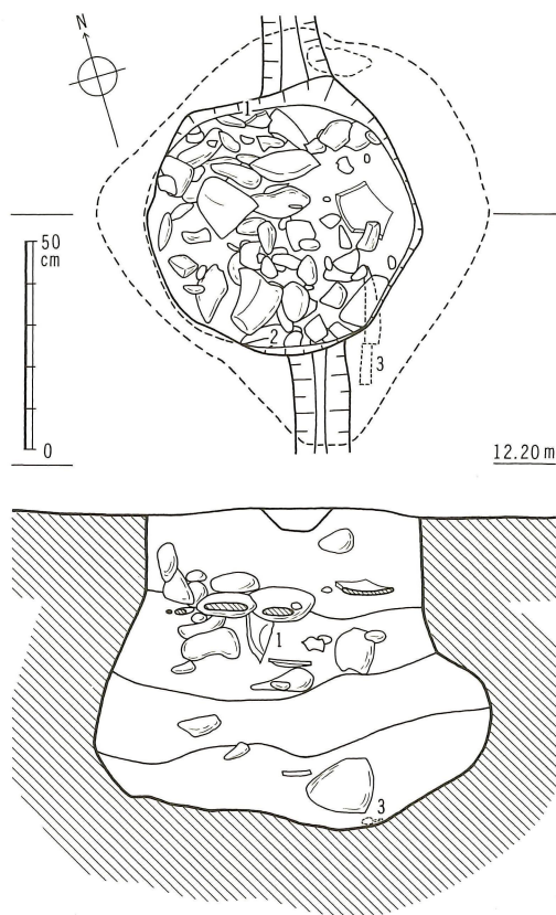
第 50 図 15 号土壙実測図（縮尺 1/20）
