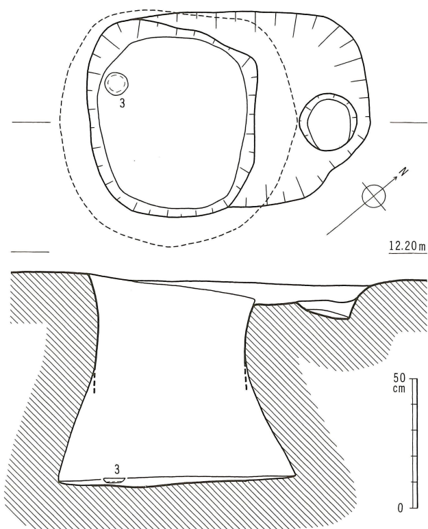
第 40 図 6号土壙実測図 (縮尺 1/20)
