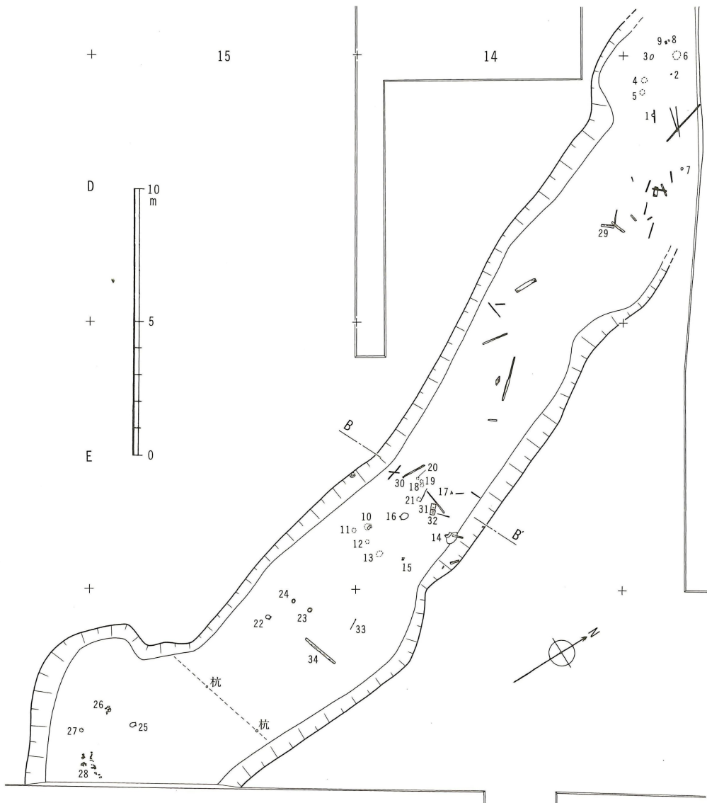
第20図 大溝南部実測図 (縮尺 1/200)
