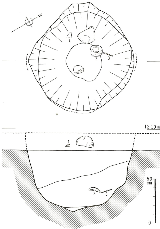
第 42 図 8 号土壙実測図（縮尺 1/25）
