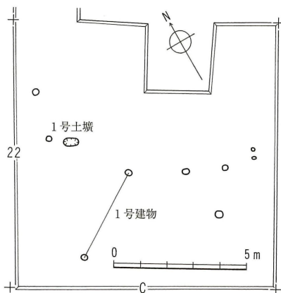
第30図 Ⅰ号遺構群実測図（縮尺1/200）
