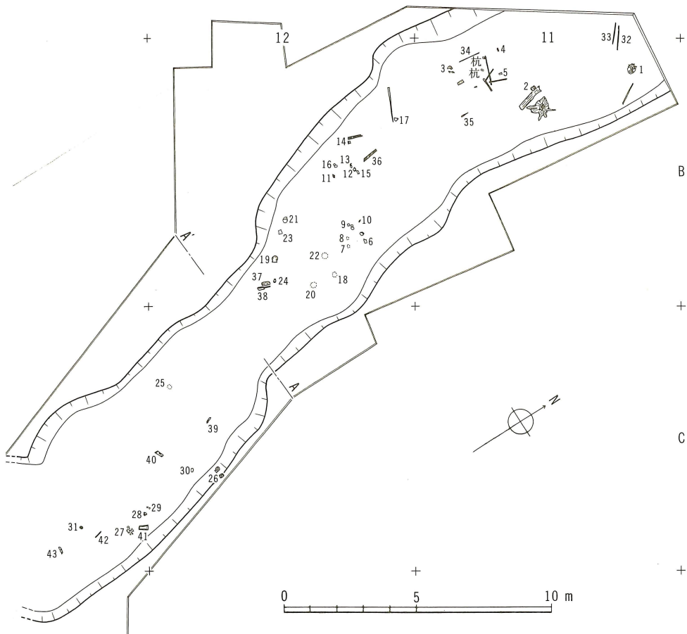
第19図 大溝北部実測図 (縮尺 1/200)
