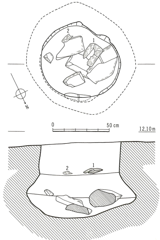
第 54 図 19 号土坑実測図 (縮尺 1/20)
