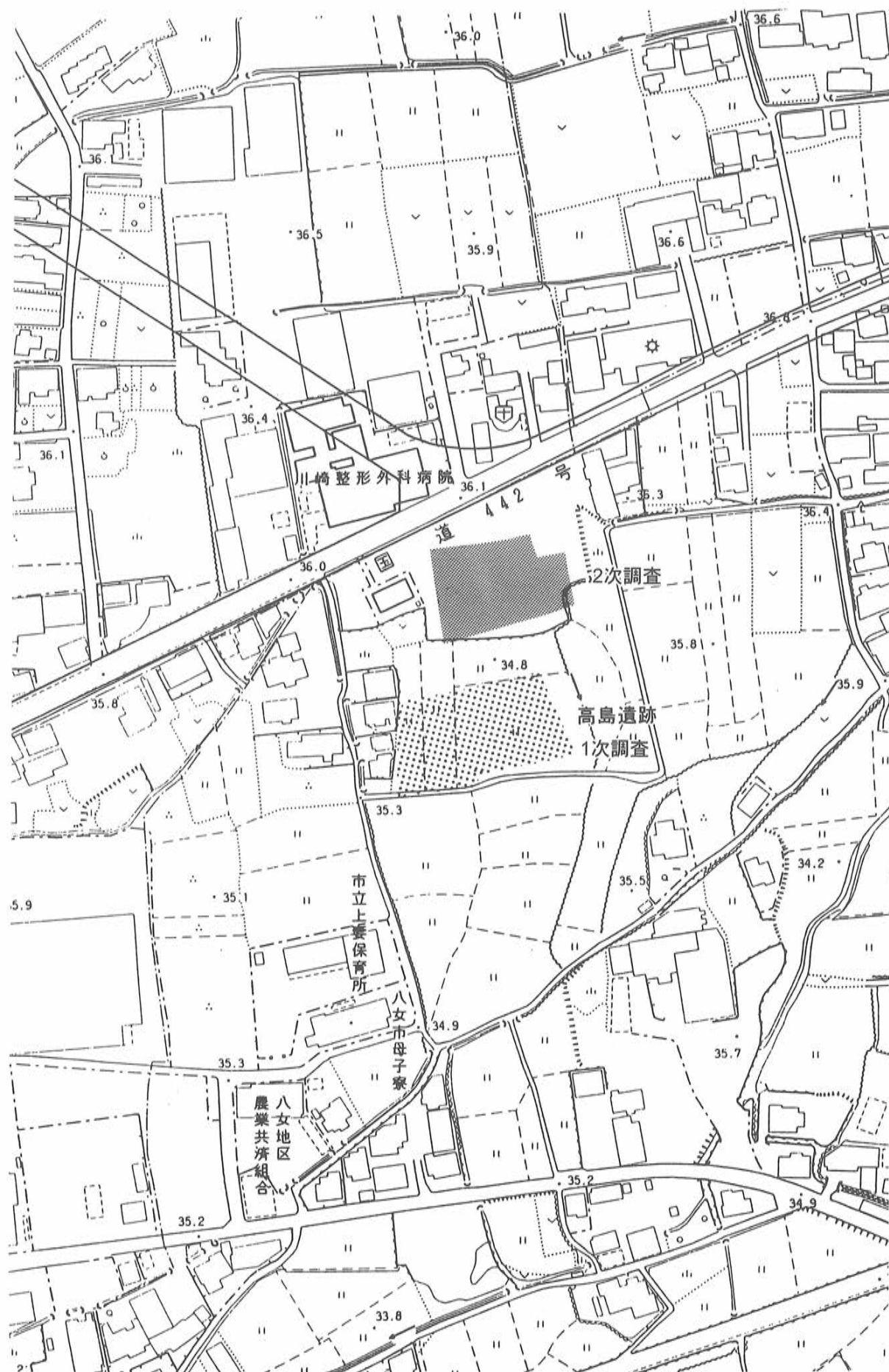
第2図 高島遺跡（2次調査）位置図〔1/2,500〕
