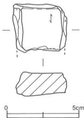
第37図 SK-17出土砥石実測図〔2/3〕
