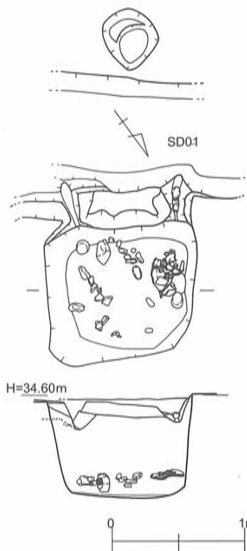
第34図 SK-39遺構実測図〔1/40〕
