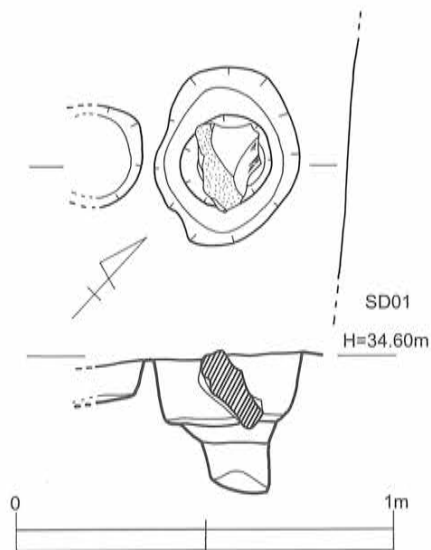
第40図 SP-02 遺構実測図〔1/20〕
