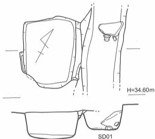
第17図 SK-04遺構実測図 [1/40]
