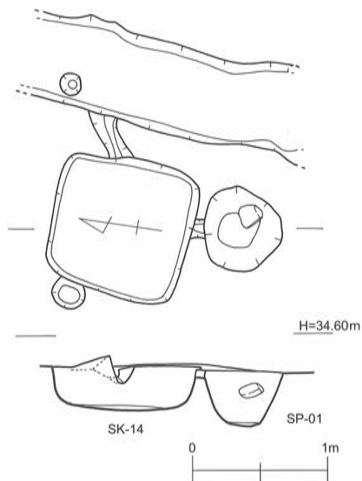
第27図 SK-14・SP-01遺構実測図〔1/40〕
