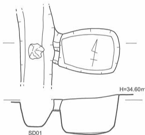
第20図 SK-07遺構実測図〔1/40〕
