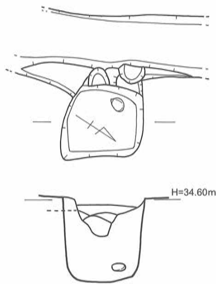
第30図 SK-16遺構実測図〔1/40〕
