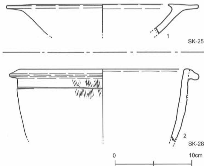
第38図 その他の土壙 (SK) 出土土器実測図 [1/3]
