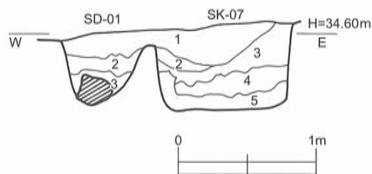
第45図 SK-05・SD-01土層断面図 [1/40]
