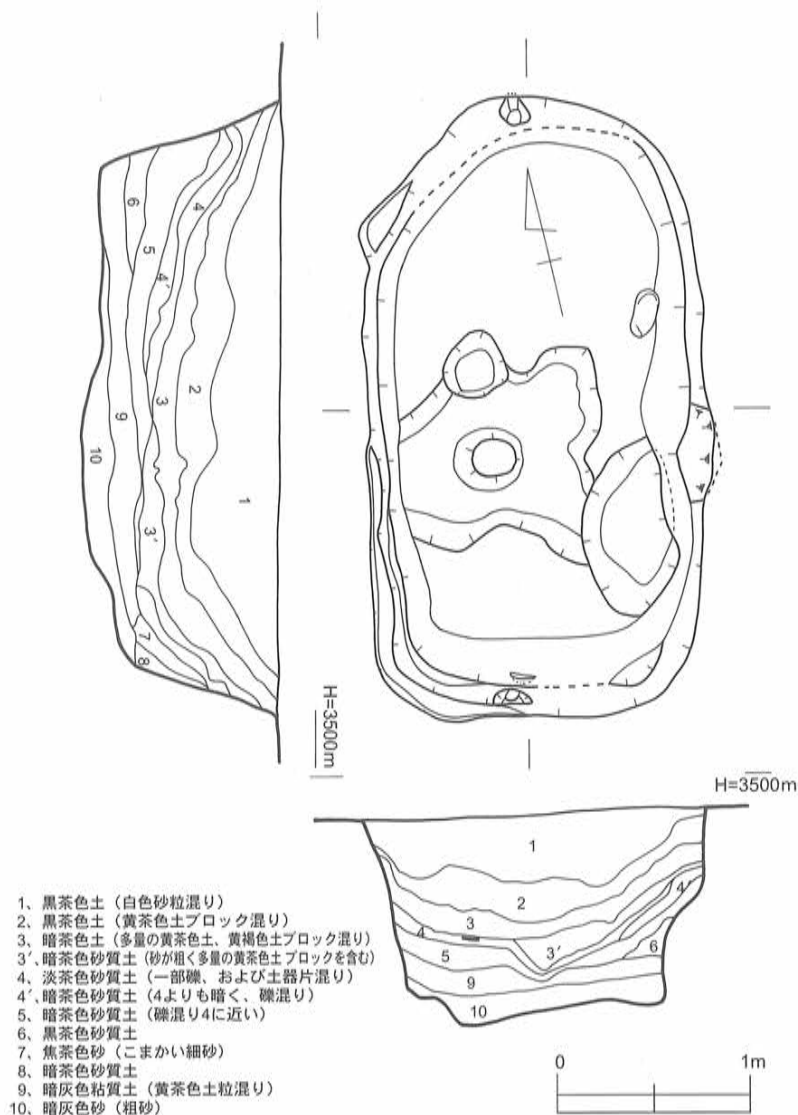
第13図 SK-01 (貯蔵穴状土壌) 遺構実測図 [1/40]
