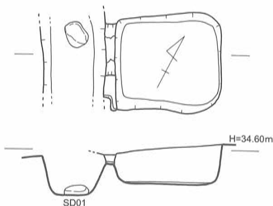
第19図 SK-06遺構実測図〔1/40〕
