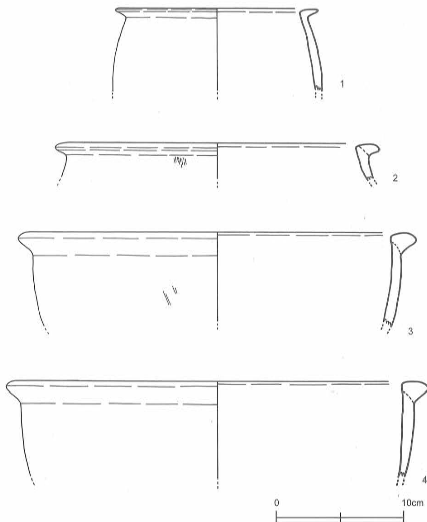
第14図 SK-01（貯蔵穴状土壙）出土土器実測図〔1/3〕
