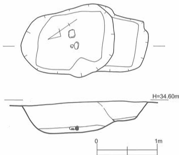
第39図 SK-34遺構実測図〔1/40〕
