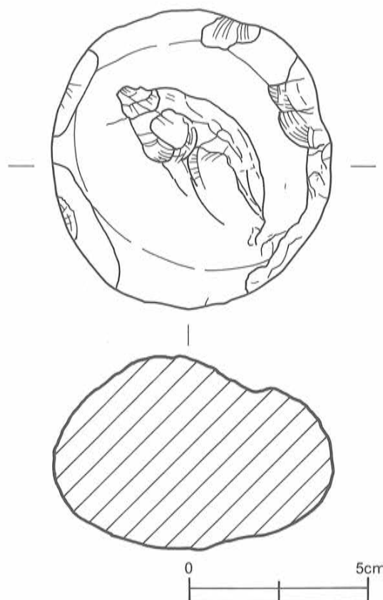
第28図 SK-14出土黒曜石原石実測図〔2/3〕
