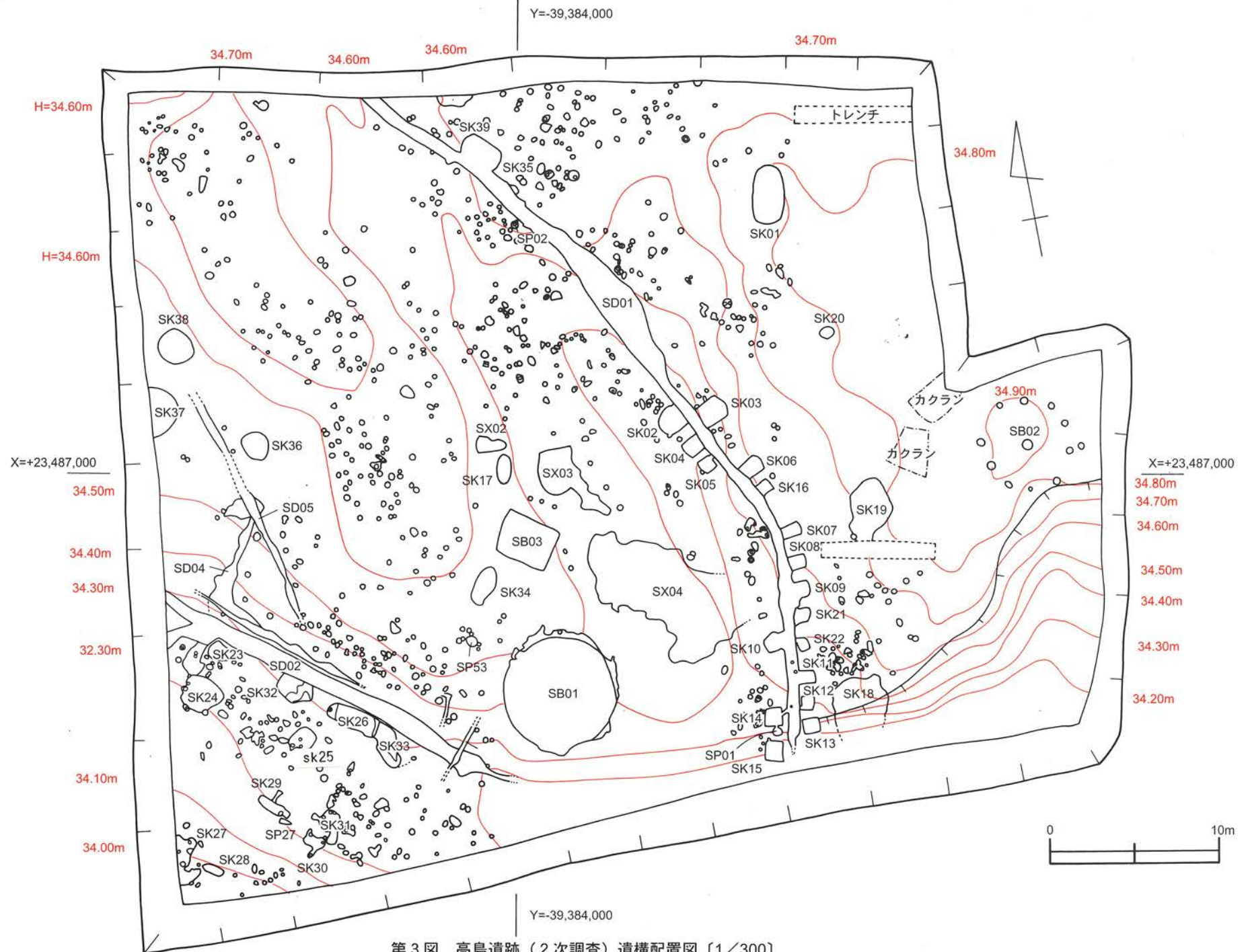
第3図 高島遺跡(2次調査)遺構配置図[1/300]
