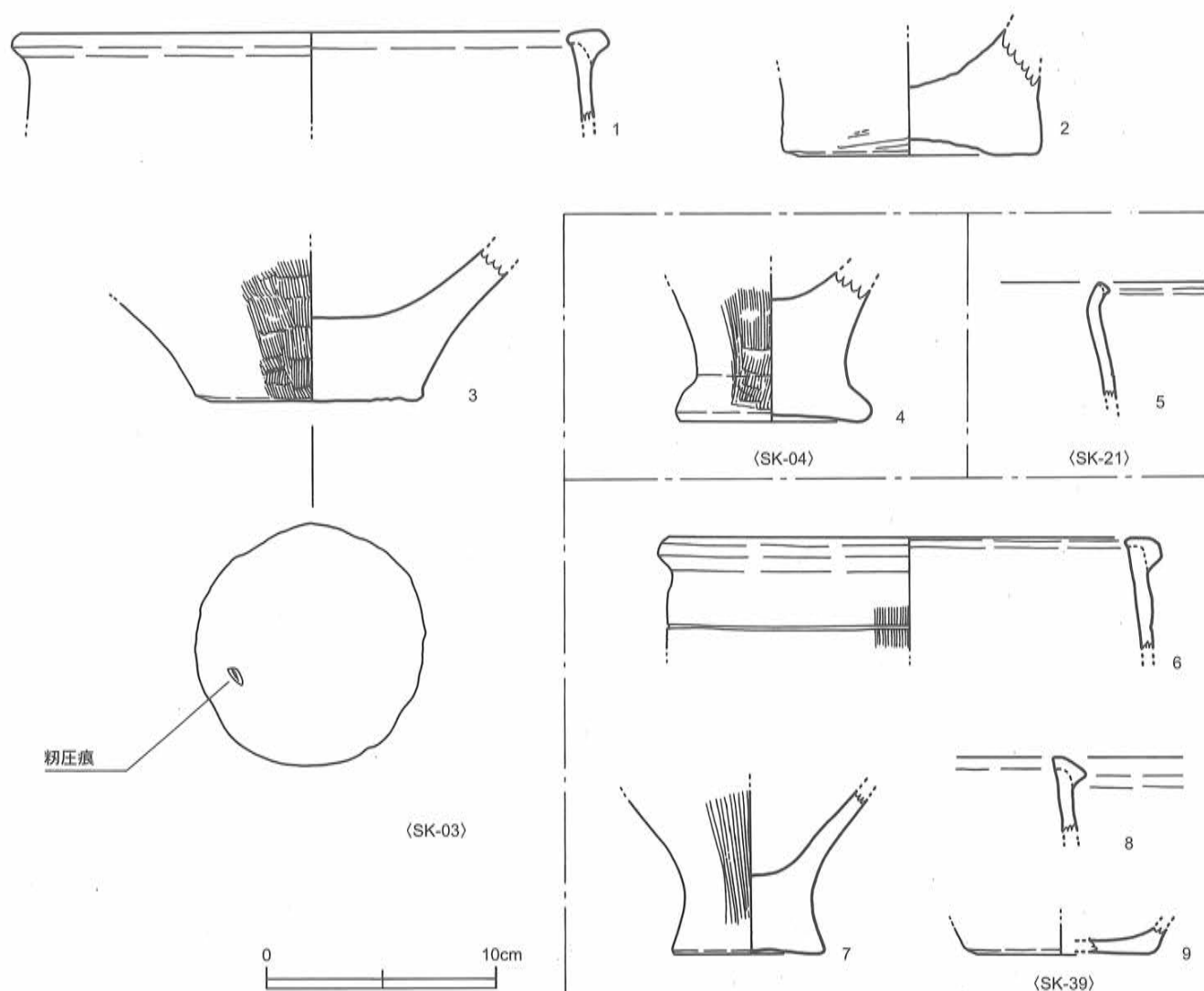
第35図 取水土壙 (SK-03,04,21,39) 出土土器実測図 [1/3]
