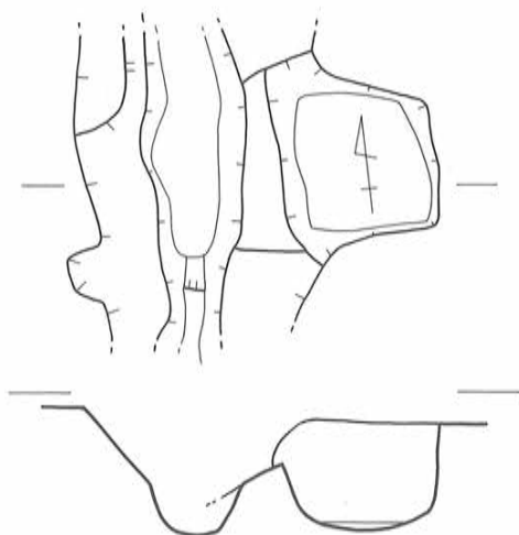
第31図 SK-21遺構実測図〔1/40〕
