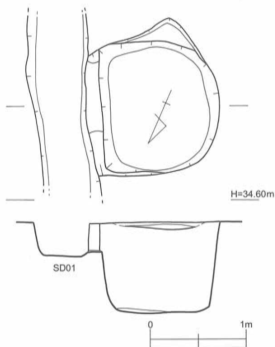
第15図 SK-02遺構実測図〔1/40〕
