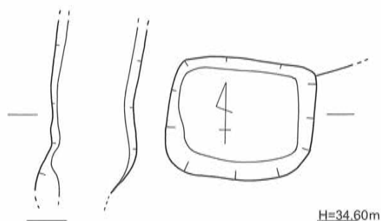
第25図 SK-12遺構実測図〔1/40〕
