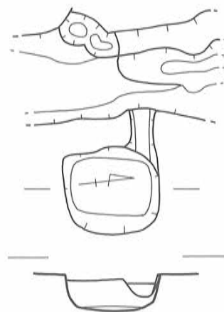
第32図 SK-22遺構実測図〔1/40〕
