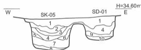
第44図 SK-04・SD-01土層断面図 [1/40]
