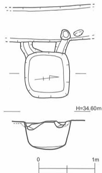
第24図 SK-11遺構実測図〔1/40〕
