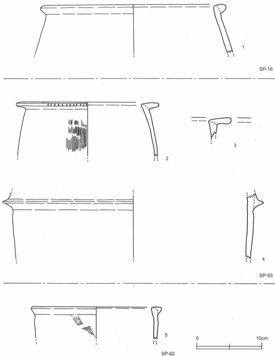
第42図 ピット (SP) 出土土器実測図 [1/3]
