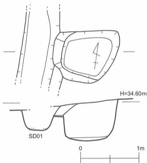
第21図 SK-08遺構実測図〔1/40〕
