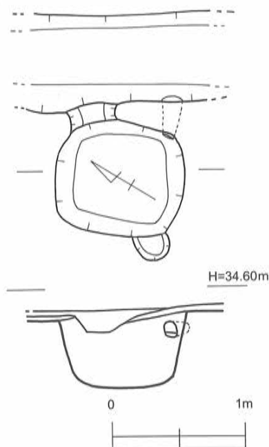
第18図 SK-05遺構実測図 [1/40]
