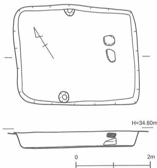
第8図 SB-03遺構実測図〔1/60〕
