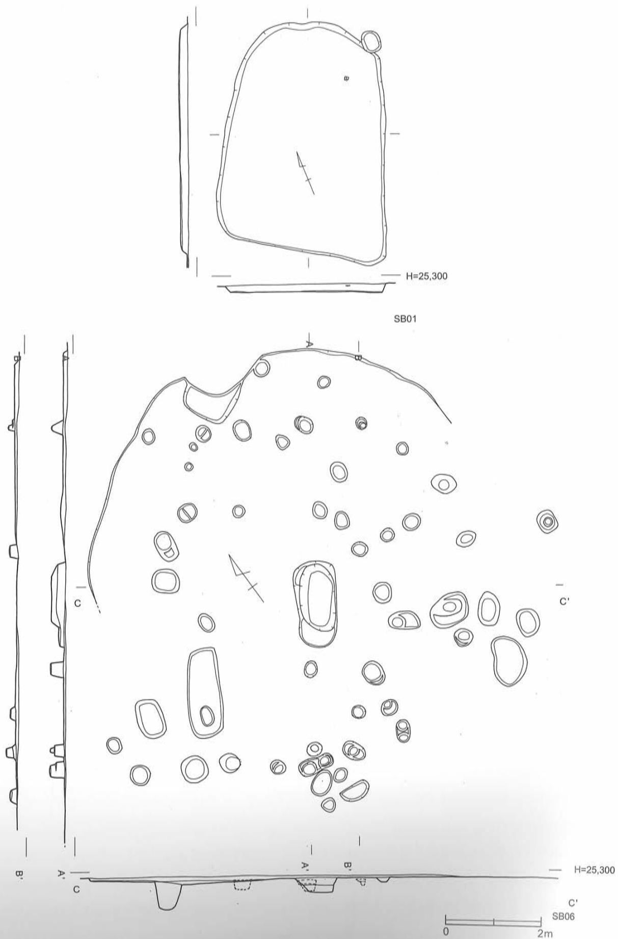
第5図 竖穴住居 (SB01、06) [1/80]
