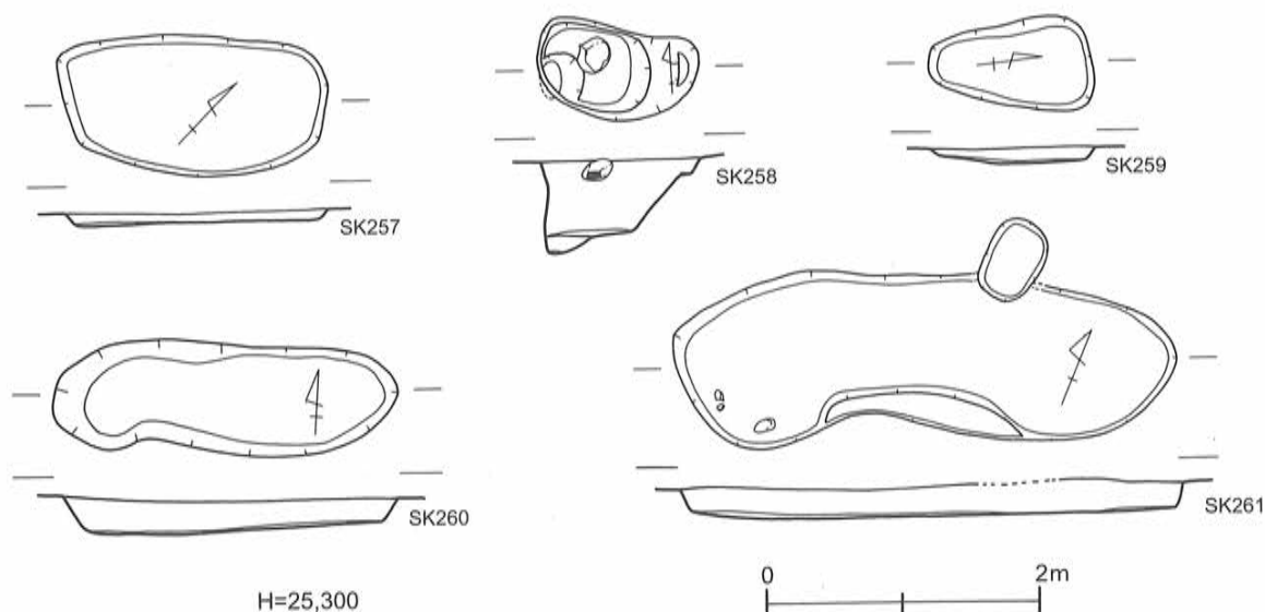
第20図 土壇 (SK257, 261) [1/60]
