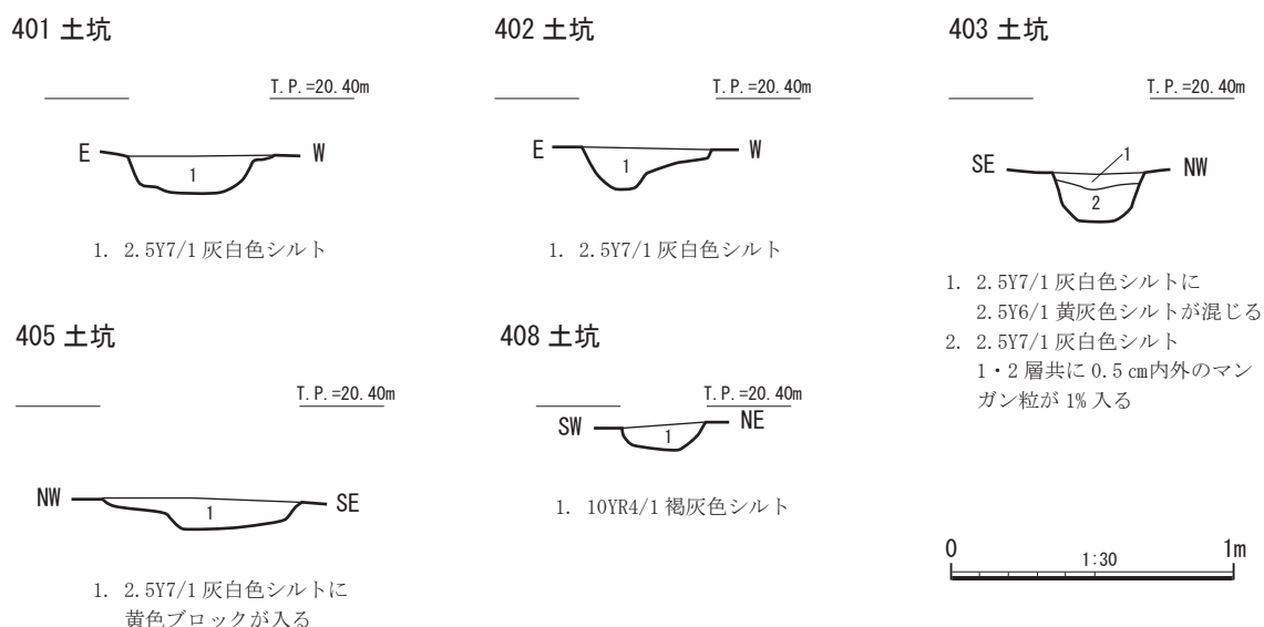
図 15 4 区 401・402・403・405・408 土坑断面土層図
