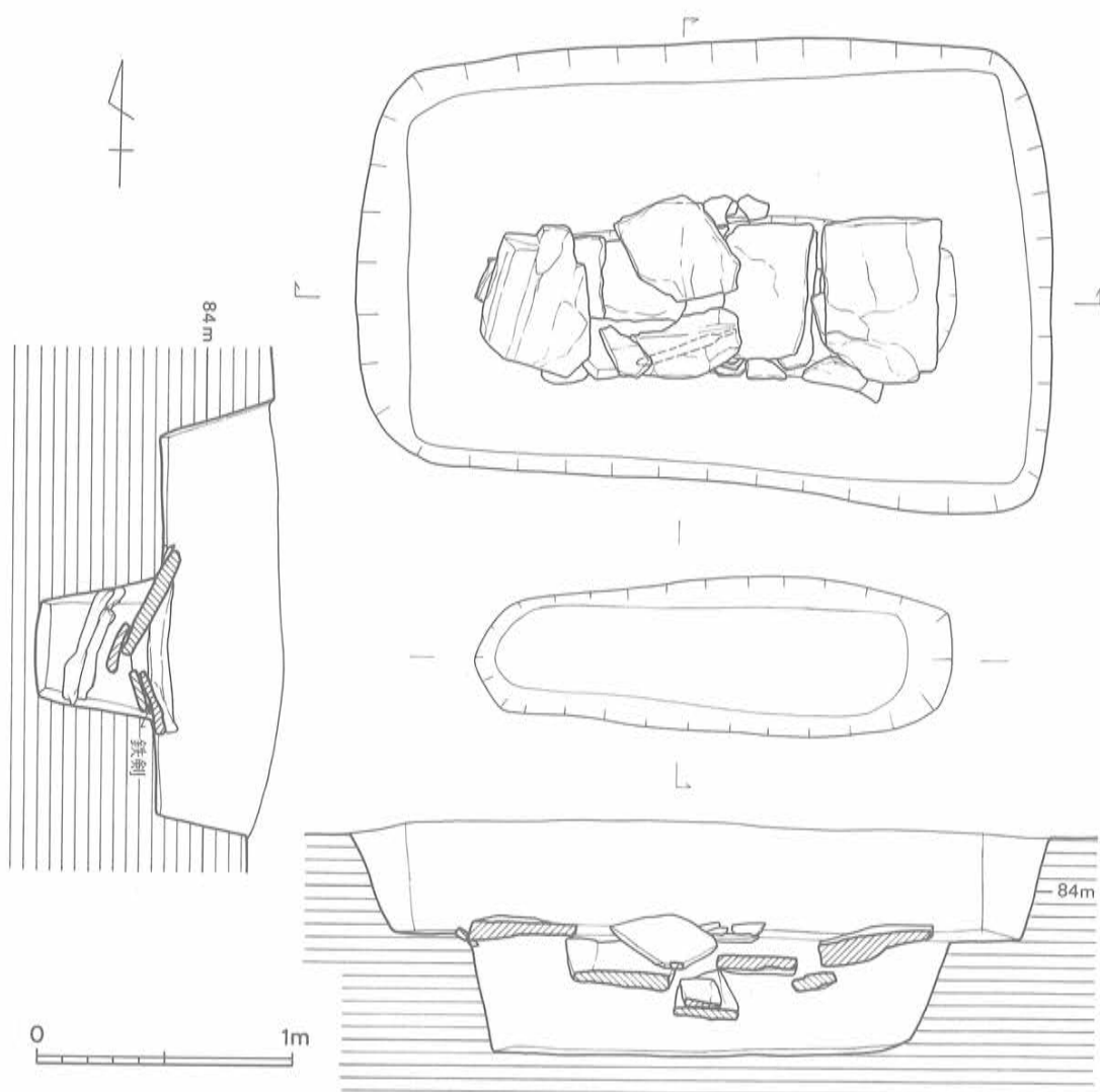
Fig. 157 SC 4号実測図 (1/30)
