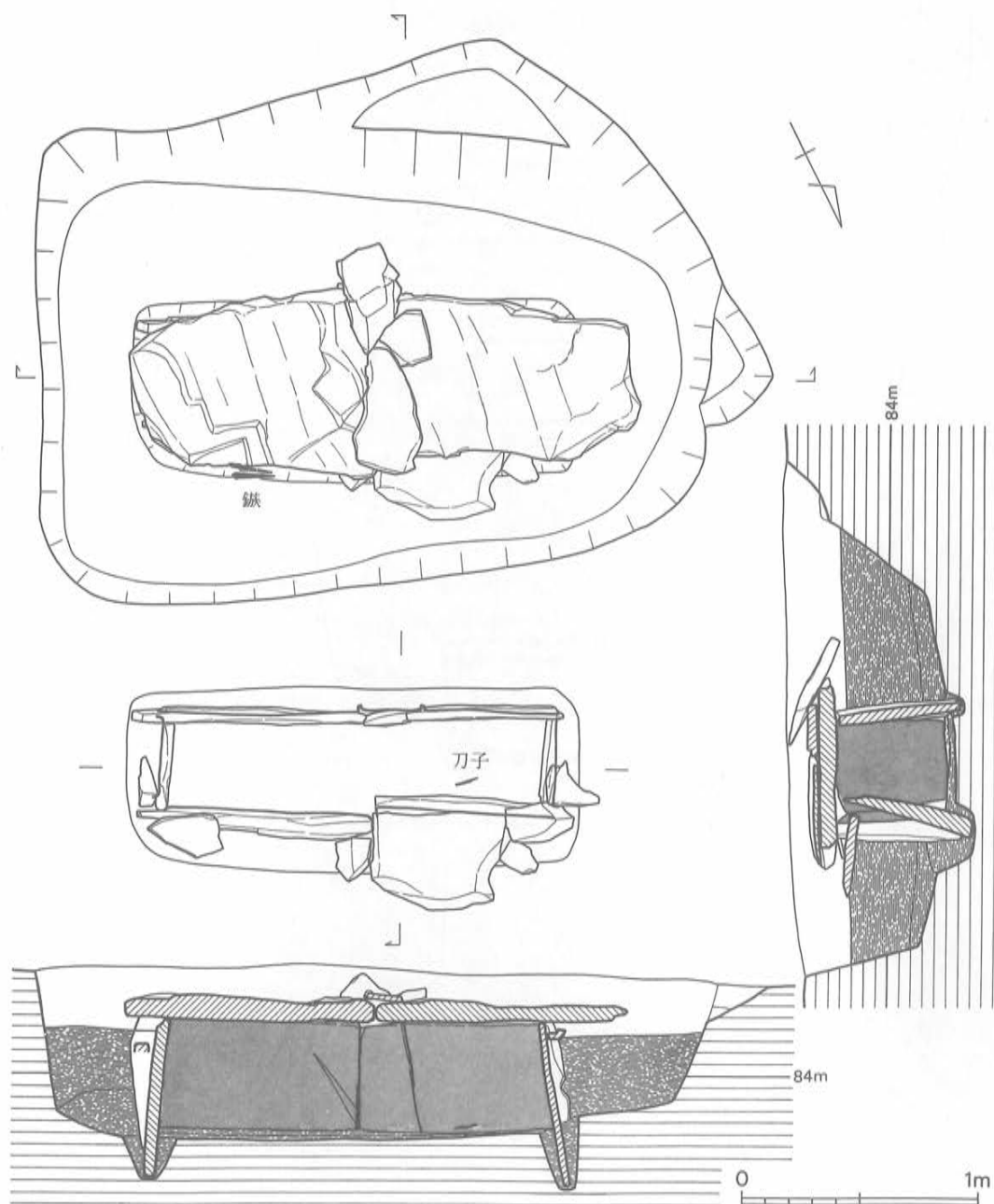
Fig. 137 41号墳主体部実測図 (1/30)
