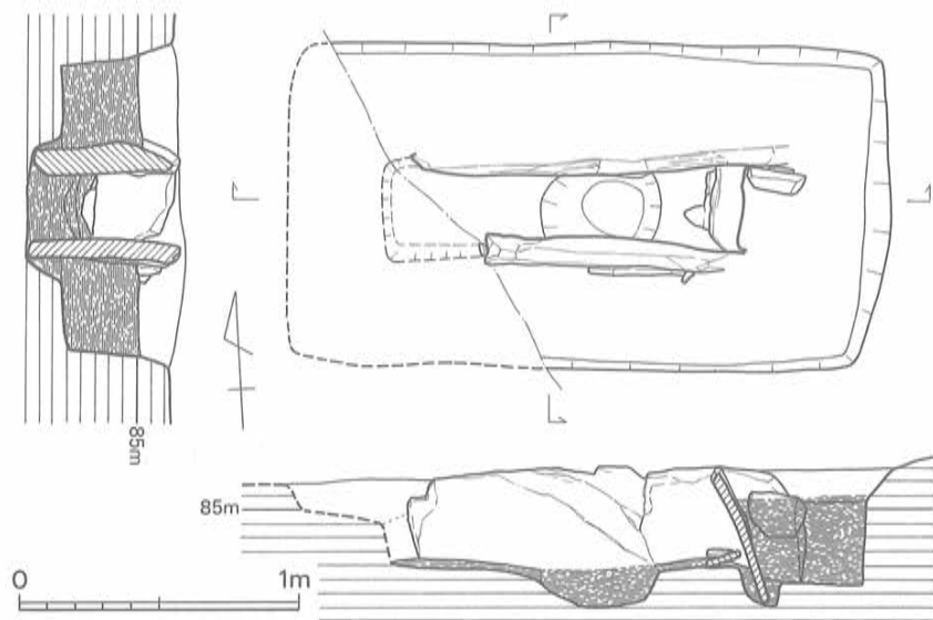
Fig. 116 32号墳主体部実測図 (1/30)
