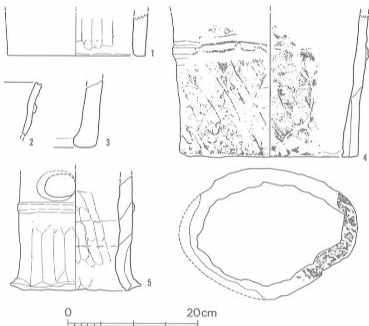
Fig. 64 9号墳出土埴輪実測図 (1/6)
