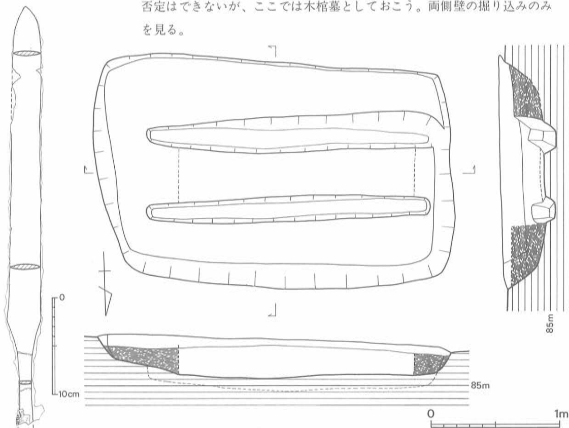
Fig. 159 M1号実測図 (1/30)
