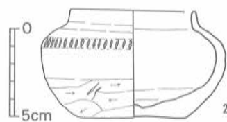
Fig. 59 8号墳付近近世墓埋土中出土土器実測図① (1/3)
