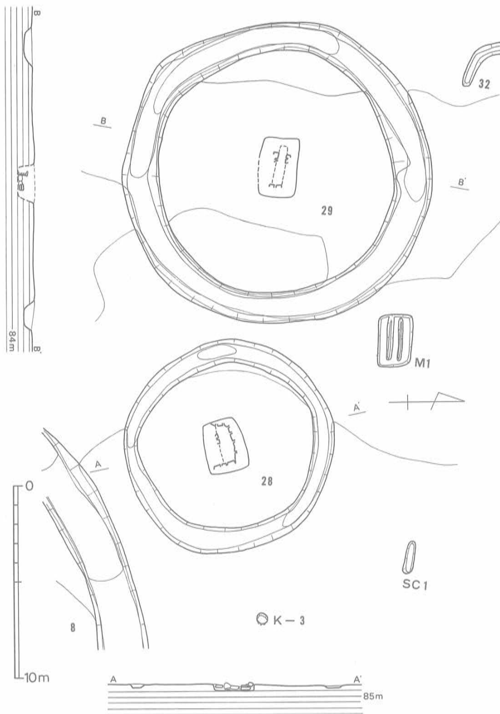
Fig. 103 28·29号墳地形測図 (1/200)
