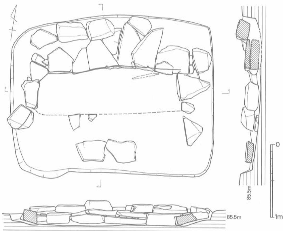
Fig. 104 28号墳主体部実測図 (1/30)
