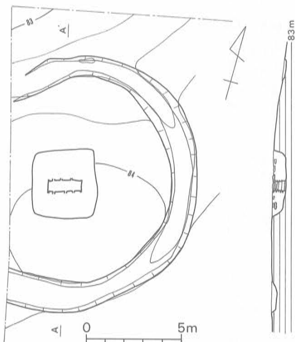
Fig. 141 12号墳地形測量図 (1/200)
