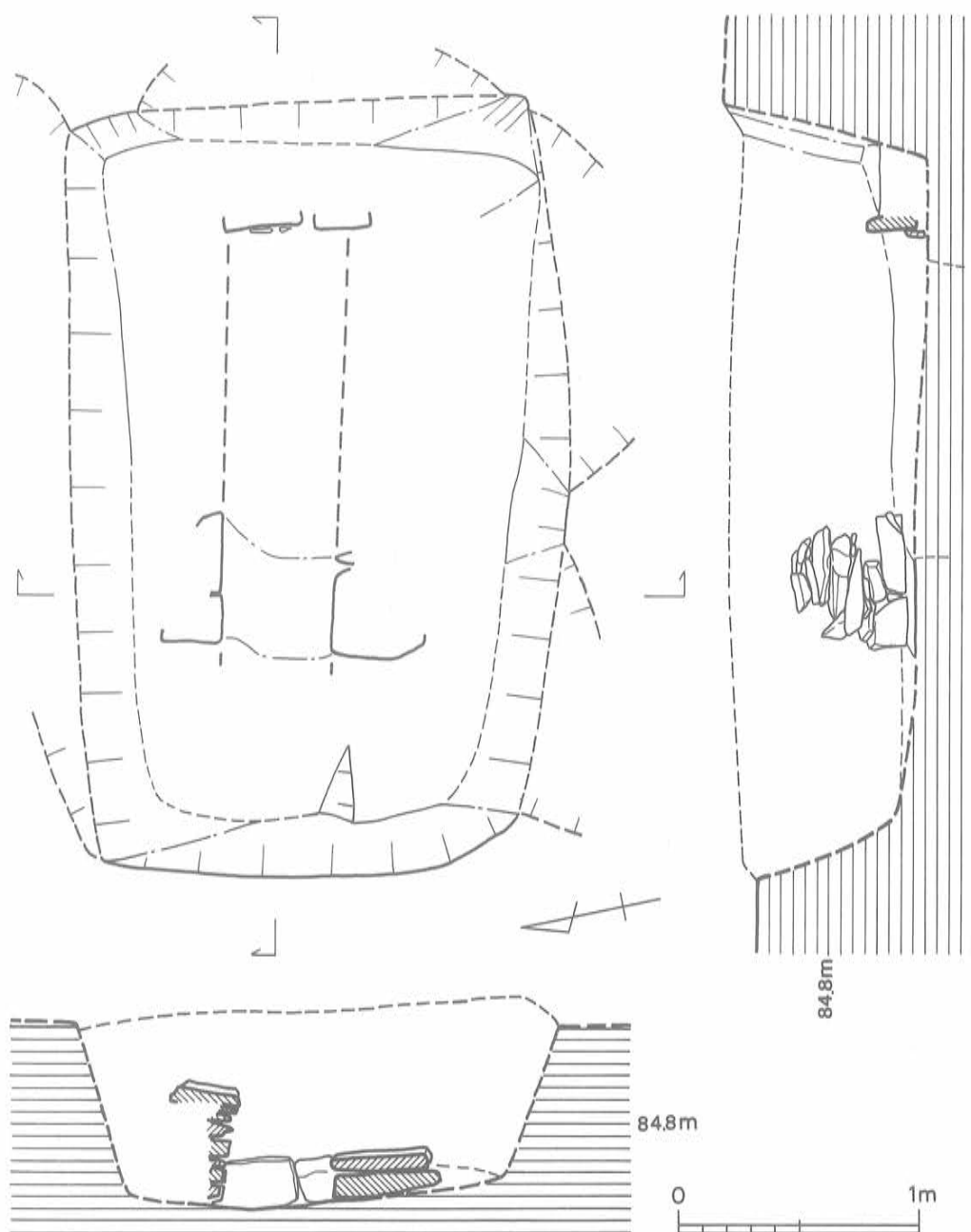
Fig. 107 29号墳主体部実測図 (1/30)
