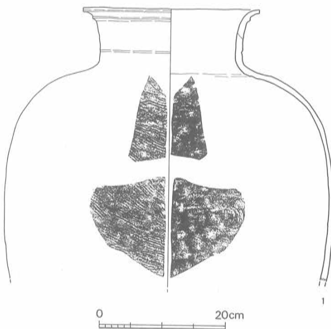
Fig. 82 24号墳出土土器実測図① (1/6)
