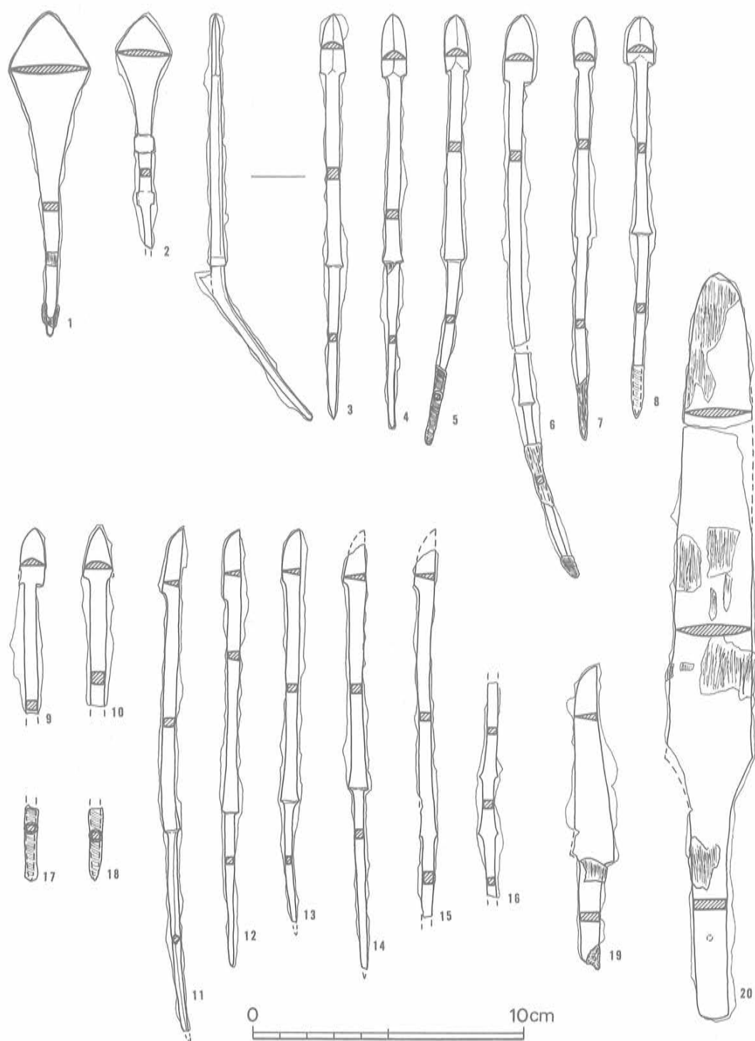
Fig. 92 25号墳出土鉄器実測図① (1/2)
