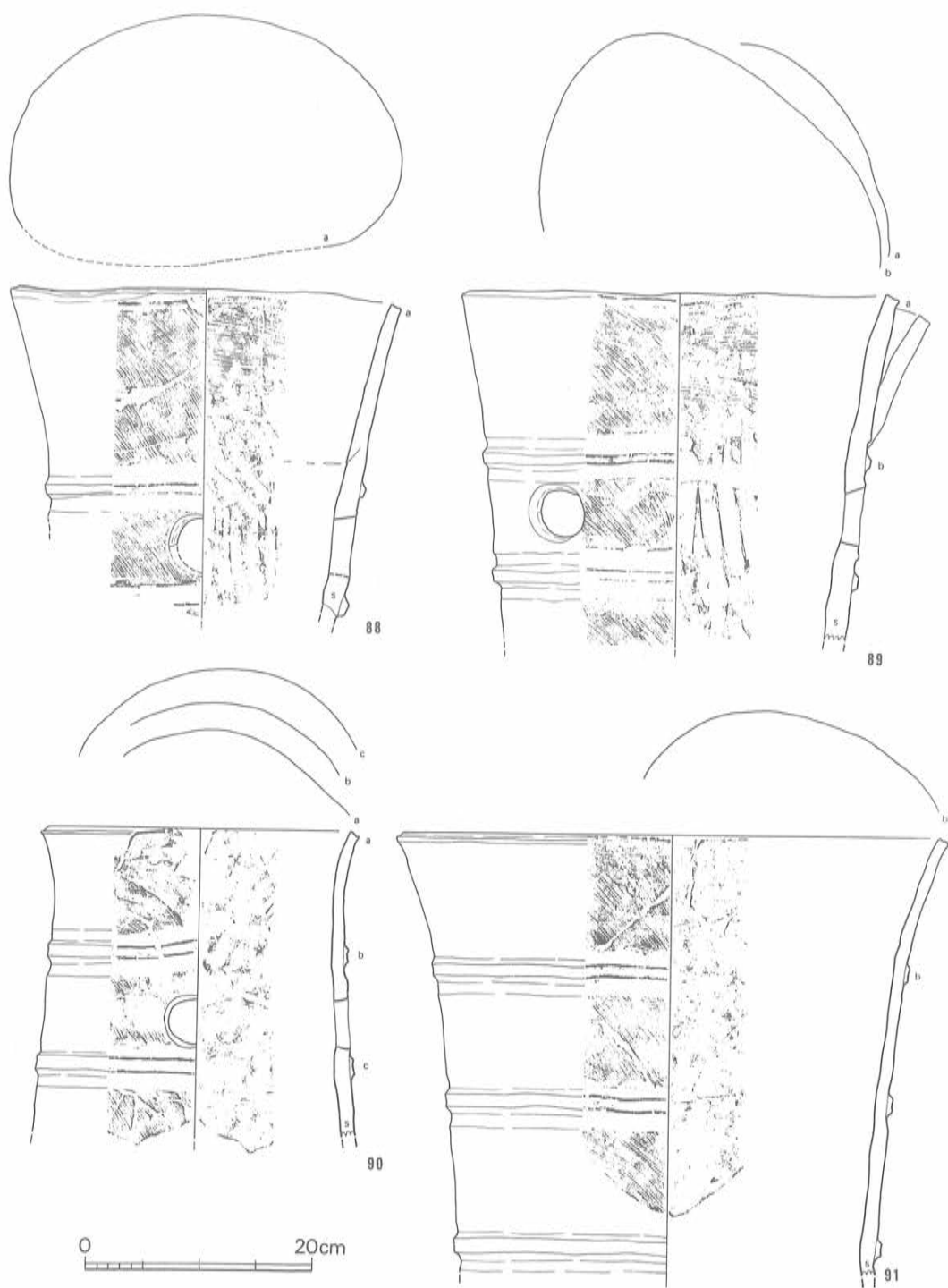
Fig. 43 8号墳出土埴輪（楕円形）実測図⑦（1/6）
