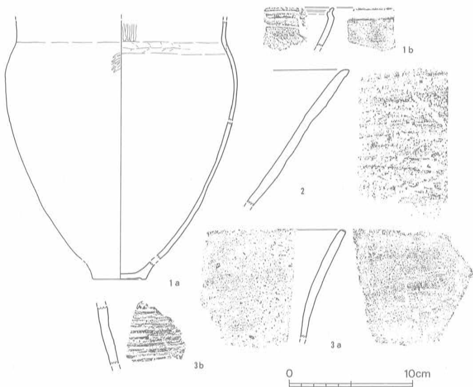
Fig. 173 K-1・2・3 土器実測図 (1/3)
