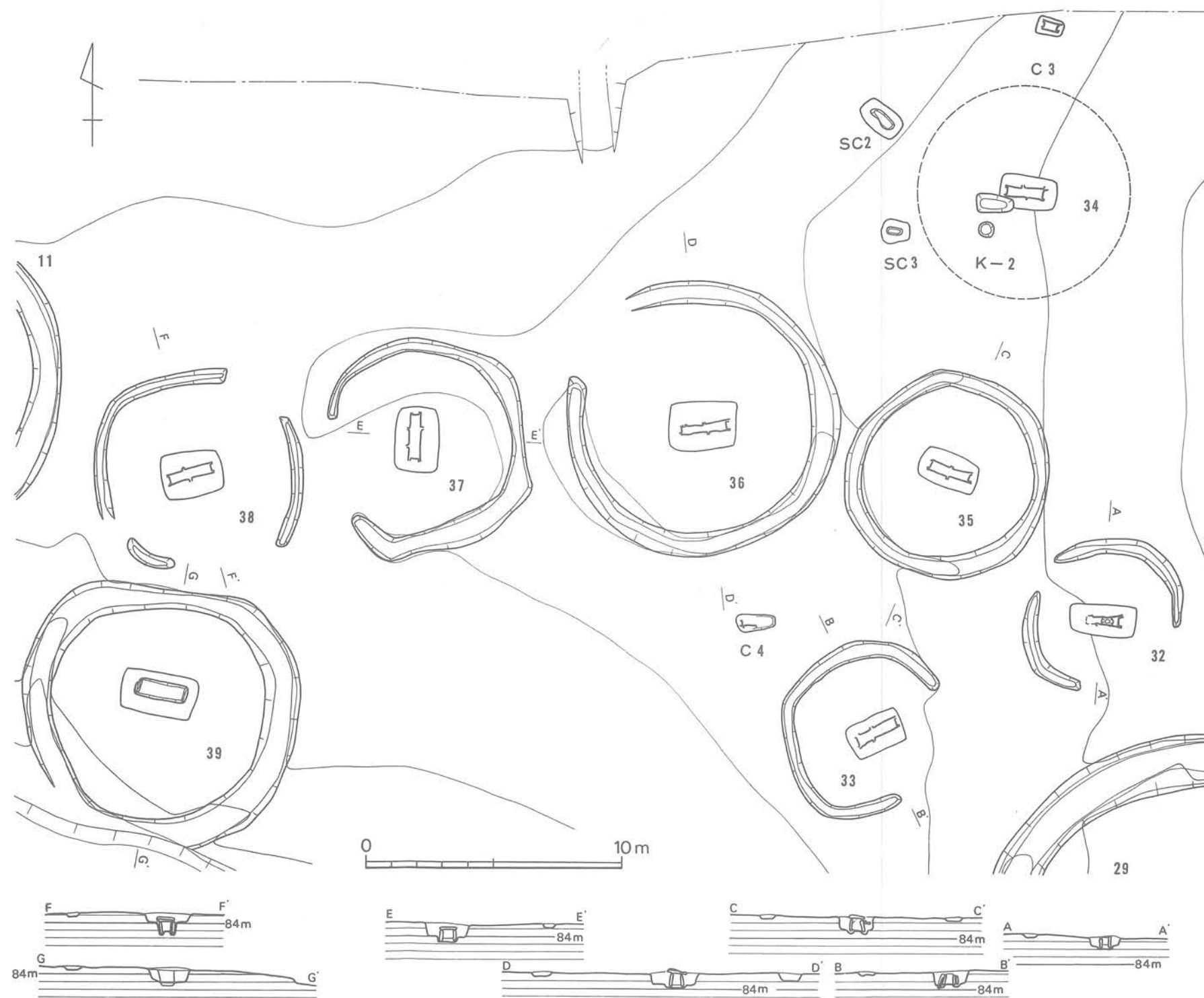
Fig. 115 32~39号墳地形測量図 (1/200)
