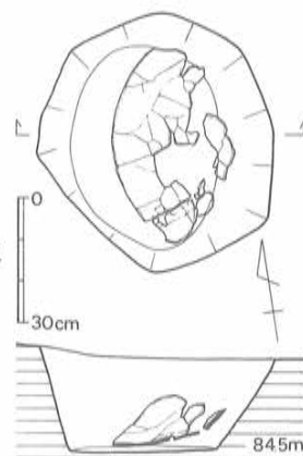
Fig. 171 K-2 実測図 (1/20)
