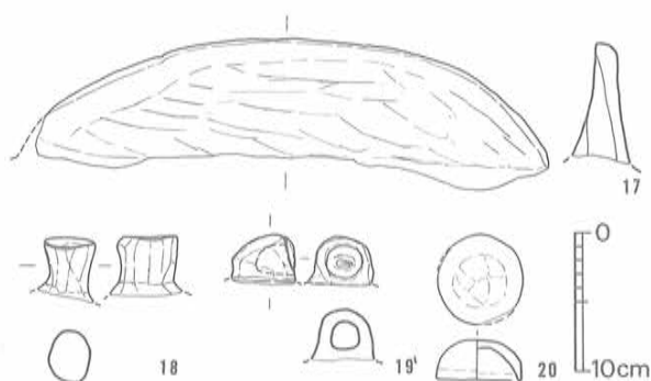
Fig. 49 8号墳出土埴輪（形象）実測図⑬（1/6）
