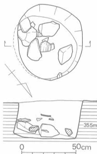
Fig. 172 K-3 実測図 (1/20)
