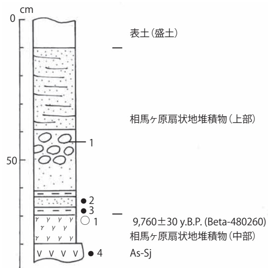
図2 調査区東壁の土層柱状図
