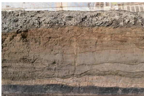
泥流層を陥入する噴砂（南から）
