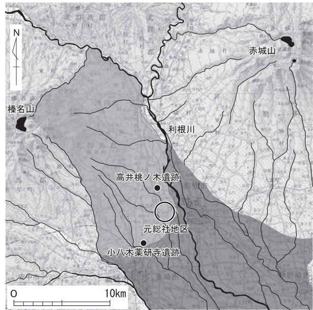
■ : 相馬ヶ原扇状地 ■ : 前橋台地
