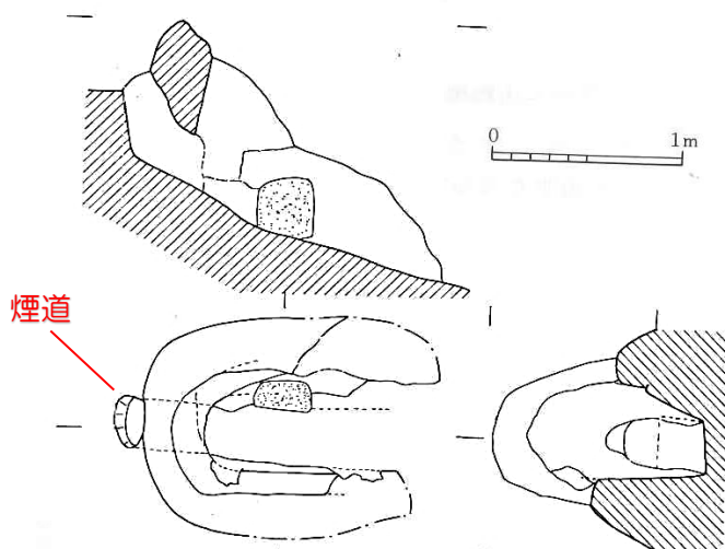
六反製鉄跡の実測図 (松本健郎 1992 より)
