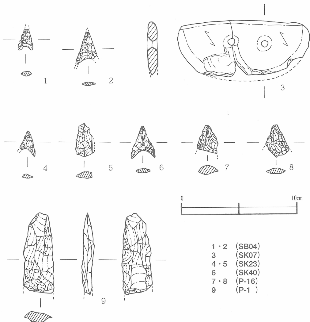
第36図 SB, SK出土石製品 (1/2)
