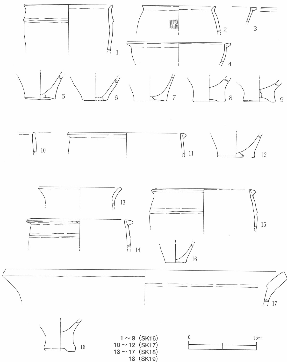
第22図 土壇 (SK16, 17, 18, 19) 出土土器 (1/4)
