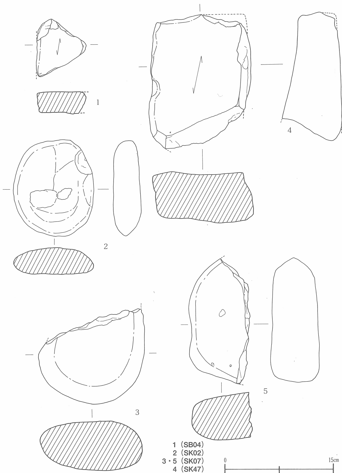
第37図 SB, SK出土石製品 (1/3)
