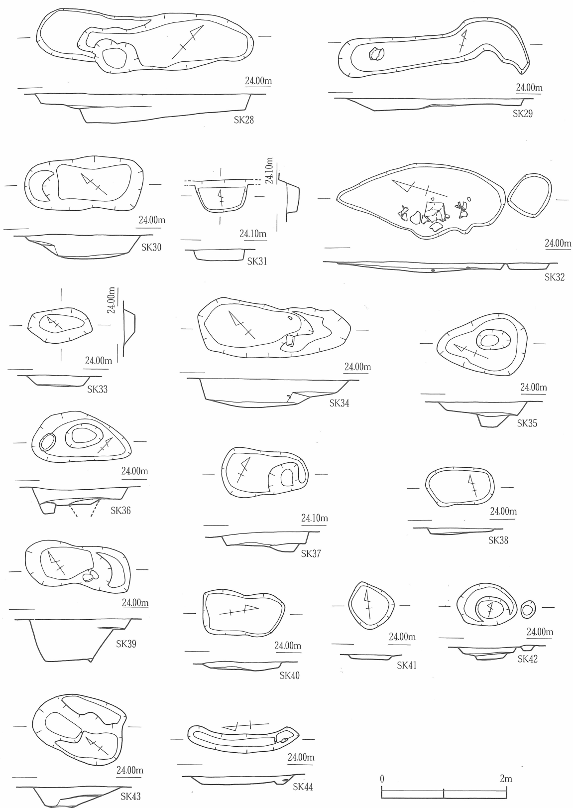
第11図 土坑 (SK28 ~ SK44) (1/60)
