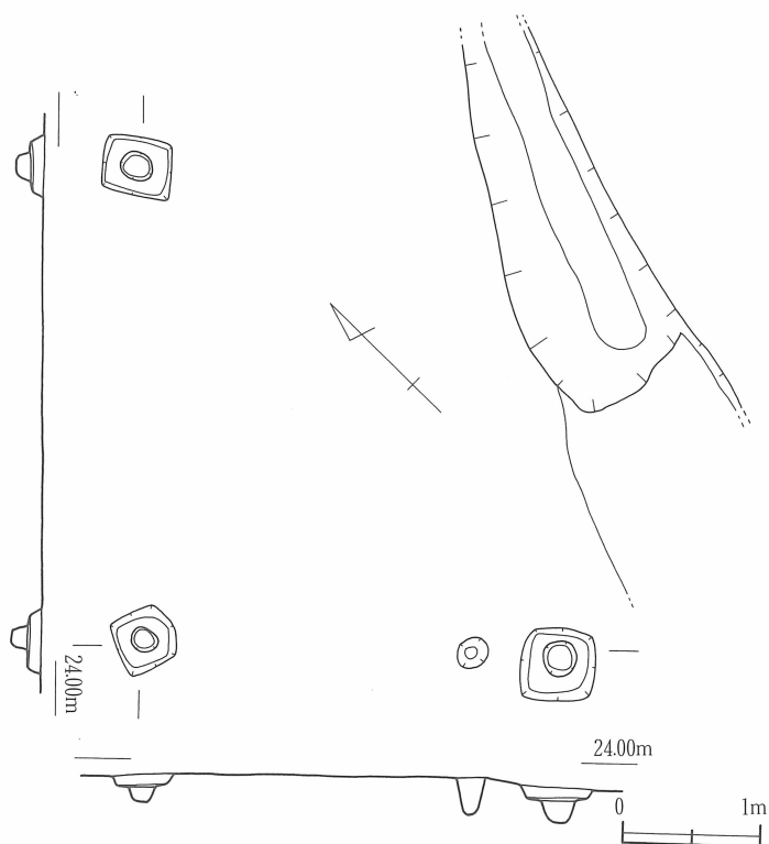
第8図 掘立柱建物 (SB03) (1/60)
