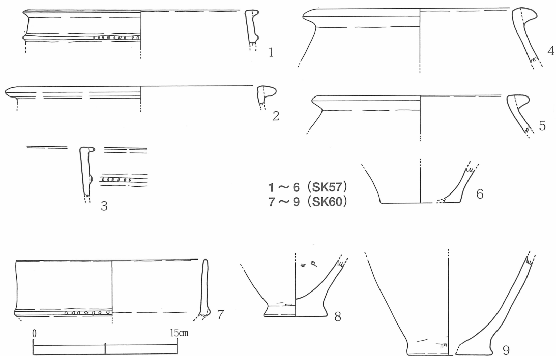
第 31 図 土壙 (SK57, SK60) 出土土器 (1/4)
