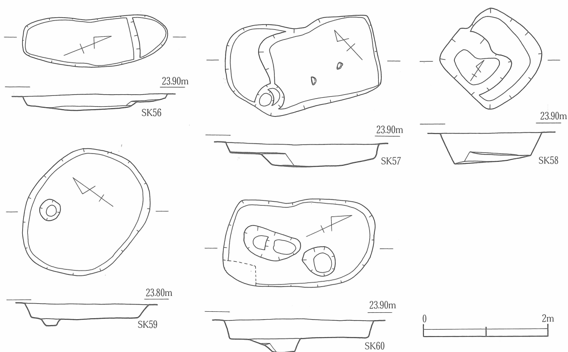
第13図 土坑 (SK56～SK60) (1/60)
