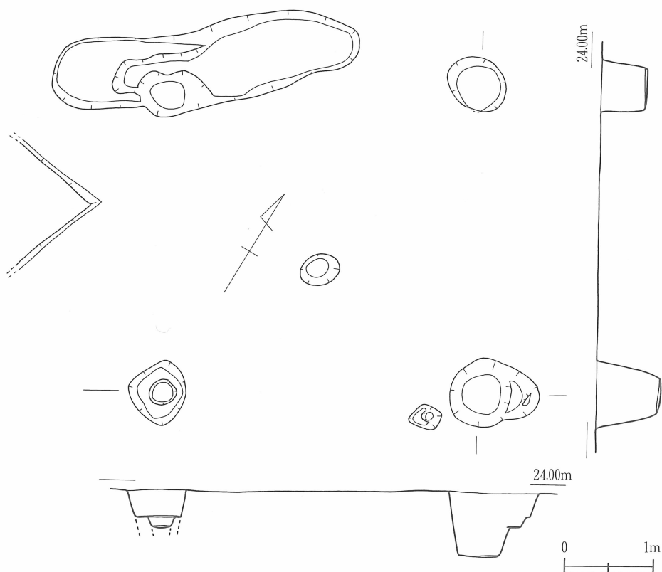
第7図 掘立柱建物 (SB02) (1/60)
