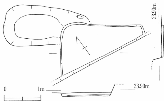
第5図 竪穴住居 (SB01) (1/60)
