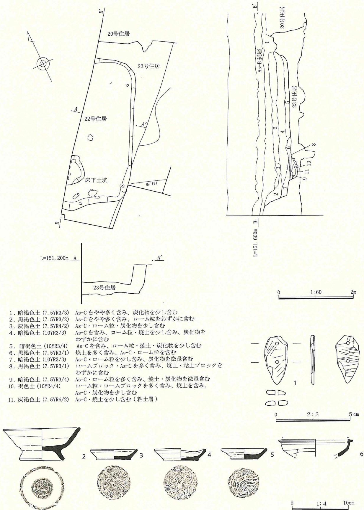
第52図 22号住居平面図・断面図(S=1/60) 出土遺物(S=1/4)
