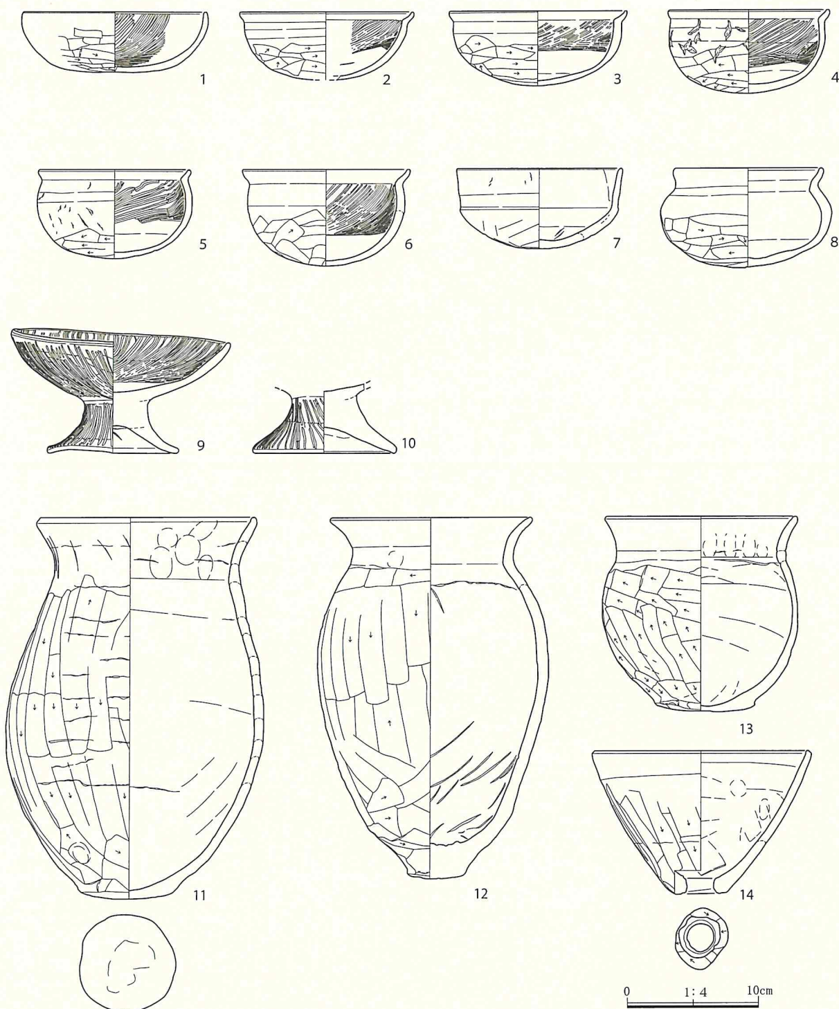
第23図 7号住居出土遺物(S=1/4)
