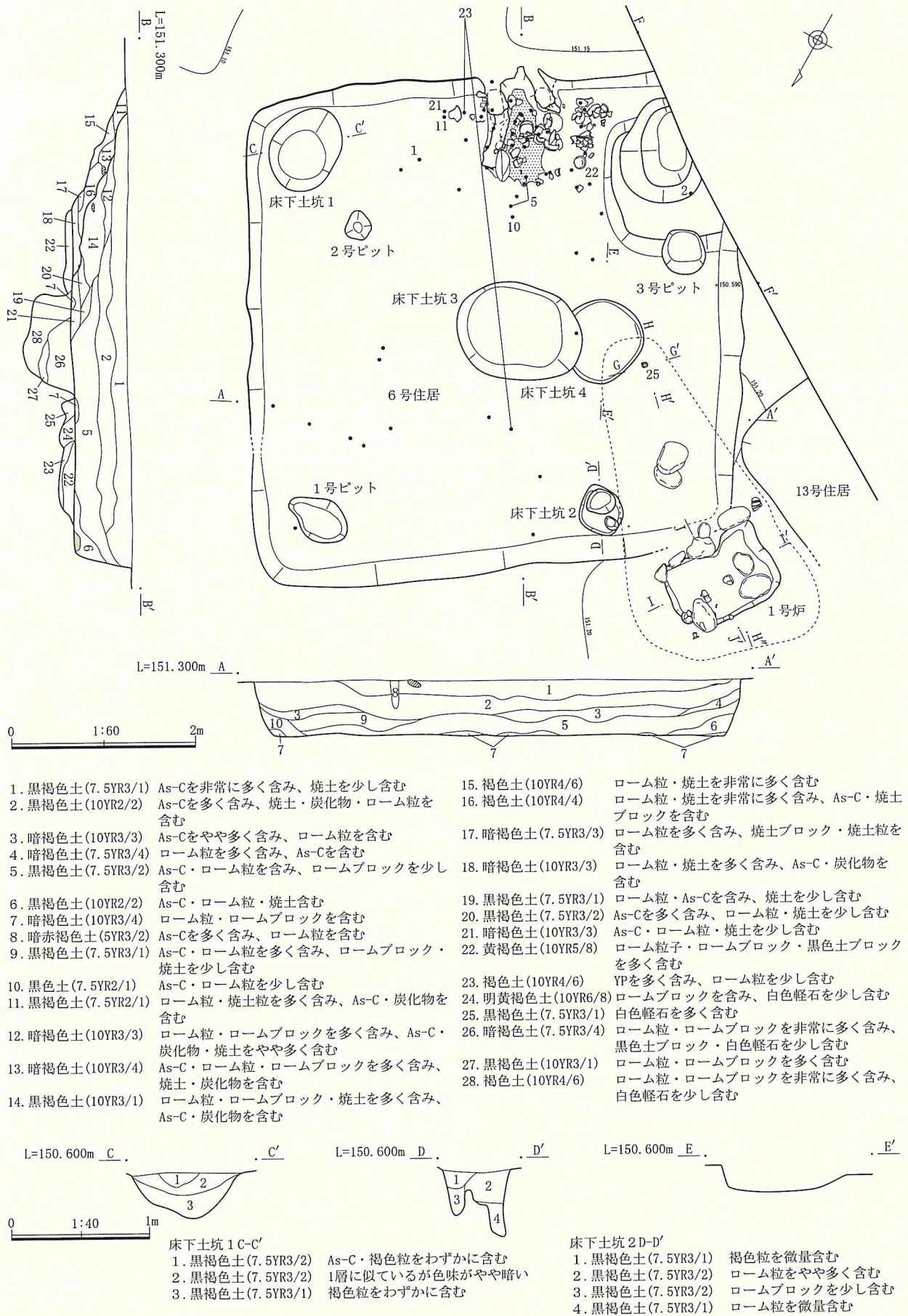
第17図 6号住居 1号炉平面図・断面図(S=1/60) 床下土坑1・2断面図(S=1/40)
