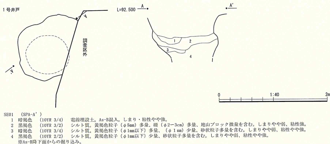
第16図 井戸 平面図・断面図(S=1/40)
