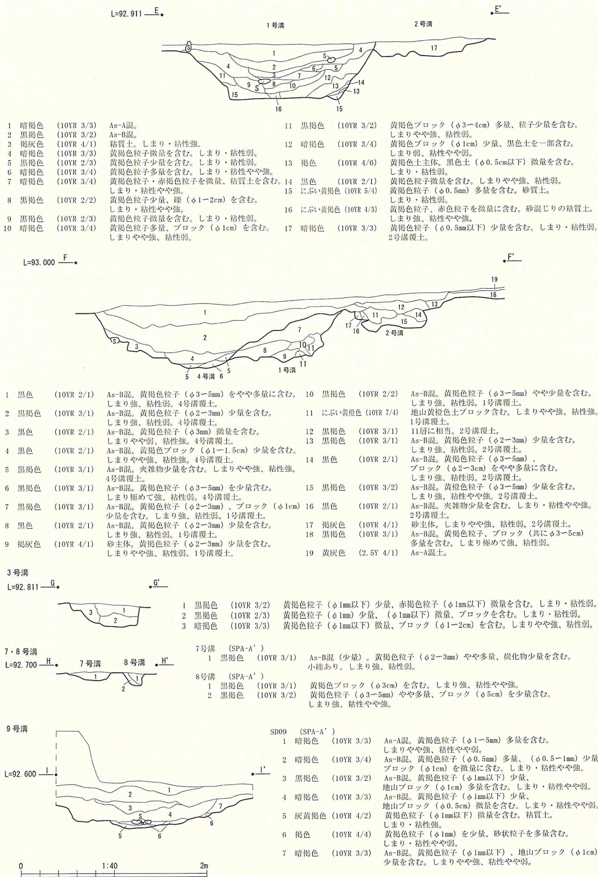
第13図 溝断面図 (S=1/40)
