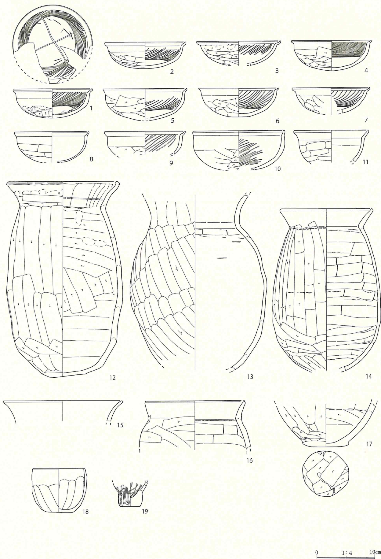
第14図 4号住居出土遺物(S=1/4)
