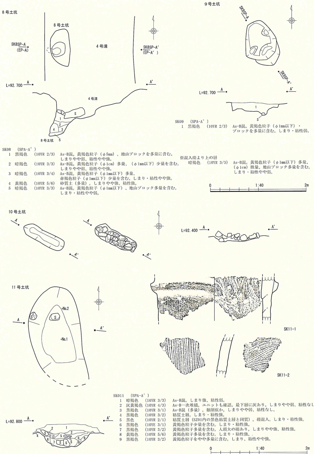
第19図 8～11号土坑 平面図・断面図(S=1/40)・11号土坑出土遺物(S=1/3)
