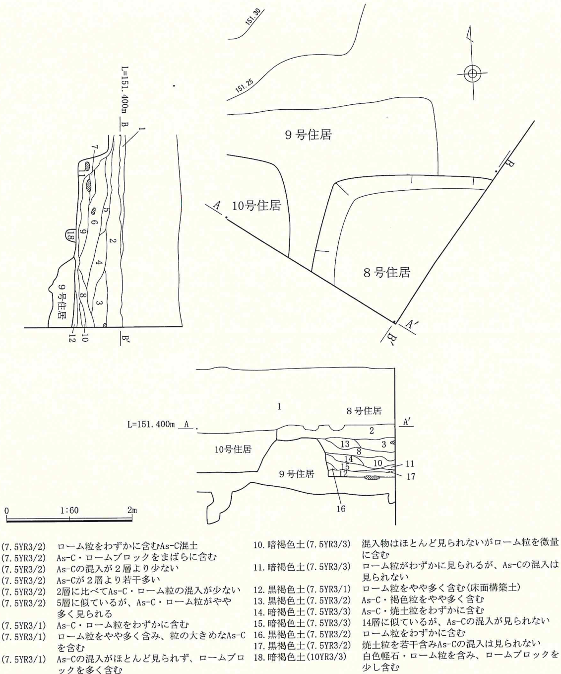
第24図 8号住居平面図・断面図(S=1/60)
