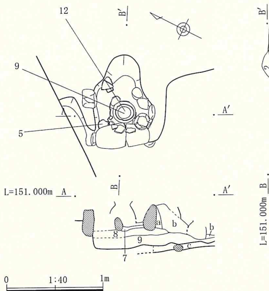
第7図 2号住居平面図・断面図(S= 1/60) カマド平面図・断面図(S=1/40)
