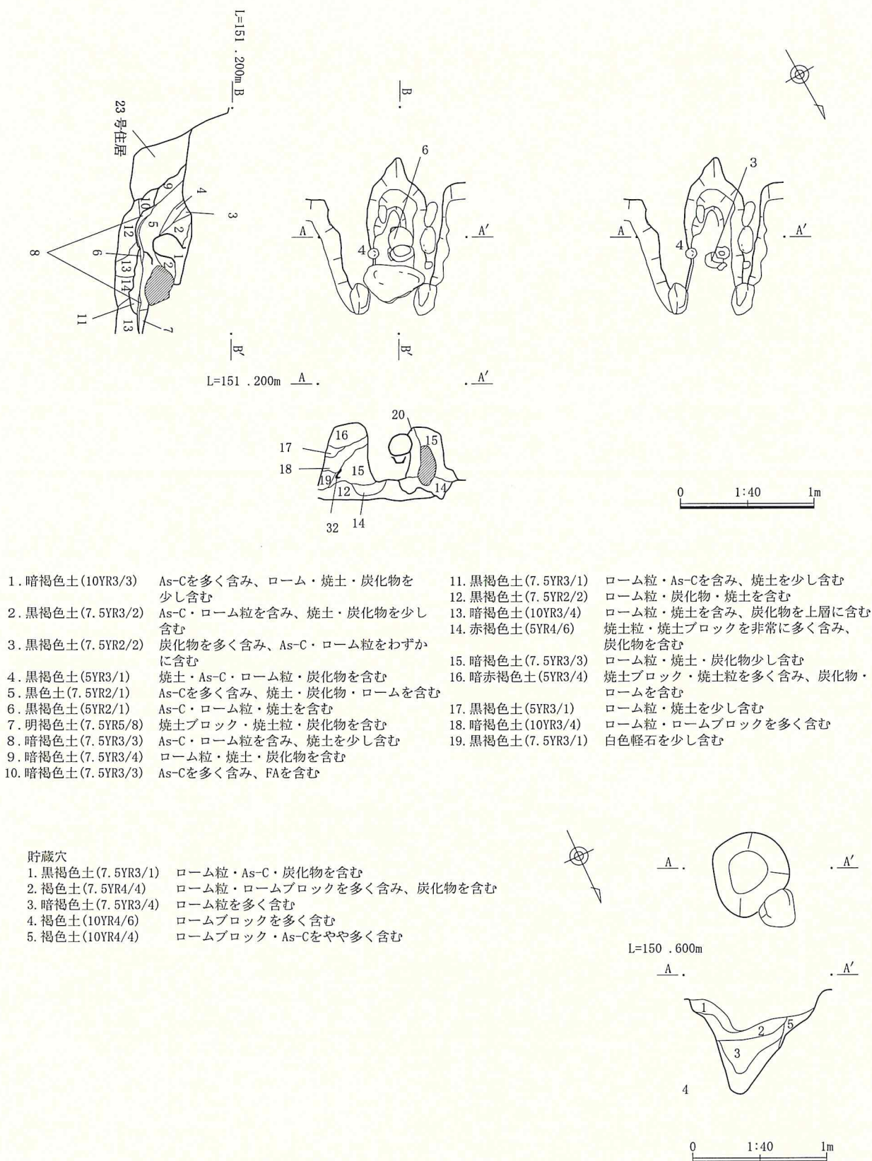
第47図 20号住居カマド・貯蔵穴平面図・断面図(S=1/40)
