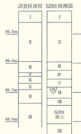
第4図 基本層序(1/40)
