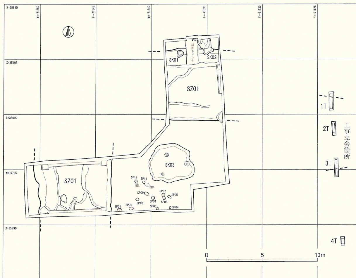
第5図 中居町一丁目遺跡4全体図（1/200）
