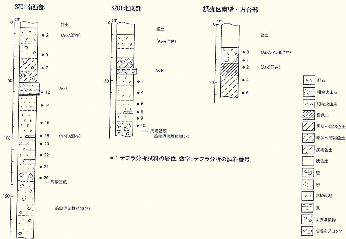
第 11 図 土層柱状図
