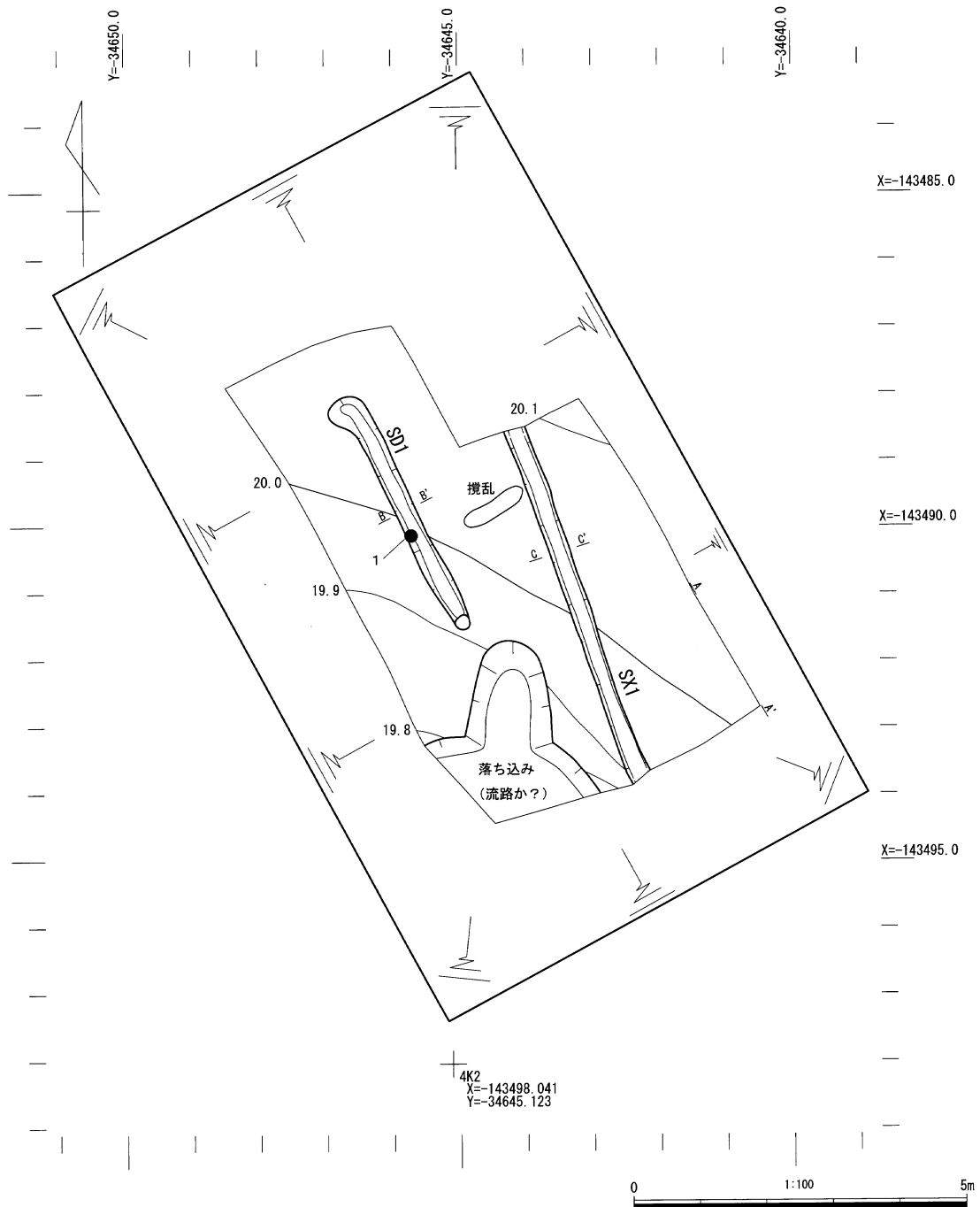
第5図 子ヶ崎遺跡遺構全体図
