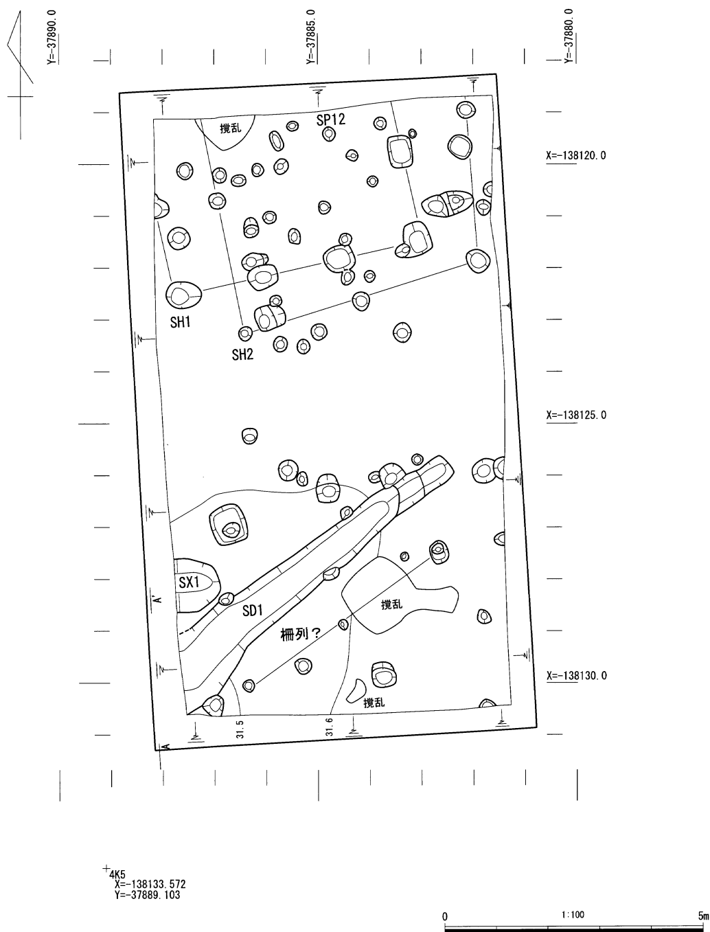
第 11 図 鹿島・打上遺跡遺構全体図
