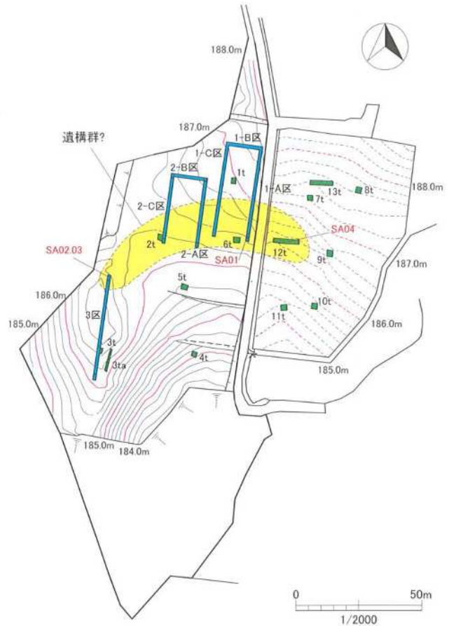
図3 調査区・トレンチ・遺構配置
